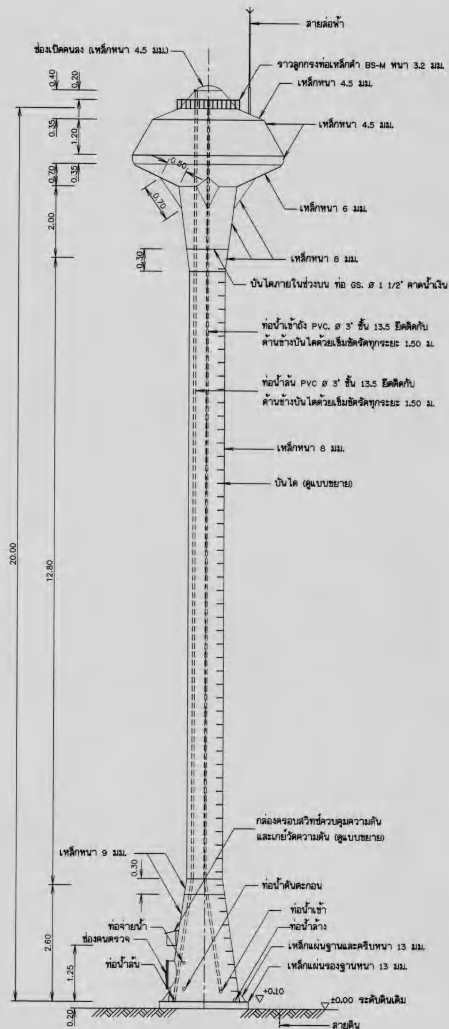
รูปด้านข้างหอถังสูง แบบถังเหล็กรูปทรงแปมแปญ
