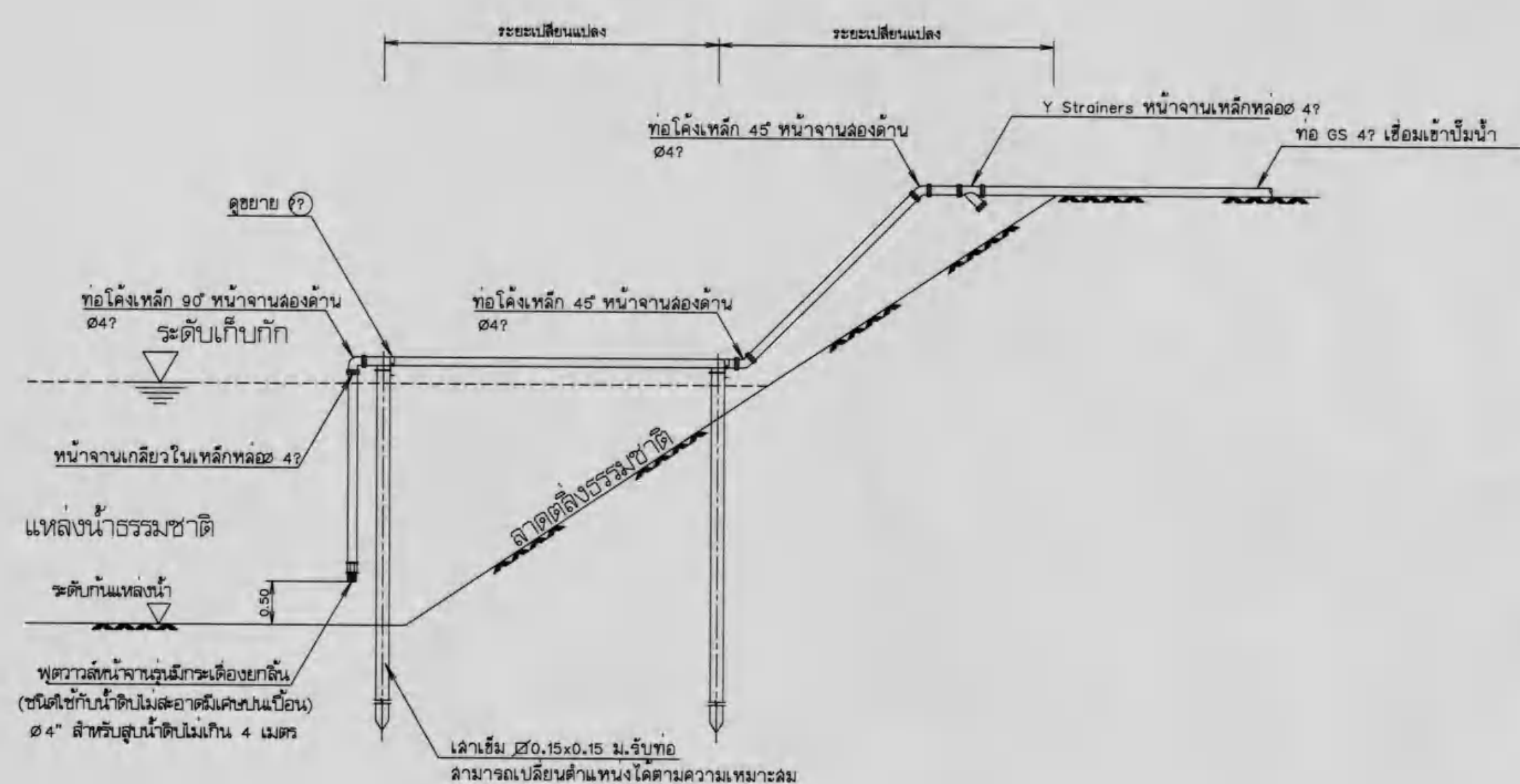
แบบขยายการเดินท่อจากแหล่งน้ำดิบ
