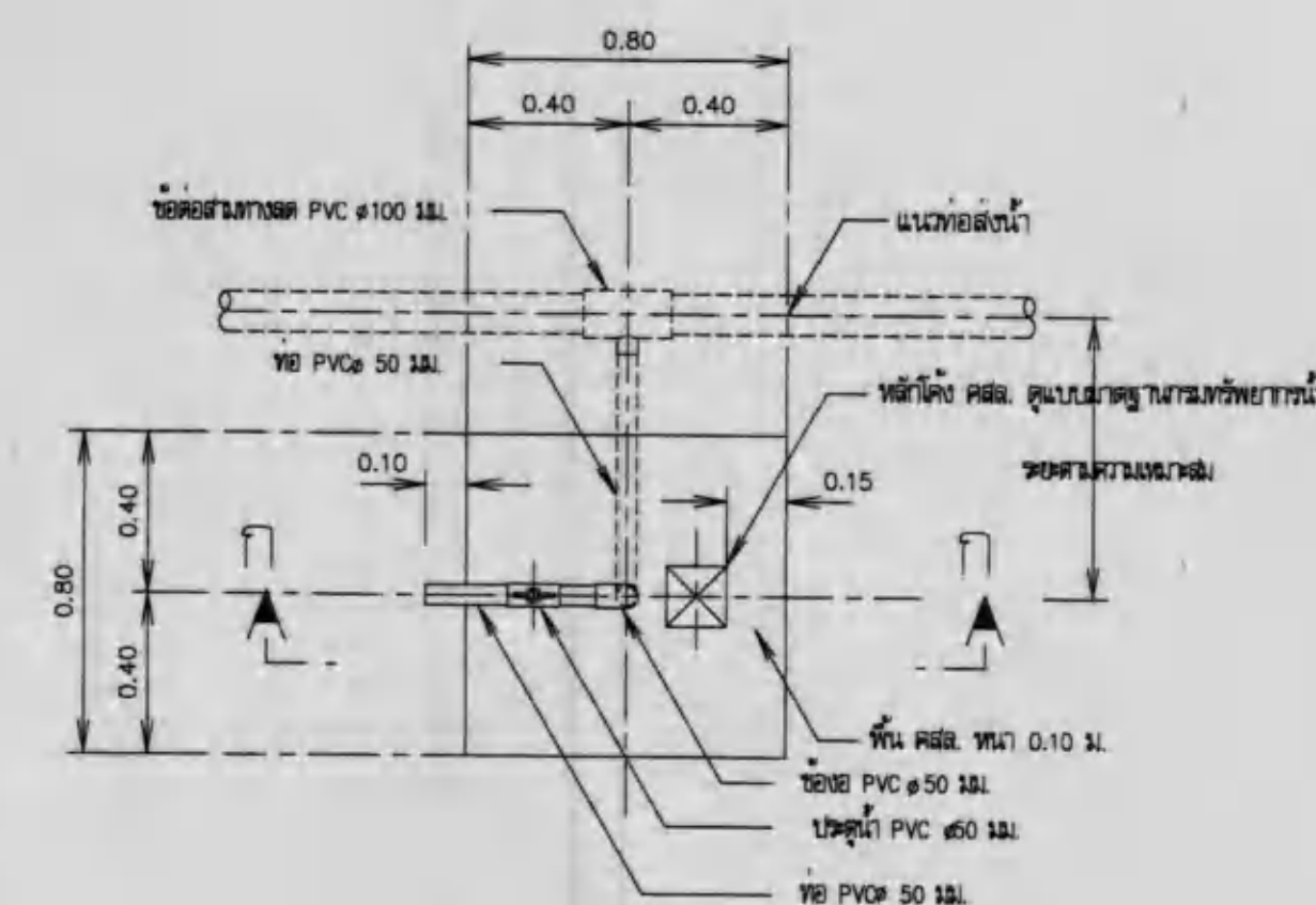
แปลนอาคารจุดปล่อยน้ำ
