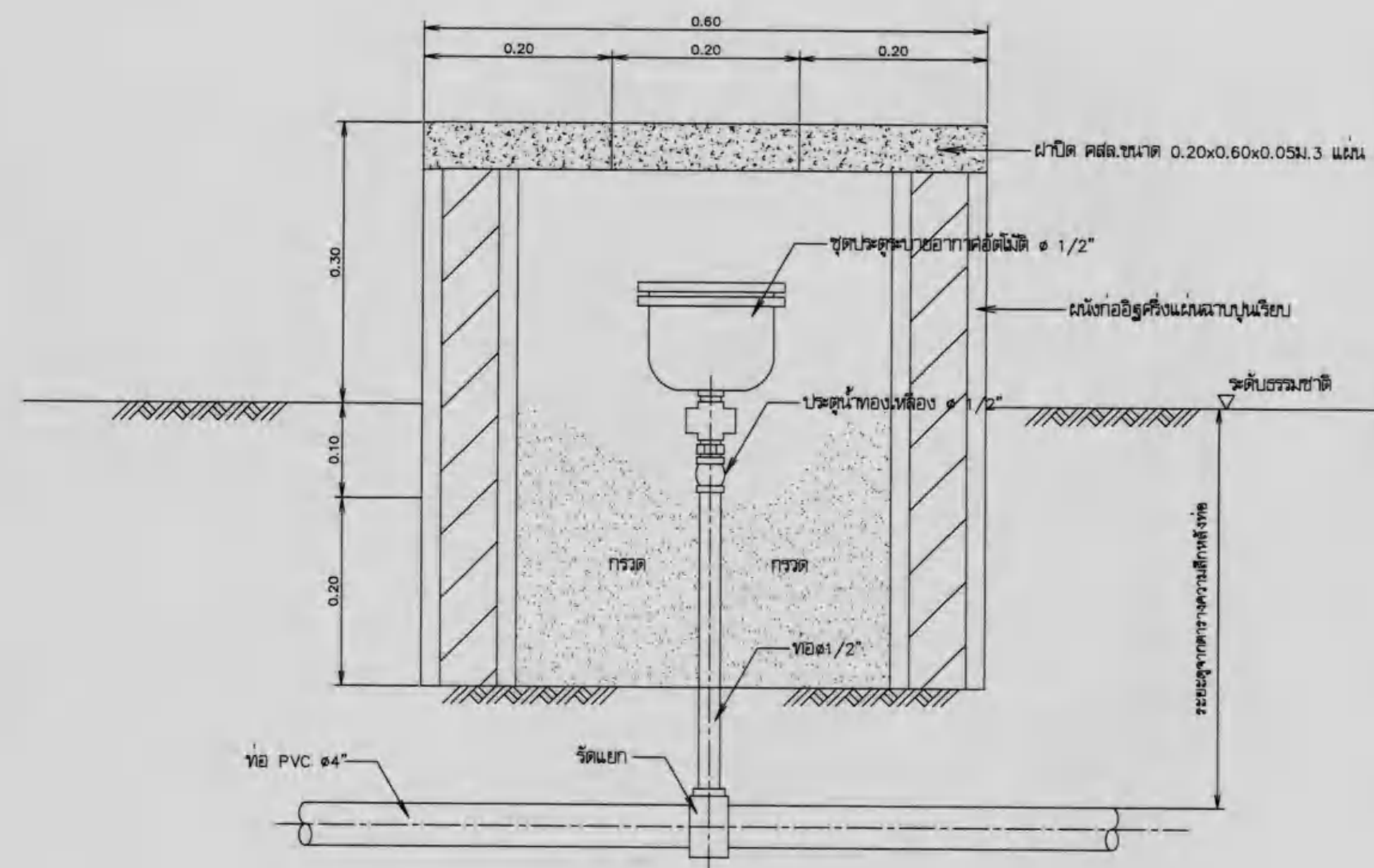
การติดตั้งประตูปรับอากาศอัตโนมัติ
