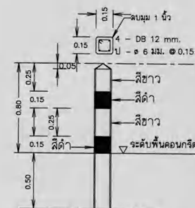
แบบขยายหลักกับกบแนว
