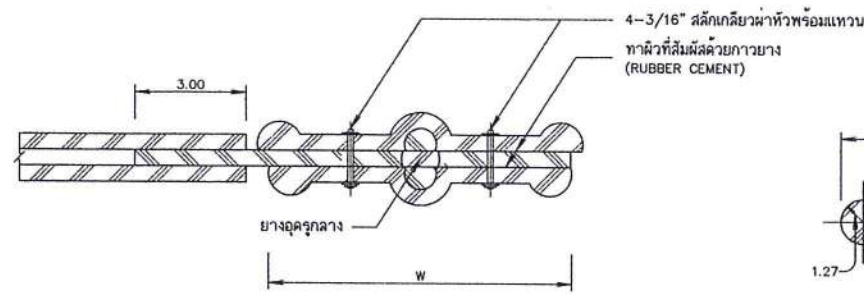
รูปตัด ก-ง ไม่แสดงมาตราส่วน
