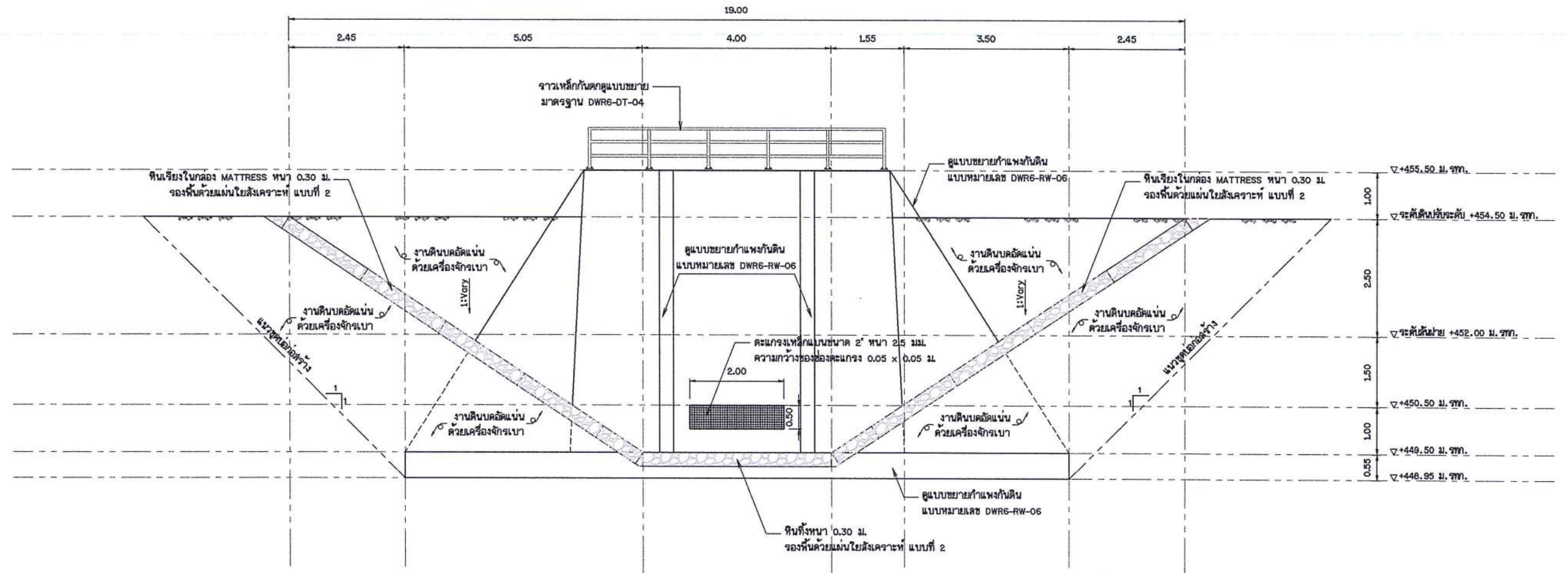
รูปตัดแนว ก - ก ไม่แสดงมาตราส่วน
