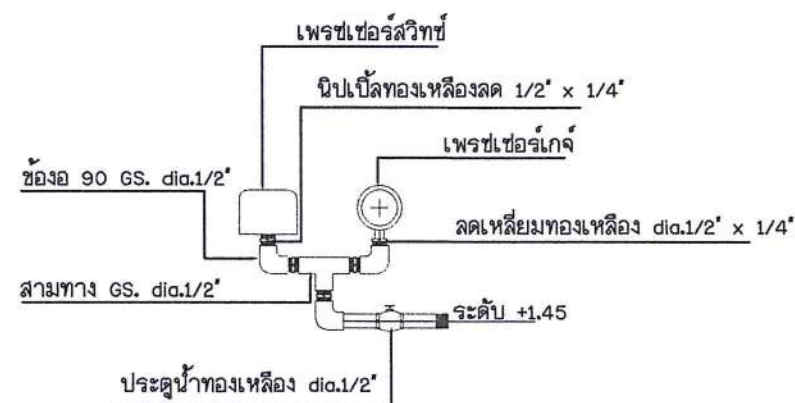
แบบขยายสิทธิ์ควบคุมและเก็้วัดความดัน
