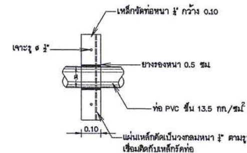
รูปขยาย "4"
