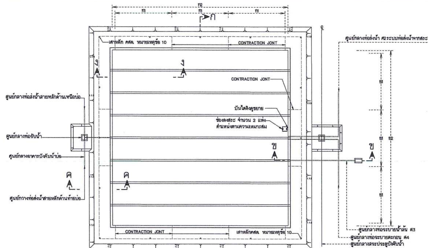
แปลนสระเก็บน้ำ มาตราส่วน 1:200
