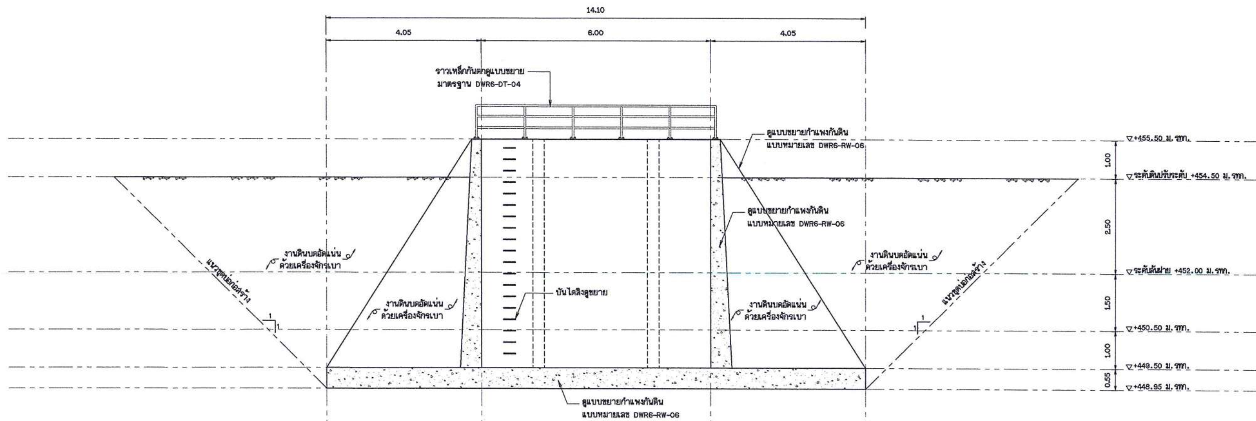
รูปตัดแนว ข - ข ไม่แสดงมาตราส่วน
