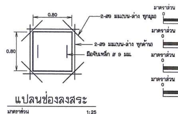
แปลนช่องลงสระ
