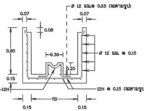
เหล็กเสริมบ่อประจุน้ำ
