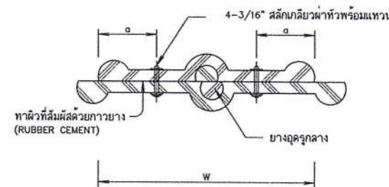
รูปตัด ก-ค ไม่แสดงมาตราส่วน
