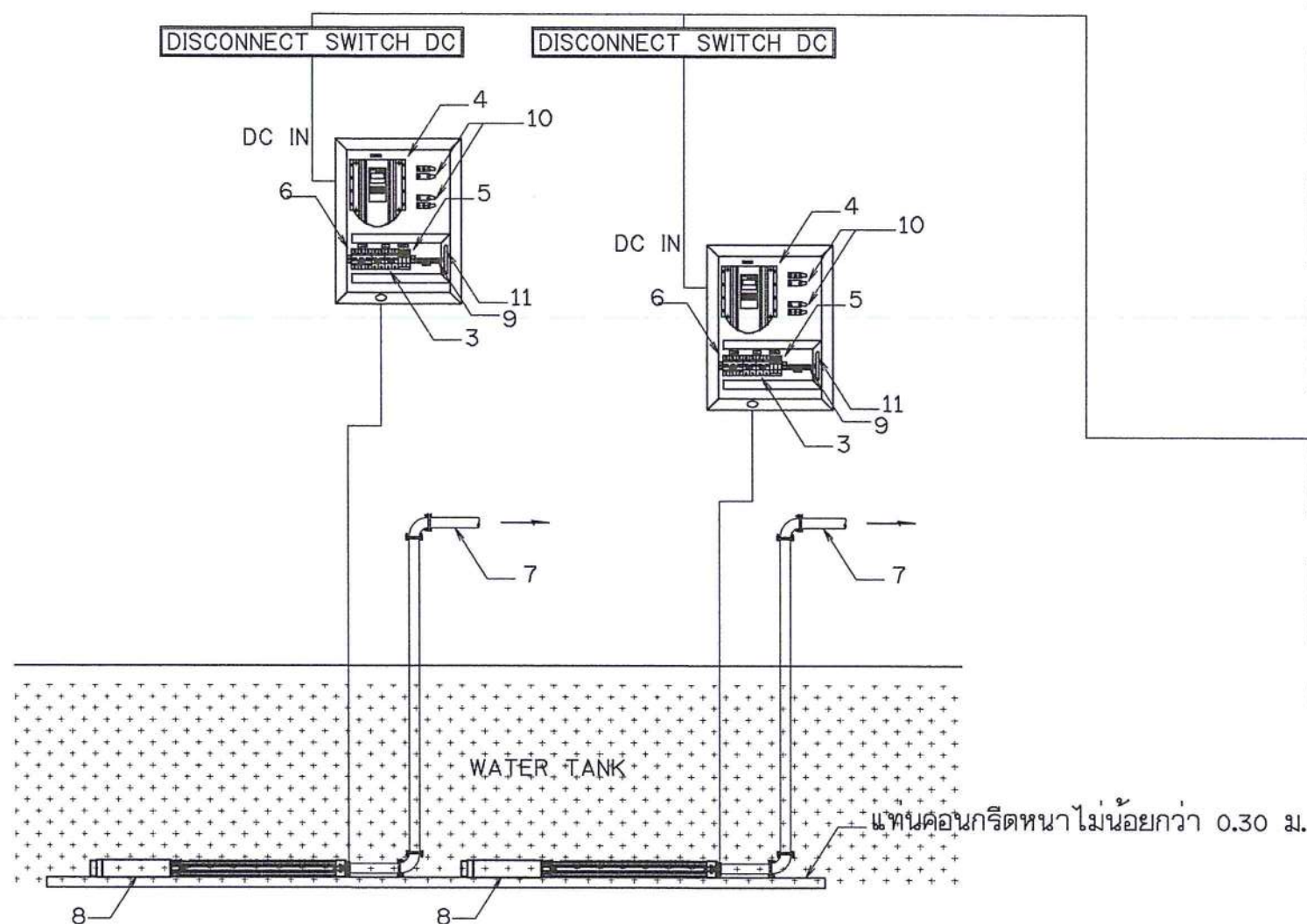
แบบระบบกระจายน้ำด้วยพลังงานแสงอาทิตย์ มาตรฐาน ไม่แสดงมาตรฐาน
