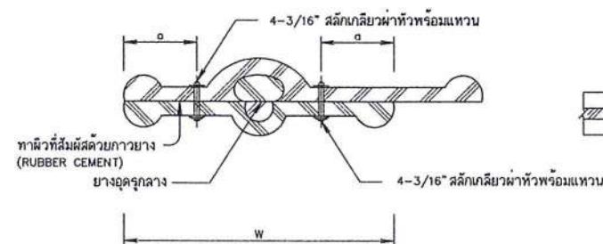
รูปตัด ก-ข ไม่แสดงมาตราส่วน
