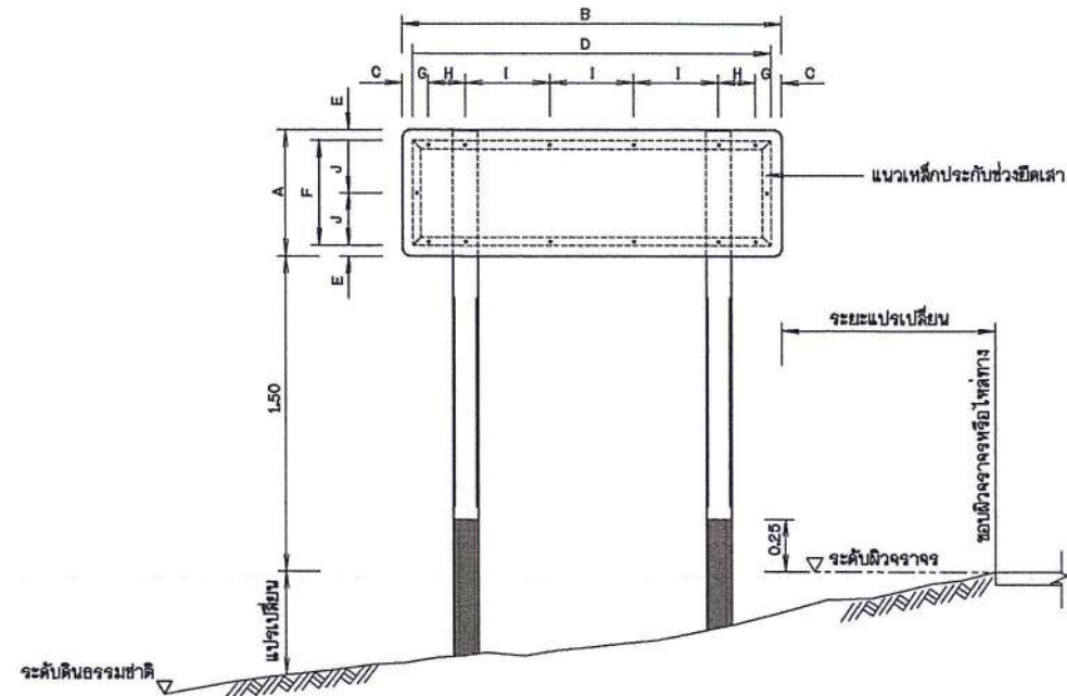
รูปแสดงการประกอบแผ่นป้าย มาตรฐาน 1:20
