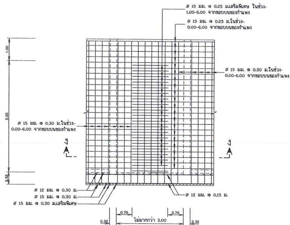
รูปตัดตามยาวของกำแพงบานไม้ตีดิน
