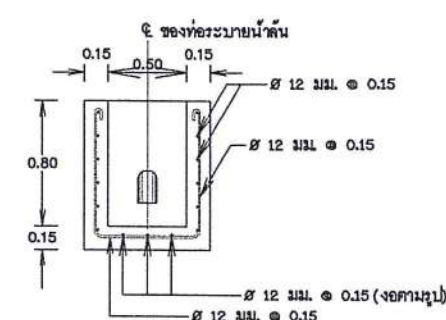
รูปตัดแนว 1 - 1
