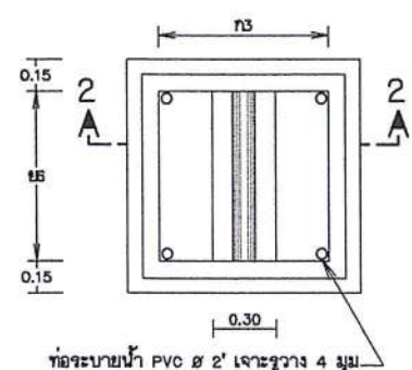
แปลนบ่อประจุบึงค้ำน้ำ
