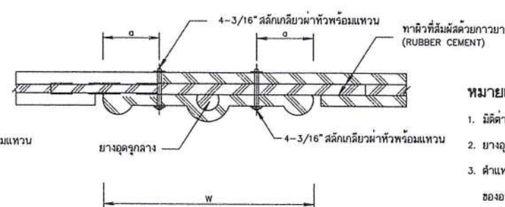
รูปตัด ก-จ ไม่แสดงมาตราส่วน
