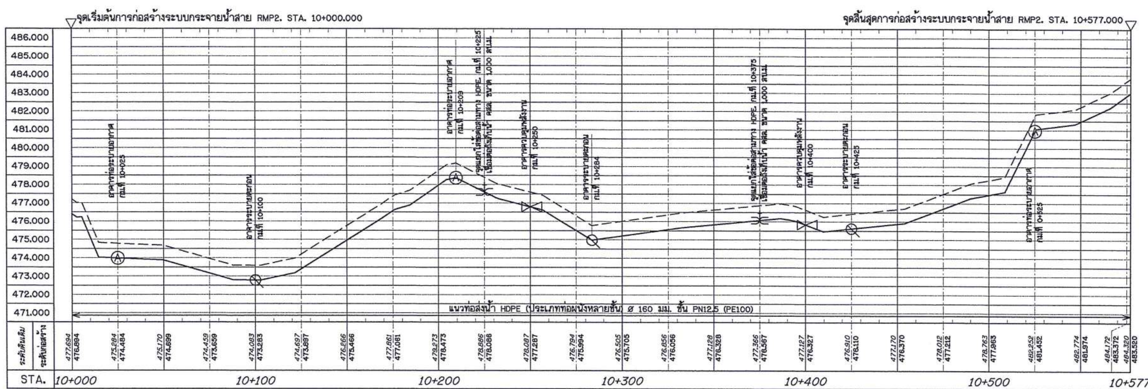
รูปตัดตามแนวยาว มาตราส่วน 1:500 แนวยาว 1:1,000
