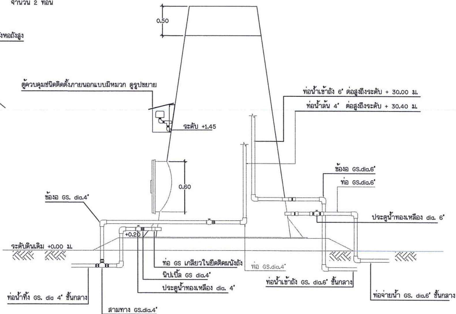
แบบแสดงการเดินท่อในถังผสมปูน ไม่แสดงมาตราส่วน
