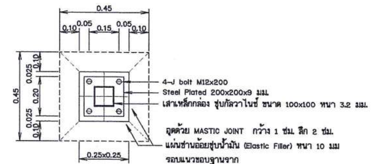
รูปตัด ก-ก
