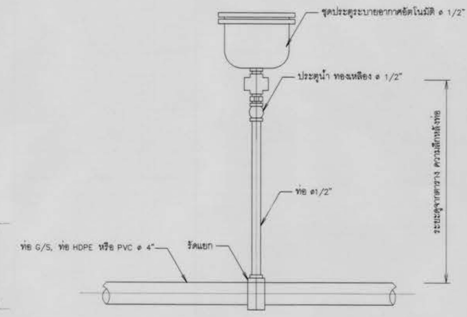
12. การติดตั้งประตูละบายอากาศอัดโนมิตี ไม่แสดงขนาดราส่วน
