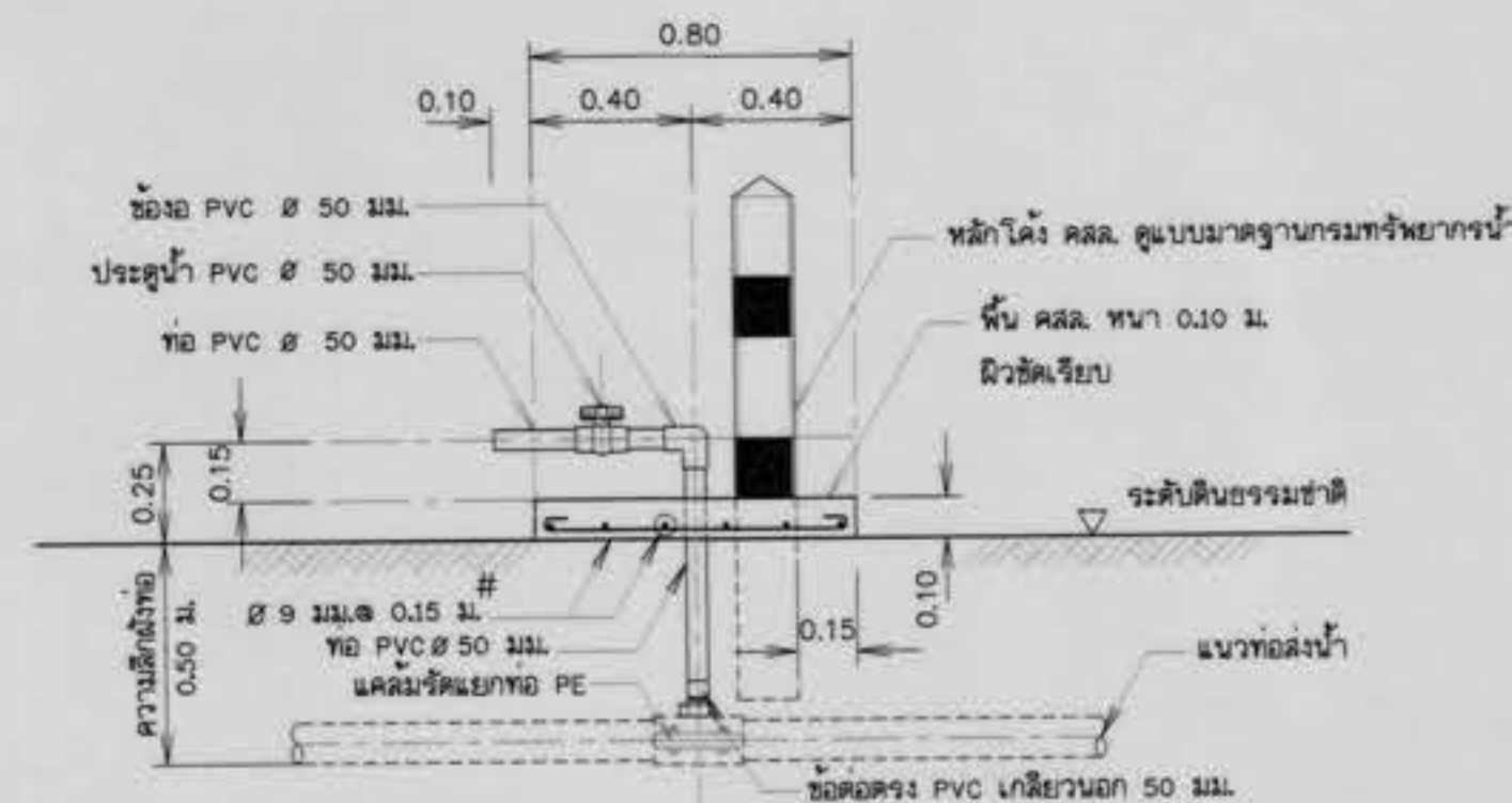
รูปตัด ก - ก แสดงการติดตั้งประตูจุดปล่อยน้ำ มาตราส่วน 1:20
