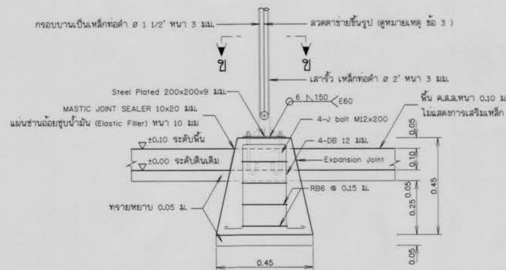
รูปขยายฐานรากโครงสร้างรับแฉง F1 (คอมโบ คสล. หล่อสำเร็จรูปพร้อมติดตั้ง) ไม่แสดงมาตราส่วน
