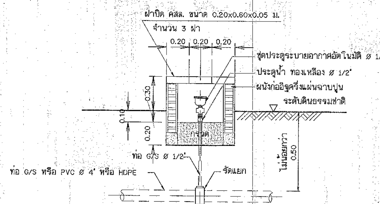
การติดตั้งประตูระบายอากาศอัตโนมัติ
