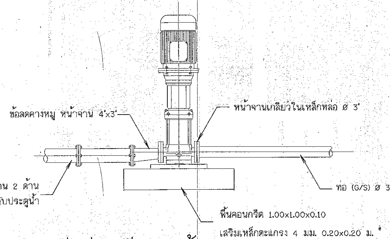
15. การต่อท่อเครื่องสูบน้ำ ไม่แสดงมาตราส่วน
