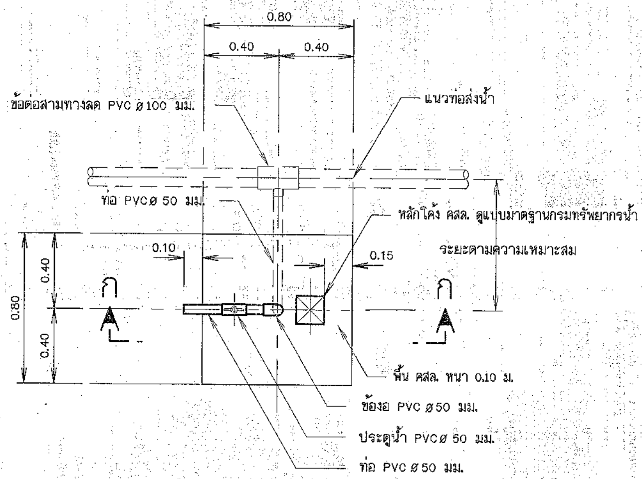
แปลนอาคารจุดปล่อยน้ำ (แบบ ก) **
