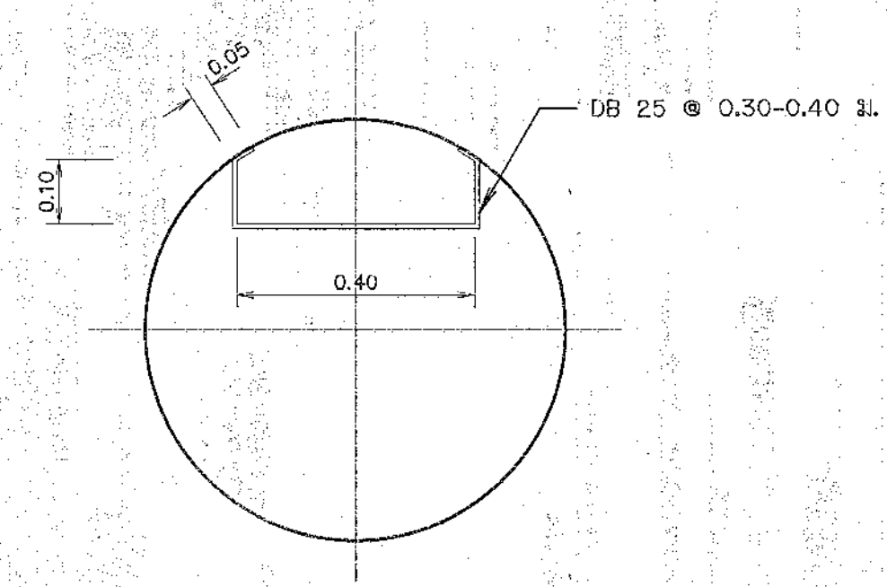
รูปขยายบันไดภายในส่วน column ไม่แสดงมาตราส่วน
