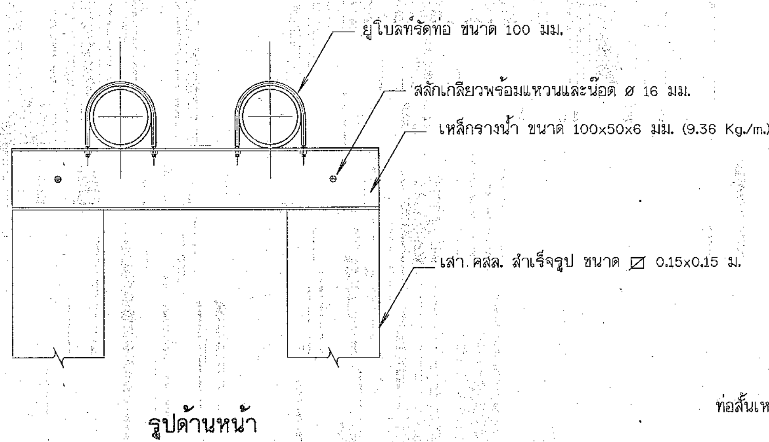
13. เสาคอมม่อนรับท่อคูด และแบบขยายอุปกรณ์รัดท่อ ไม่แสดงมาตราส่วน
