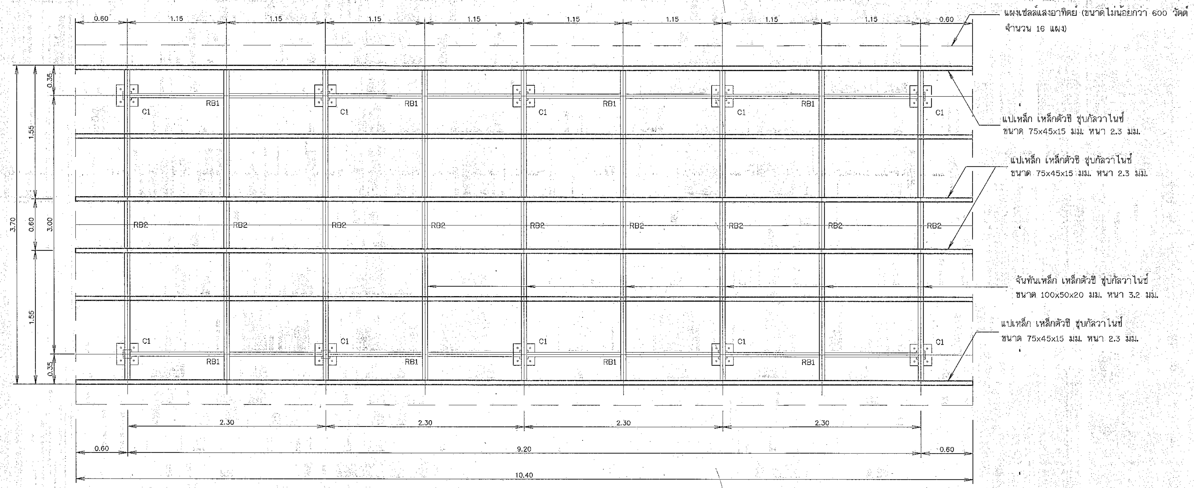
แปลนฐานรากและโครงหลังคา ไม่แสดงขนาดราส่วน
