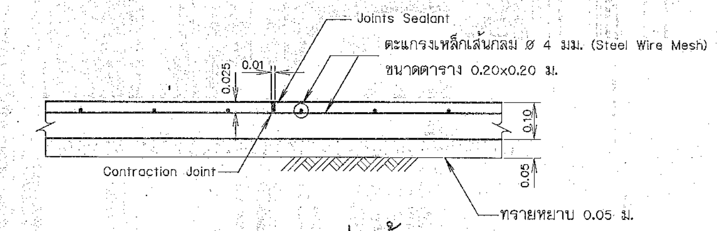
แบบขยายรอยต่อพื้น (Contraction Joint) ไม่แสดงขนาดราส่วน
