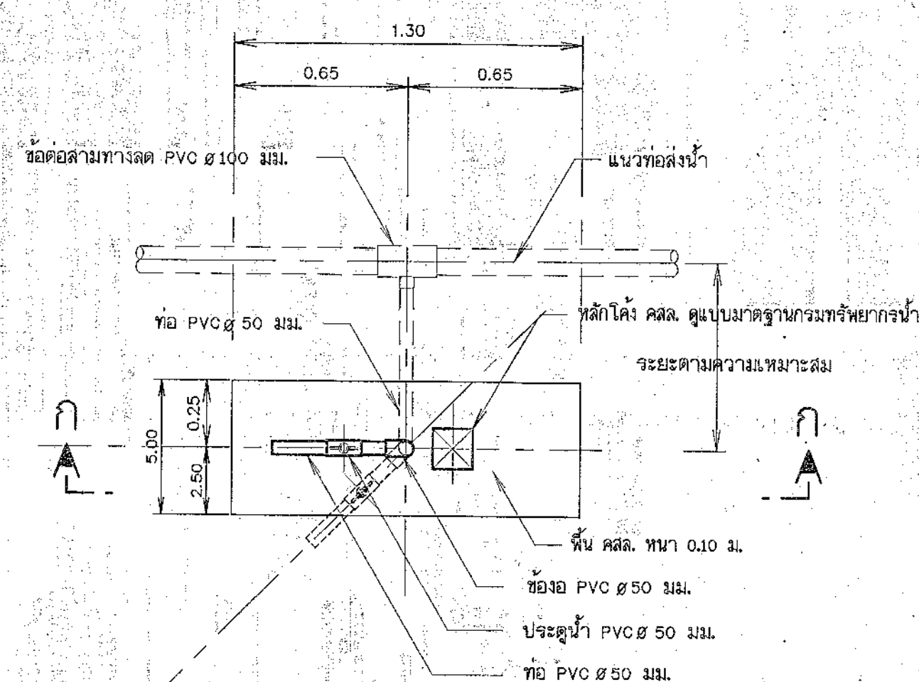
แปลนอาคารจุดปล่อยน้ำ (แบบ ข) **
