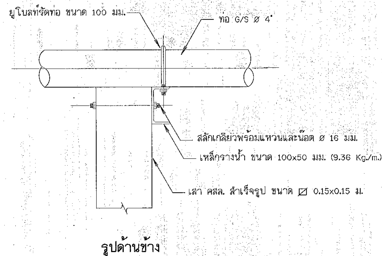
13. เสาคอมม่อนรับท่อคูด และแบบขยายอุปกรณ์รัดท่อ ไม่แสดงมาตราส่วน
