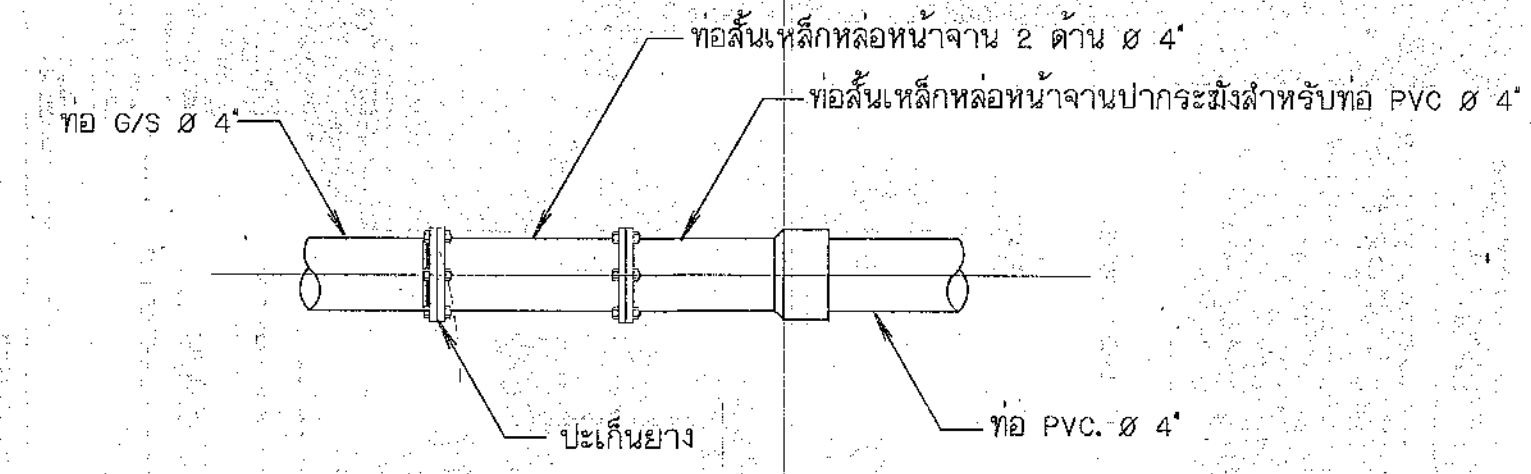
8. การบรรจุบ่อเหล็กอบสังกะสี G/S กับท่อ PVC. ไม่แสดงมาตราส่วน
