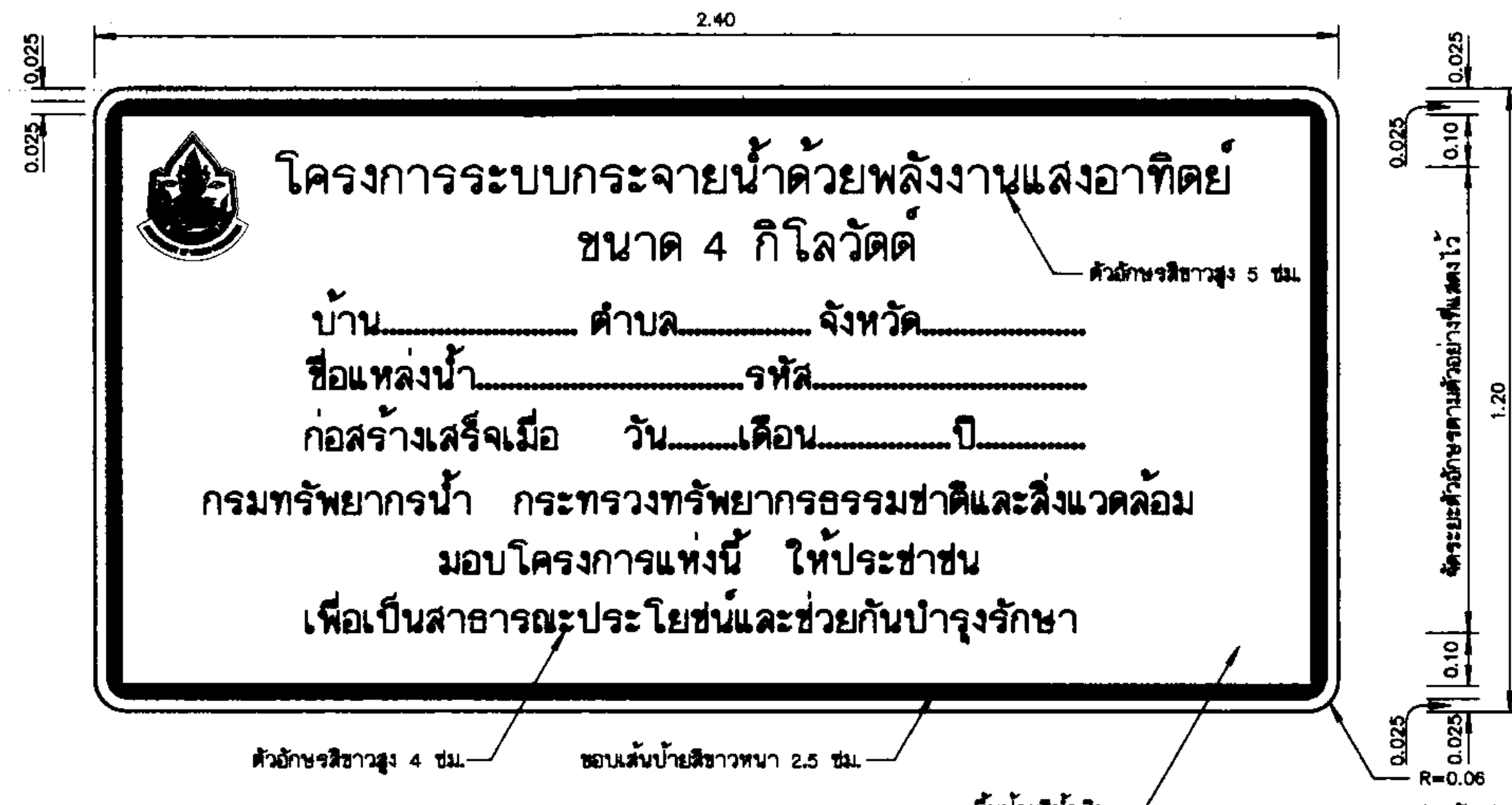
ป้ายโครงการ ไม่แสดงมาตราส่วน
