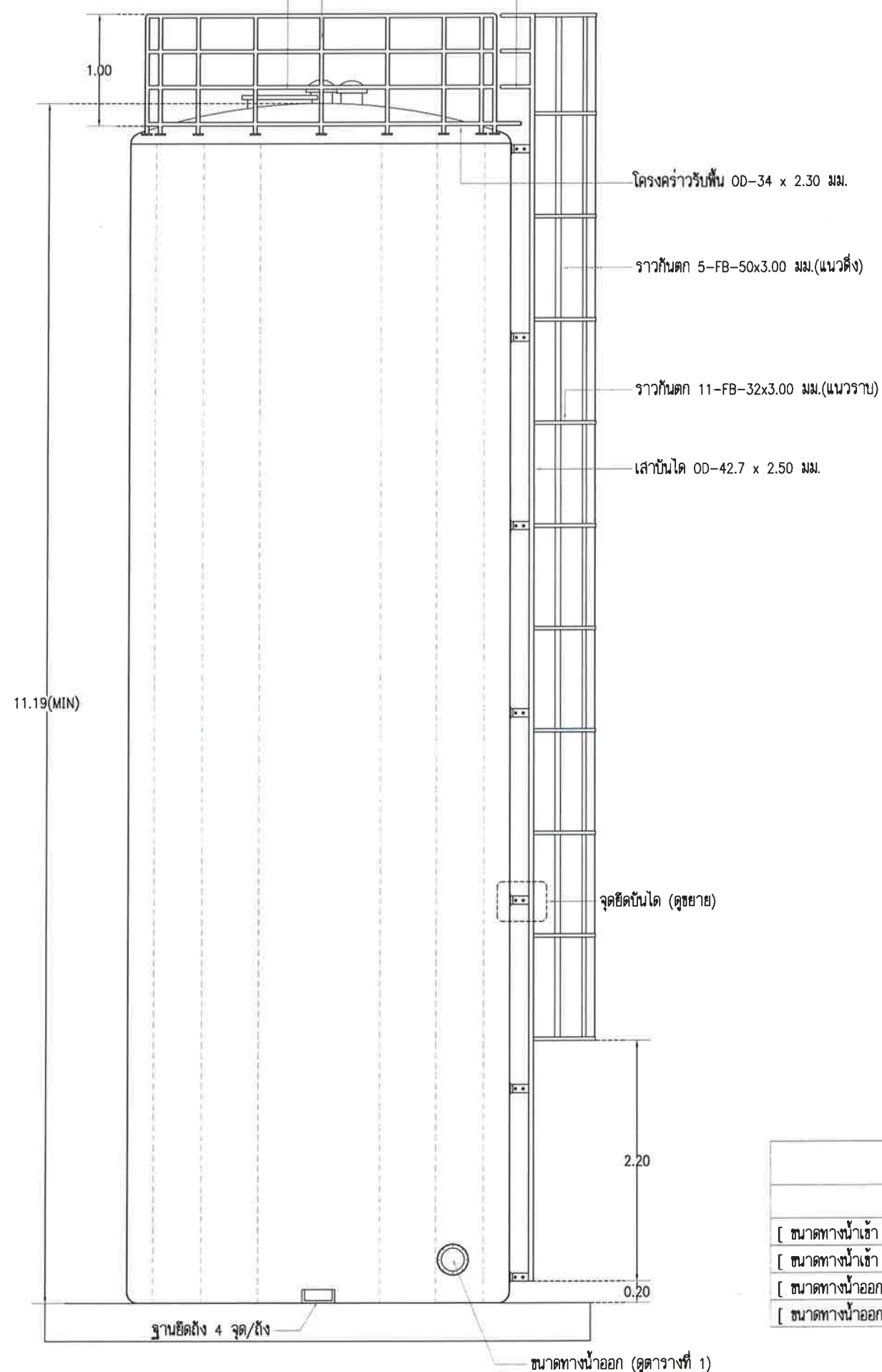
รูปด้านถังเก็บน้ำ SCALE 1:50
