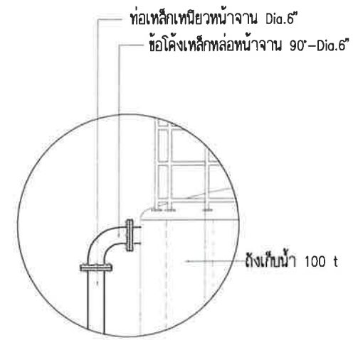
ขยายทางน้ำเข้าถึง (ด้านบนถึง) SCALE 1:50
