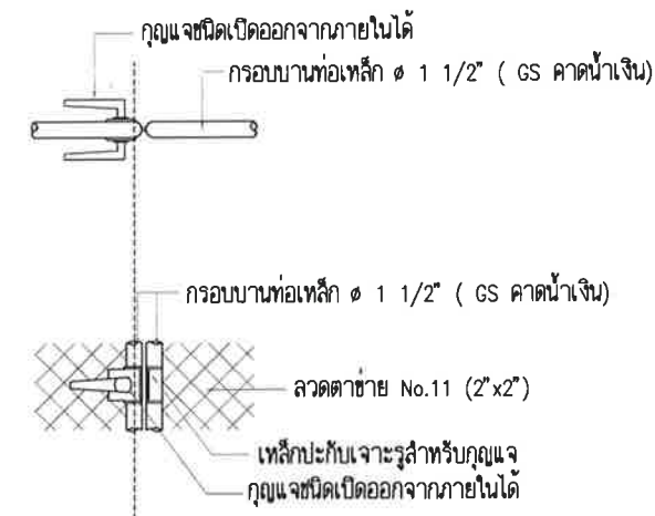
แบบขยาย 2 SCALE 1:20
