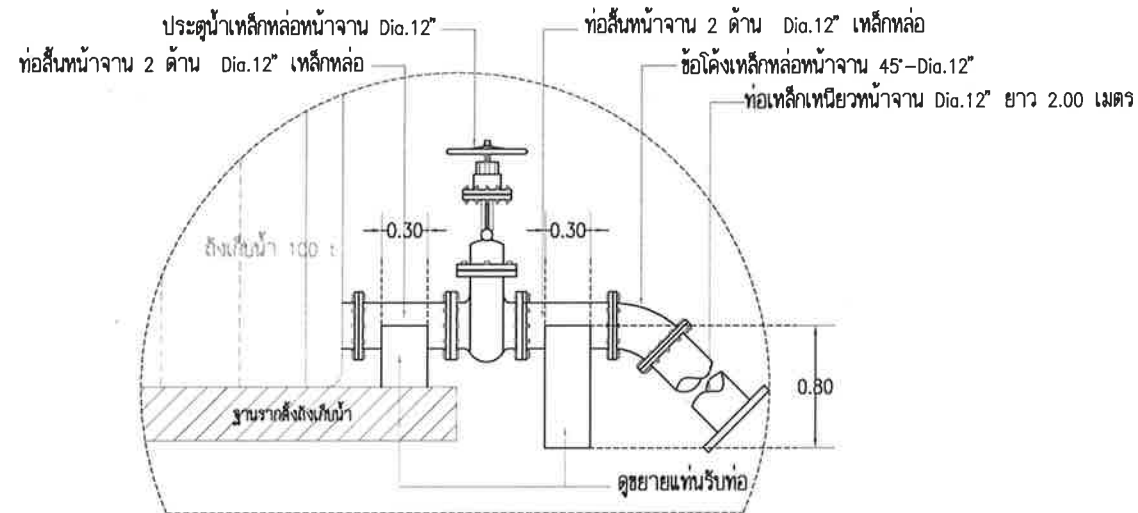
ขยายทางน้ำออกถึง (ด้านล่างถึง) SCALE 1:50
