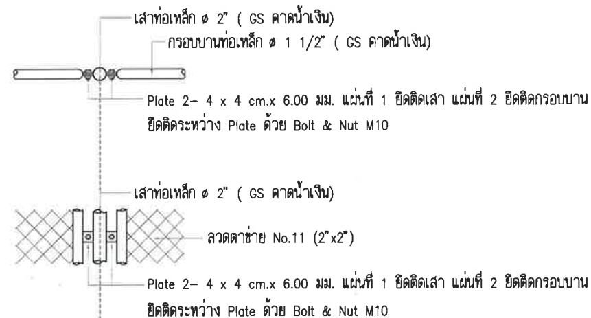
แบบขยาย 1 SCALE 1:20
