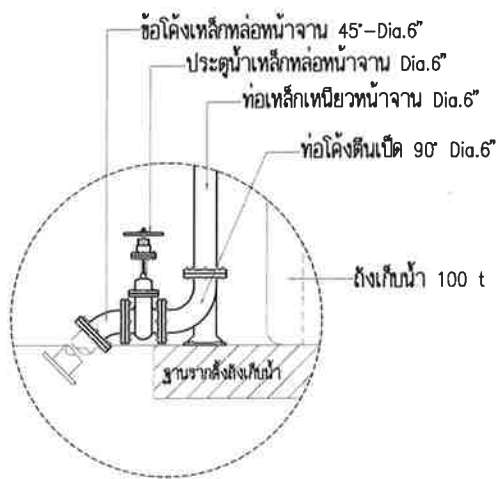
ขยายทางน้ำเข้าถึง (ด้านล่างถึง) SCALE 1:50
