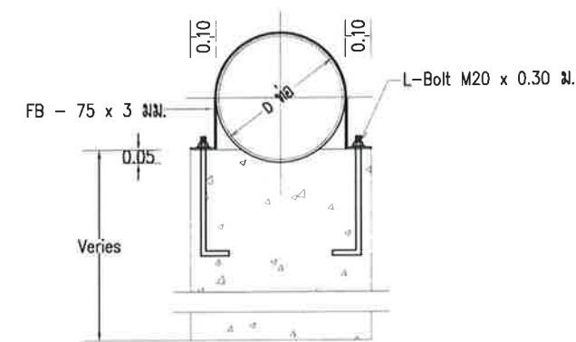
รูปขยายแท่นรับท่อ
