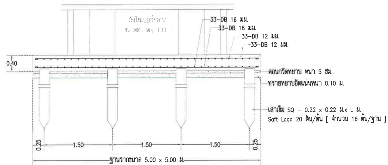
รูปตัดฐานรากแบบเสาเข็ม
