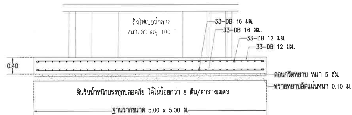
รูปตัดฐานรากแบบแผ่
