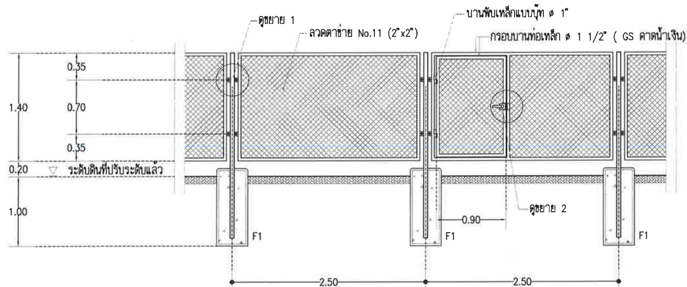
รูปด้านรื้อโปร่ง-ประตู SCALE 1:50
