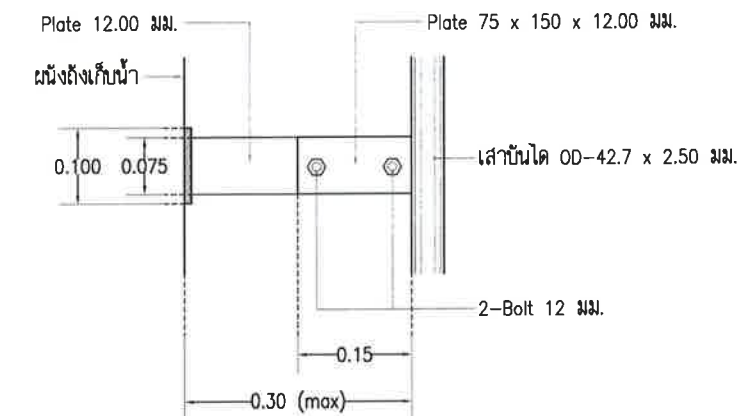
ขยายจุดยึดบันได SCALE 1:10
