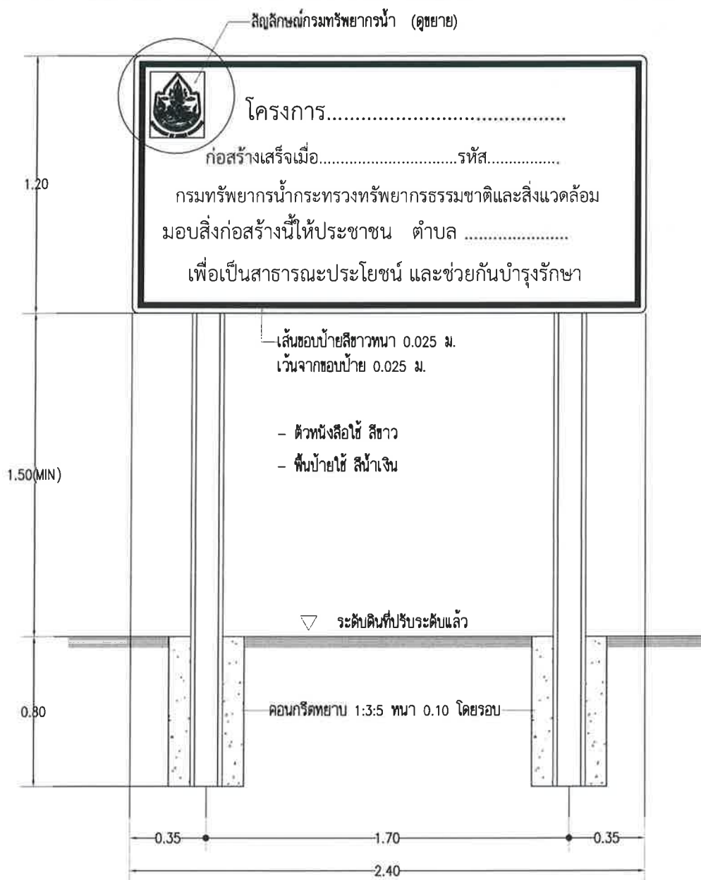
แสดงรูปด้านหน้าป้ายโครงการ SCALE 1:25
