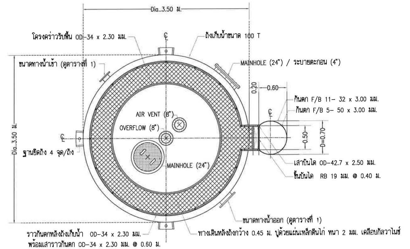
แปลนถังเก็บน้ำ SCALE 1:50
