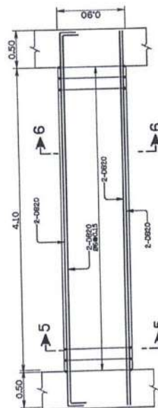
คาน B8
