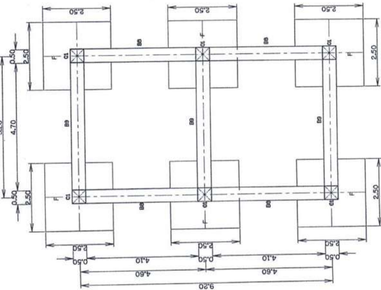
แปลนฐานราก,คานคอดิน
