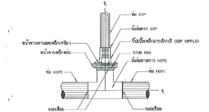
การบรรจุท่อสามทาง HDPE กับท่อ GSP แบบข้อต่อ (สำหรับอาคารจุดปล่อยน้ำ อาคารประจําขยะคอน อาคารทิ้งขยะอากาศ กรณีท่อส่งน้ำขนาดเส้นผ่าศูนย์กลางมากกว่า 315 มม.)
