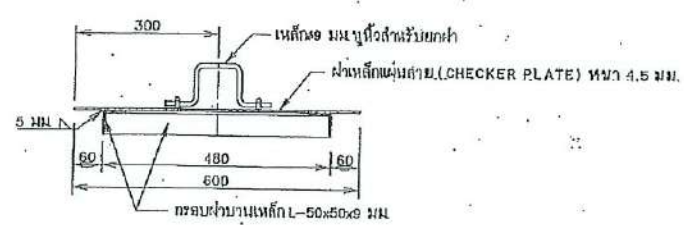
รูปตัด จ-ข ไม่แสดงมาตรฐาน
