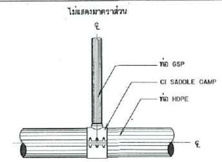
การบรรจุท่อสามทาง HDPE กับท่อ GSP แบบ CI SADDLE CLAMP (สำหรับอาคารจุดปล่อยน้ำ อาคารประจําขยะคอน อาคารทิ้งขยะอากาศ กรณีท่อส่งน้ำขนาดเส้นผ่าศูนย์กลางน้อยกว่าหรือเท่ากับ 315 มม.)
