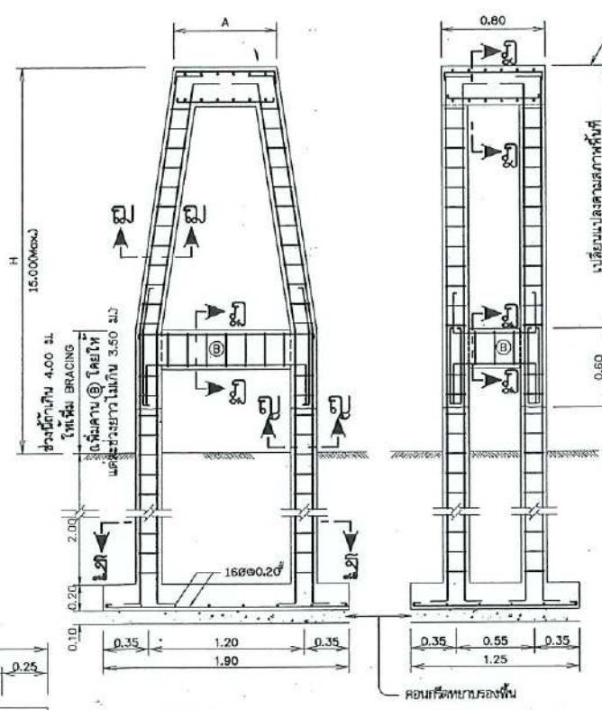
ตอม่อรับท่อแบบที่ 1
