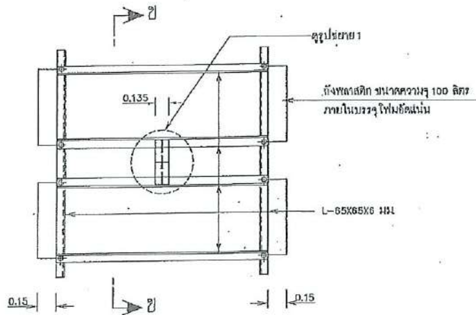
แปลน รายละเอียดท่อนางที่ยังค้างหมอน
