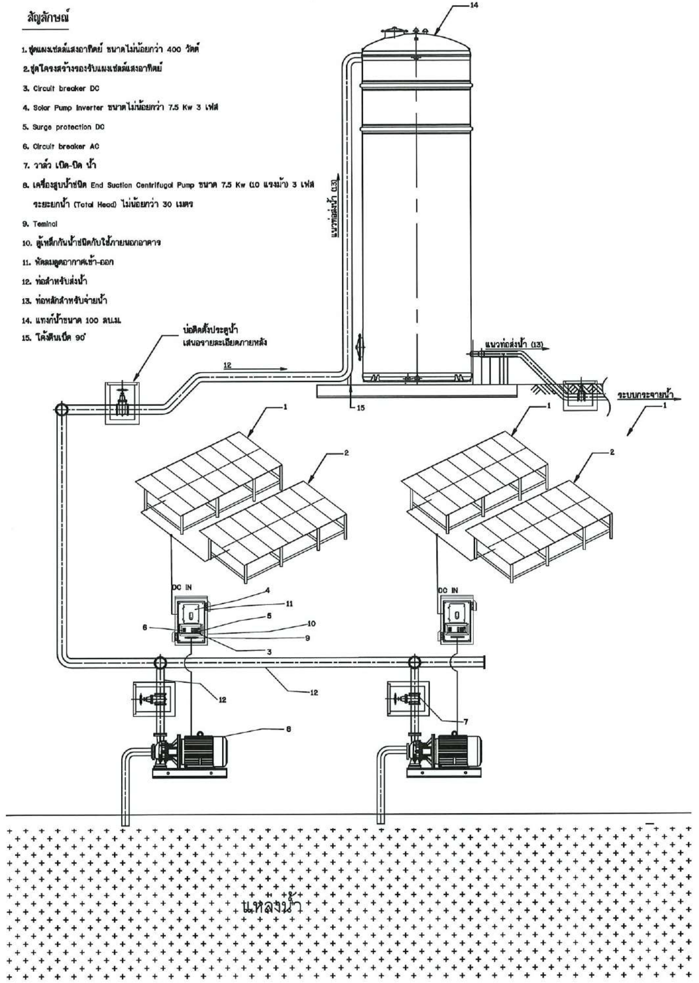
แบบระบบกระจายน้ำด้วยพลังงานแสงอาทิตย์ มาตราส่วน โมเสกขนาดจาวน
