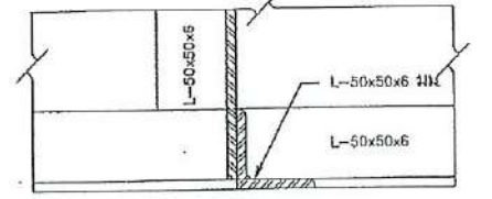
รูปตัด ๘-๘ ขนาดส่วน 1 : 2.5
