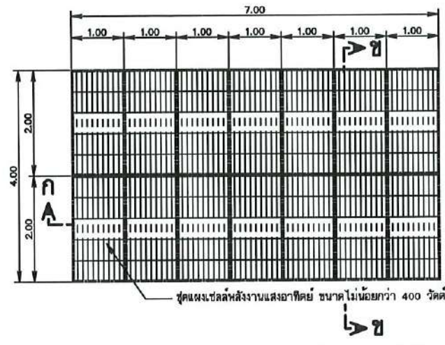
แปลนแผงเซลล์พลังงานแสงอาทิตย์ขนาดไม่น้อยกว่า 400 วัตต์ มาตรฐาน 1:100
