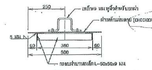
รูปตัด ก-ก ไม่แสดงมาตรฐาน
