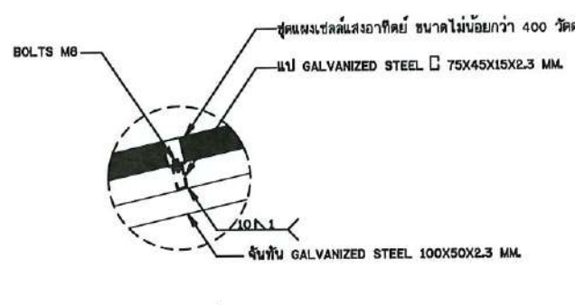
รูปขยาย 1 มาตรฐาน 1:10
