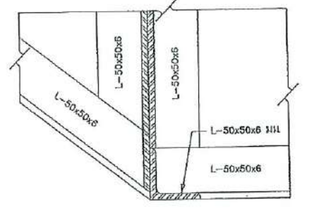
รูปตัด ๗-๗ ขนาดส่วน 1 : 2.5
