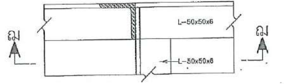
รูปขยาย 6 ขนาดส่วน 1 : 2.5
