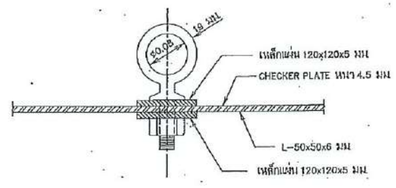
รูปขยายห่วงยึดแพะสูบน้ำ มาตราส่วน 1 : 5
