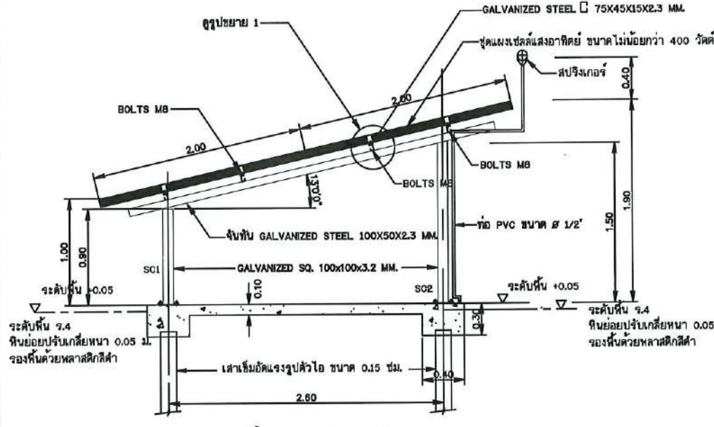
รูปตัด ข - ข มาตรฐาน 1:50
