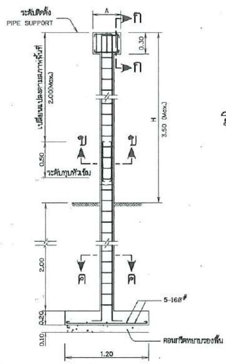
การเสริมเหล็ก ตอม่อแบบที่ 1
