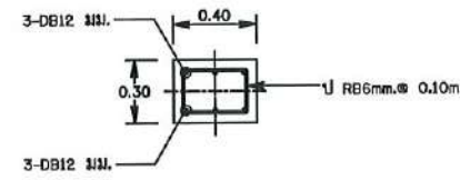
แบบขยายคาน B1
