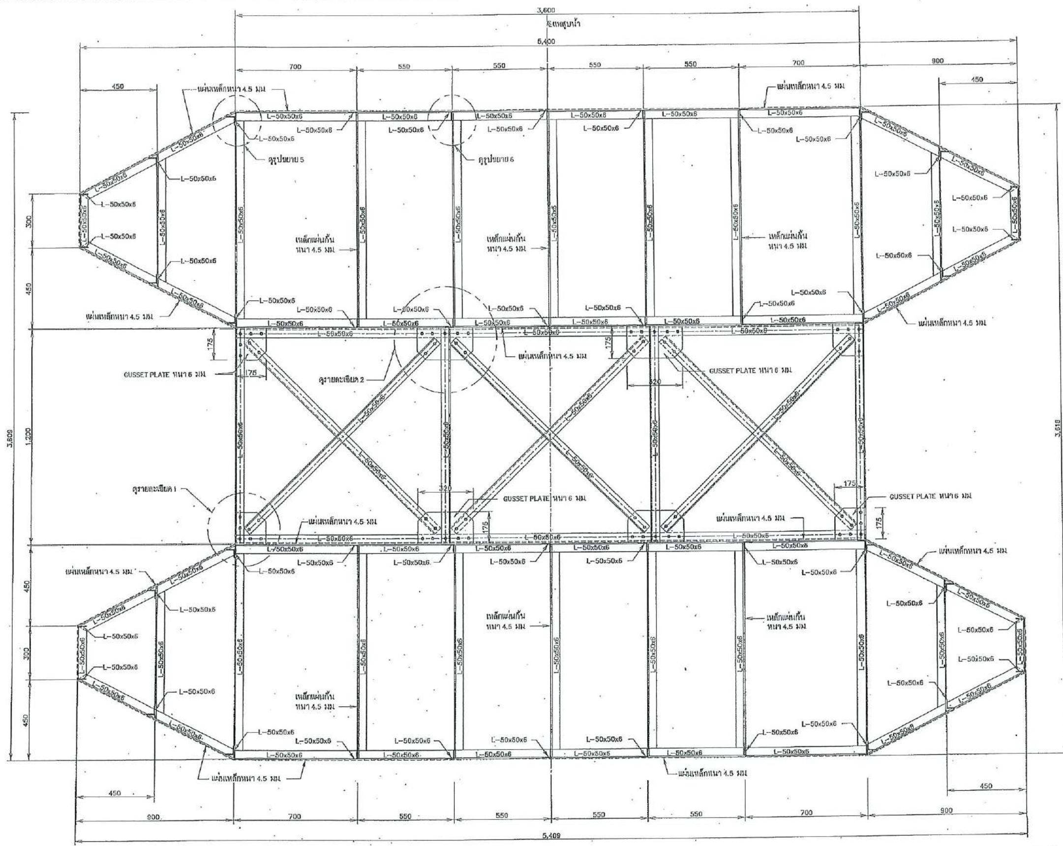
รูปตัด ๓-๓ ขนาดส่วน 1 : 10
