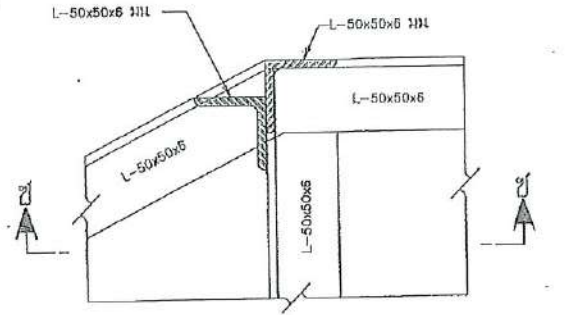
รูปขยาย 5 ขนาดส่วน 1 : 2.5
