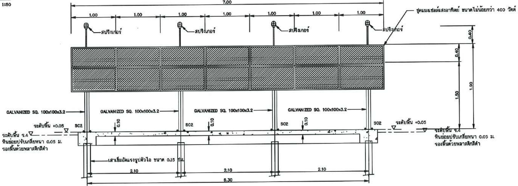
รูปตัด ก - ก มาตรฐาน 1:50
