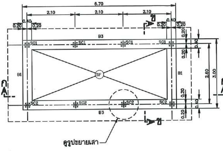
แปลนคานคอดิน มาตรฐาน 1:100
