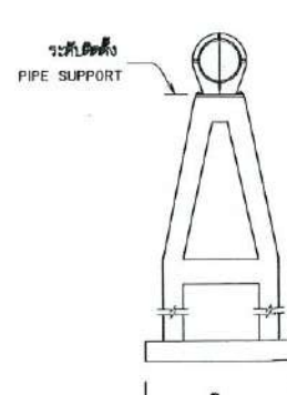
รูปด้านหน้า
