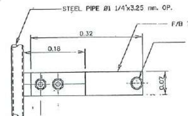
รูปตัด ง - ง มาตราส่วน 1:5
