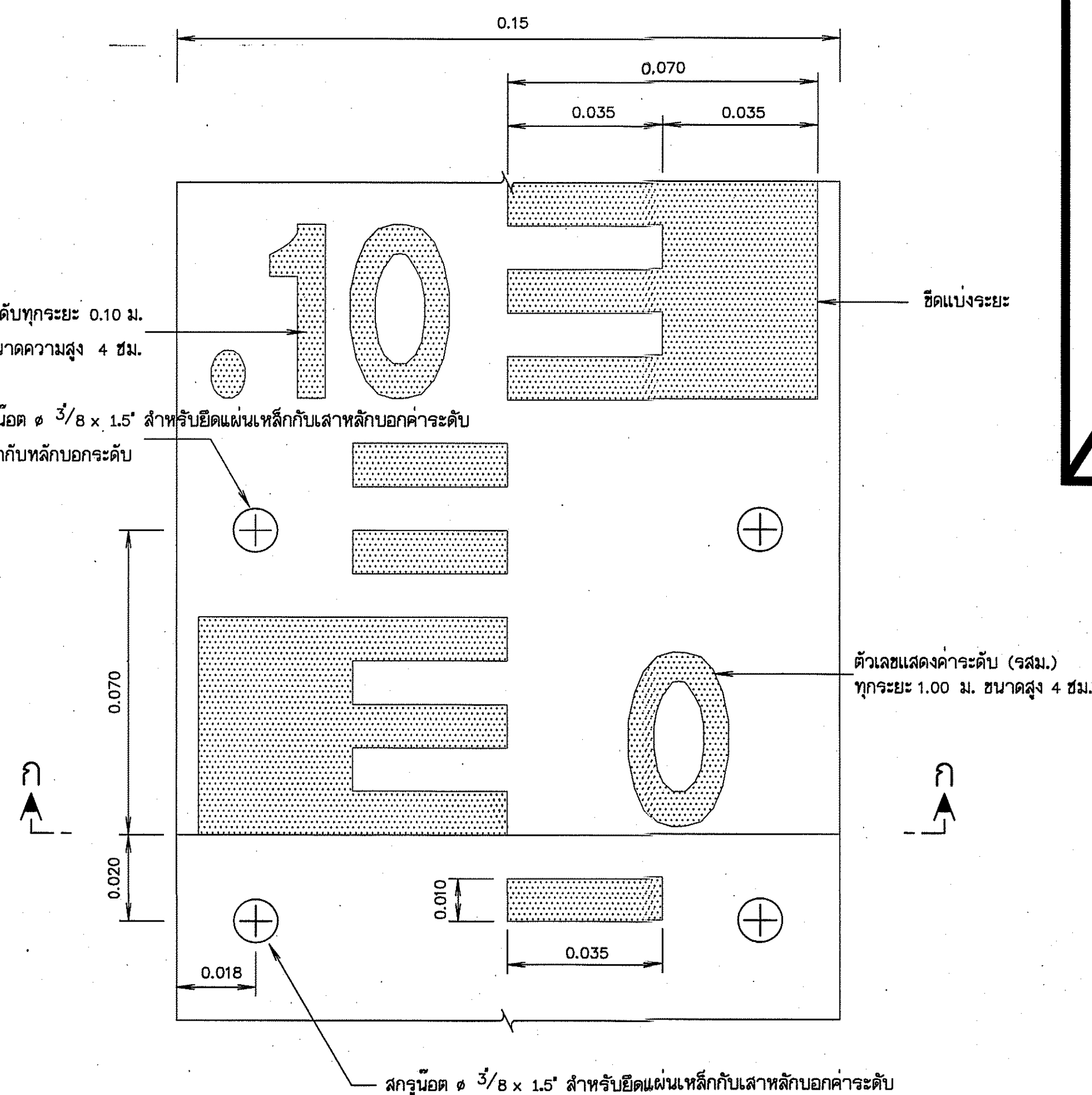
ขยายแผนหลักบอการค้าระดับ มาตราส่วน 1:1
