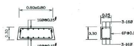
รูปตัด ช-ช รูปตัด ซ-ซ
