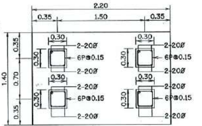
รูปตัด จ-จ
