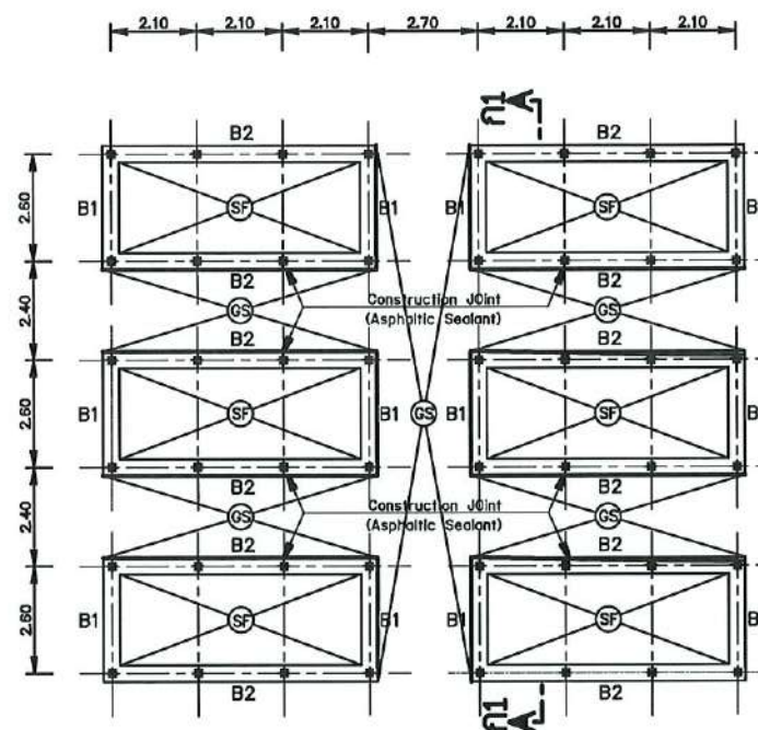
แปลนคานคอดินแฉงเพลล์พลังงานแสงอาทิตย์
