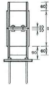
รูปด้านข้าง
