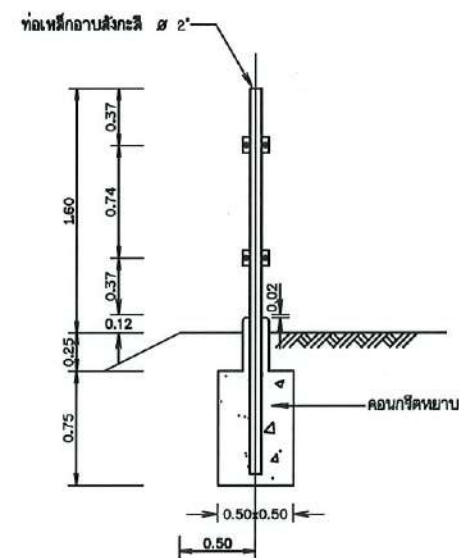
แบบขยายรู้ (รูปด้านข้าง) มาตราส่วน 1:25
