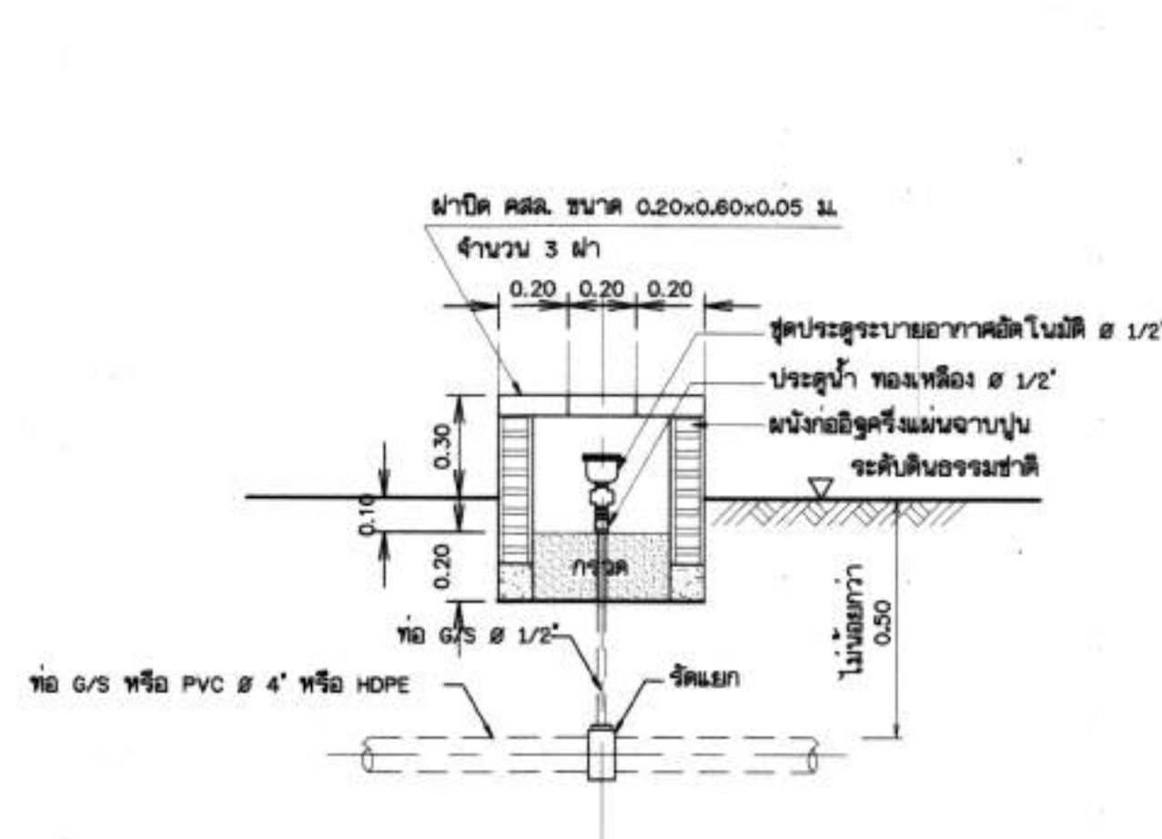
การติดตั้งประตูดระบายอากาศอัตโนมัติ
