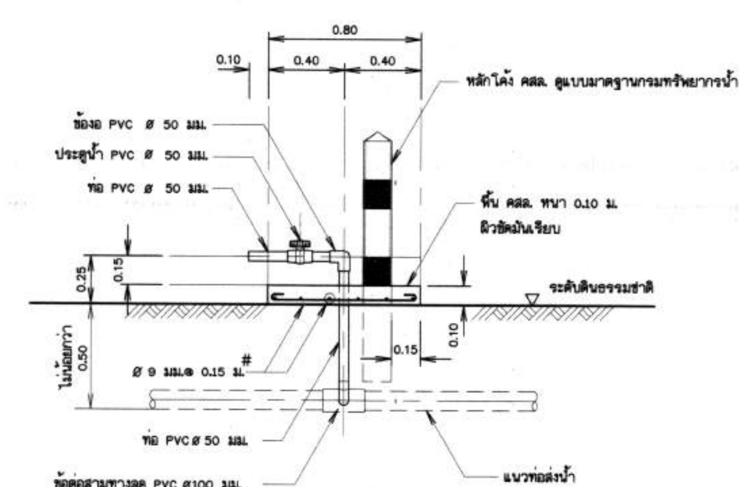
รูปตัด ก - ก แสดงการติดตั้งประตูดปล่อยน้ำ
