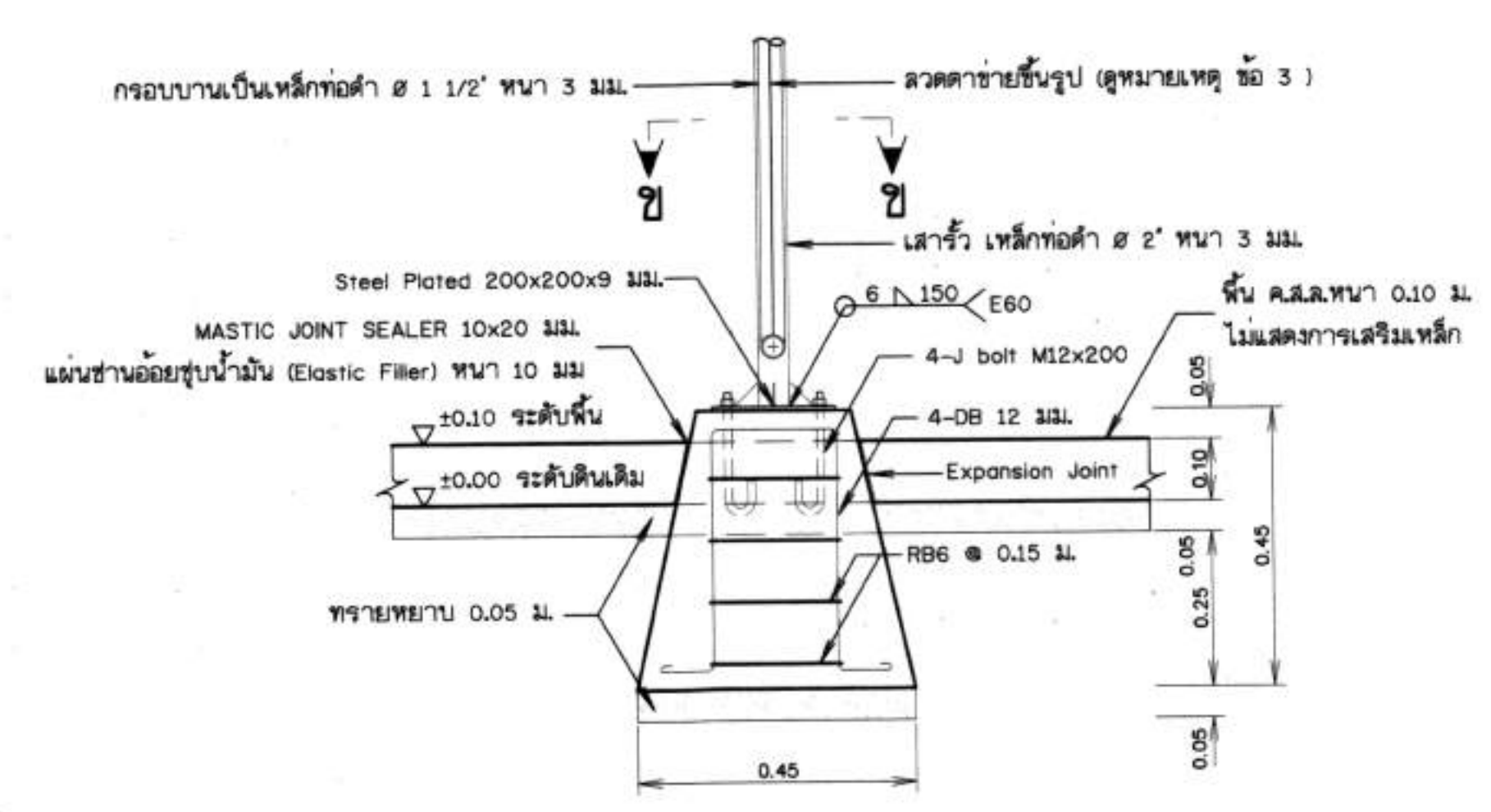
รูปขยายฐานรากโครงสร้างรับแผง F1 (ต่อม่อ คสส. หล่อสำเร็จรูปพร้อมติดตั้ง) ไม่แสดงมาตราส่วน
