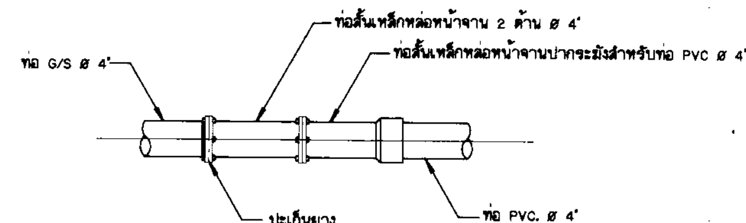
8. การบรรจุท่อเหล็กอาบสังกะสี G/S กับท่อ PVC. ไม่แสดงมาตราส่วน
