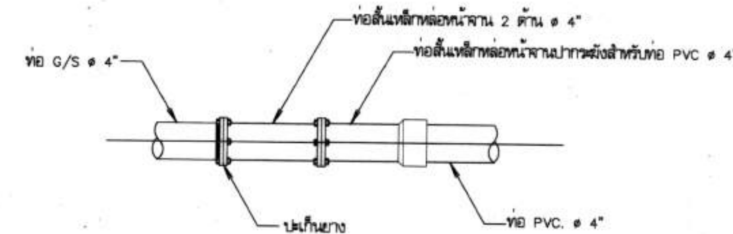
8. การบรรจบท่อเหล็กอาบสังกะสี G/S กับท่อ PVC. ไม่แสดงมาตรฐาน
