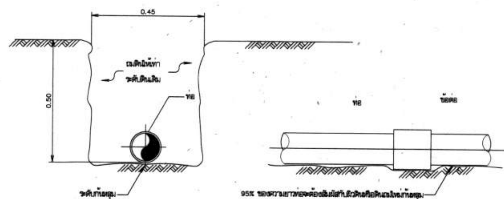
1. แบบการวางท่อทั่วไป มาตรฐาน
