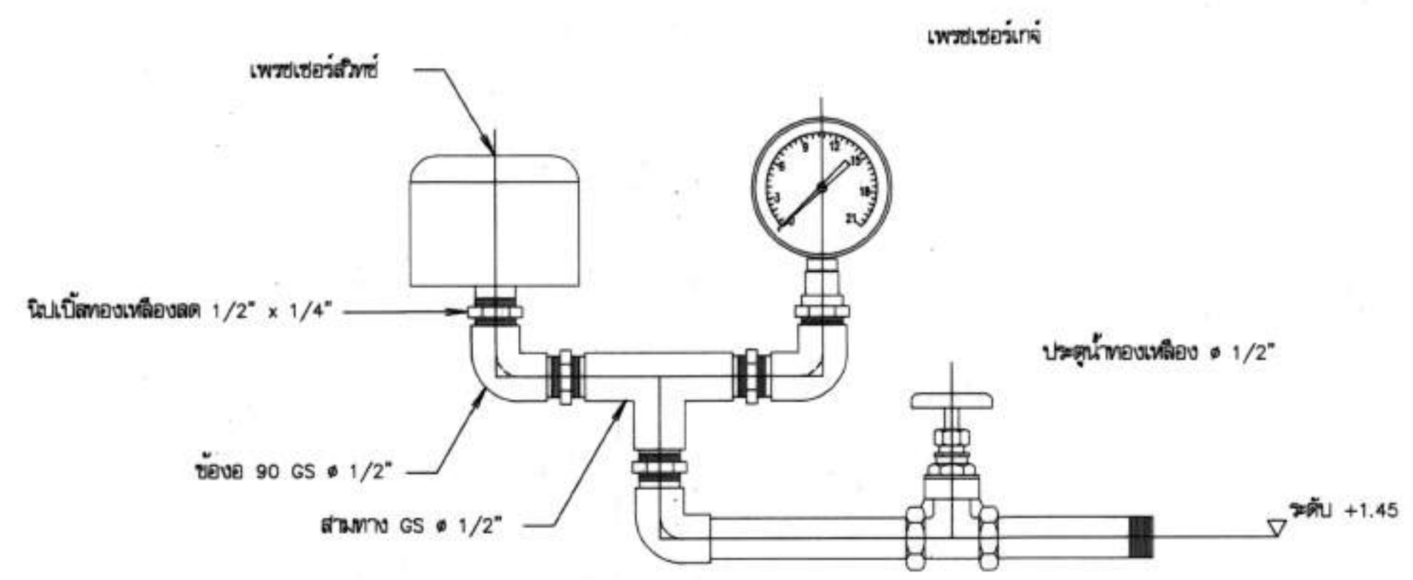
แบบขยายลิ้นชักควบคุมและแก้วัดความดัน ไม่แสดงมาตราส่วน
