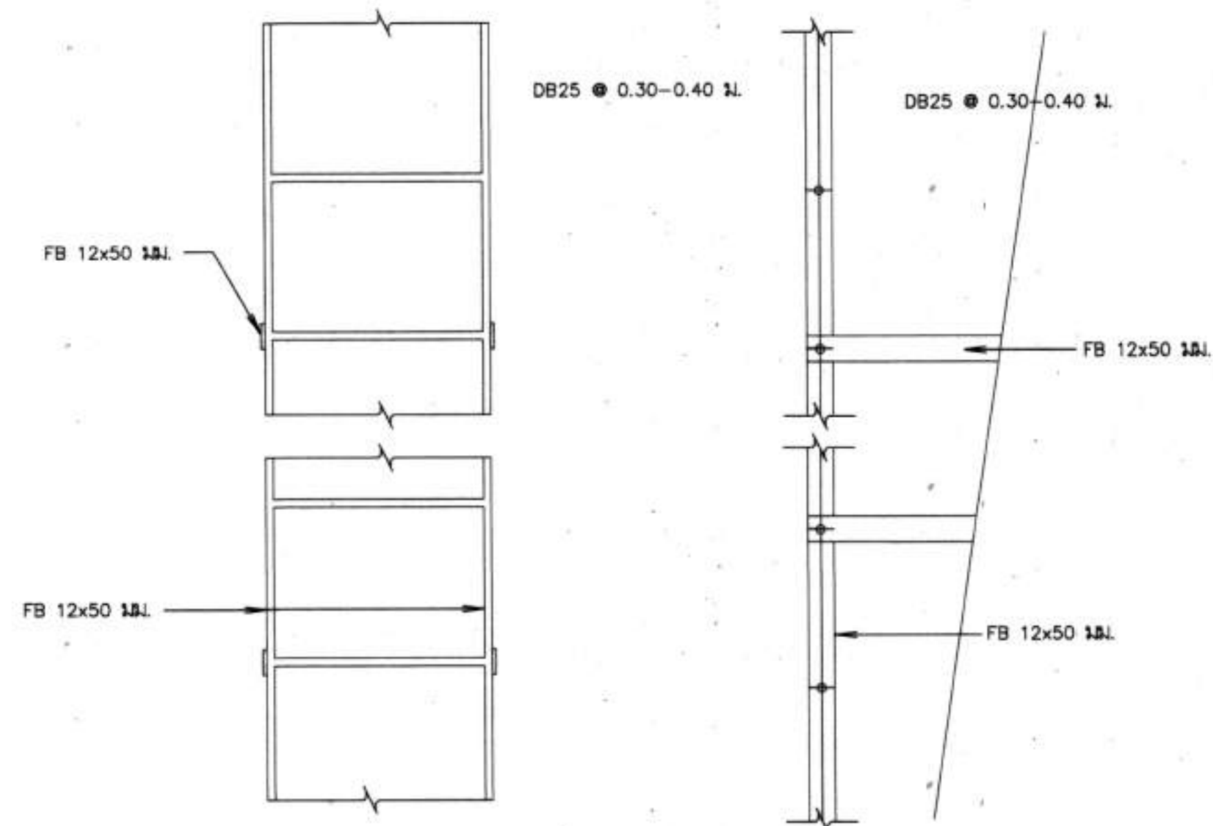
แบบขยายบันได ภายในหอถังสูง ไม่แสดงมาตราส่วน
