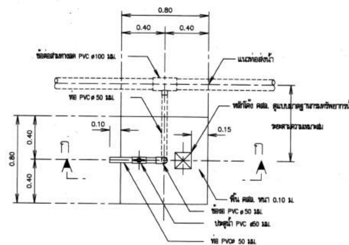
แปลนอาคารจุดปล่อยน้ำ มาตรฐาน 1:20
