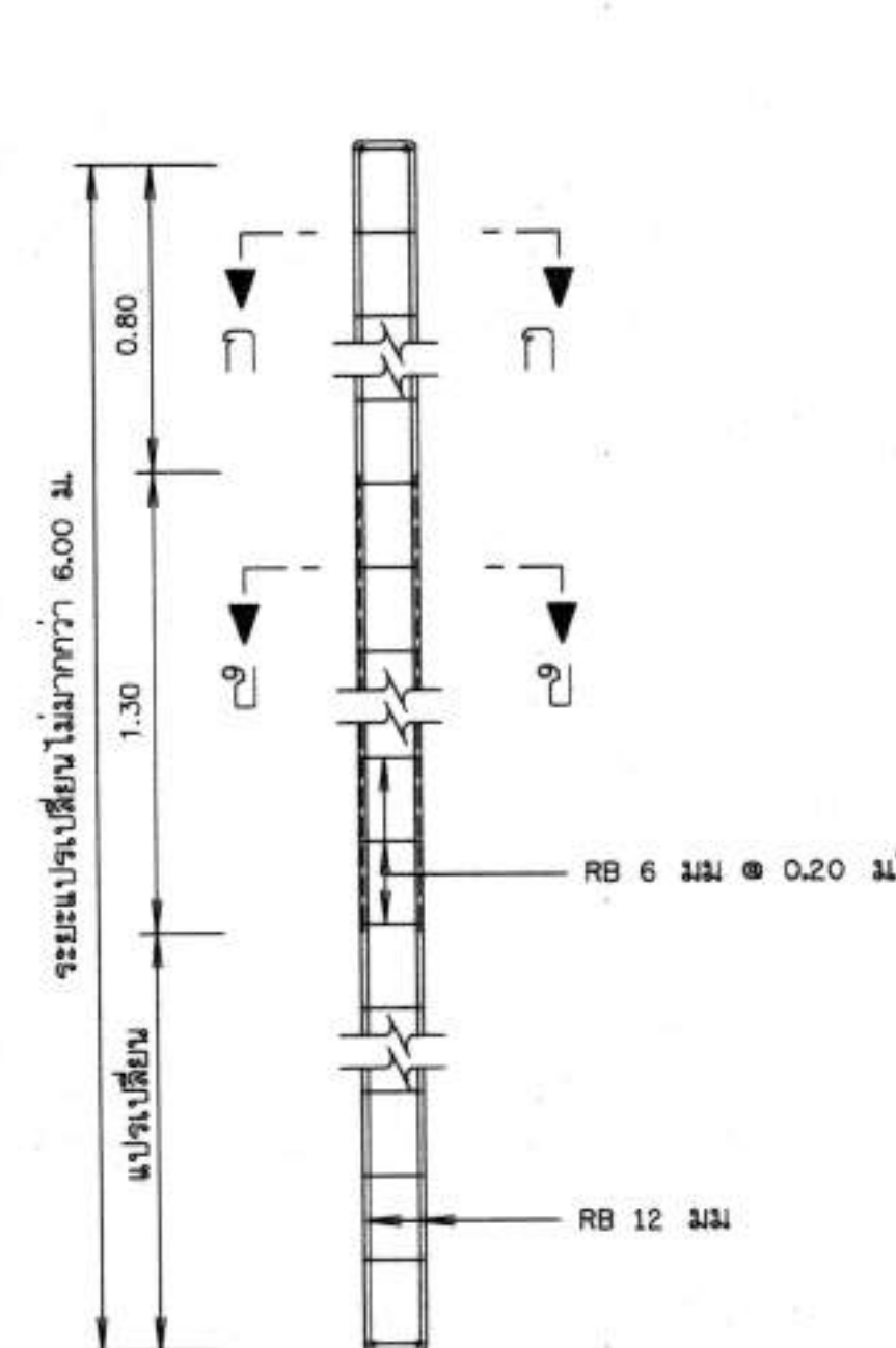
รายละเอียดเสาป้าย คลส. ไม่แสดงมาตราส่วน
