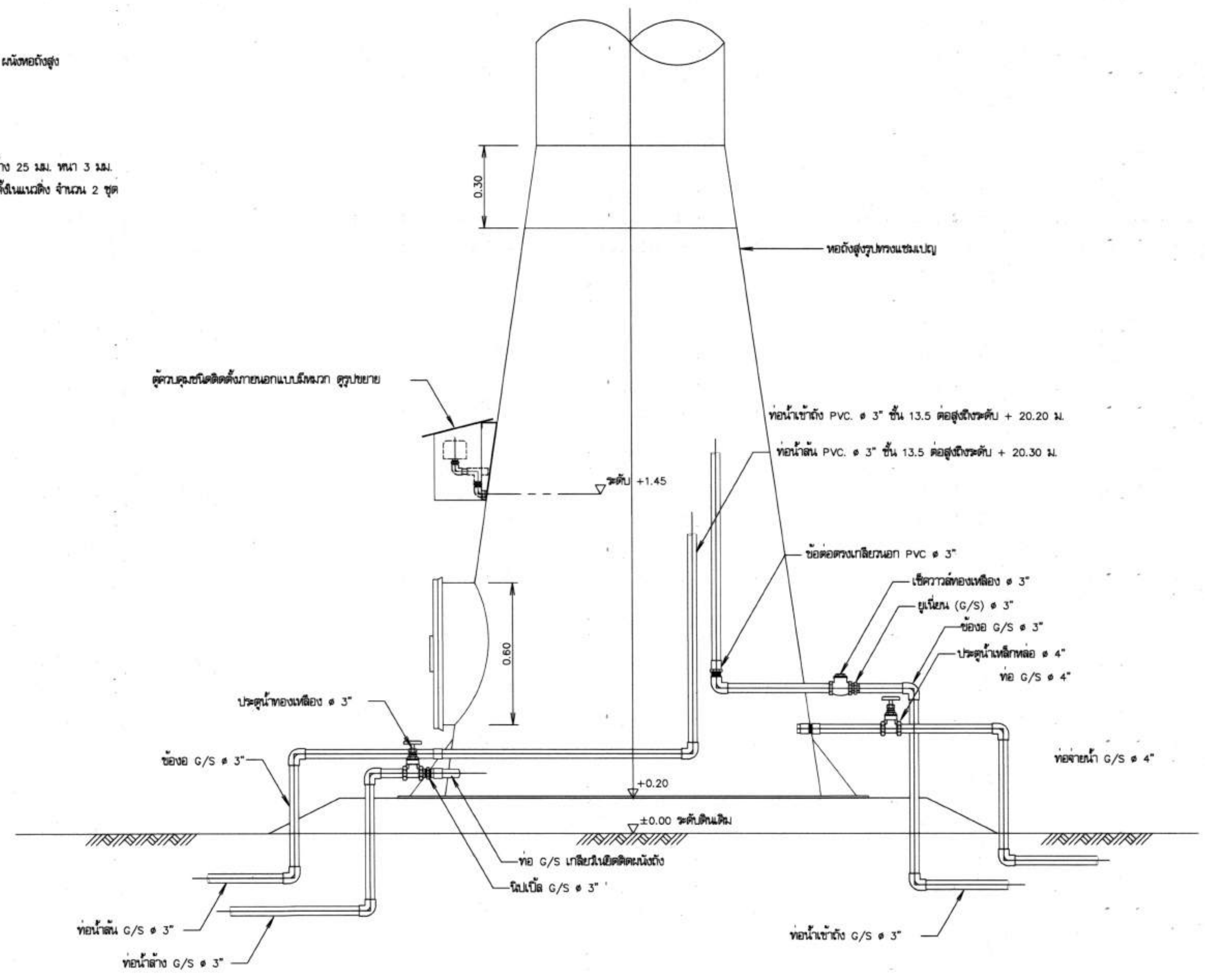
แบบแสดงการเดินท่อในหอถังสูง ไม่แสดงมาตราส่วน
