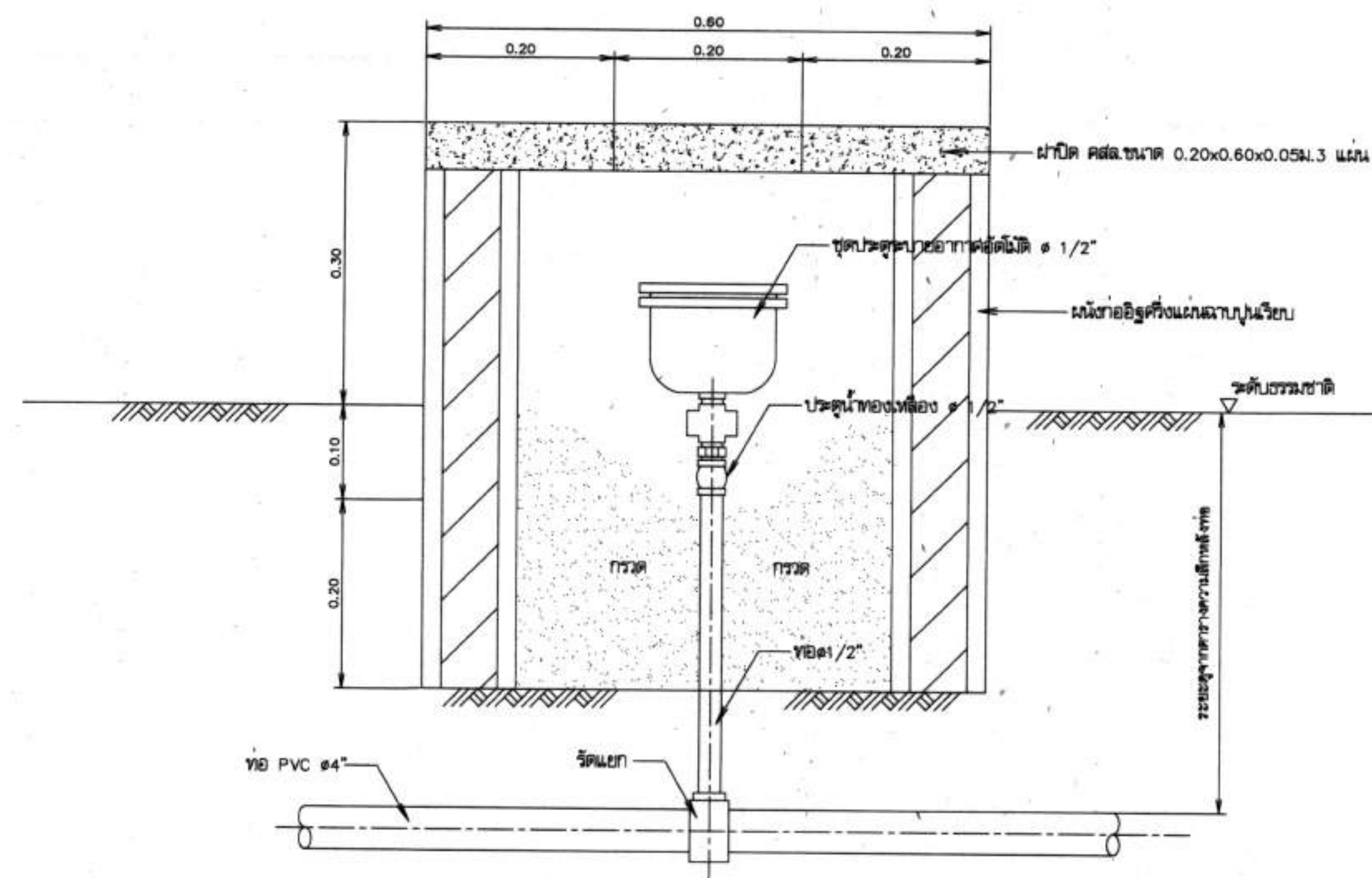
12 การติดตั้งประตูระบายอากาศอัตโนมัติ มาตรฐาน 1:5
