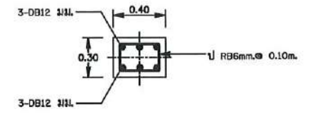
แบบขยายคาน B1 มาตราส่วน 1:40
