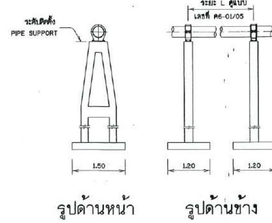
ตอม่อรับท่อแบบที่ 4 มาตรฐาน
