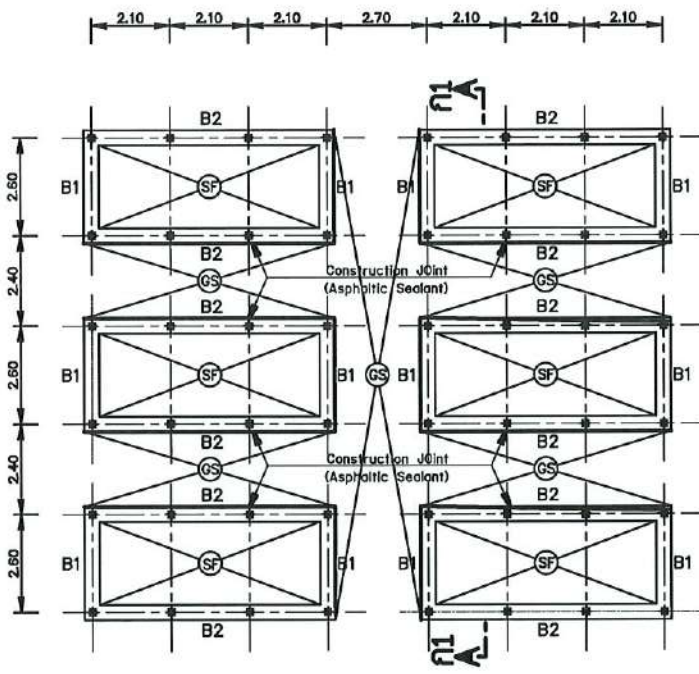
แปลนคานาคอนกรีตแผงเซลล์พลังงานแสงอาทิตย์ มาตราส่วน 1:20
