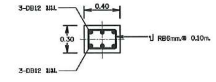
แบบขยายคาน B2 มาตราส่วน 1:40
