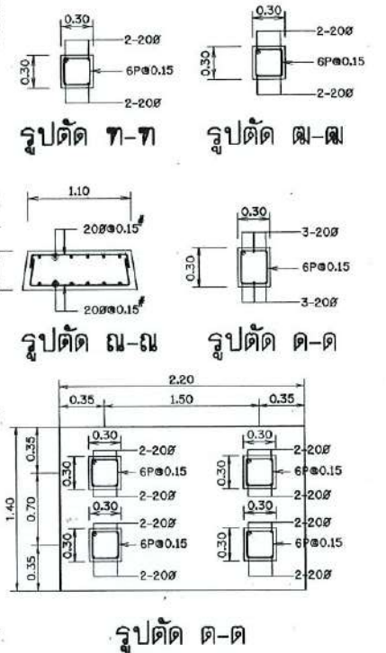
รูปตัดตามขวาง รูปตัดตามยาว
