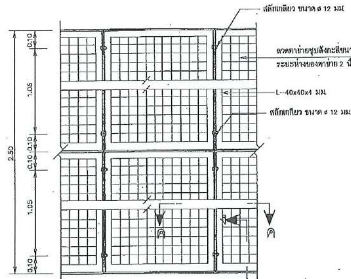
รูปด้านผนังลวดตาข่าย
