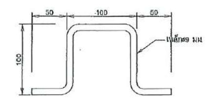
รูปขยายเหล็กหล่อหัวฝาทะ MANHOLE ไม่แสดงขนาดส่วน
