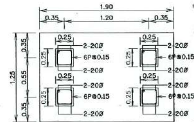
รูปตัด 13-13
