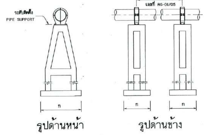
ตอม่อรับท่อแบบที่ 3,4 มาตรฐาน
