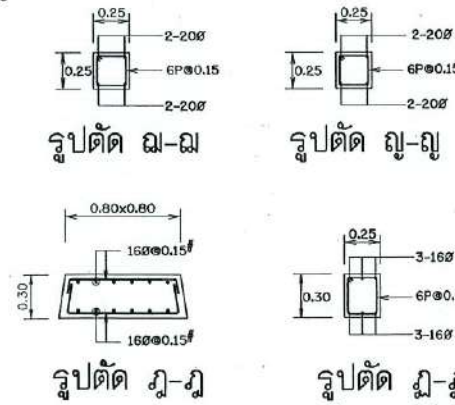
รูปตัด 8-8 รูปตัด 9-9 การเสริมเหล็ก ตอม่อแบบที่ 3 มาตรฐาน
