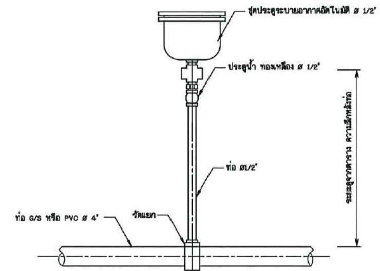
การติดตั้งประตูปะทะอากาศอัตโนมัติ ไม่แสดงมาตราส่วน
