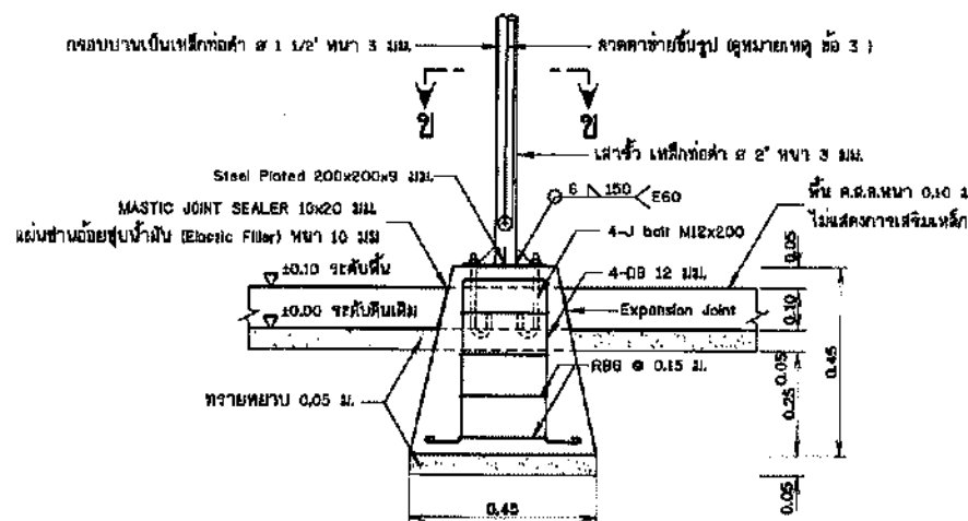
รูปขยายฐานรากโครงสร้างรับแผง F1 ตามข้อ ค.ค.พว ๐.๑๐ ม. หรือรูปหรือมอดี้ ไม่แสดงขนาดบางส่วน
