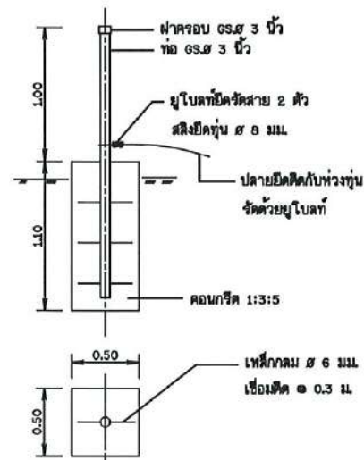
รูปขยายสายยึดแพ มาตราส่วน 1:50
