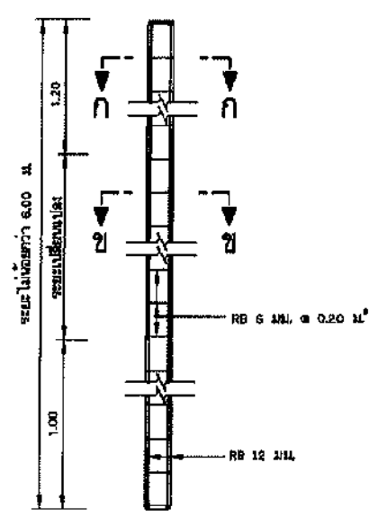
รายละเอียดเสาป้าย สล. ไม่แสดงมาตราส่วน
