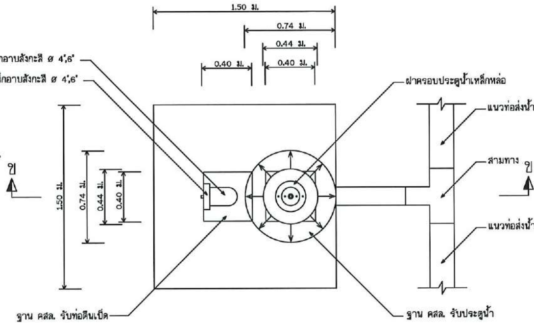
แปลนประตุน้ำระบายตะกอน มาตราส่วน No Scale
