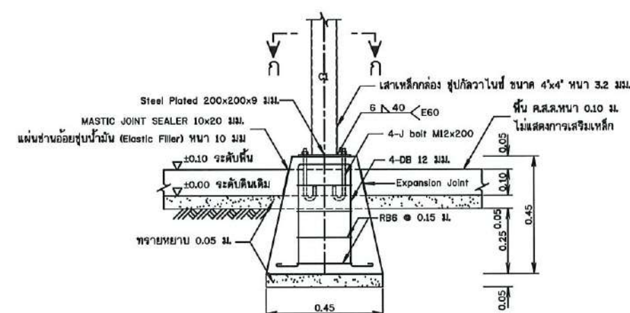
รูปขยายฐานรากโครงสร้างรับแผง F1 (ตอนล่าง คสล. หลังผ้าเบรกรับมิดคิง) ไม่แสดงมาตราส่วน
