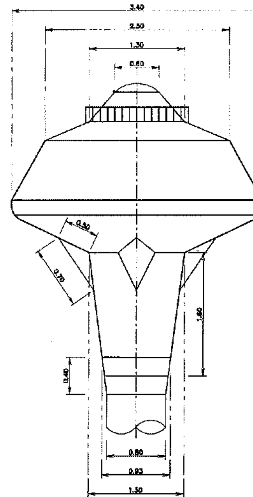
แบบขยายแมนโฮลบนท่อถังสูง ไม่แสดงขนาดบางส่วน
