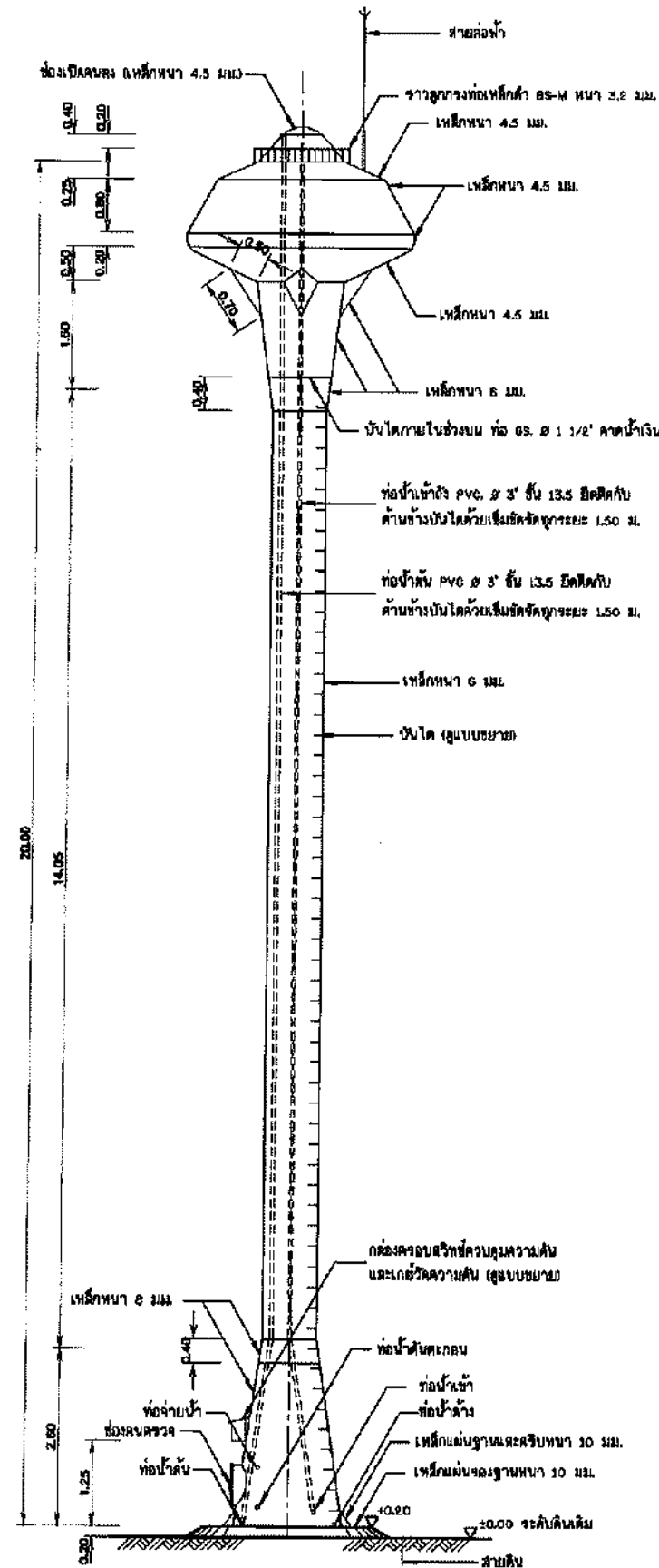
รูปด้านข้างของถังสูง แบบถังเหล็กรูปทรงแป้น ไม่แสดงขนาดบางส่วน
