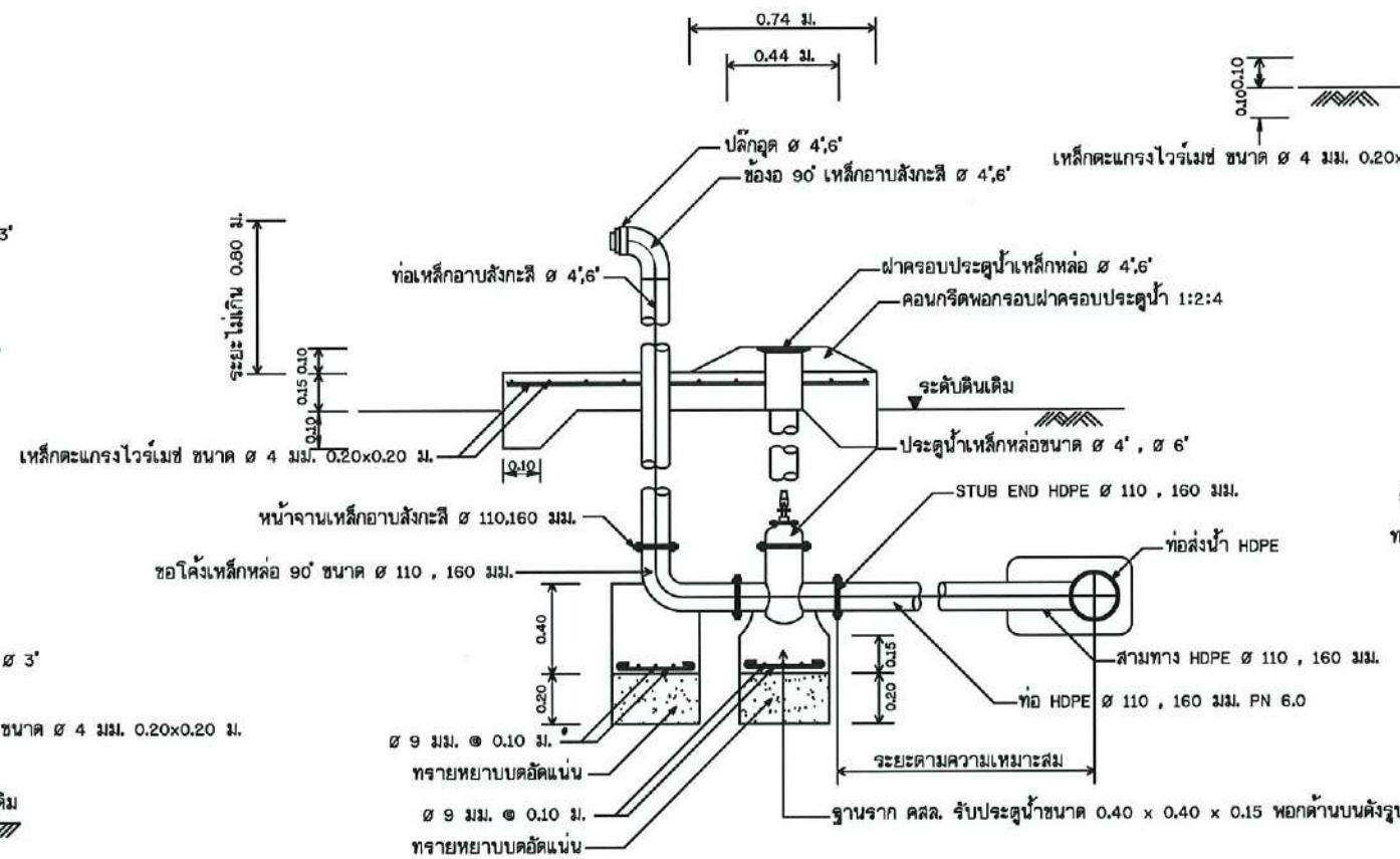
รูปตัด ข - ข แสดงการติดตั้งประตุน้ำระบายตะกอน
