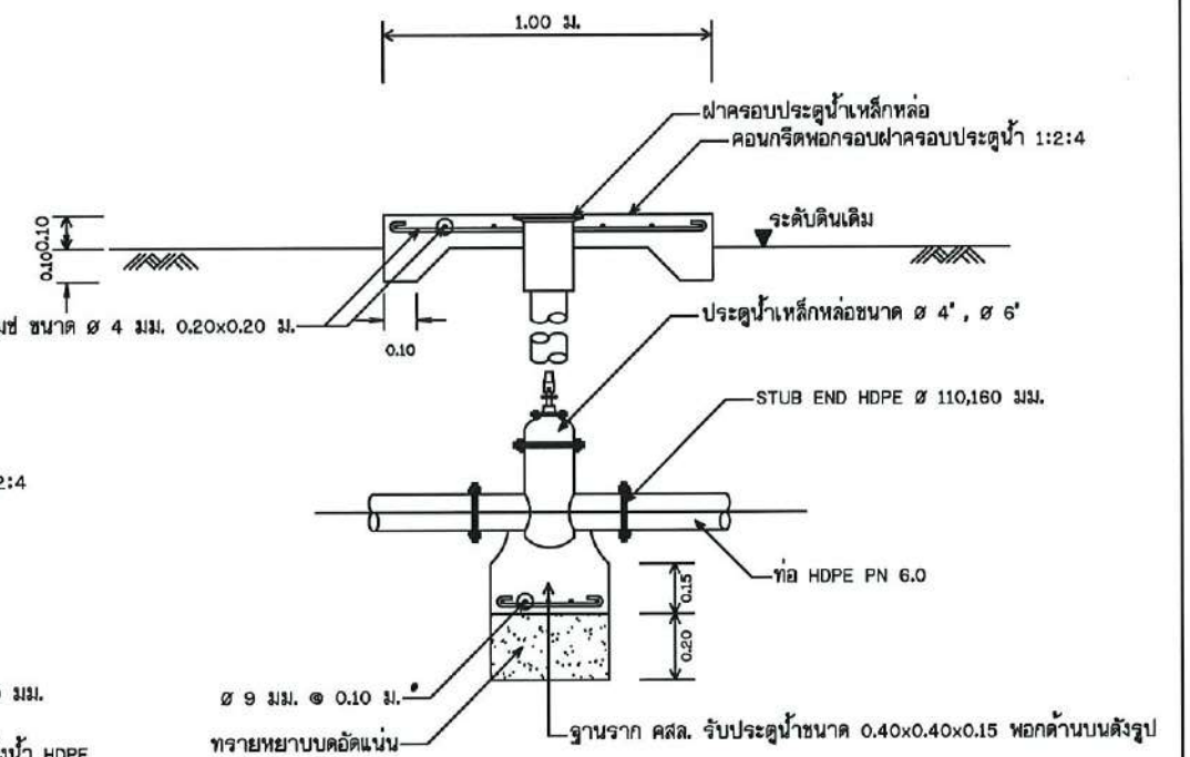
รูปตัด ค - ค แสดงการติดตั้งประตุน้ำใต้ดิน
