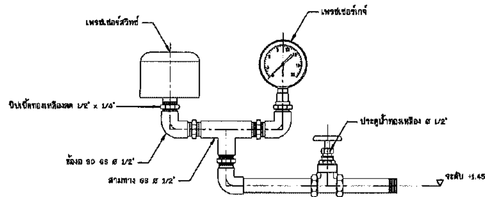
แบบขยายสวิตช์ควบคุมและเกจวัดความดัน ไม่แสดงขนาดส่วน
