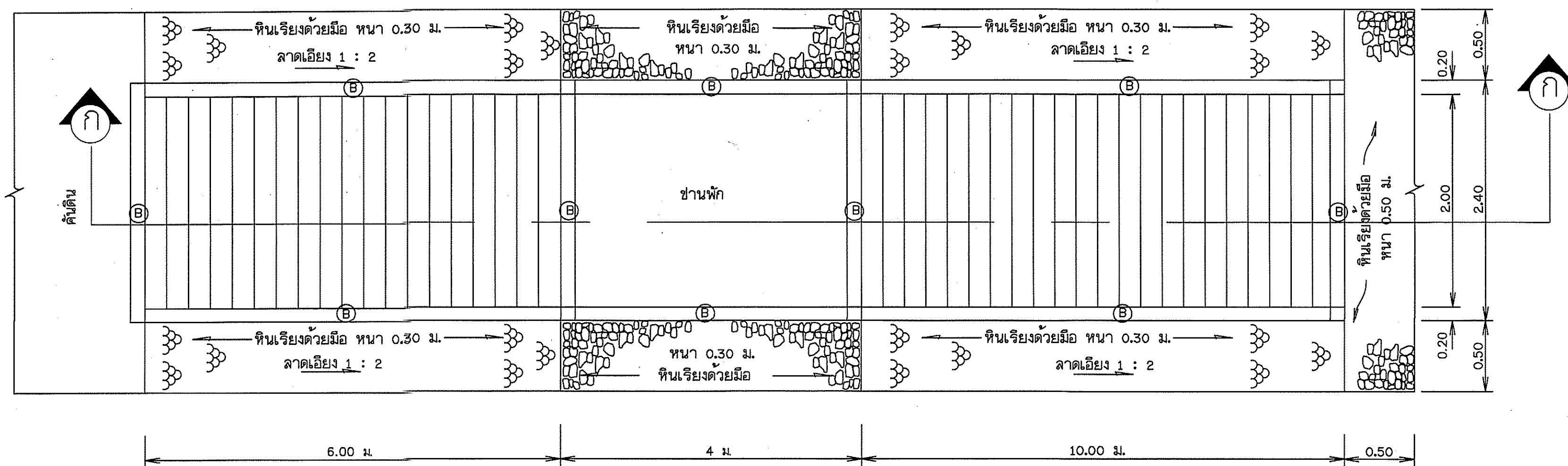
แบบบ้านโด คสล. แบบมีชานพัก
