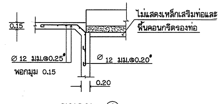
ขยาย (4) ไม่แสดงมาตราส่วน
