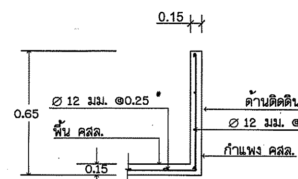
รูปตัด (ค) - (ค) (ความหนาพื้น 0.15 ม.) ไม่แสดงมาตราส่วน
