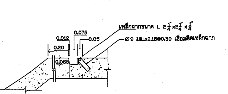
ขยายร่องใส่บานประตูไม้ ไม่แสดงมาตราส่วน
