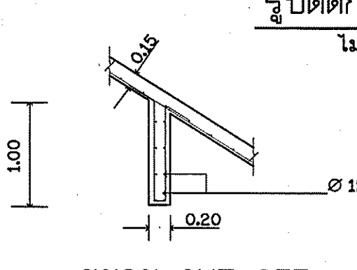
ขยาย CUT OFF ไม่แสดงมาตราส่วน
