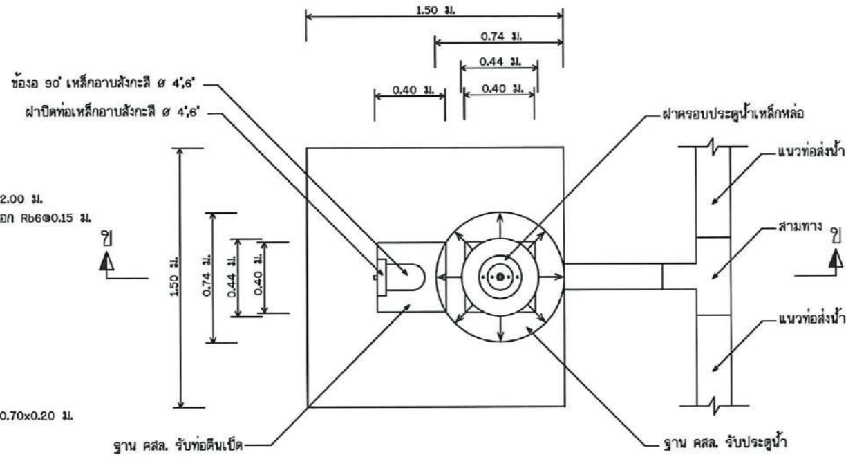
แปลนประตูละลายตะกอน มาตรฐาน No Scale
