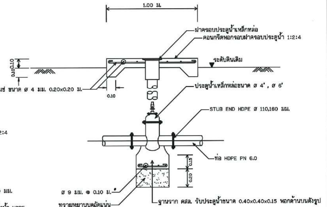
รูปตัด ค - ค แสดงการติดตั้งประตูละลายตะกอนใต้ดิน มาตรฐาน No Scale
