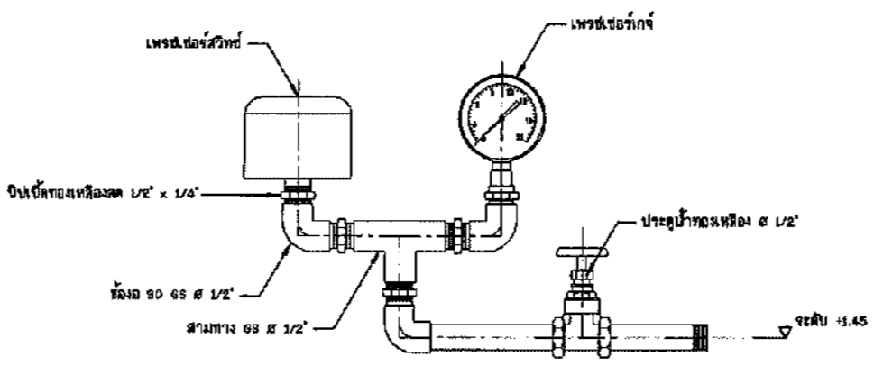
แบบขยายสวิตช์ควบคุมและแก้วัดความดัน ไม่แสดงขนาดจั่วส่วน
