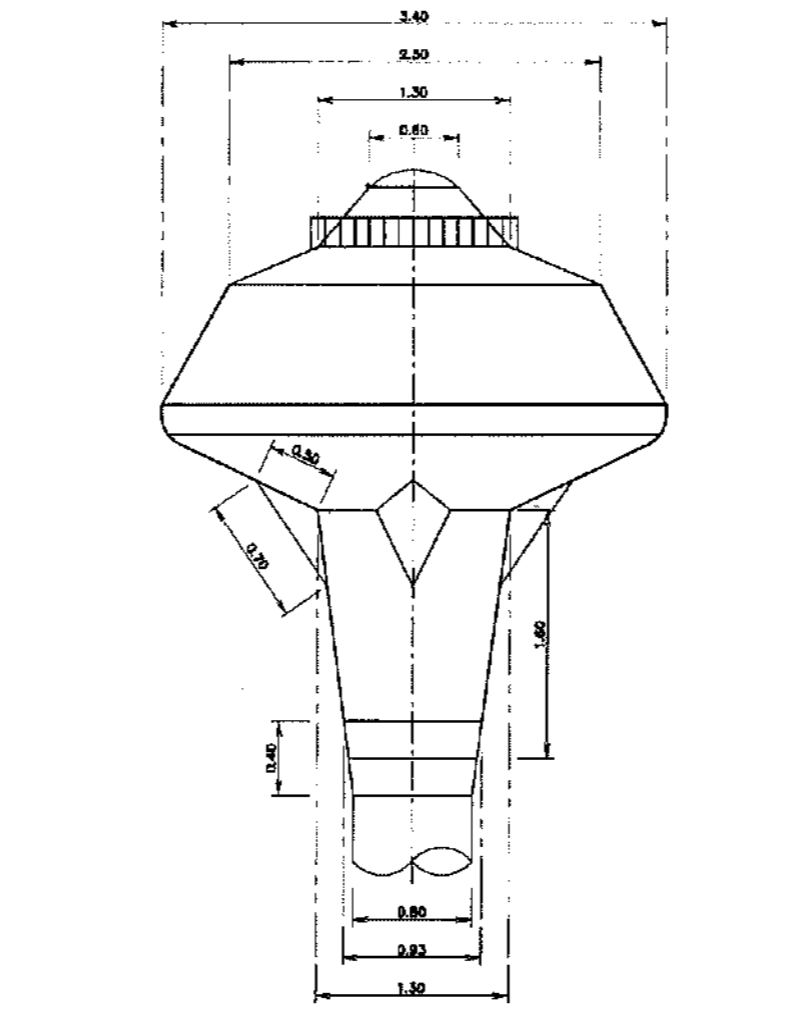
แบบขยายแมนโฮลสูง ไม่แสดงขนาดบางส่วน
