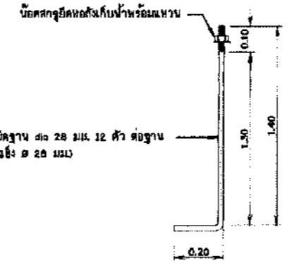
แบบขยายสลักเกลียวยึดฐาน
