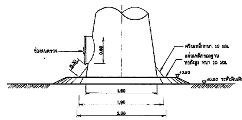
แบบขยายแมนโฮลต่ำ ไม่แสดงขนาดบางส่วน
