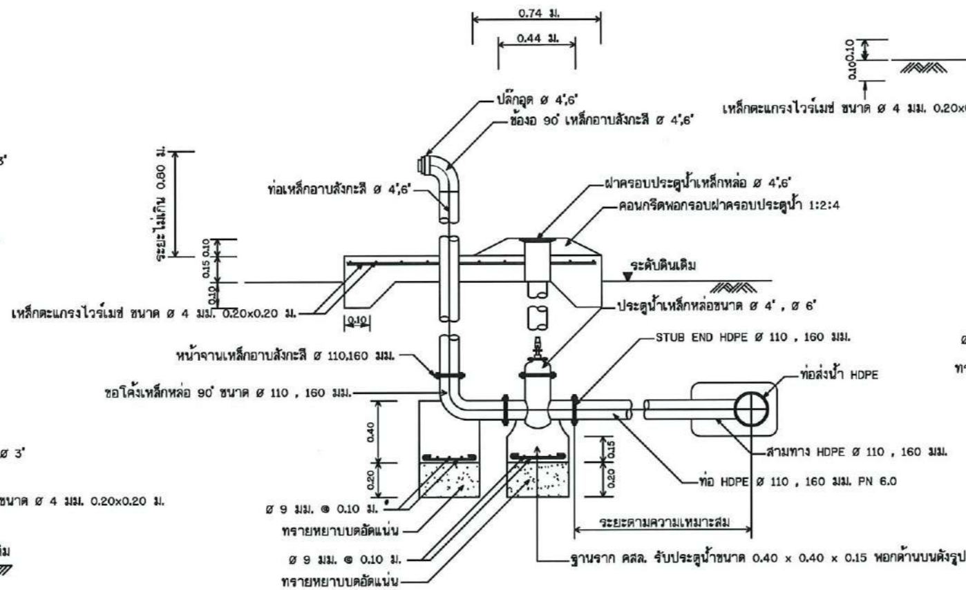
รูปตัด ข - ข แสดงการติดตั้งประตูละลายตะกอน มาตรฐาน No Scale
