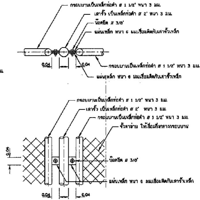
แบบขยายรายละเอียดแสดงการยึดระหว่างซี่ลวดกับเสา ไม่แสดงมาตราส่วน
