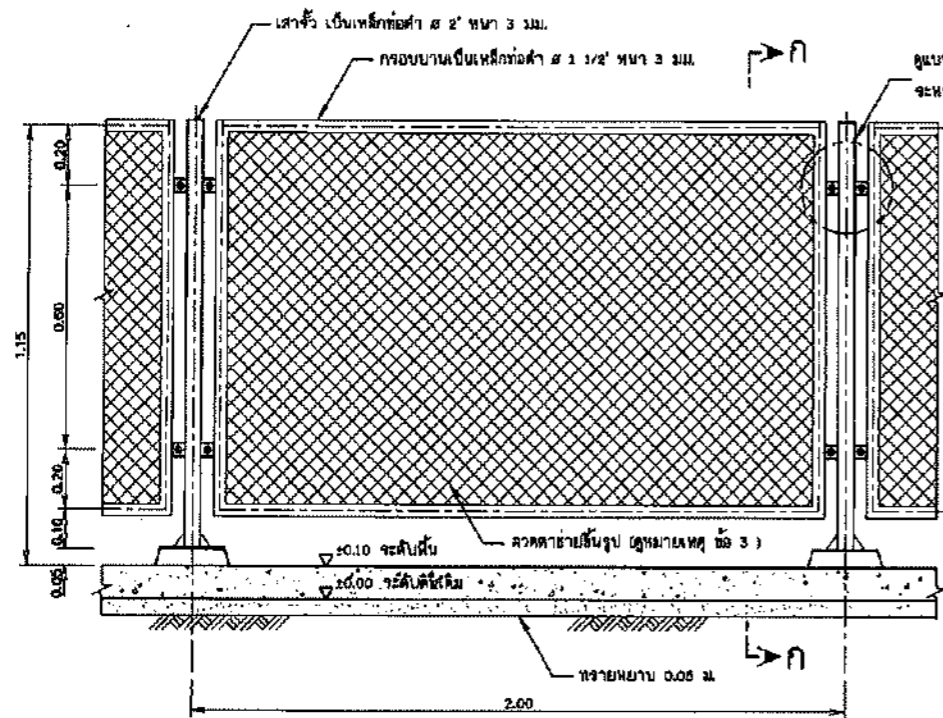
แบบขยายซี่ลวดตาข่าย ไม่แสดงมาตราส่วน
