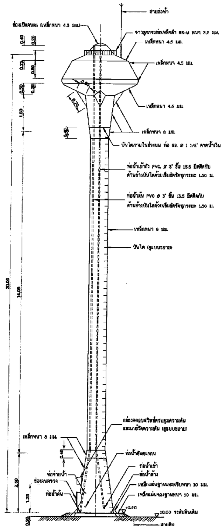
รูปด้านข้างท่อถังสูง แบบถังเหล็กรูปทรงแปมแปญ ไม่แสดงขนาดบางส่วน
