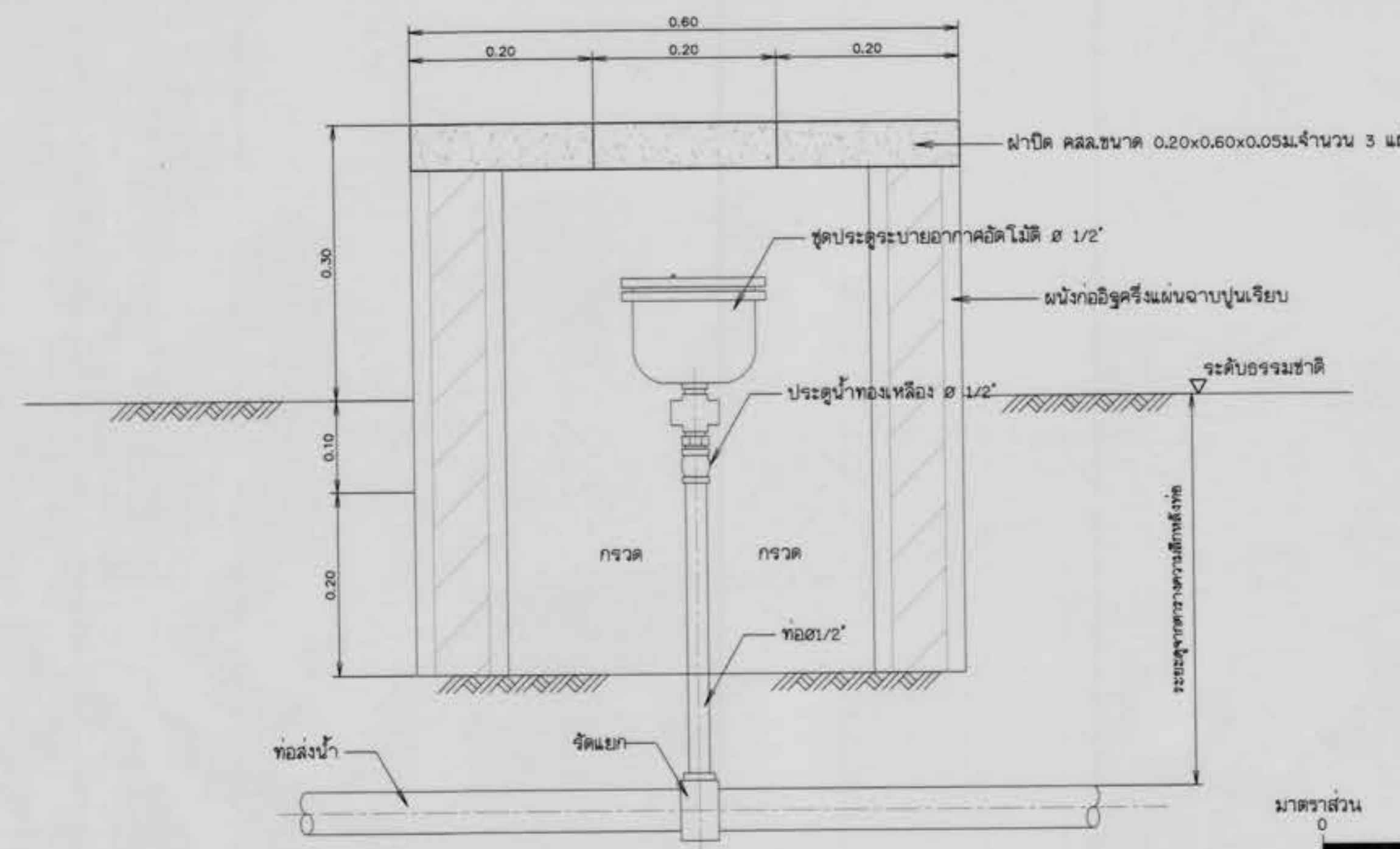
12 การติดตั้งประตูระบายอากาศอัตโนมัติ มาตราส่วน 1:5
