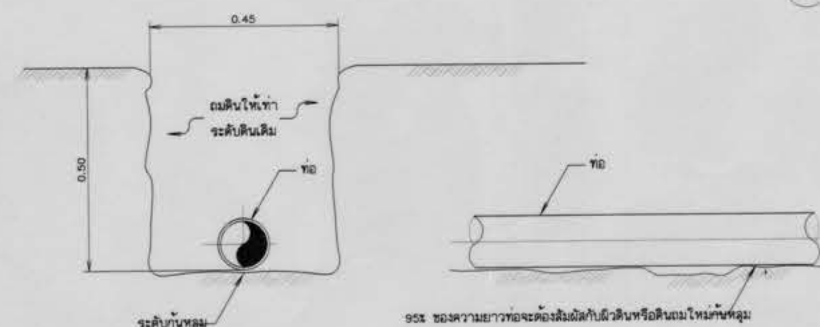
1. แบบการวางท่อทั่วไป ไม่แสดงมาตราส่วน
