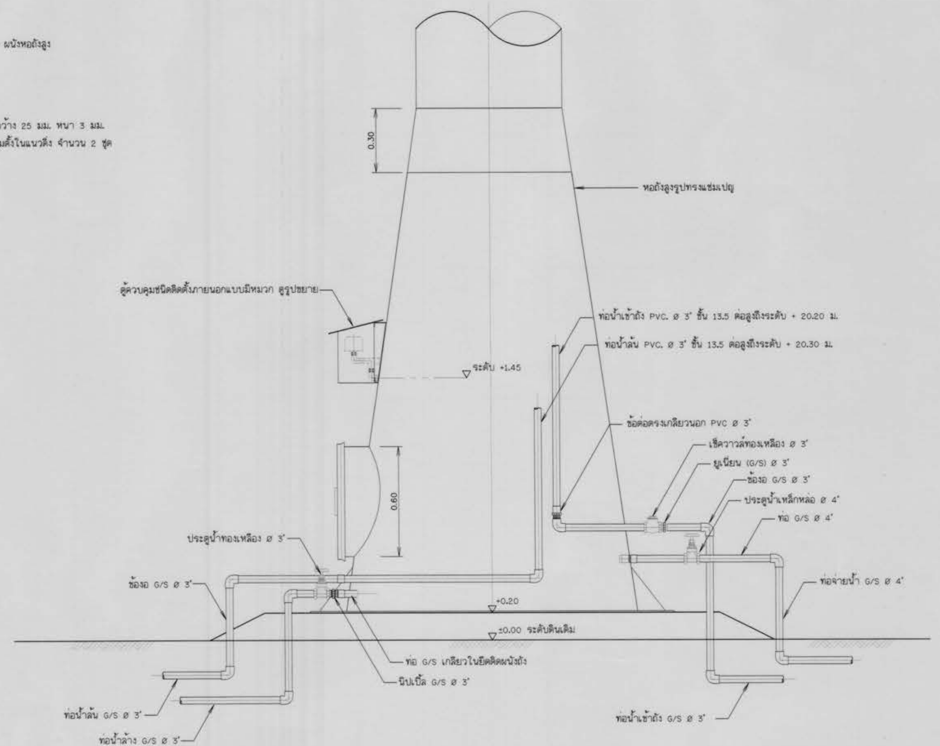
แบบแสดงการเดินท่อในหอถังสูง ไม่แสดงมาตราส่วน
