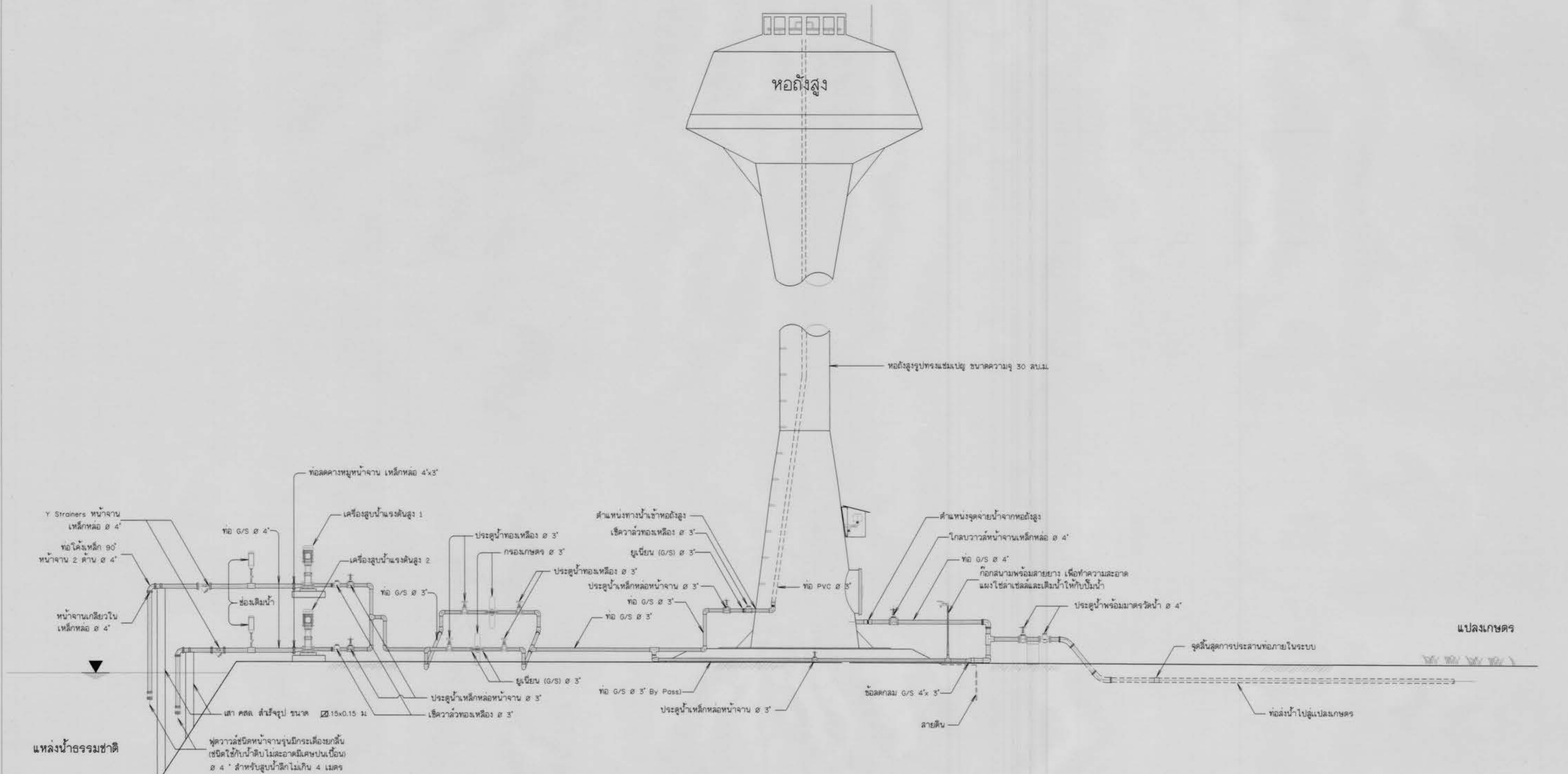
รูปแสดงรายละเอียดท่อและอุปกรณ์ระบบสูบน้ำพลังงานแสงอาทิตย์ ไม่แสดงขนาดราส่วน
