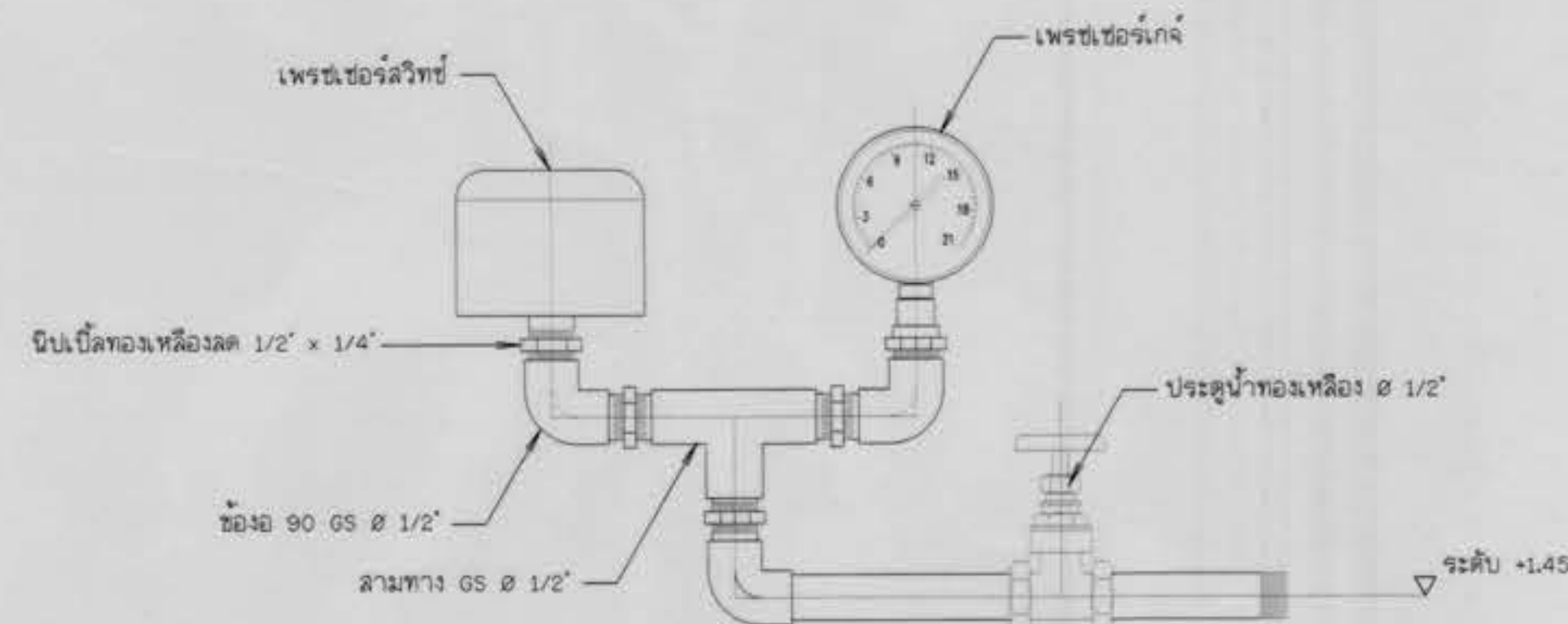
แบบขยายสิทธิ์ควบคุมและเกื้อวัดความดัน
