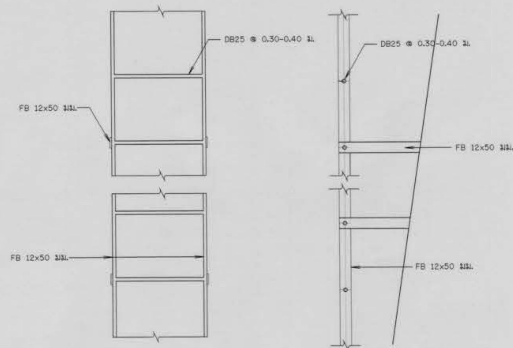
แบบขยายบันได ภายในห้องถึงสูง
