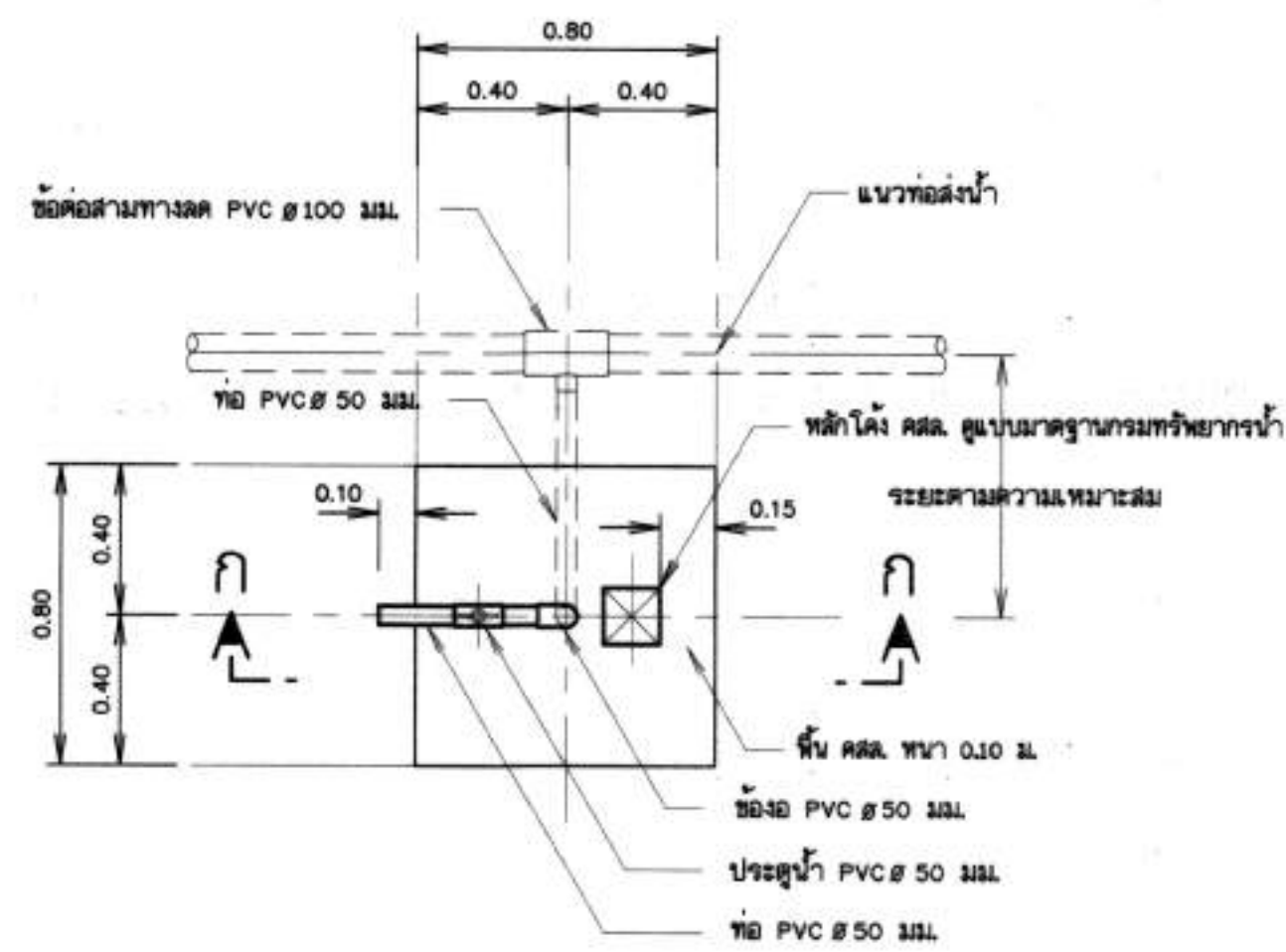
แปลนอาคารจุดปล่อยน้ำ (แบบ ก) xx
