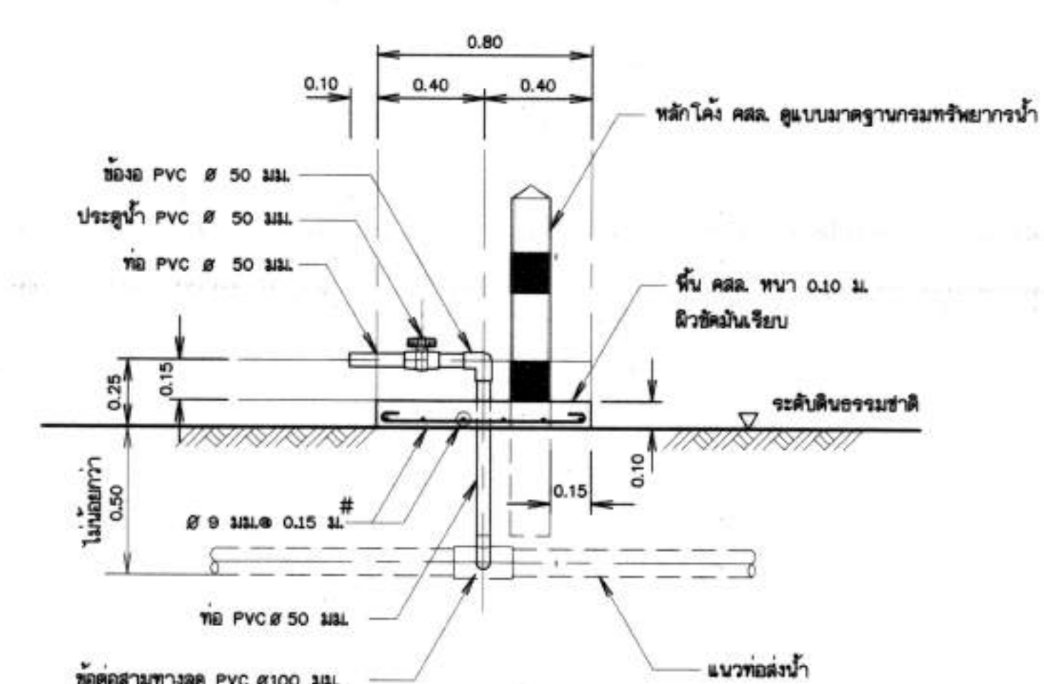
รูปตัด ก - ก แสดงการติดตั้งประตุน้ำปล่อยน้ำ
