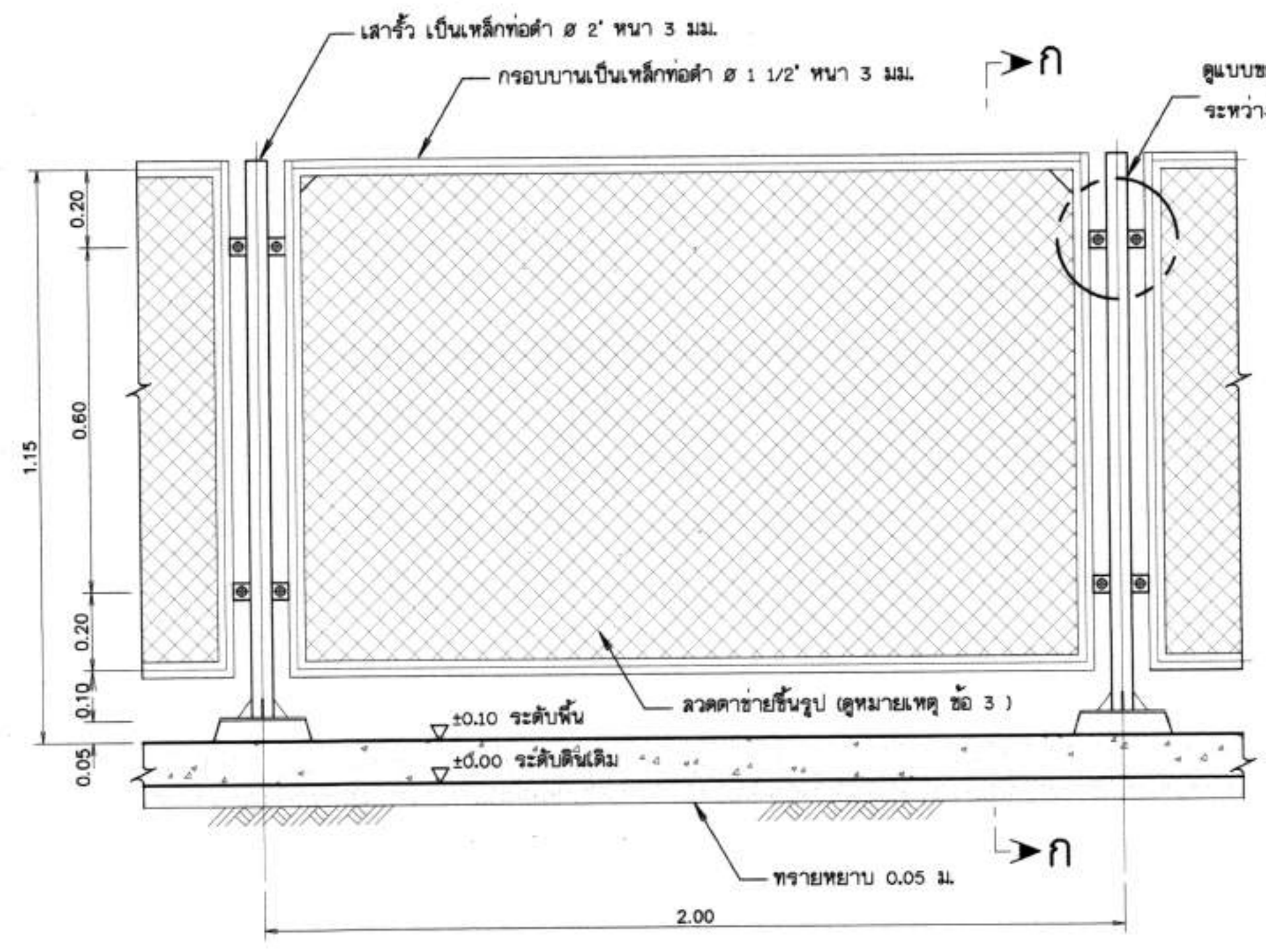
แบบขยายรื้อลวดตาข่าย ไม่แสดงมาตราส่วน
