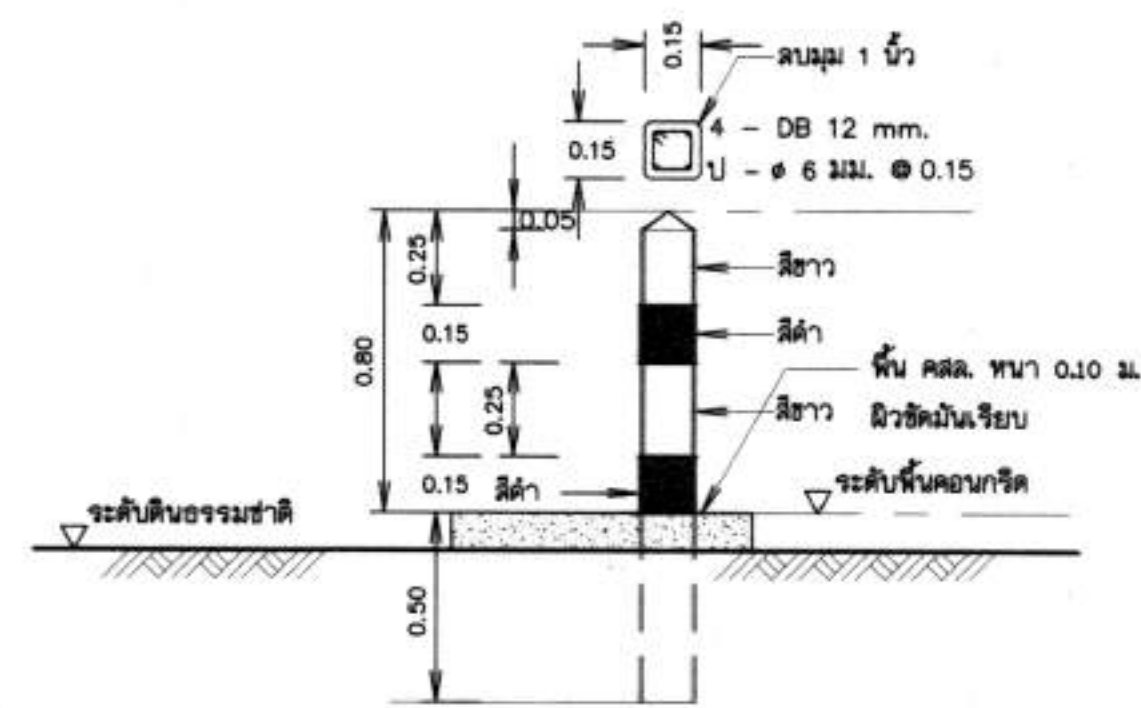
แบบขยาย หลักโคง คสล.
