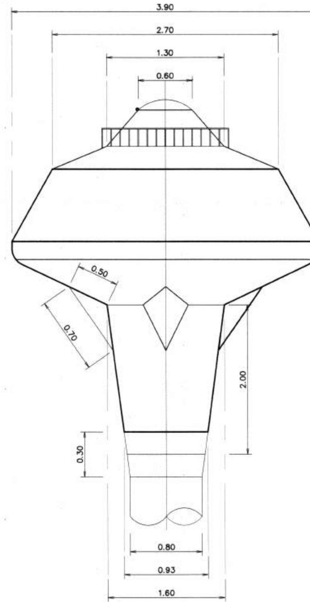
แบบขยายแมนโฮลบนหอถังสูง ไม่แสดงมาตราส่วน
