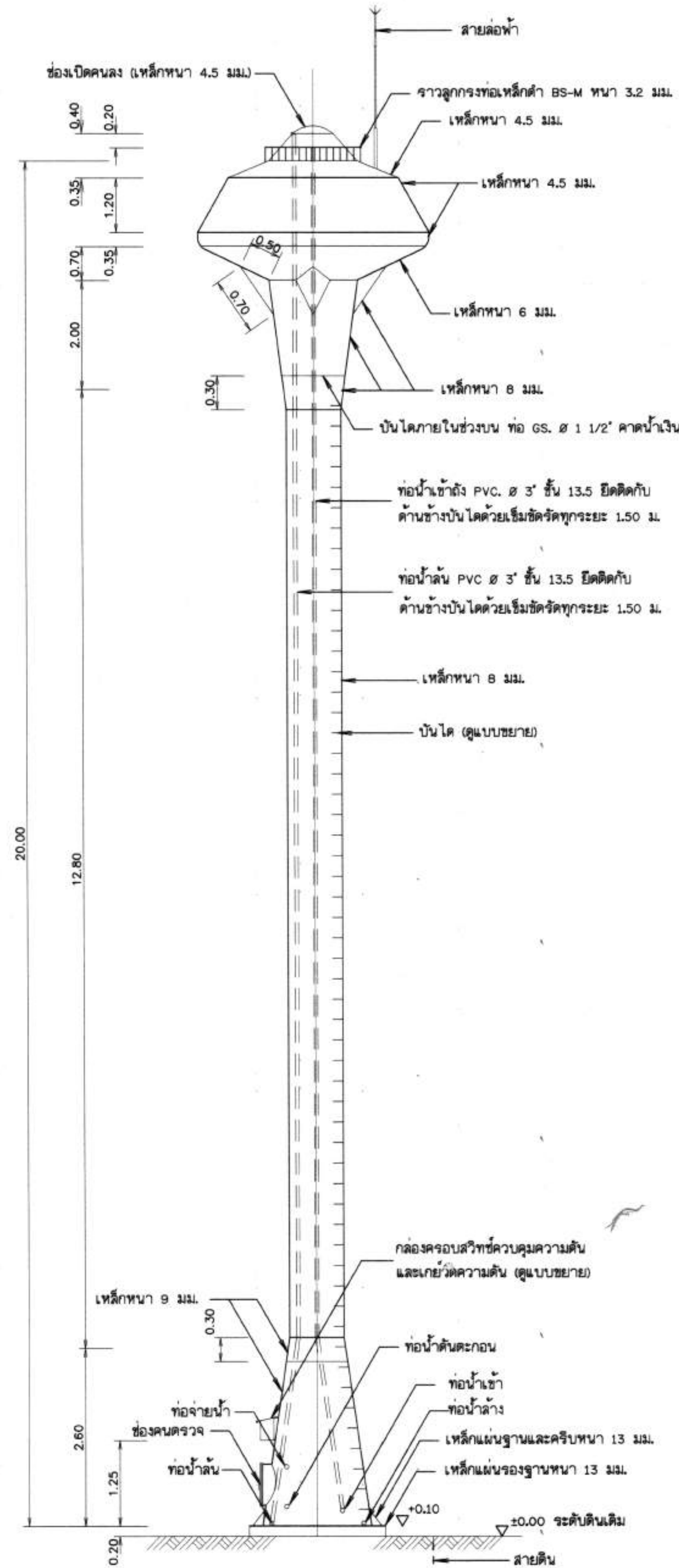
รูปด้านข้างหอถังสูง แบบถังเหล็กรูปทรงแปมเปญ ไม่แสดงมาตราส่วน
