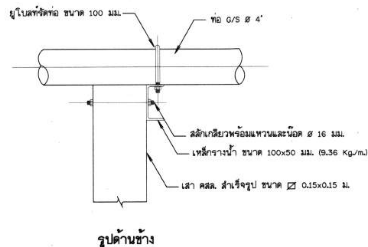
13. เสาดอม่อรับท่อชุด และแบบขยายอุปกรณ์วัดท่อ ไม่แสดงขนาดราส่วน
