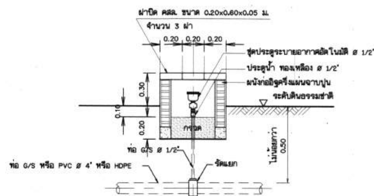
การติดตั้งประตุน้ำระบายอากาศอัตโนมัติ
