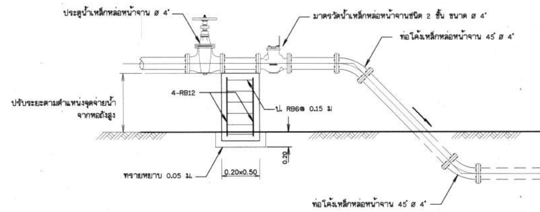
14. การติดตั้งมาตรวัดน้ำบนพื้นดิน Ø 4" ไม่แสดงขนาดราส่วน
