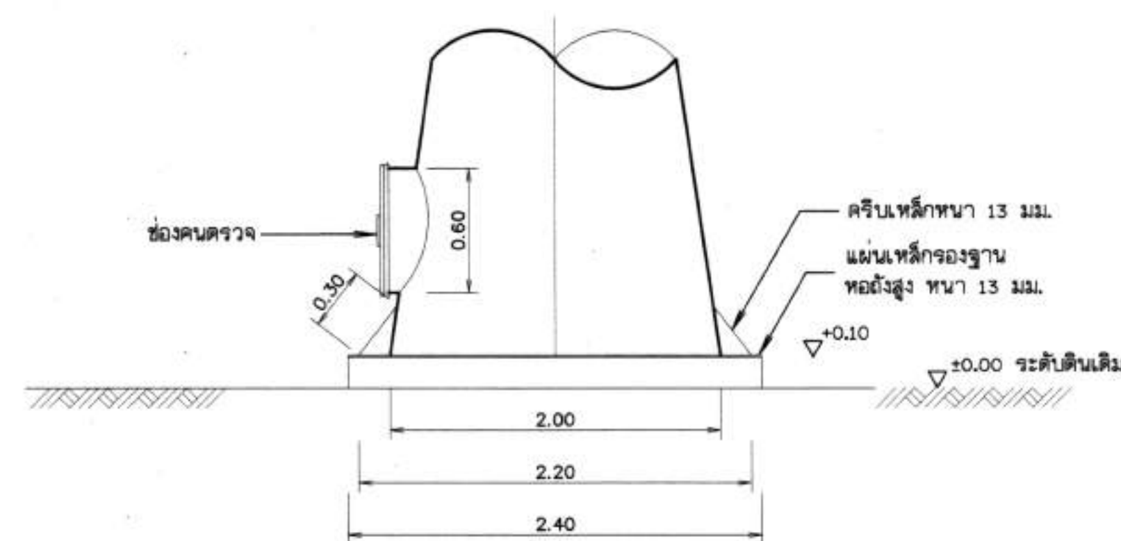
แบบขยายแมนโฮลล่างหอถังสูง ไม่แสดงมาตราส่วน
