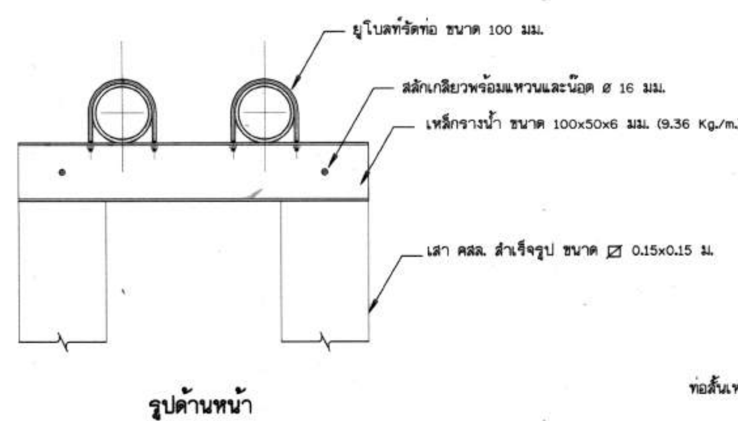
13. เสาดอม่อรับท่อชุด และแบบขยายอุปกรณ์วัดท่อ ไม่แสดงขนาดราส่วน
