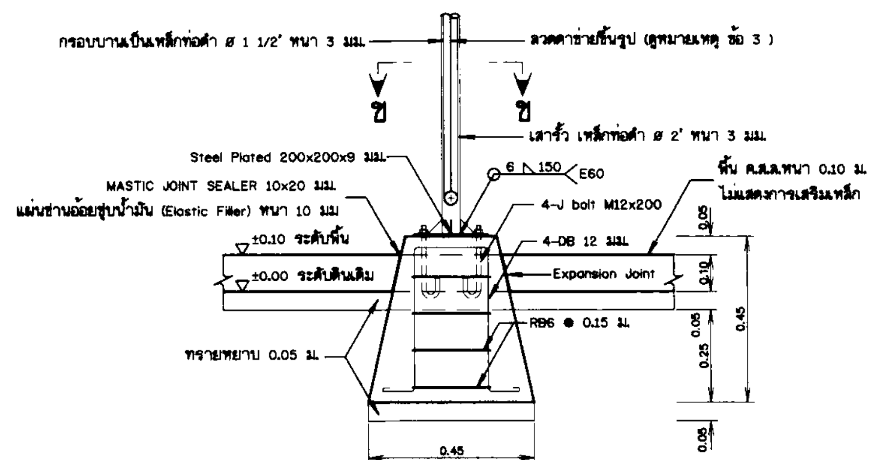
รูปขยายฐานรากโครงสร้างรับแผง F1 (คอมม. ค.ส.ล. ท่อสำเร็จรูปพร้อมติดตั้ง) ไม่แสดงขนาดราส่วน
