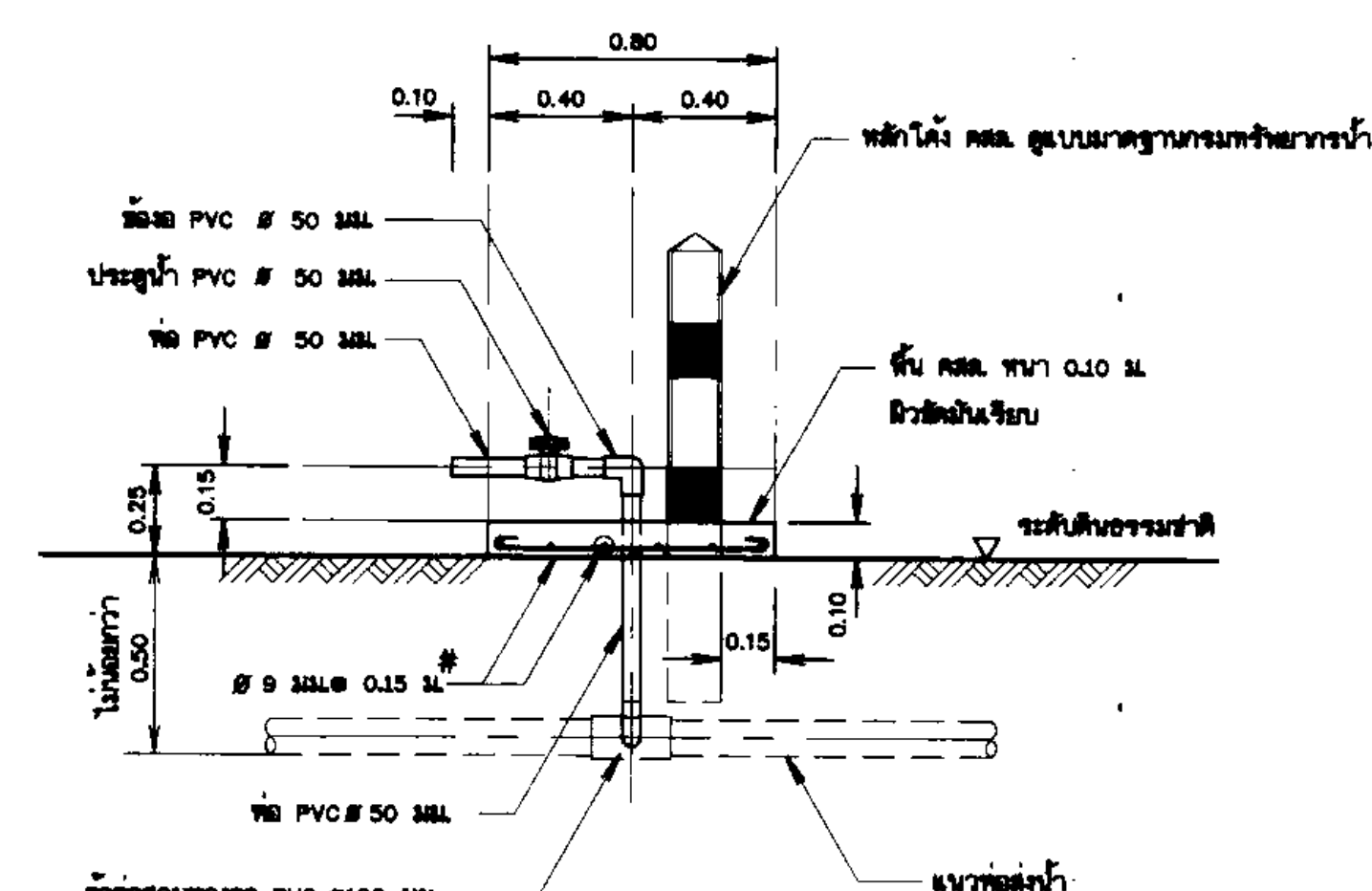
รูปตัด ก - ค แสดงการติดตั้งประตูดปล่อยน้ำ
