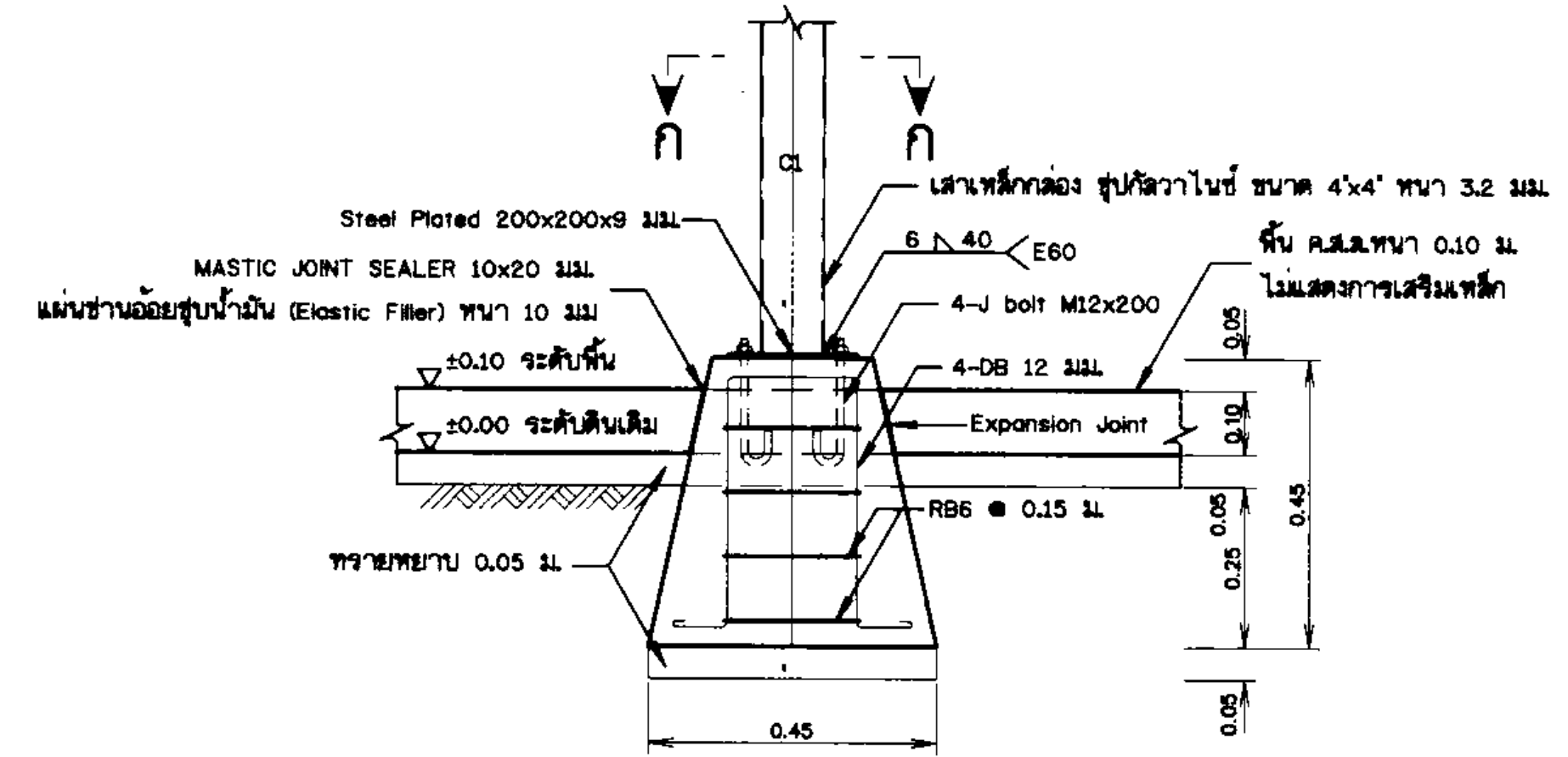
รูปขยายฐานรากโครงสร้างรับแผง F1 (คอมโบ คสล. ท่อสำหรับพรมองเห็นค้ำ) ไม่แสดงมาตราส่วน
