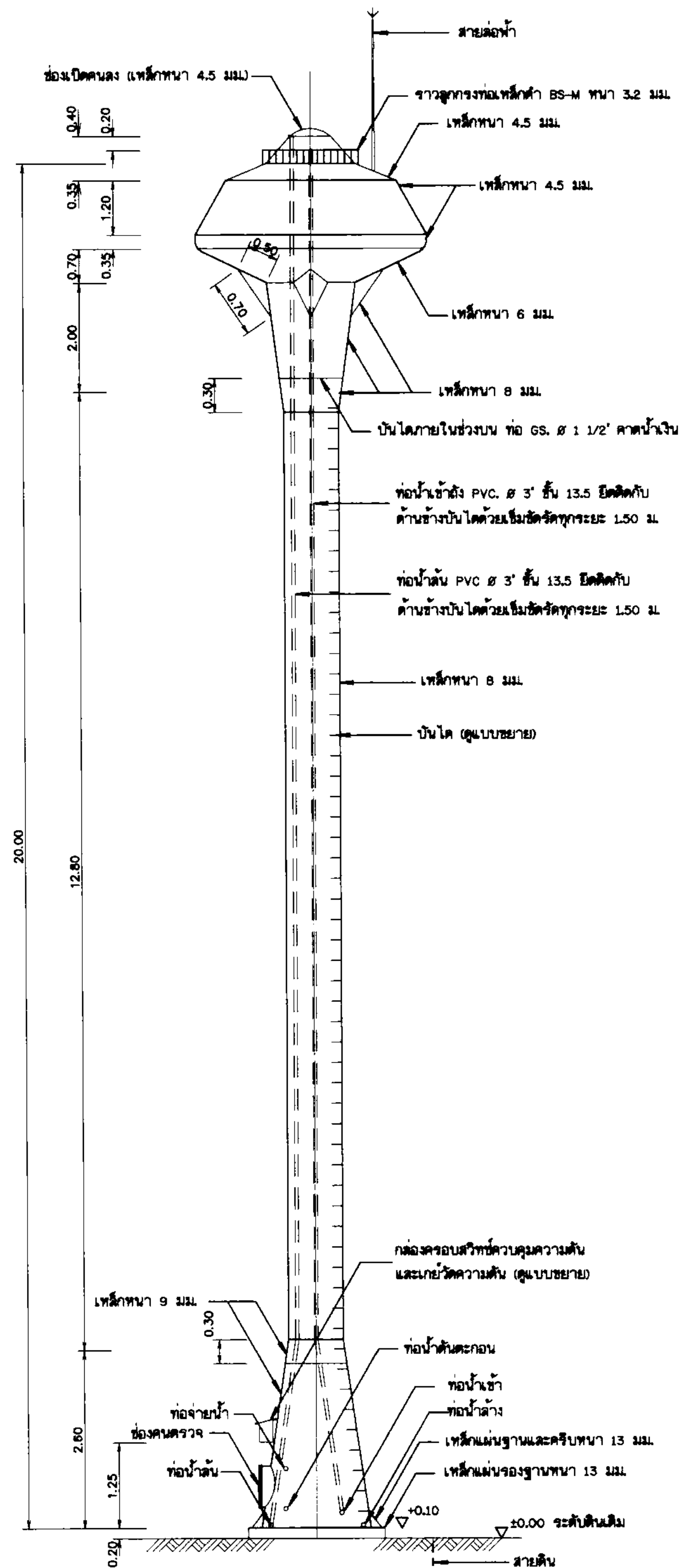
รูปด้านข้างท่อถึงสูง แบบถังเหล็กรูปทรงกลมแป้น ไม่แสดงมาตราส่วน
