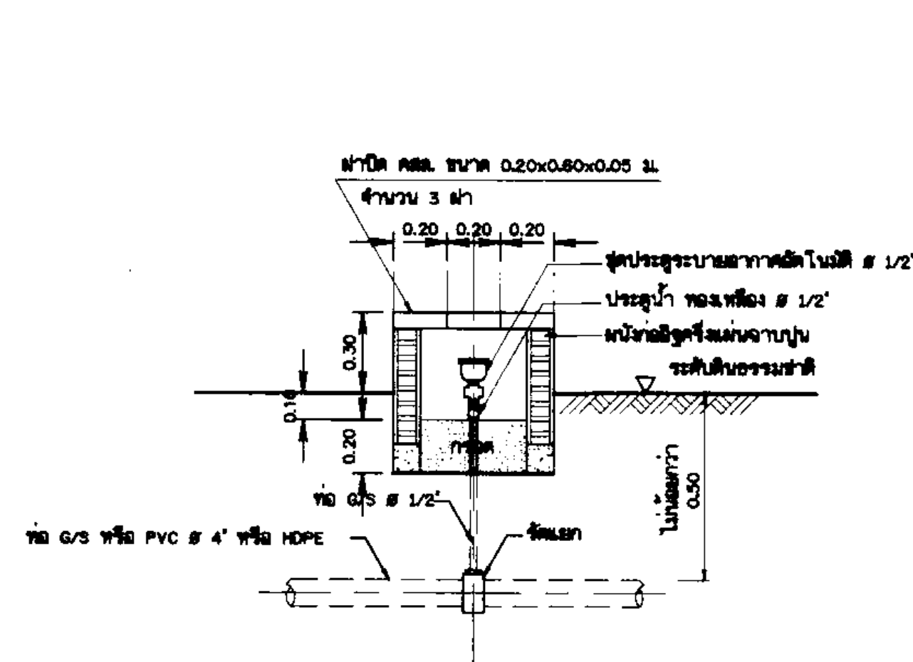
การติดตั้งประตูระบายอากาศอัตโนมัติ
