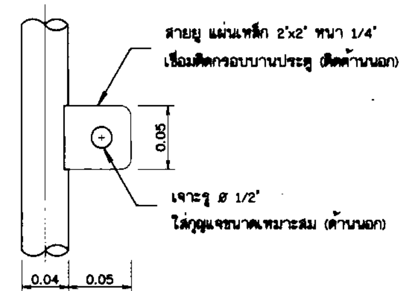
แบบขยายสายยู ไม่แสดงขนาดราส่วน
