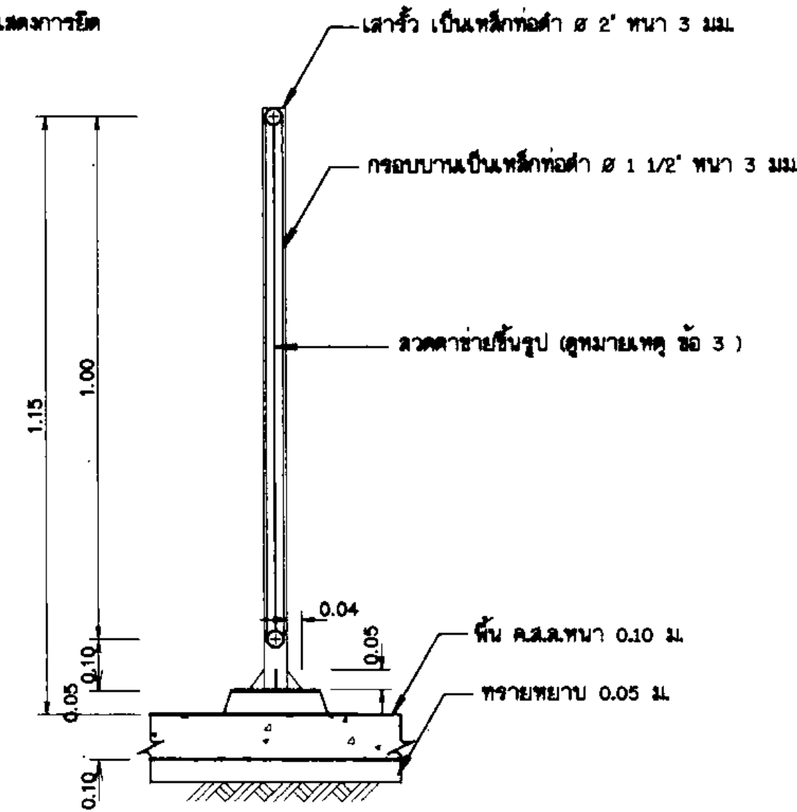
รูปตัด ก-ก ไม่แสดงขนาดราส่วน
