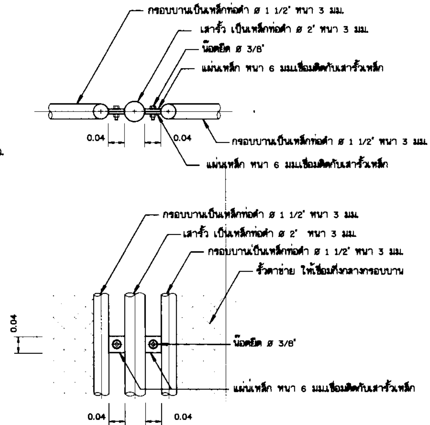
แบบขยายรายละเอียดแสดงการยึดระหว่างหัวกับเสา ไม่แสดงขนาดราส่วน
