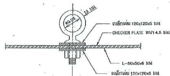
รูปขยายห่วงยึดแพสบูบน้ำ มาตราส่วน 1 : 5
