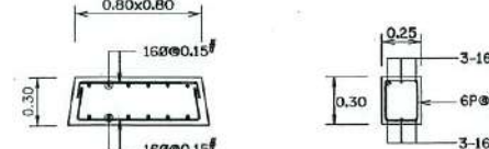
รูปตัด 17-17 รูปตัด 18-18
