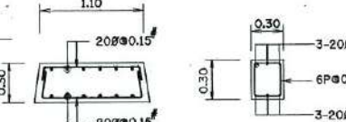
รูปตัด 9-9 รูปตัด 10-10
