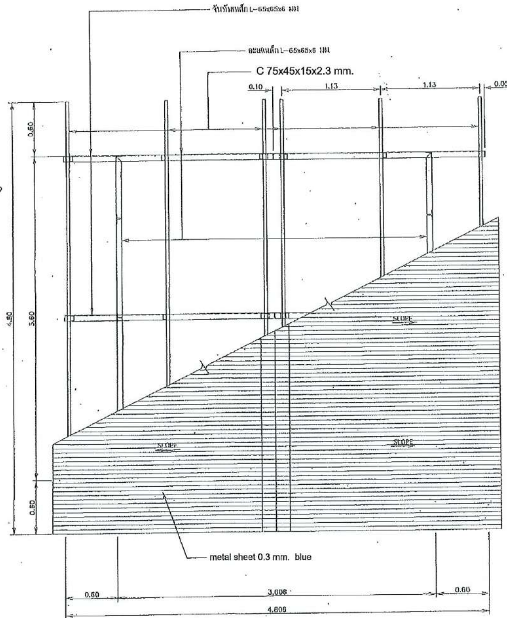
แปลนโครงสร้าง
