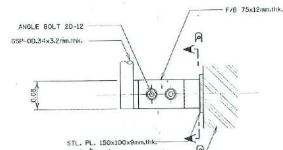
แบบขยาย 1 มาตราส่วน 1:5
