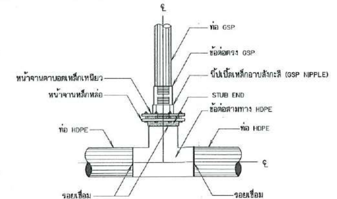
การบรรจุท่อสามทาง HDPE กับท่อ GSP แบบข้อต่อ (สำหรับอาคารจุดปล่อยน้ำ อาคารประตูลอยน้ำ อาคารระบายน้ำ อาคารท่อระบายอากาศ กรณีท่อส่งน้ำขนาดเส้นผ่านศูนย์กลางมากกว่า 315 มม.)
