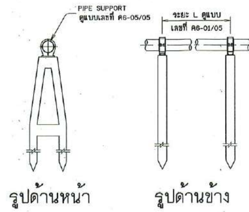
คอมม่อรับท่อแบบที่ 2
