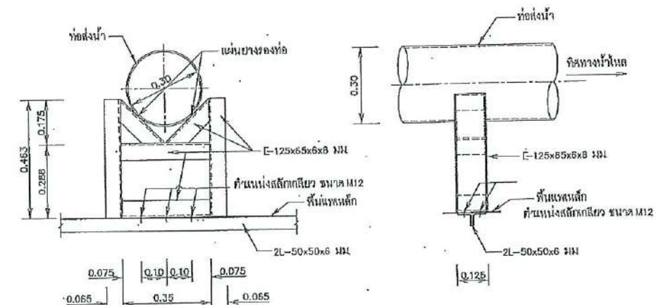
รูปขยาย SUPPORT "B" ไม่แสดงขนาดตัว
