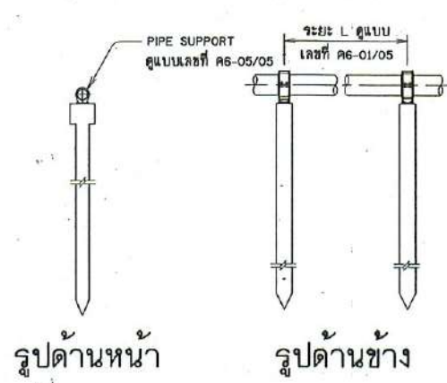
คอมม่อรับท่อแบบที่ 1
