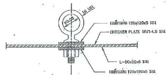
รูปขยายห่วงยึดแพสูบน้ำ
