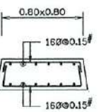
รูปตัด ญ-ญ
