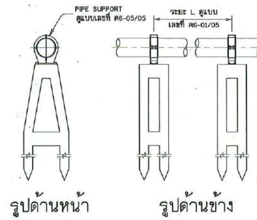
คอมม่อรับท่อแบบที่ 3,4
