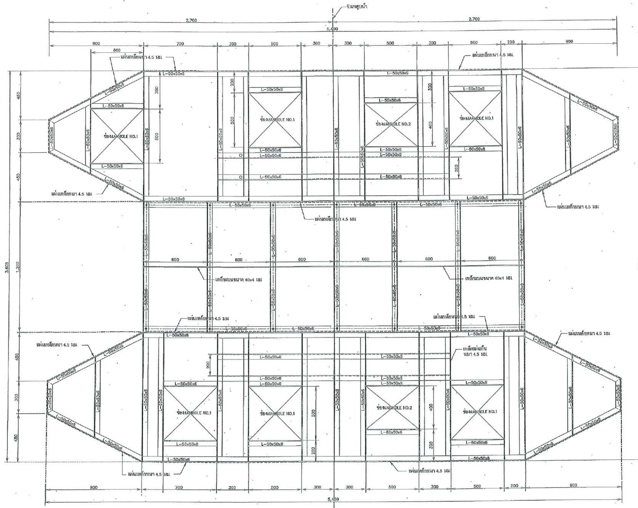
แปลนแสดงโครงเหล็กพื้นบน รวมทุก 1:10
