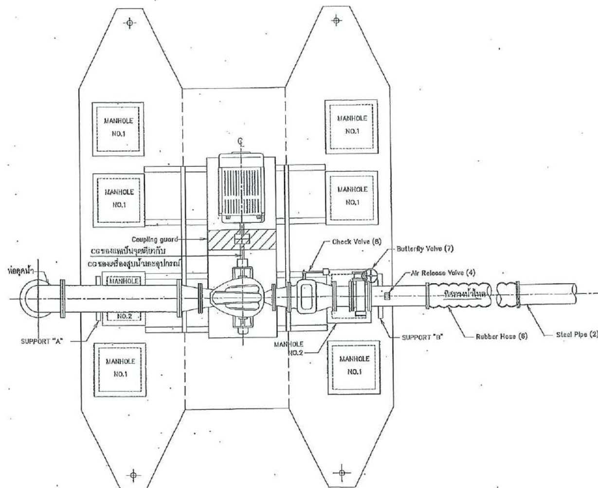
แปลนแสดงการติดตั้งเครื่องสูบน้ำ ไม่แสดงขนาดตัว
