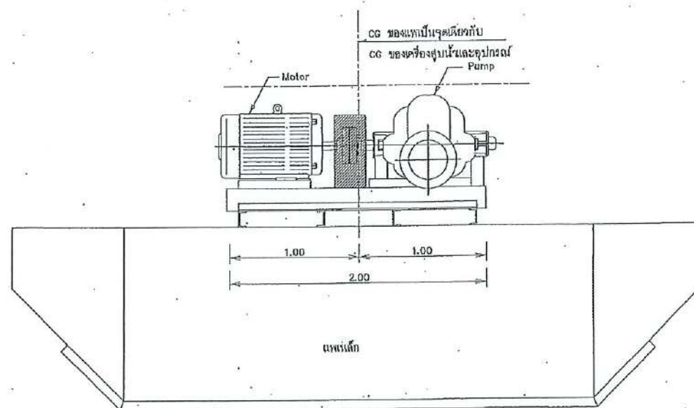
รูปด้านข้าง ไม่แสดงขนาดตัว
