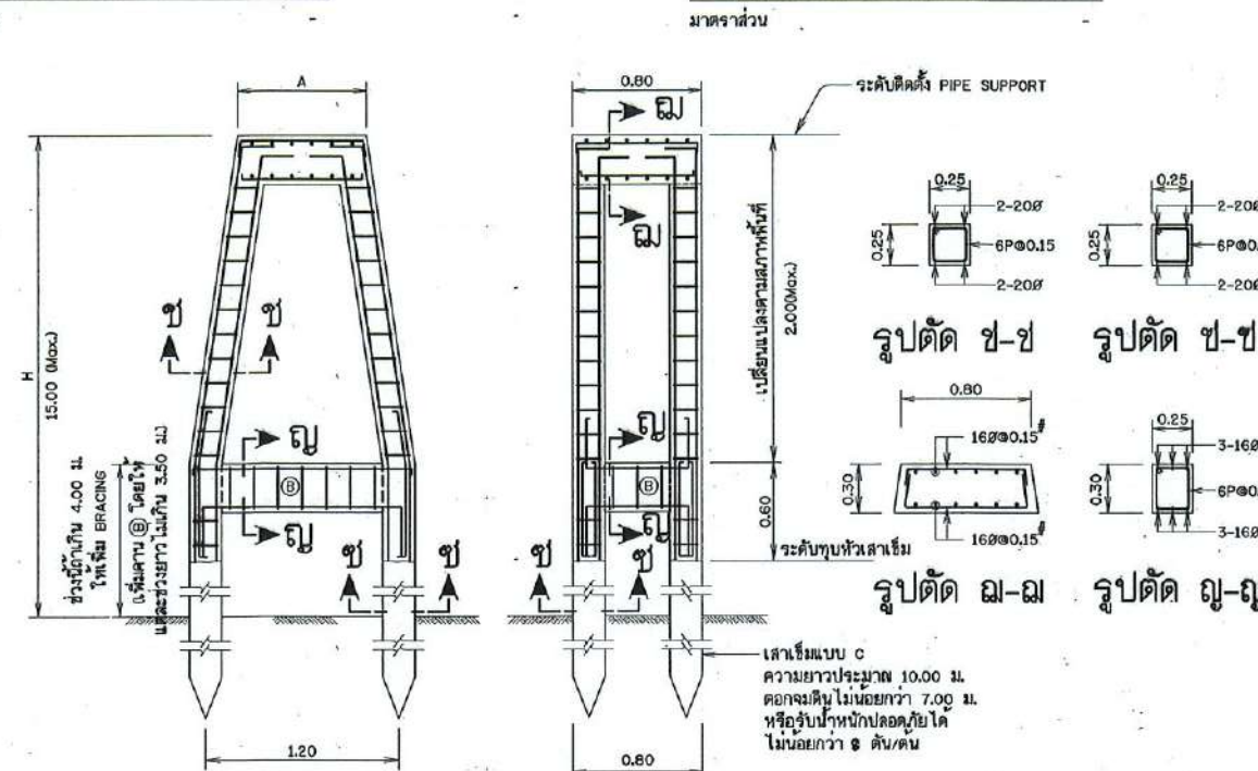
คอมม่อรับท่อแบบที่ 2
