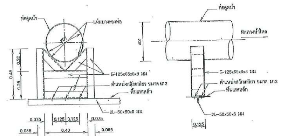
รูปขยาย SUPPORT "A" ไม่แสดงขนาดตัว
