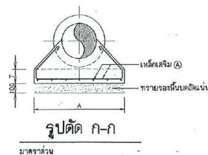
ตารางแสดงมิติและการเสริมเหล็ก THRUST BLOCK รับข้อต่อโค้งแนวตั้ง
