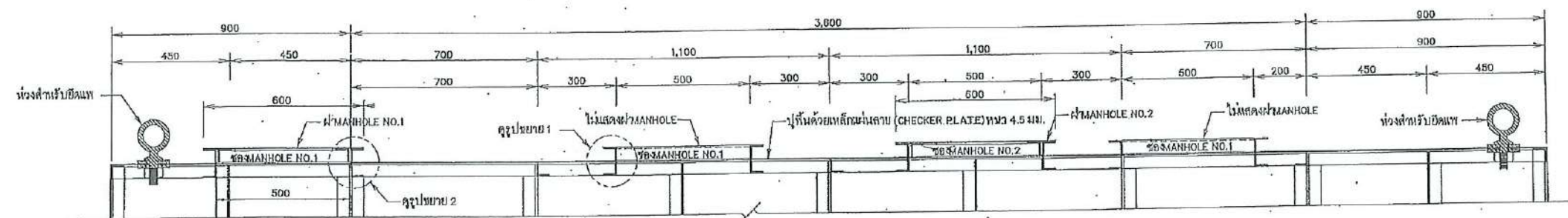
รูปตัด ก - ก. (แสดงรายละเอียดพื้นแบบ) มาตราส่วน 1:10
