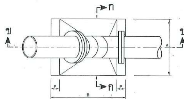
แปลน THRUST BLOCK รับข้อต่อโค้งแนวตั้ง มาตรฐาน (สำหรับท่อเดี่ยว)
