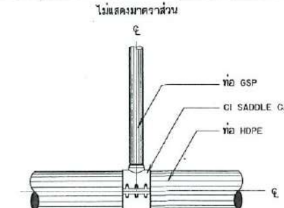
การบรรจุท่อสามทาง HDPE กับท่อ GSP แบบ CI SADDLE CLAMP
