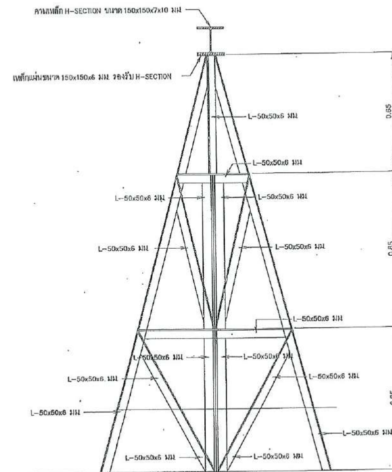
รูปขยายขาตั้งรูปตัว A รับคานาเหล็ก
