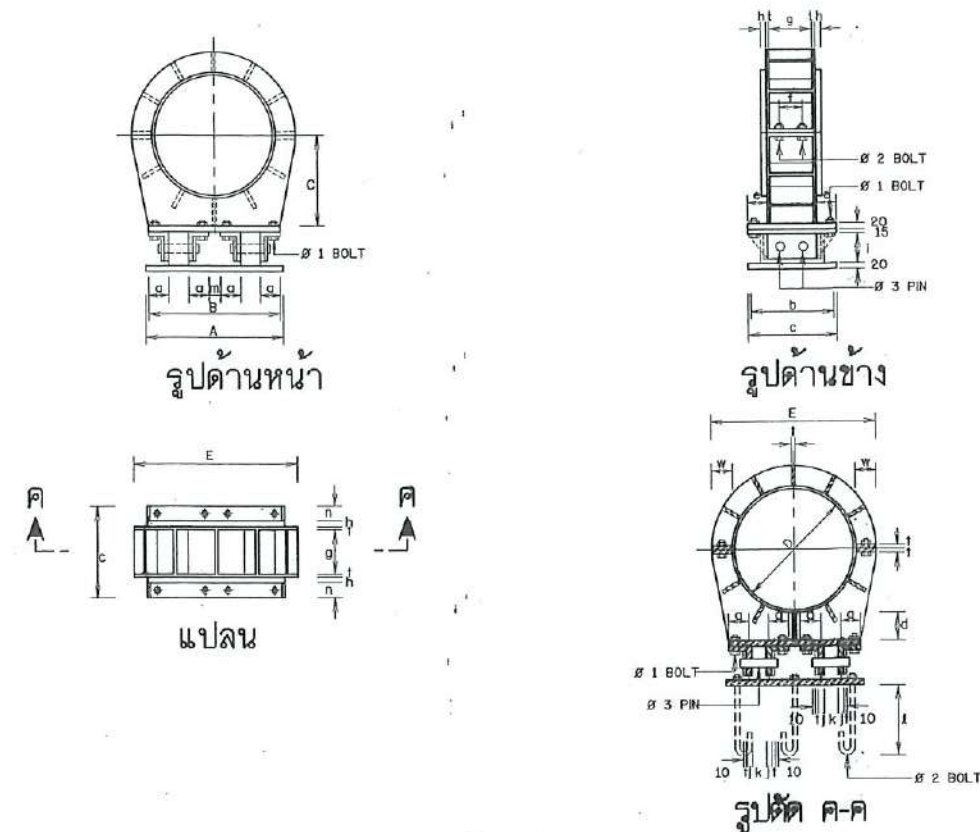
PIPE SUPPORT สำหรับท่อเหล็กขนาด \varnothing 400 มม. - \varnothing 800 มม. มาตรฐาน
