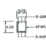
รูปตัด ฎ-ฎ
