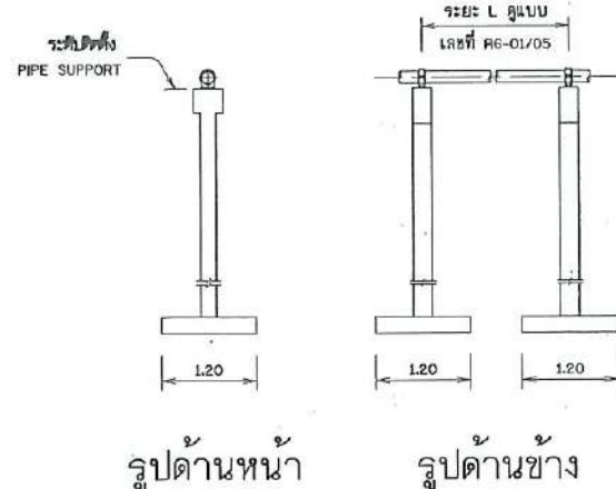
ตอม่อรับท่อแบบที่ 1
