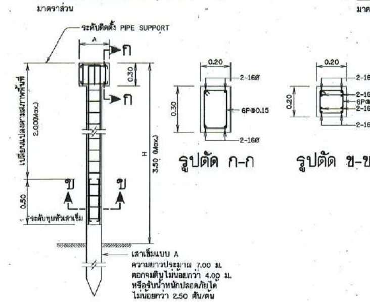
การเสริมเหล็ก คอมม่อแบบที่ 1
