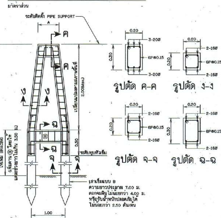
การเสริมเหล็ก คอมม่อแบบที่ 2
