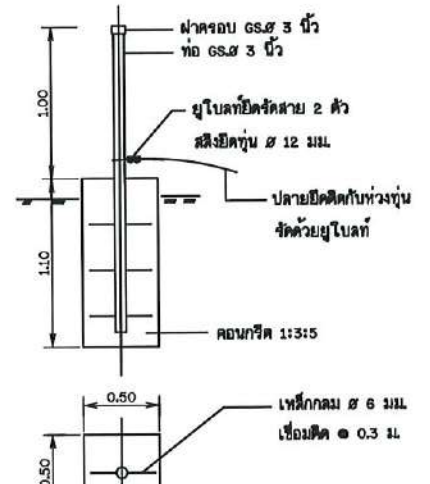
รูปขยายสายยึดแพ มาตราส่วน 1:50
