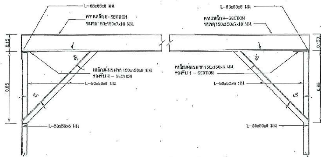
รายละเอียดคานาเหล็กยกเครื่องสูบน้ำ
