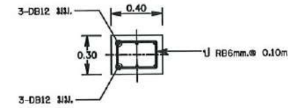
แบบขยายคาน B1
