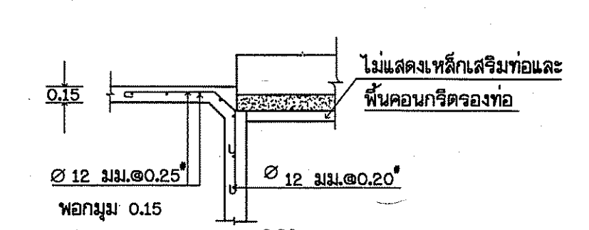
ขยาย (4) ไม่แสดงมาตราส่วน
