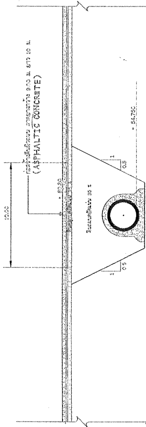
รูปตัดขวางทางระบาย STA.2+07.51-1+216.82
