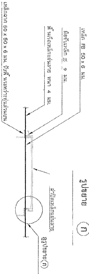
แปลนเหล็กยึดสลึง 1:5
