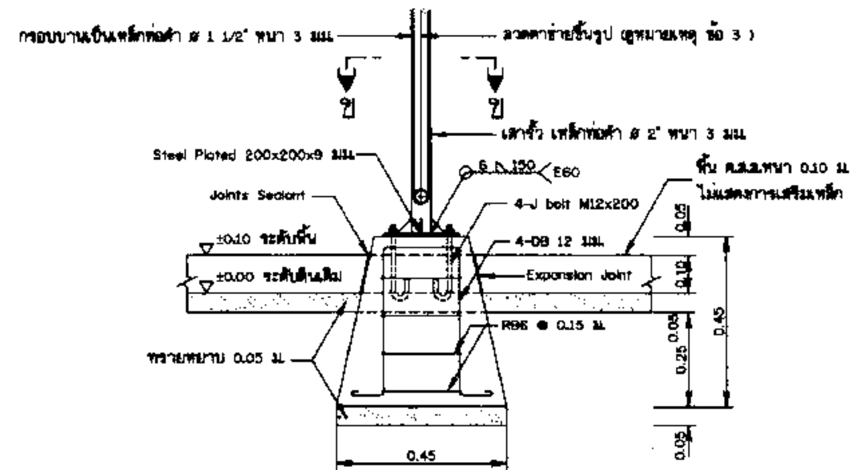
รูปขยายฐานจากโครงสร้างรับแผง F1 (ตามข้อ ค.ค. พร้อมสร้างรูปพร้อมติดคือ) ไม่แสดงมาตราส่วน
