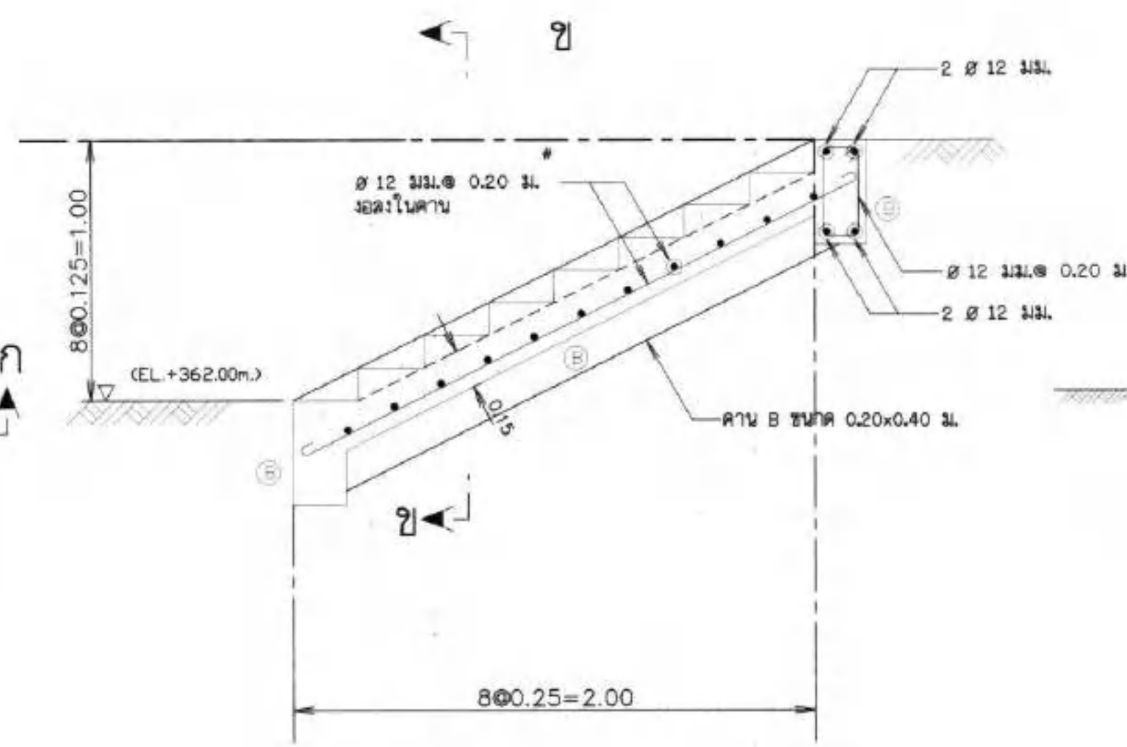
รูปตัดแนว ก - ก
