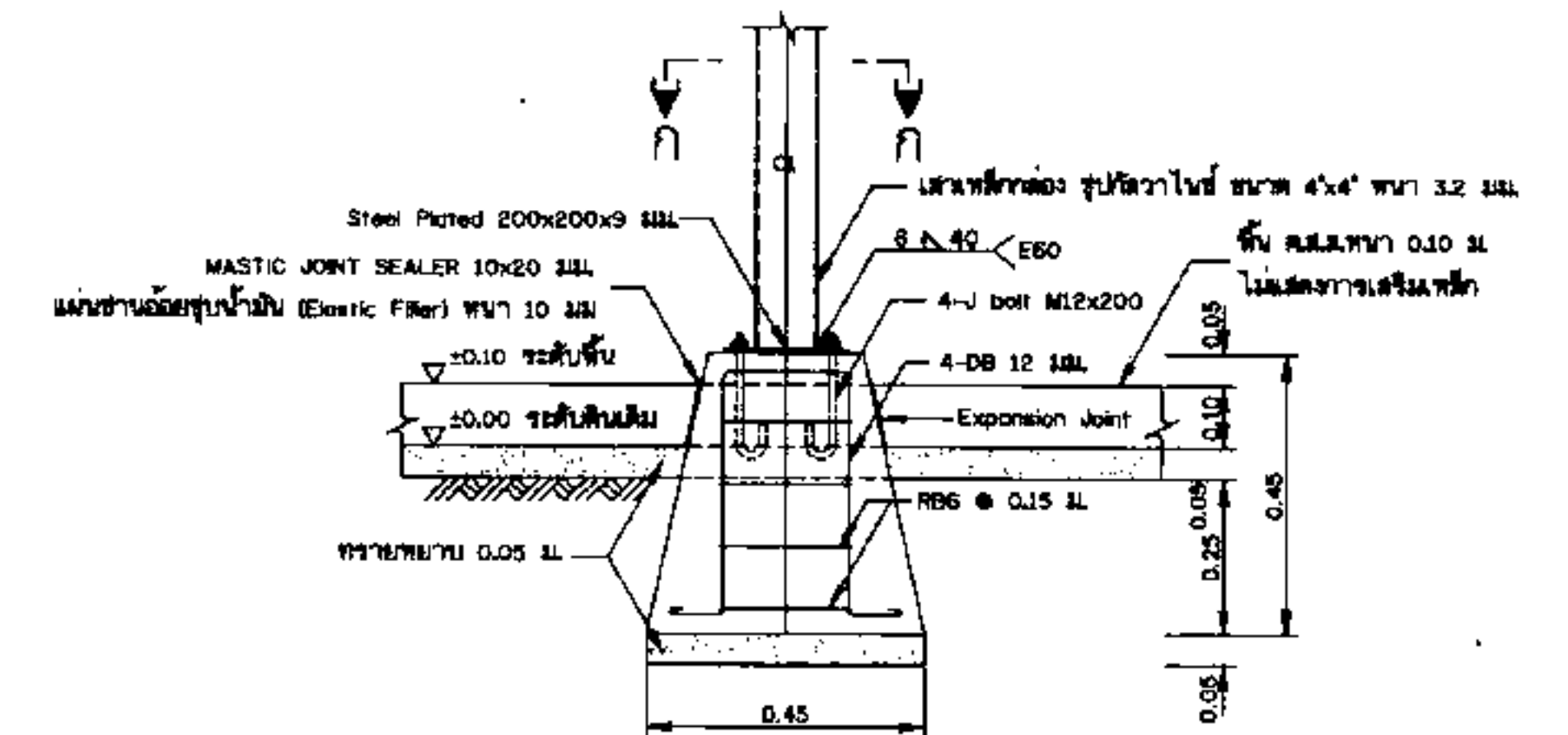
รูปขยายฐานจากโครงสร้างรับแรง F1 ต่อเนื่อง ต่อมา ท่อตันในรูปพร้อมติดตั้ง ไม่แสดงขนาดส่วน
