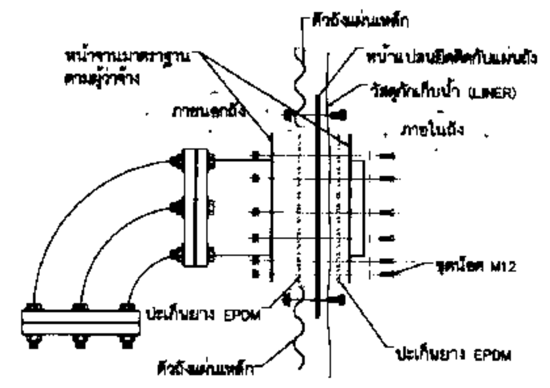
แบบขยาย 5-รูปแบบประกอบท่อน้ำดิบ Scale NTC
