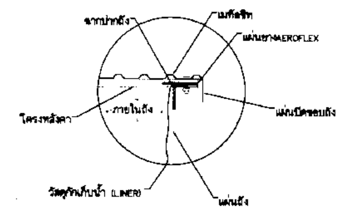
แบบขยาย 3-จุดยึดติดถังกับแผ่นดัง Scale NTC
