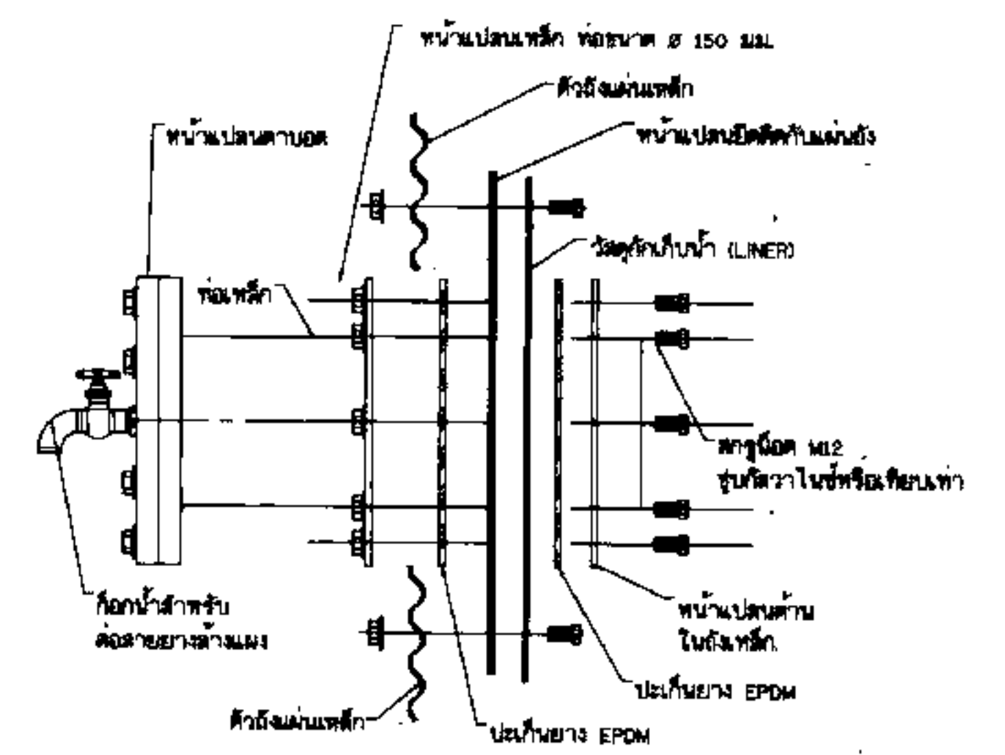
แบบขยาย ท่อน้ำดิบที่ติดกับแผ่นดัง Scale NTC
