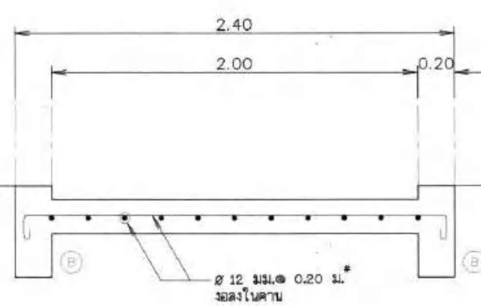
รูปตัดแนว ข - ข
