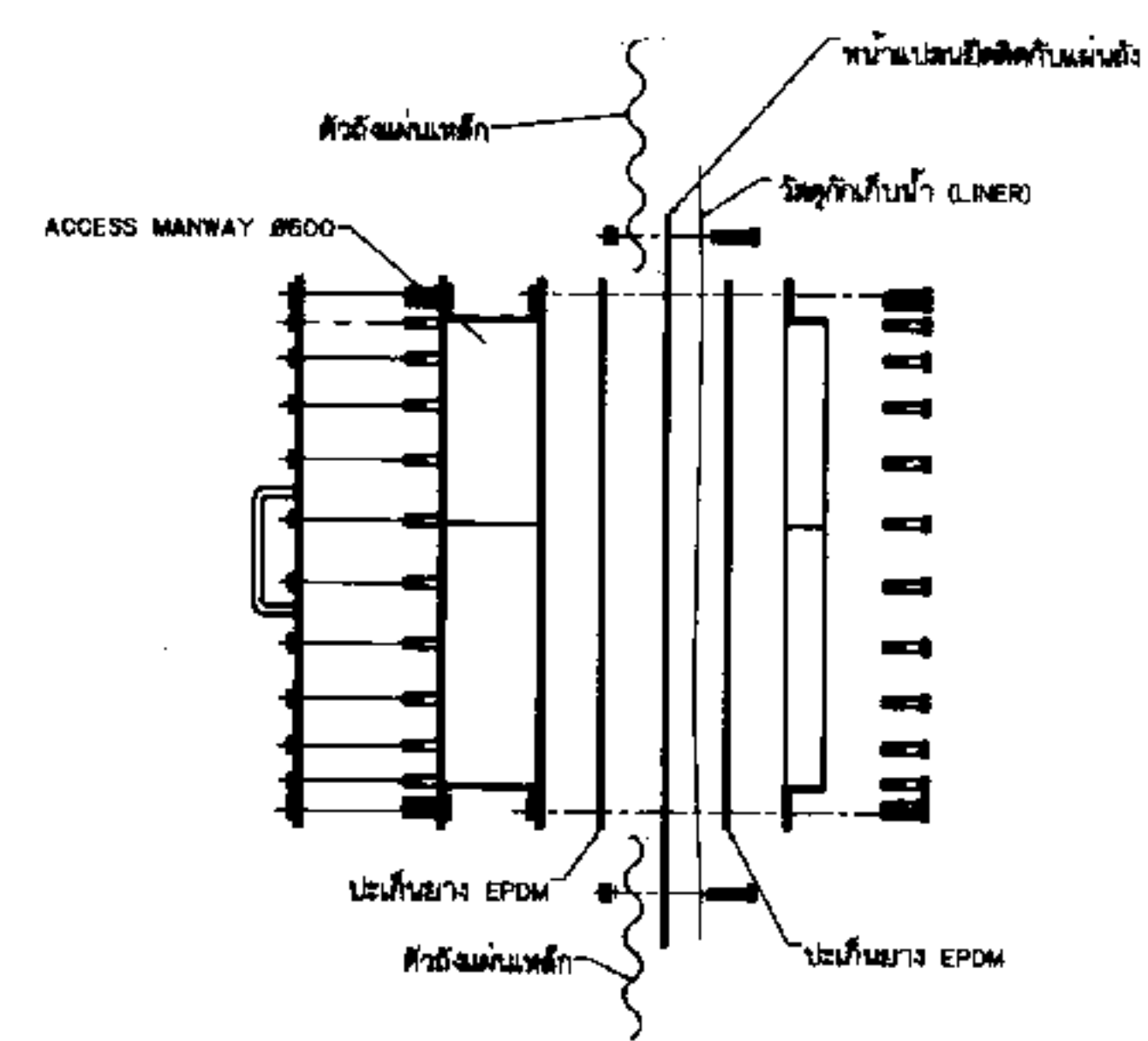
แบบขยาย ประตูตรวจสอบน้ำจืด Scale NTC
