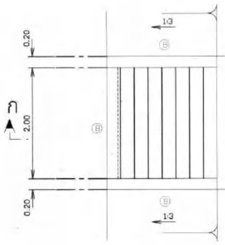
แปลนอาคารบันได คสล.
