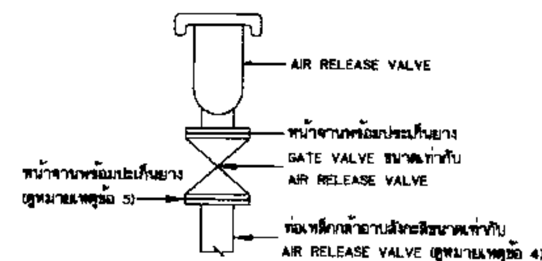
การติดตั้ง AIR RELEASE VALVE ในตะกอนทราย
