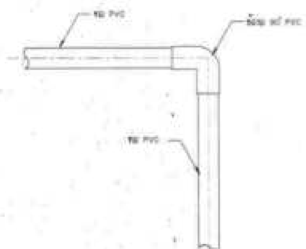
7. แบบการต่อข้องอ 90° PVC ในเขตเทศบาล
