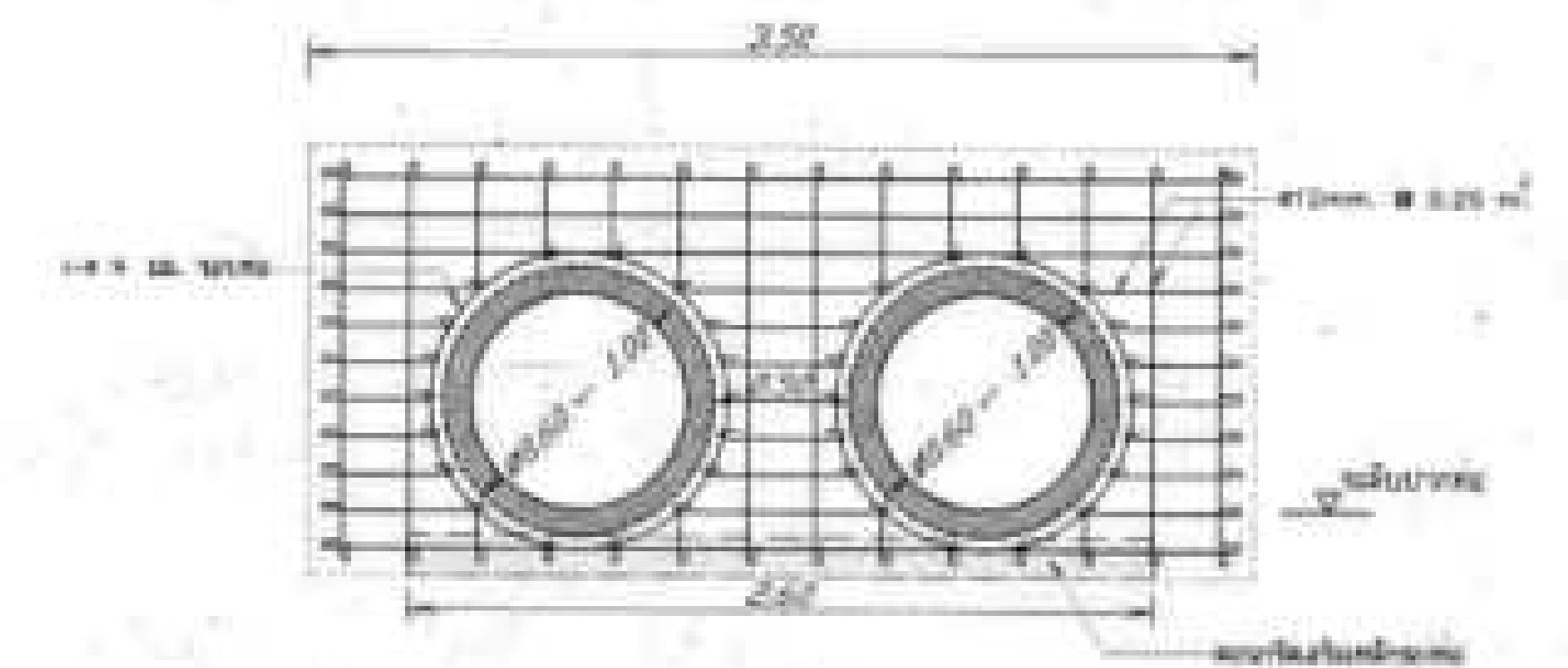
แบบขยายเหล็กเสริมคานกรัดปากท่อ
