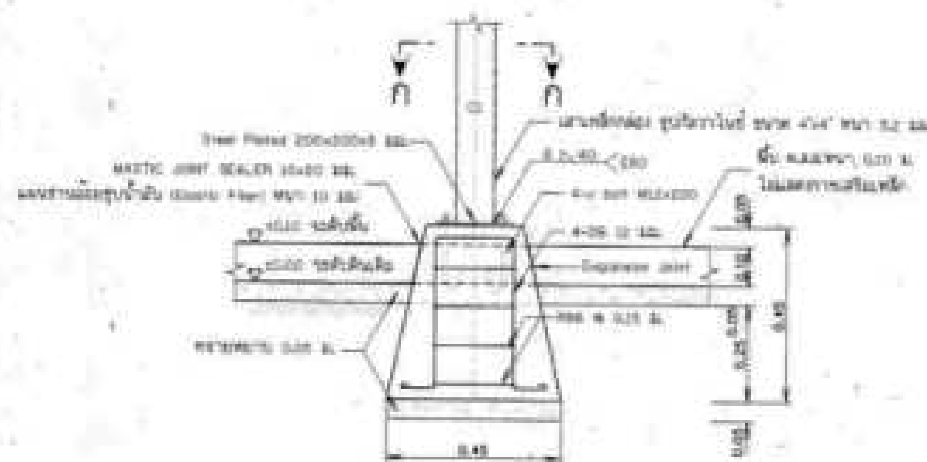
รูปขยายฐานรากโครงสร้างรับแรง F1 ขนาด 300. พลาซ่า/รูปหน้าตัดจริง โมเดลอาคารจริง
