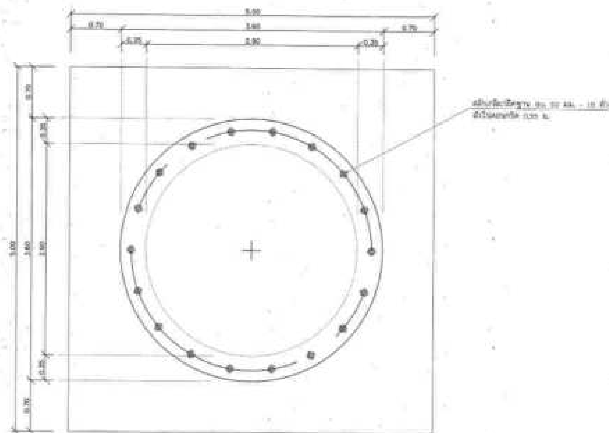
แบบขยายฐานรากหม้อถึงสูง (แบบฐานแห้)
