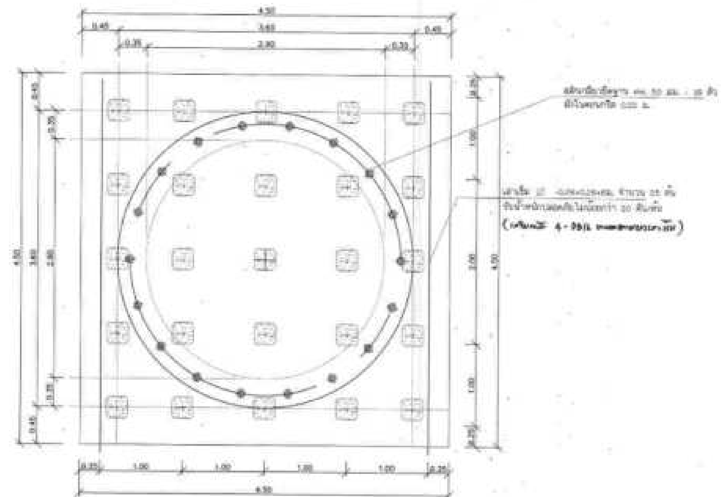
แบบขยายฐานรากหม้อถึงสูง (แบบเสาเข็ม)
