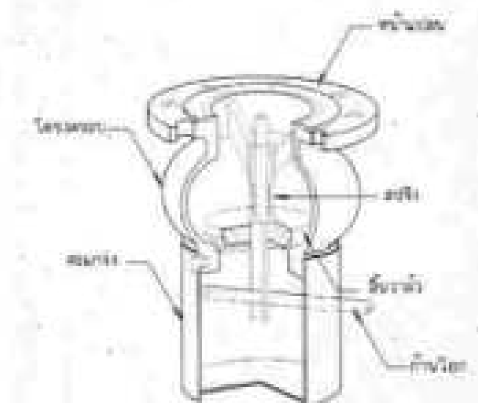
15. ฟุตวาล์ว แบบก้านโยก ในเขตเทศบาล
