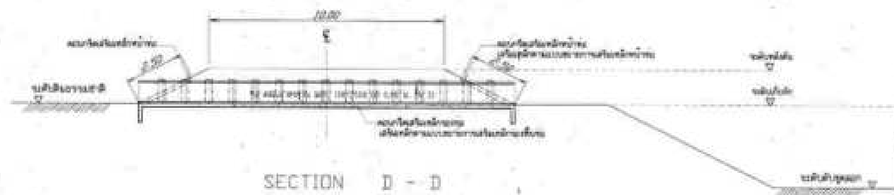
รูปตัดค้ำดิน แสดงการวางท่อนแบบ 2 แถว ขนาด 1:50
