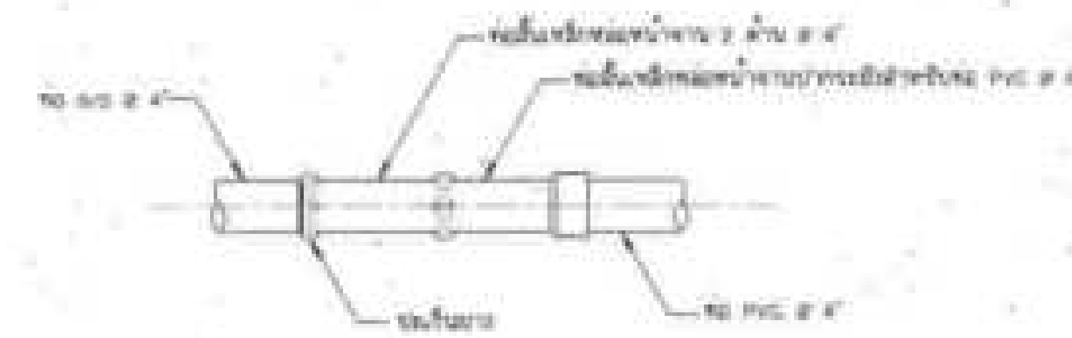
8. การบรรจุท่อเหล็กอาบสังกะสี G/S กับท่อ PVC. ในเขตเทศบาล
