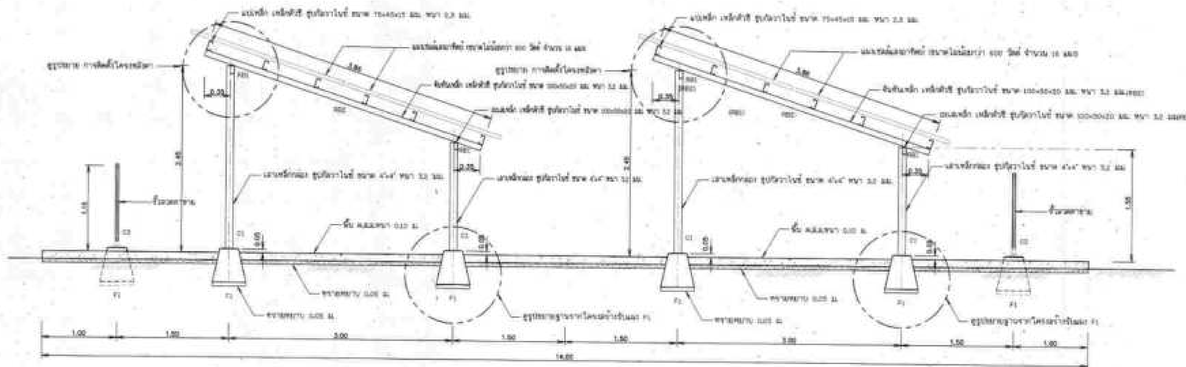
รูปด้านข้าง โมเดลอาคารจริง
