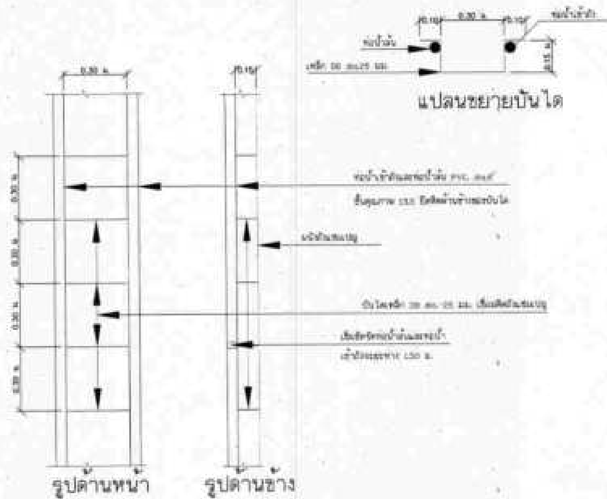
แบบขยายบันได และการยึดท่อน้ำขึ้นและท่อน้ำเข้าถึง ขนาดหน้ากระดาษ 1 : 20
