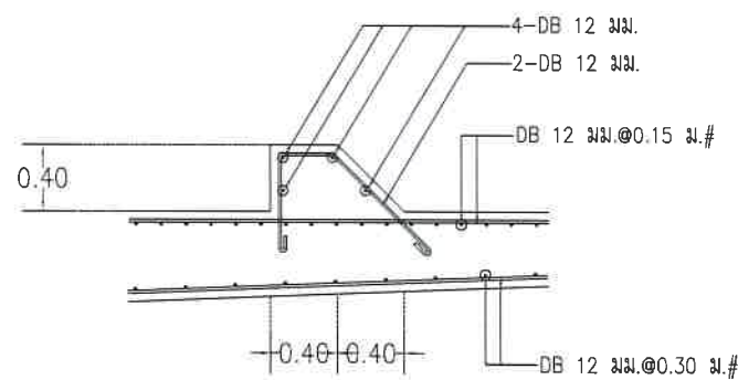
แบบขยาย 9 มาตราส่วน 1:50
