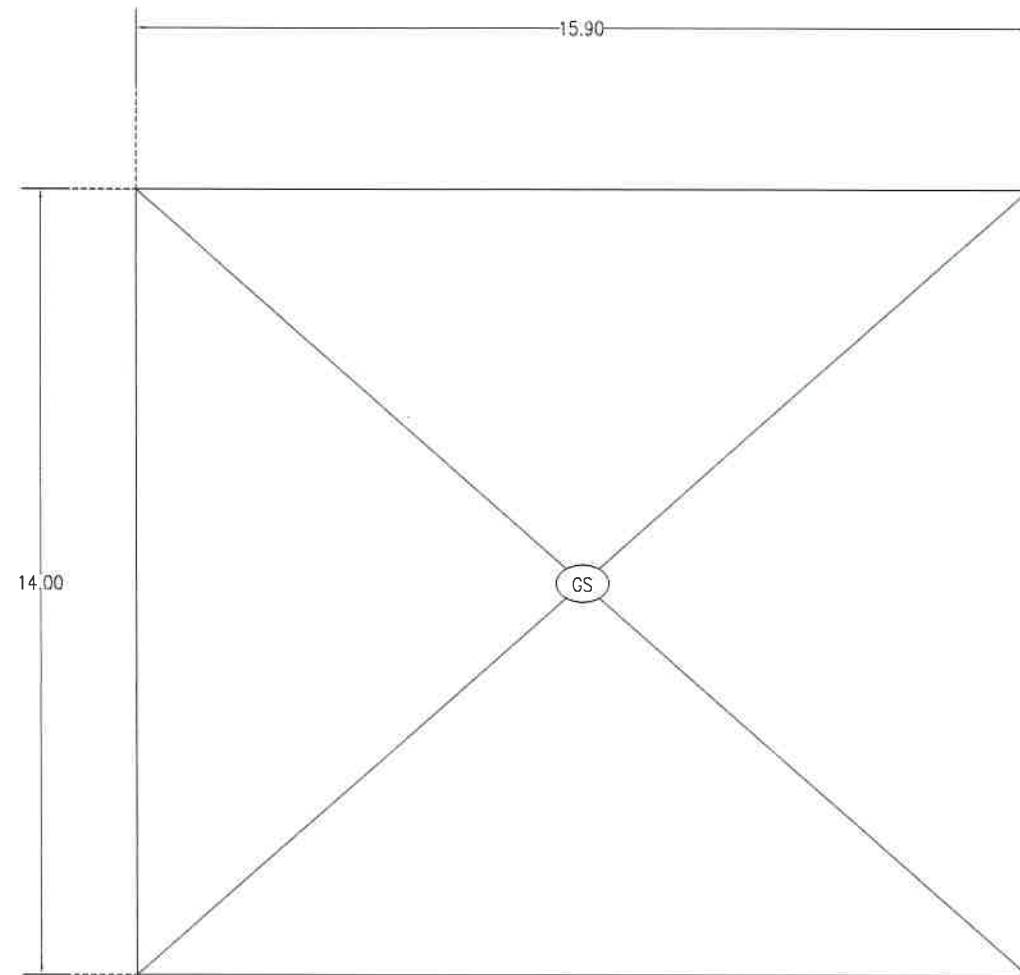
แปลนฐานรากแบบแผ่ SCALE 1:135
