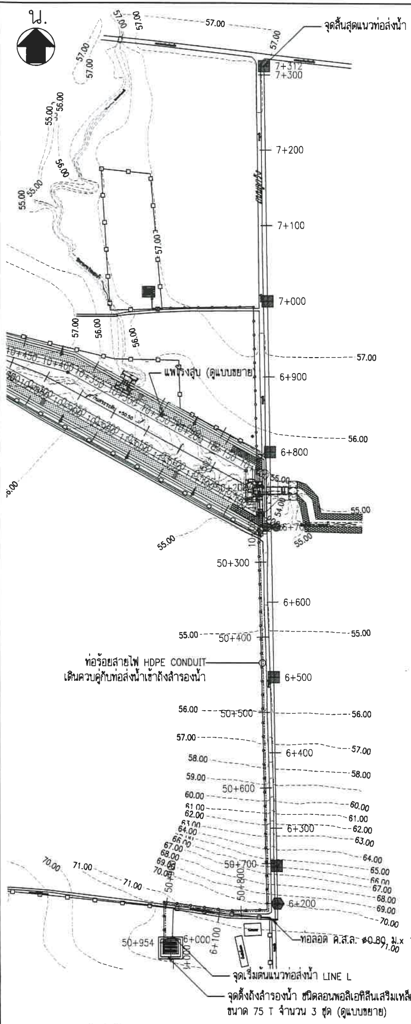
แปลนแนวท่อส่งน้ำ LINE L (STA. 6+000 ถึง 7+312) มาตราส่วน 1:4,000
