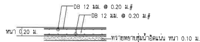
ขยายพื้นฐานราก GS Scale 1:50
