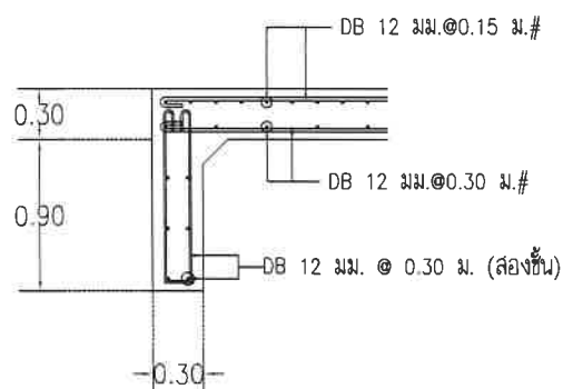
แบบขยาย CUTOFF มาตราส่วน 1:50
