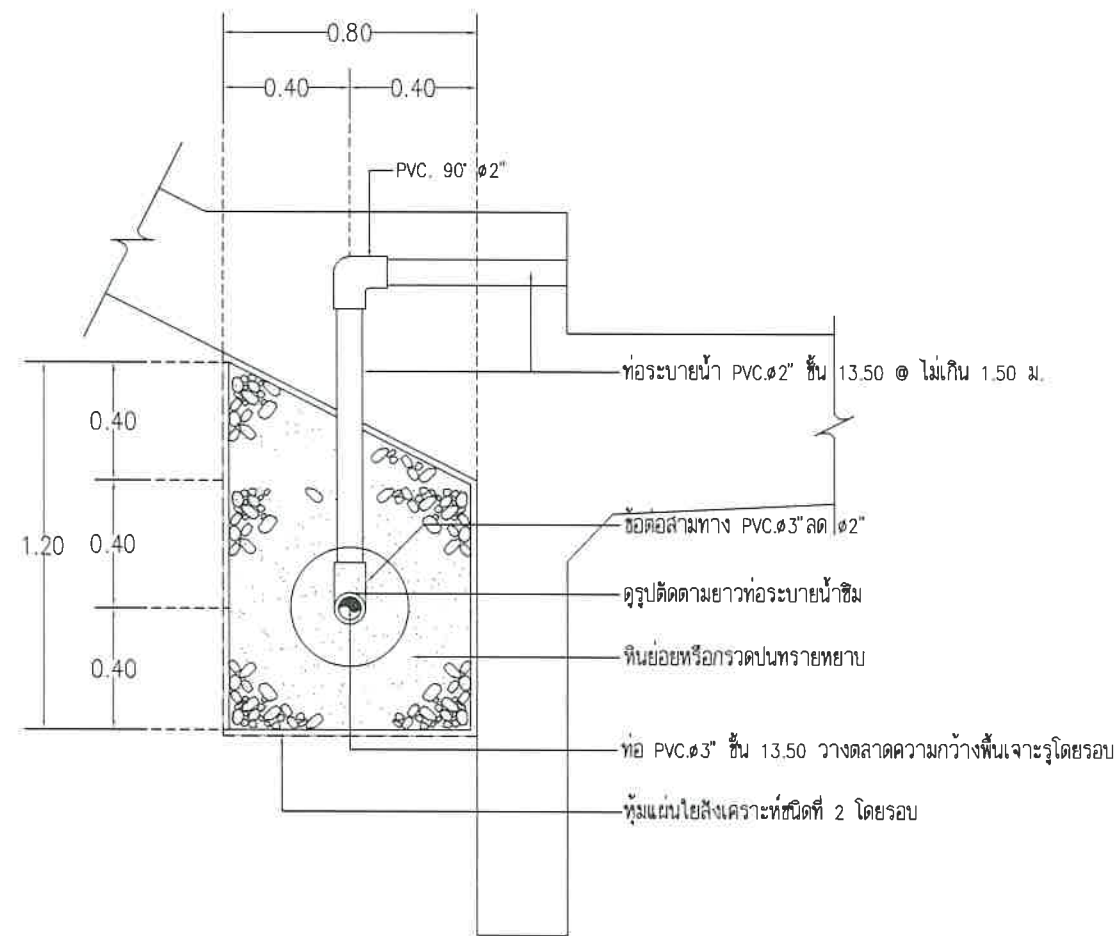
ขยายท่อลดแรงดันน้ำที่พื้นแบบที่ 2 [ท้องพื้นเอียง] SCALE 1:25
