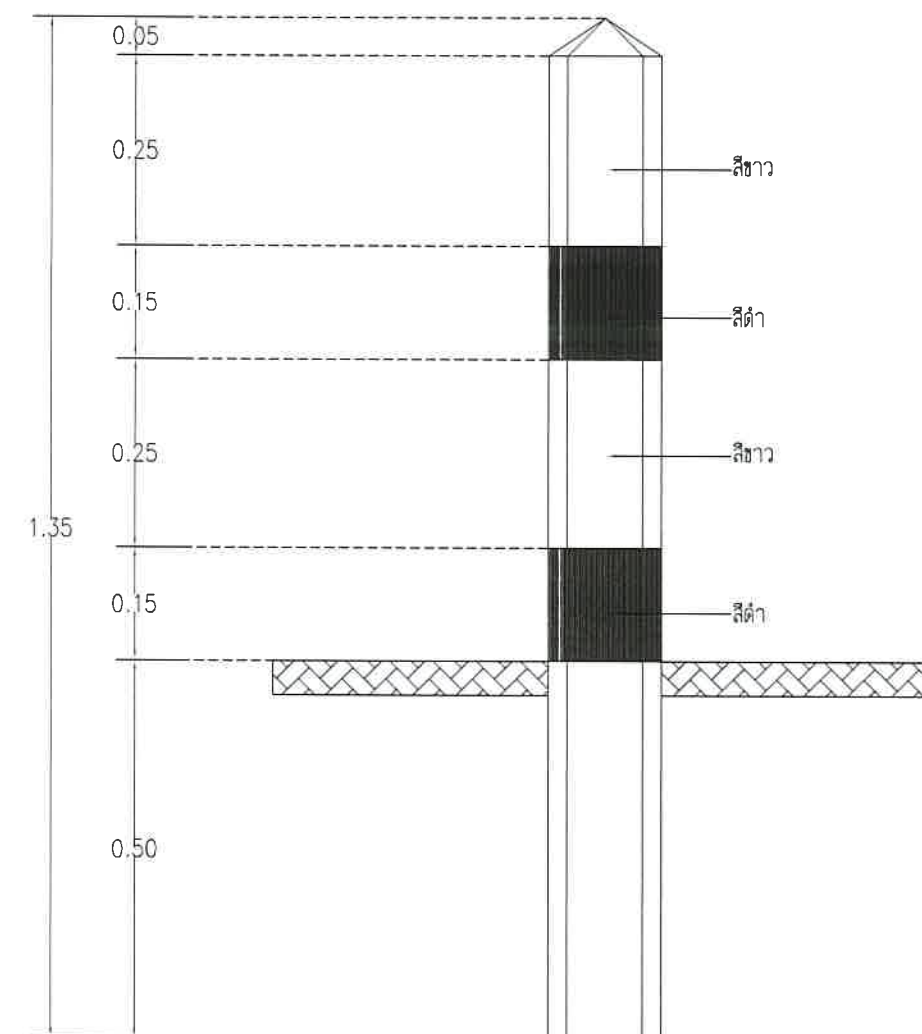
แบบขยายหลักบ่อแนว มาตราส่วน 1:10
