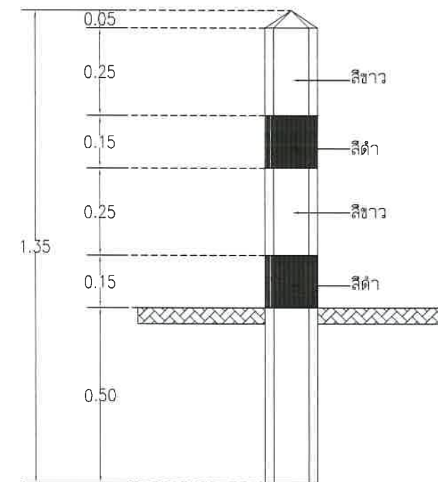
แบบขยายหลักบ่อแก้ว มาตราส่วน 1:15
