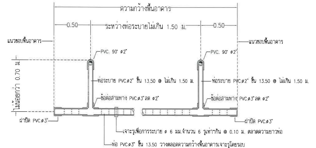
ขยายท่อลดแรงดันน้ำที่พื้นแบบที่ 2 [ท้องพื้นเอียง] SCALE 1:25
