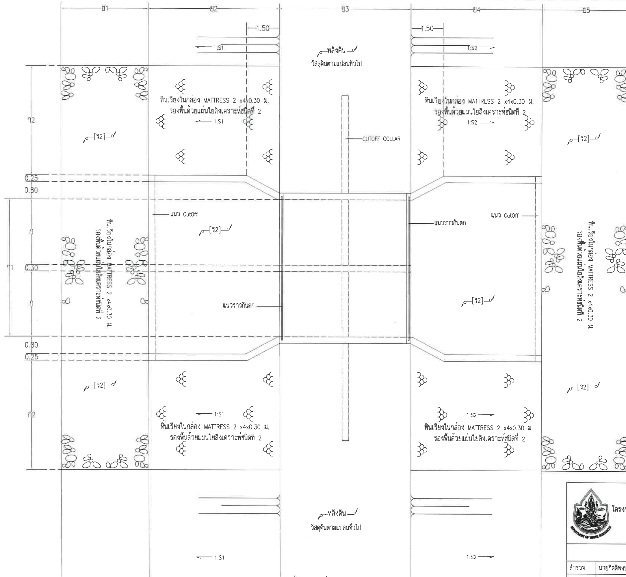
แปลนอาคารท่อเหลี่ยม(ดูขนาดมิติตามตาราง) มาตราส่วน 1:100
