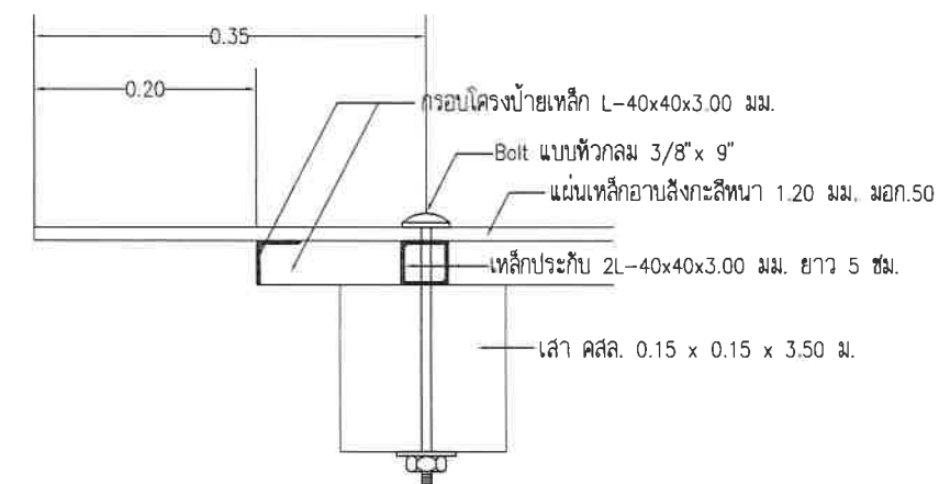
ขยายการยึดแผ่นป้ายและเสา
