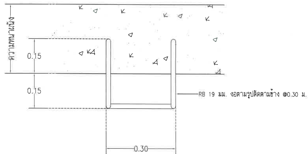
แปลนบันไดลิง
