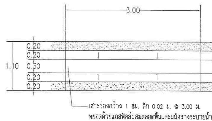
แปลนรางระบายน้ำ มาตราส่วน 1:50
