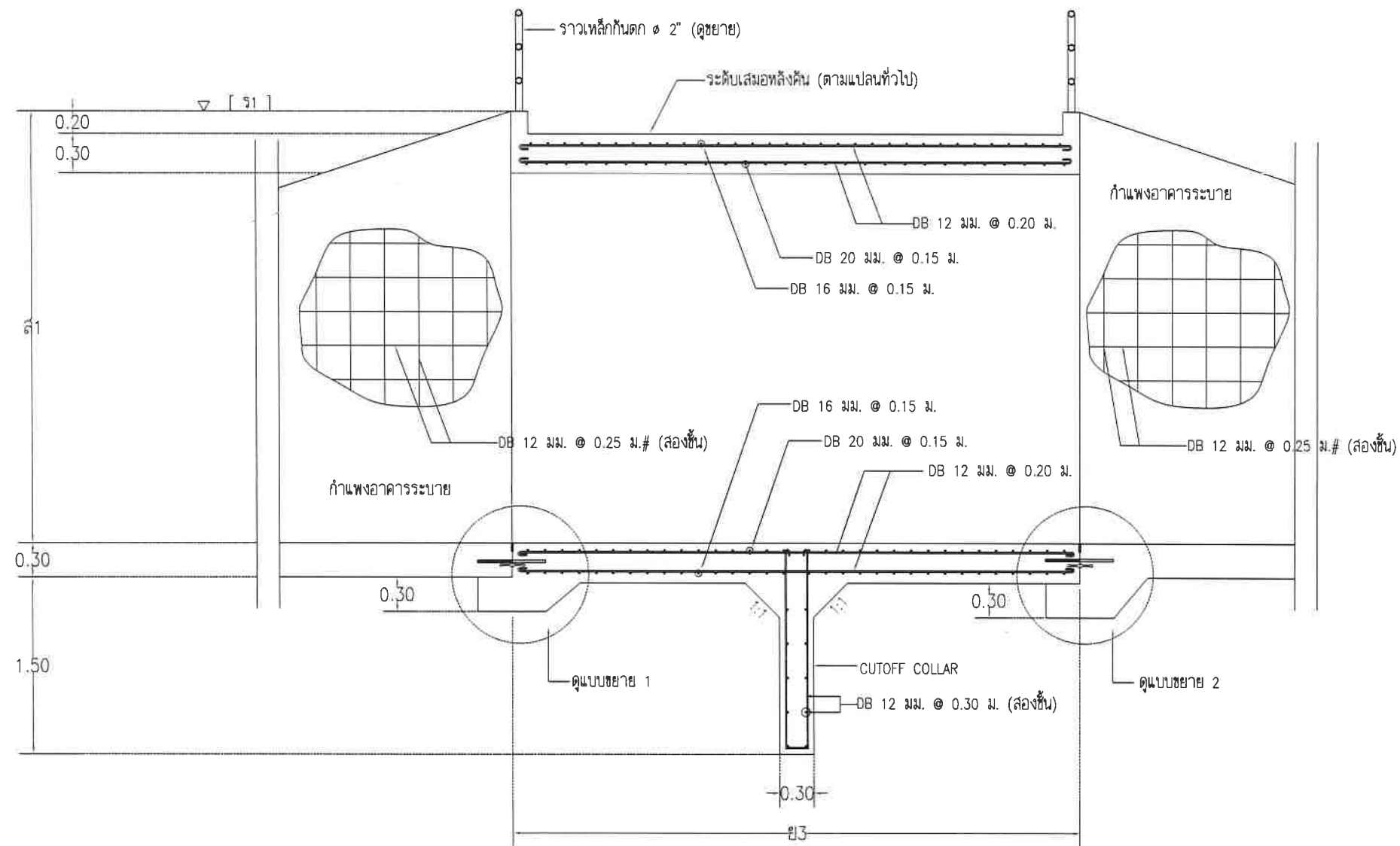
รูปตัดตามยาวท่อเหลี่ยม คลส. มาตราส่วน 1:50
