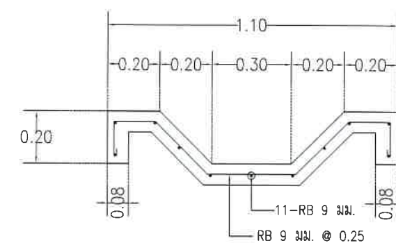
รูปตัดรางระบายน้ำ มาตราส่วน 1:20
