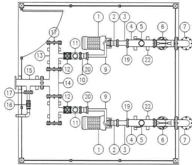
แปลนแสดงการประสานอุปกรณ์ภายในโรงสูบน้ำ SCALE 1:50
