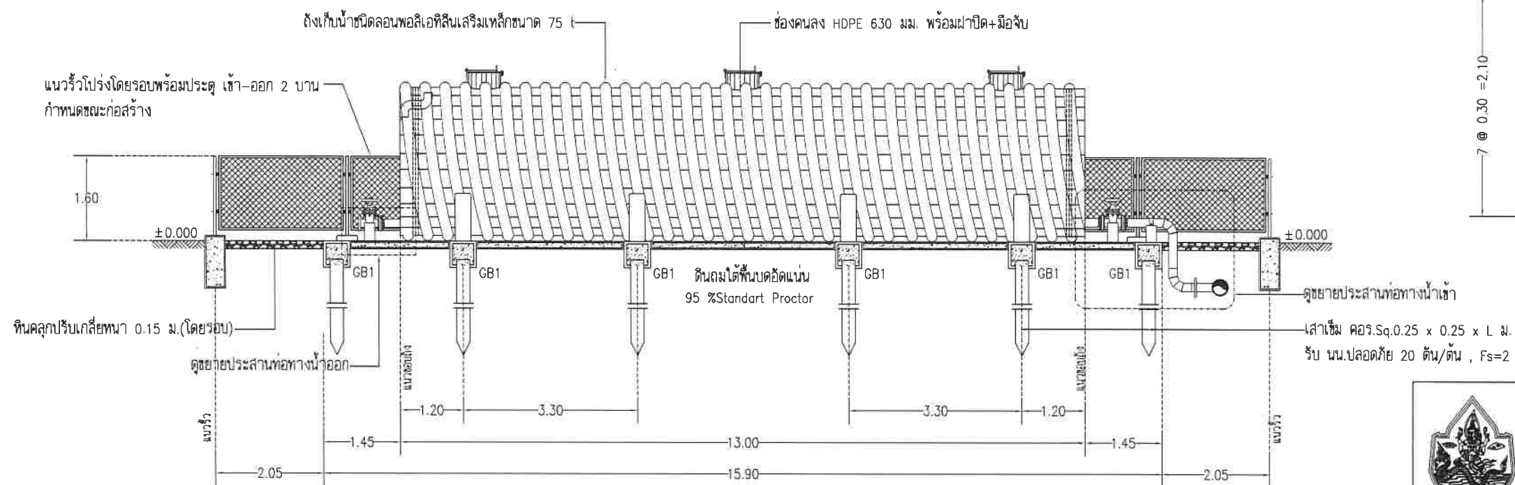
รูปตัดตามยาวถังเก็บน้ำสำรอง A - A (กรณีฐานรากเสาเข็ม) SCALE 1:100
