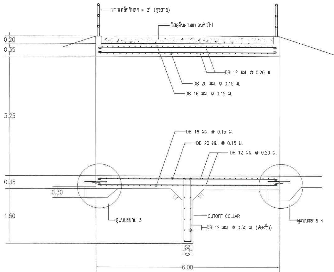
รูปตัดตามยาวท่อเหลี่ยม คสล. มาตราส่วน 1:50
