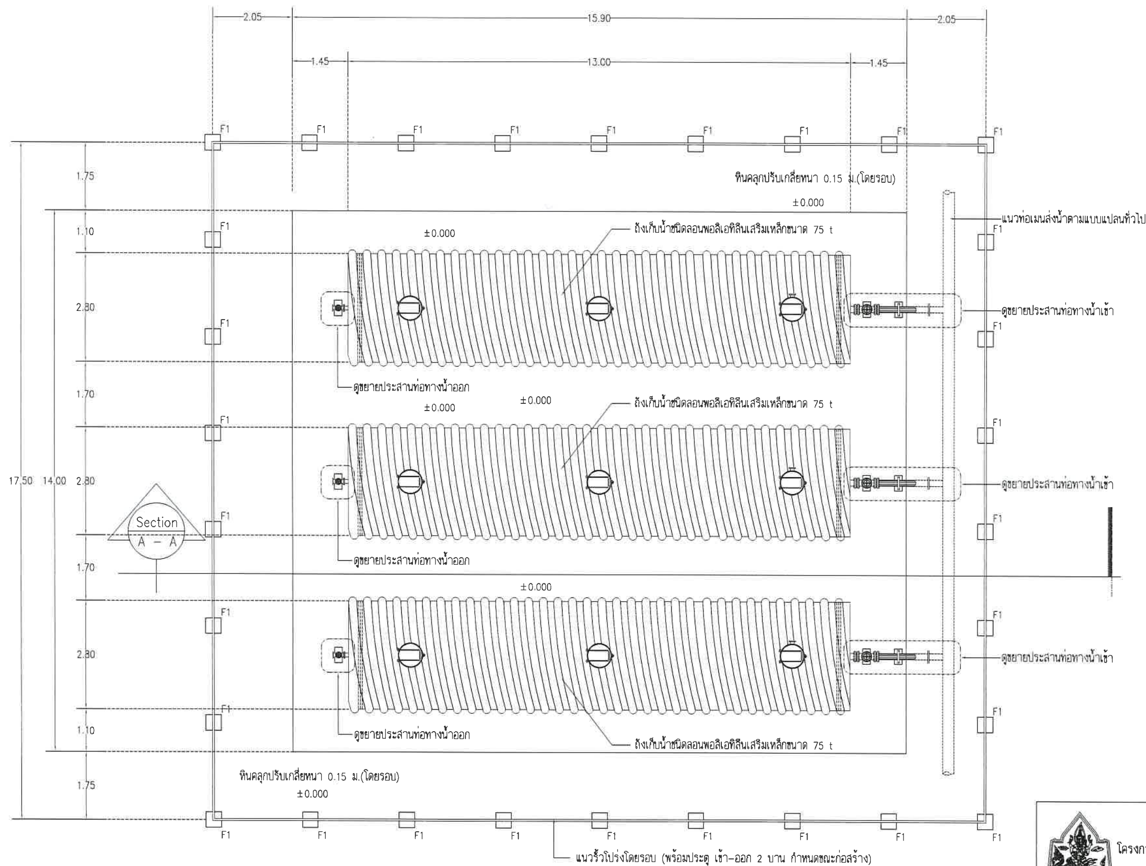
แปลนถังเก็บน้ำสำรอง ชนิดลอนพอลิเอทิลีนเสริมเหล็ก ขนาด 75 T จำนวน 3 ชุด
