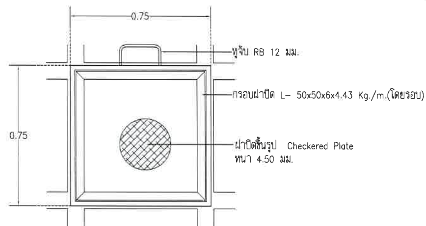
แปลน MAIN HOLE SCALE 1:20
