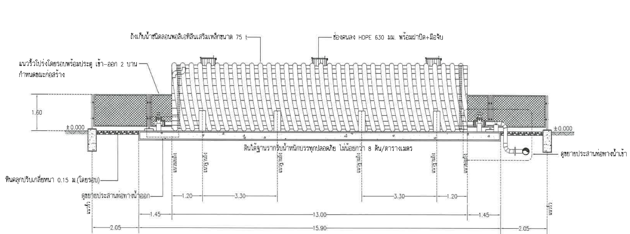
รูปตัดตามยาวถังเก็บน้ำสำรอง A - A (กรณีฐานรากแผ่) SCALE 1:100
