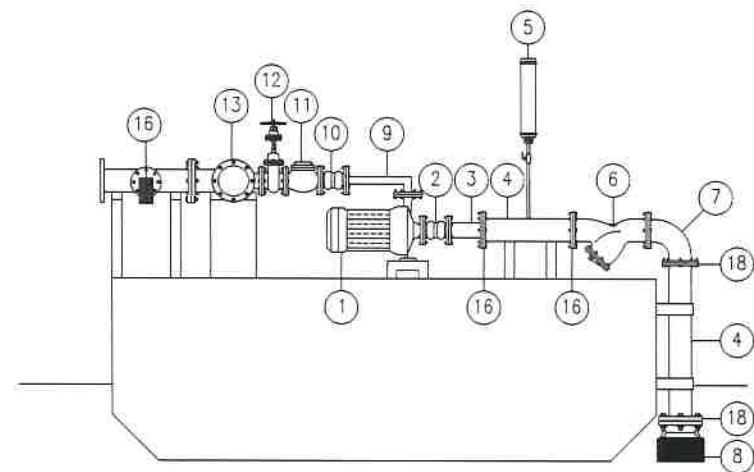
รูปตัดแสดงการประสานอุปกรณ์ภายในโรงสูบน้ำ SCALE 1:50
