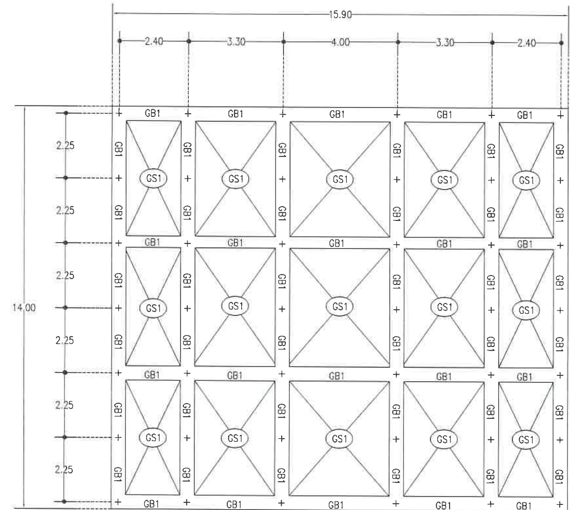
แปลนฐานรากแบบเสาเข็ม SCALE 1:135
