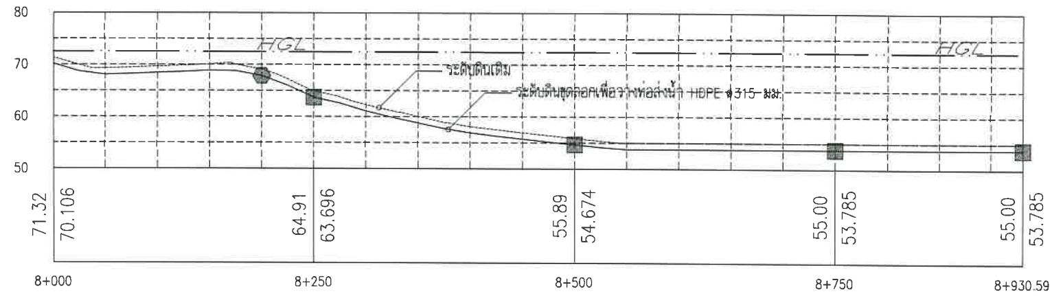
PROFILE แนวท่อน้ำ LINE R
