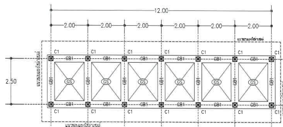
แปลนคานคอดิน เสา พื้น รับแผงโซล่าเซลล์
