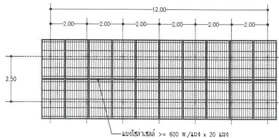
แปลนแสดงอาคารแผงโซล่าเซลล์
