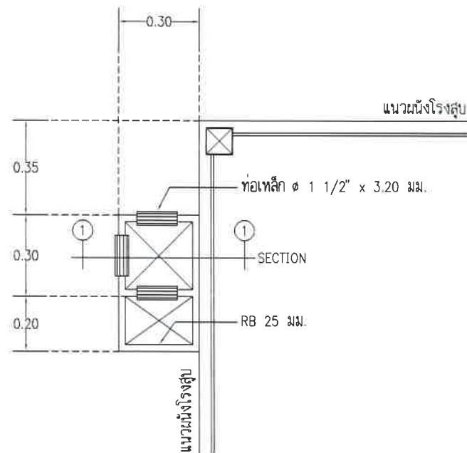
แปลนชุดโยงยึด SCALE 1:20
