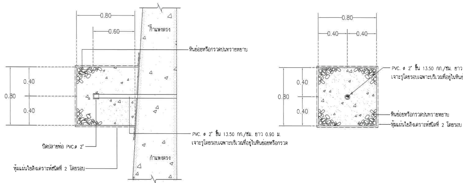
ขยายท่อลดแรงดันด้านข้างกำแพงแบบที่ 1 [กำแพงตรง] SCALE 1:25
