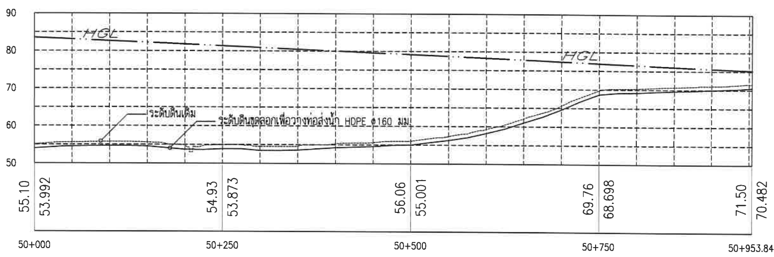
PROFILE แนวท่อส่งน้ำไปยังถังสำรองน้ำ มาตราส่วน แนวดิ่ง 1:1,000 แนวนอน 1:5,000
