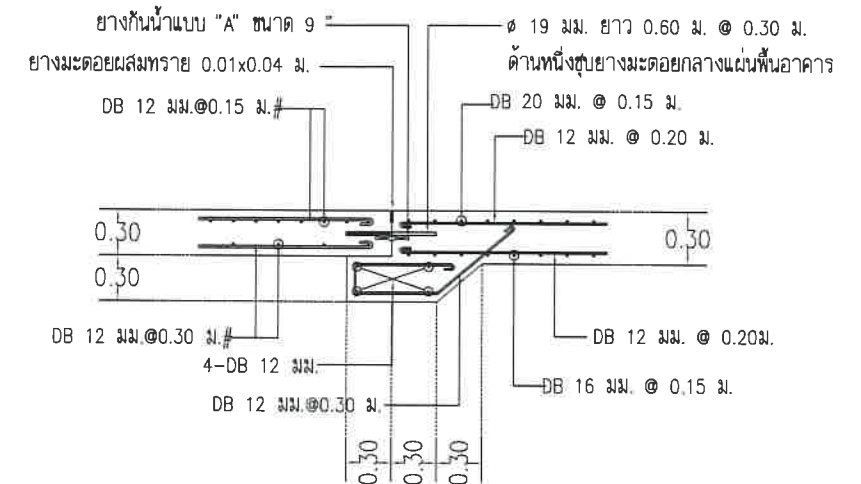
แบบขยาย 1 มาตราส่วน 1:50
