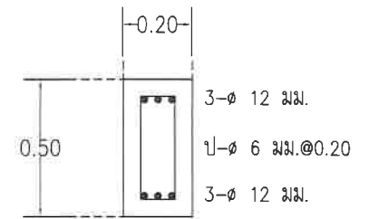
ขยายคานขอบโดยรอบบันได มาตราส่วน 1:25
