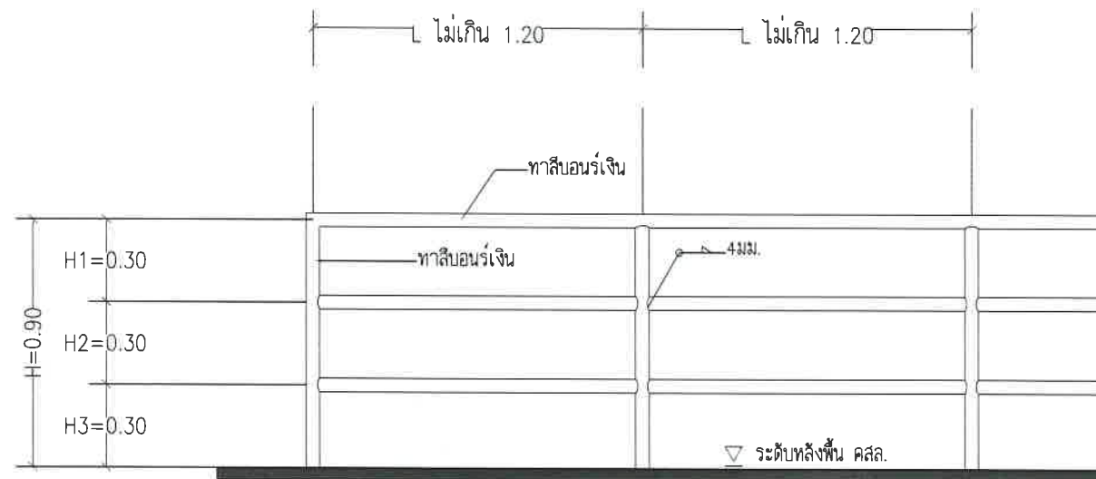
แสดงรูปด้านราวกันตก มาตราส่วน 1:25
