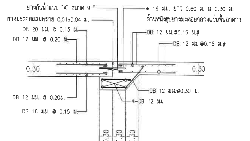
แบบขยาย 2 มาตราส่วน 1:50
