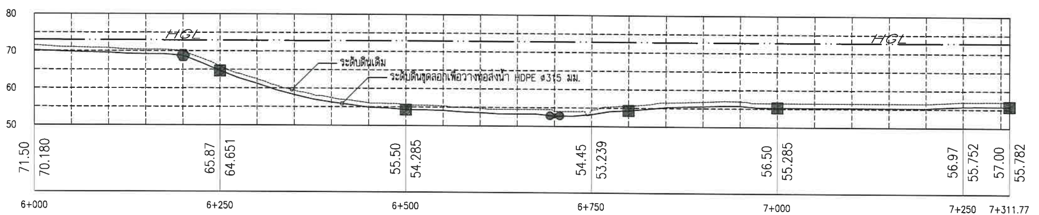
PROFILE แนวท่อส่งน้ำ LINE L มาตราส่วน แนวดิ่ง 1:1,000 แนวนอน 1:5,000
