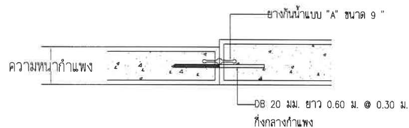
แบบขยายรอยต่อกำแพง มาตราส่วน 1:25
