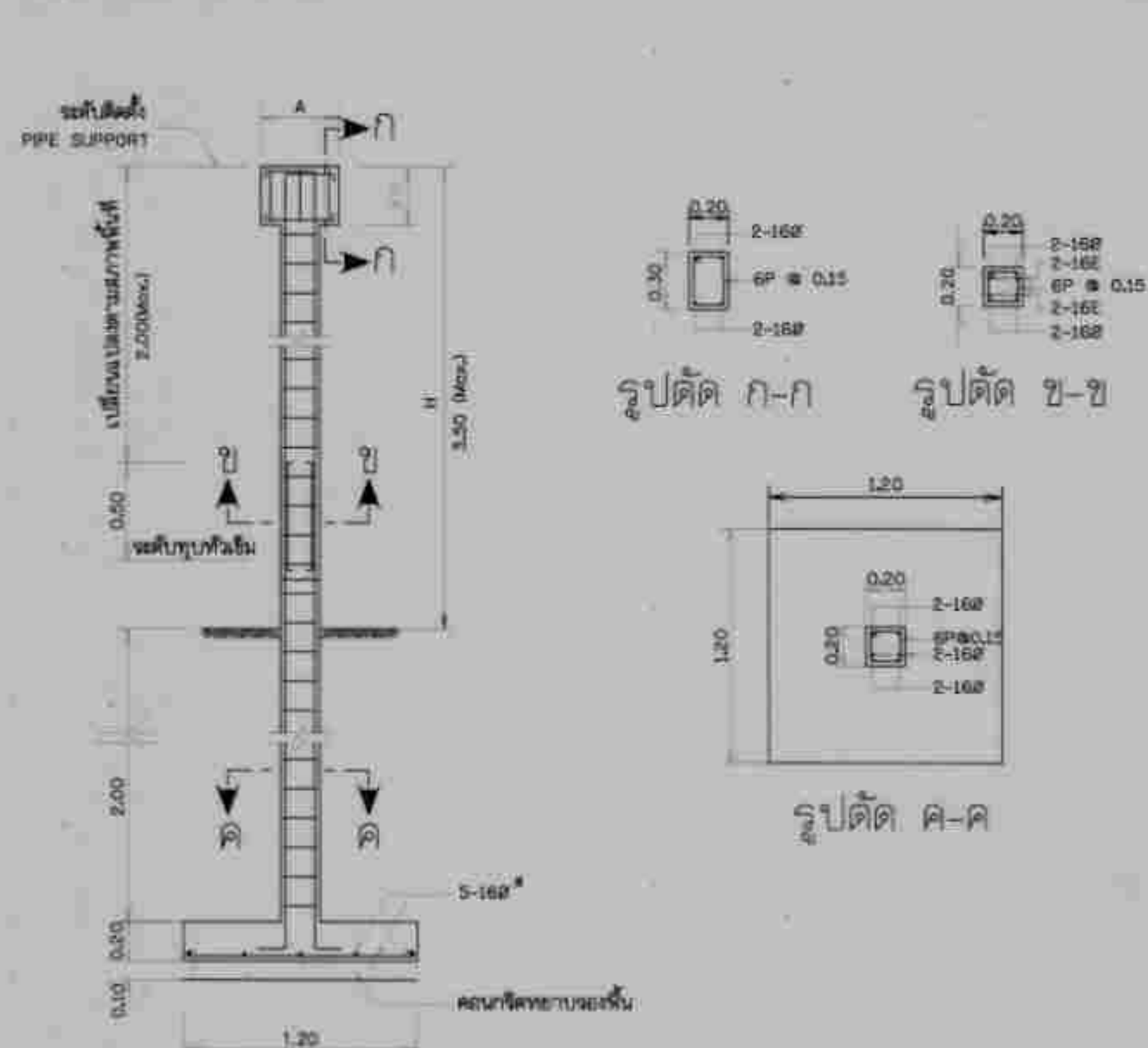
การเสริมเหล็ก ดอมอแบบที่ 1
