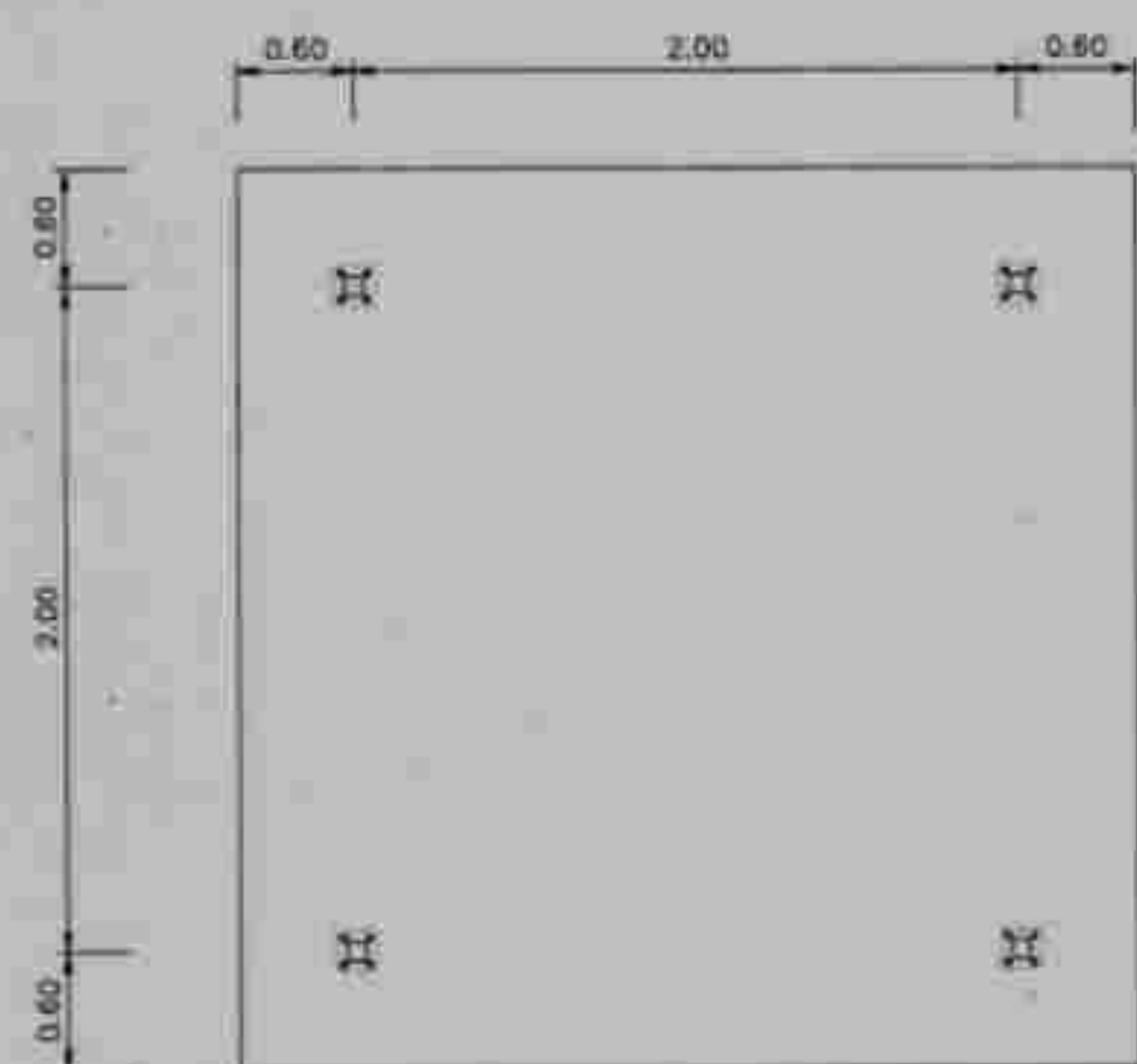
แปลนเครื่องกรองเกษตร โมดูลขนาดฐาน
