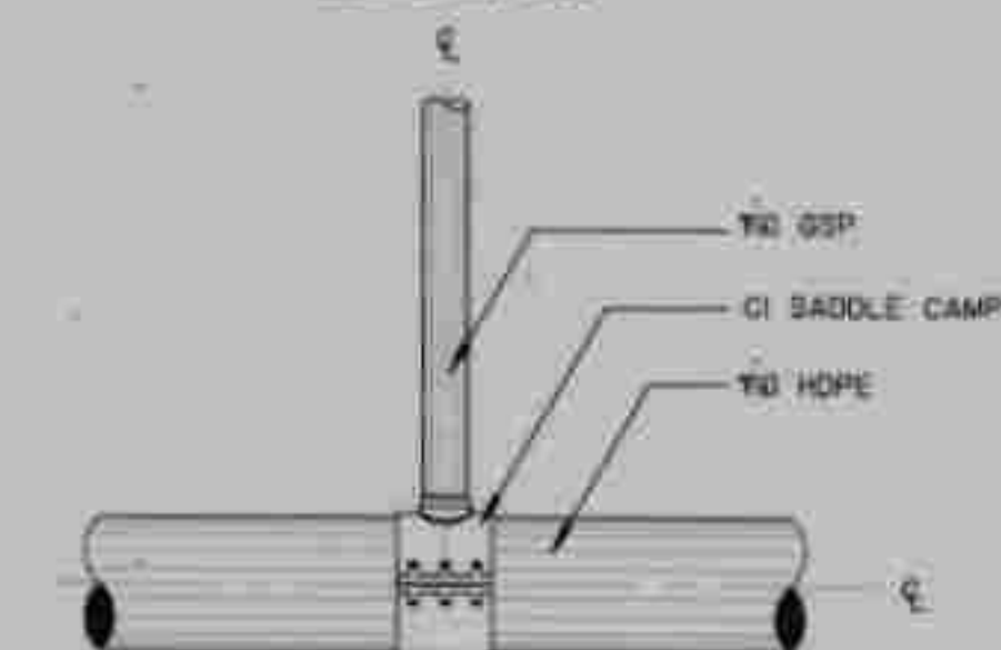
การบรรจุบล็อกลูกท่อสามทาง HDPE กับท่อ GSP
