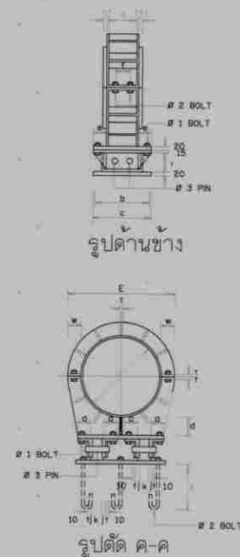
PIPE SUPPORT สำหรับท่อเหล็กขนาด Ø400 มม. - Ø800 มม.
