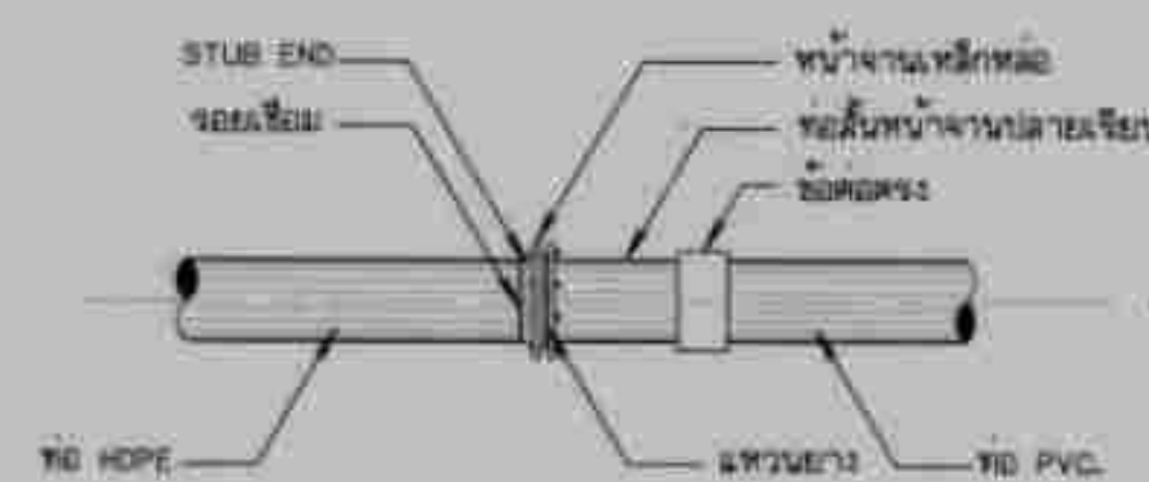
การบรรจุบล็อกลูกท่อ HDPE กับท่อ PVC.
