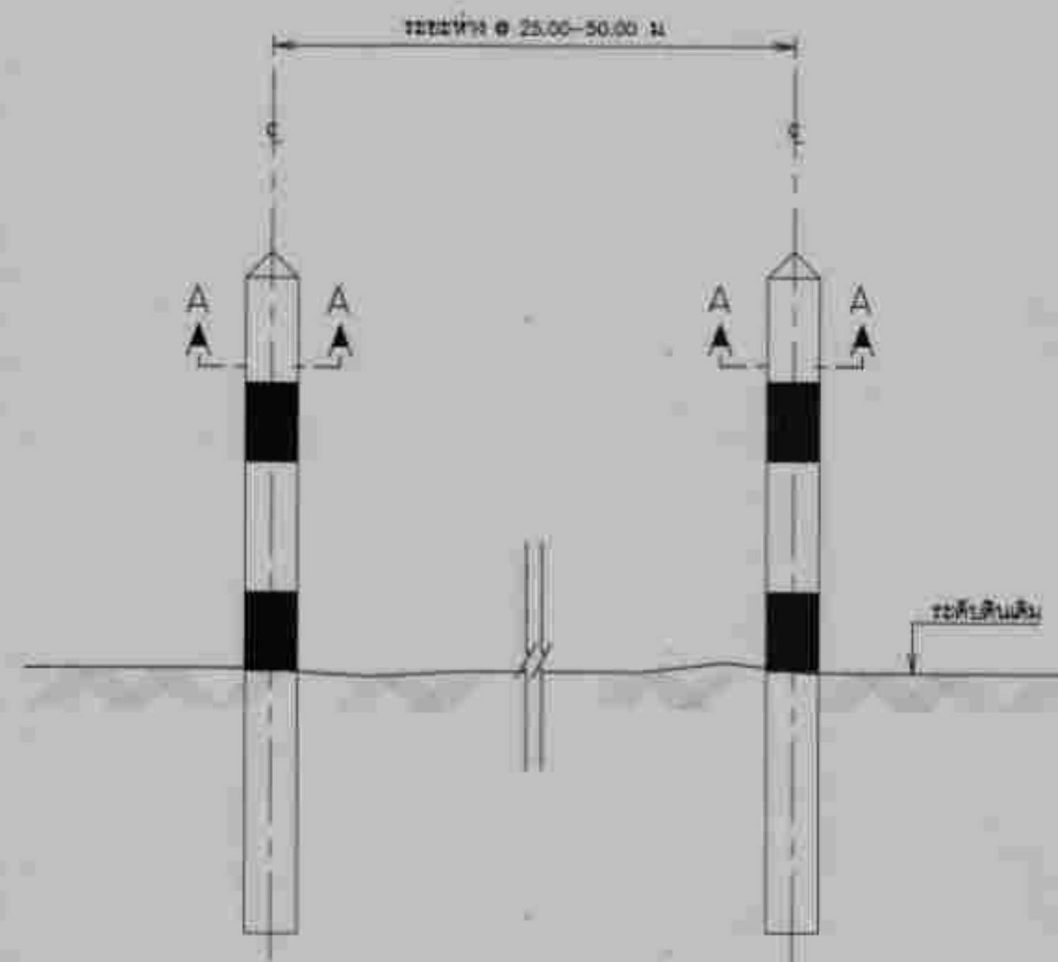
แสดงการวางหลักบ่อแกวท่อ มาตราส่วน 1:20
