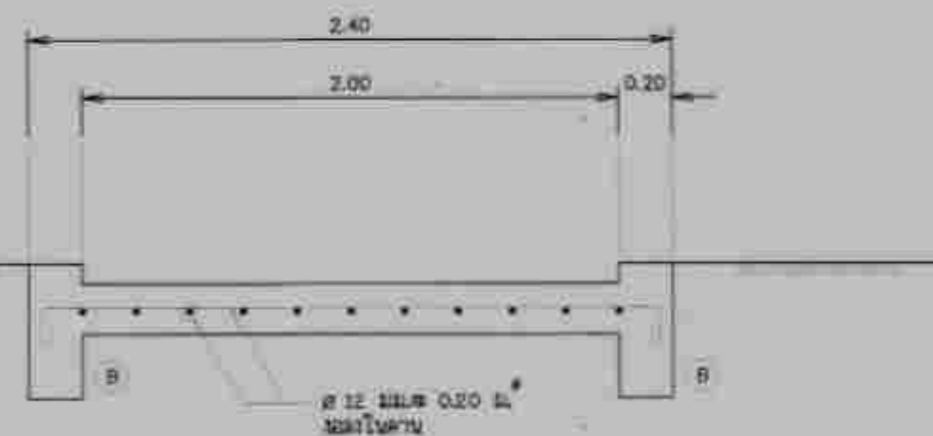
รูปตัดแนว ข - ข
