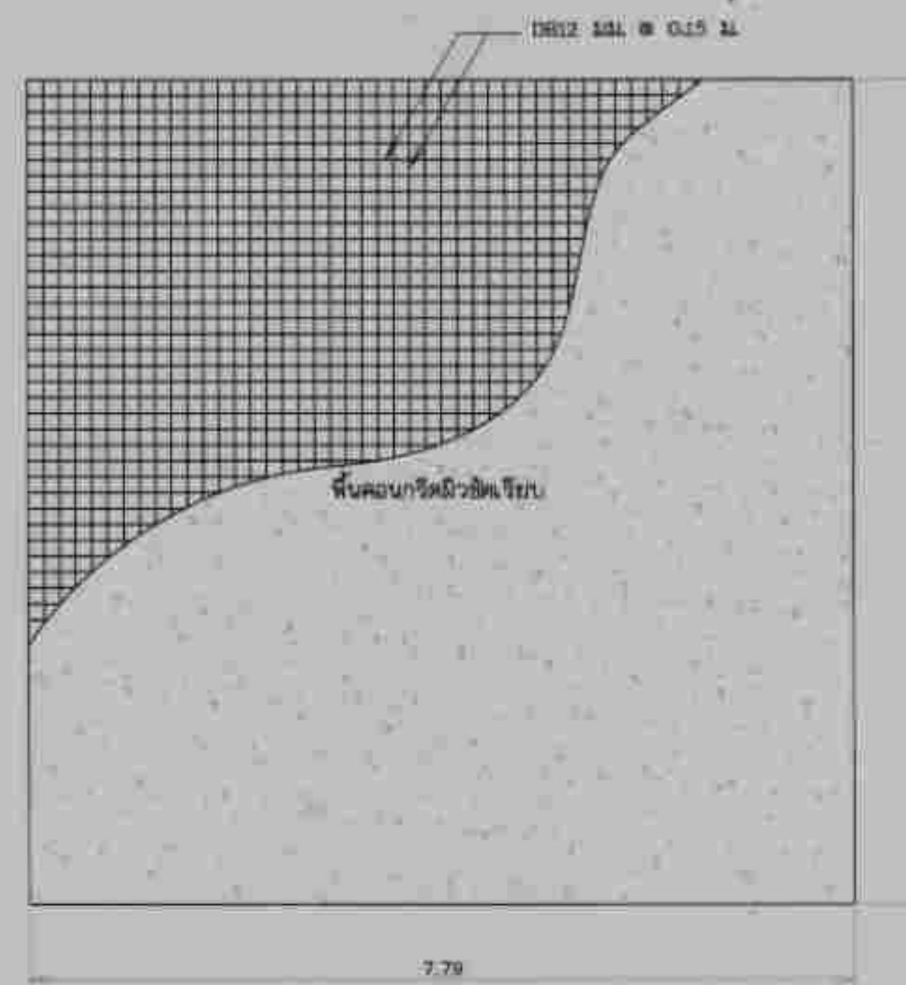
แบบพื้น
