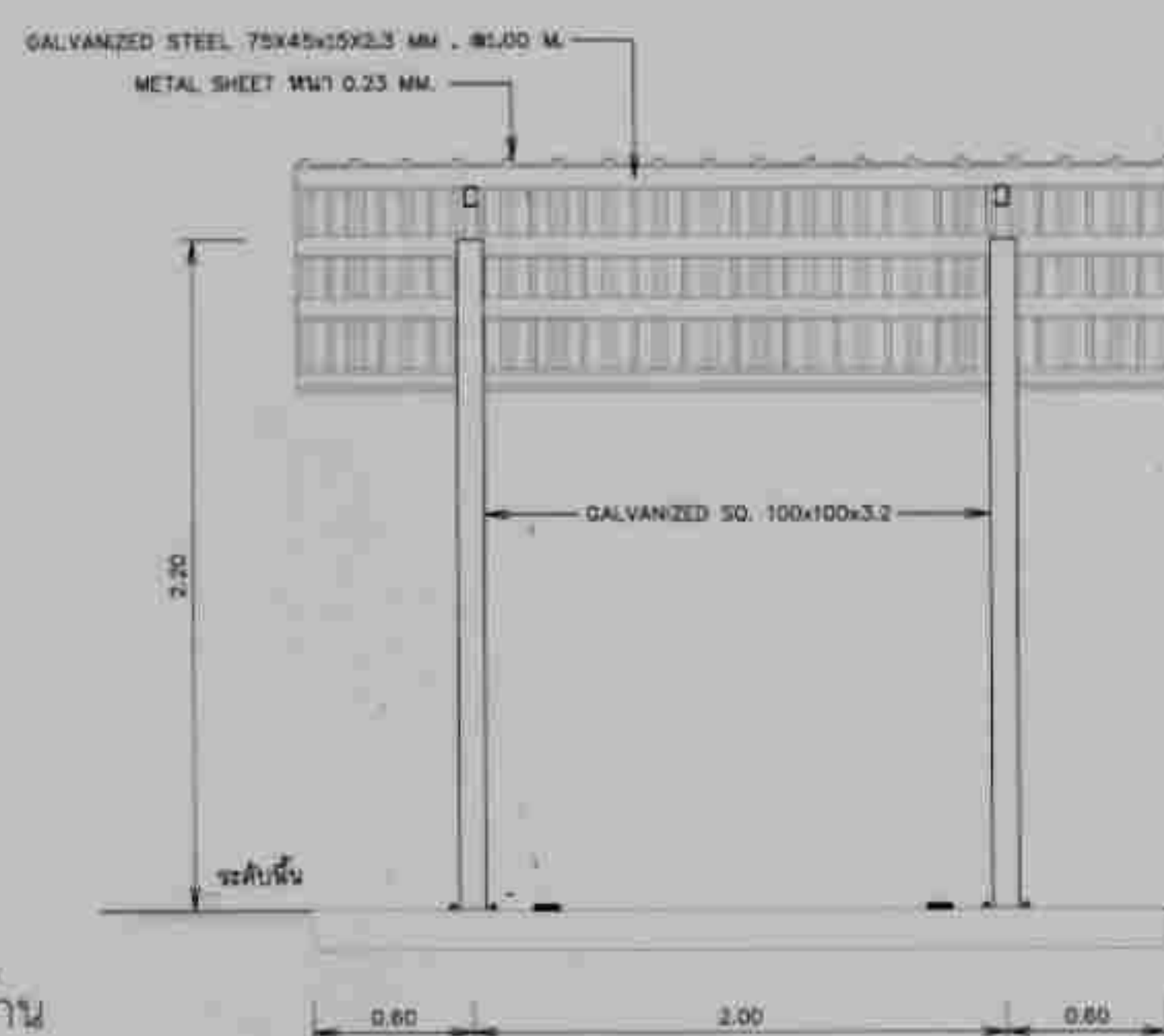
รูปด้าน 1 โมดูลขนาดฐาน
