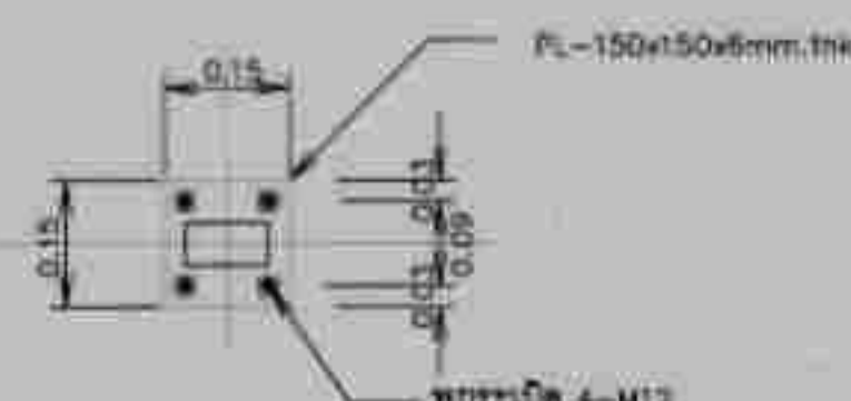
แบบขยายเล้า 2 ขนาดฐาน 1:10
