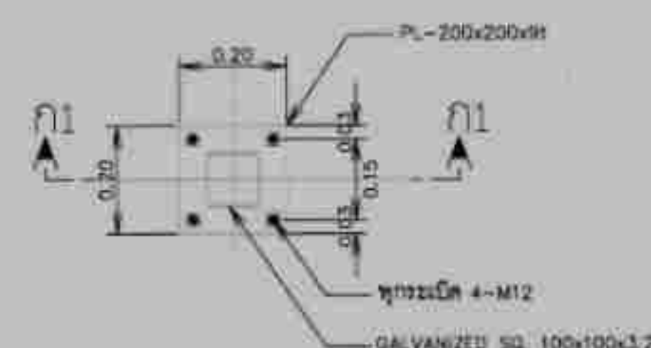
แบบขยายเล้า 1 ขนาดฐาน 1:10
