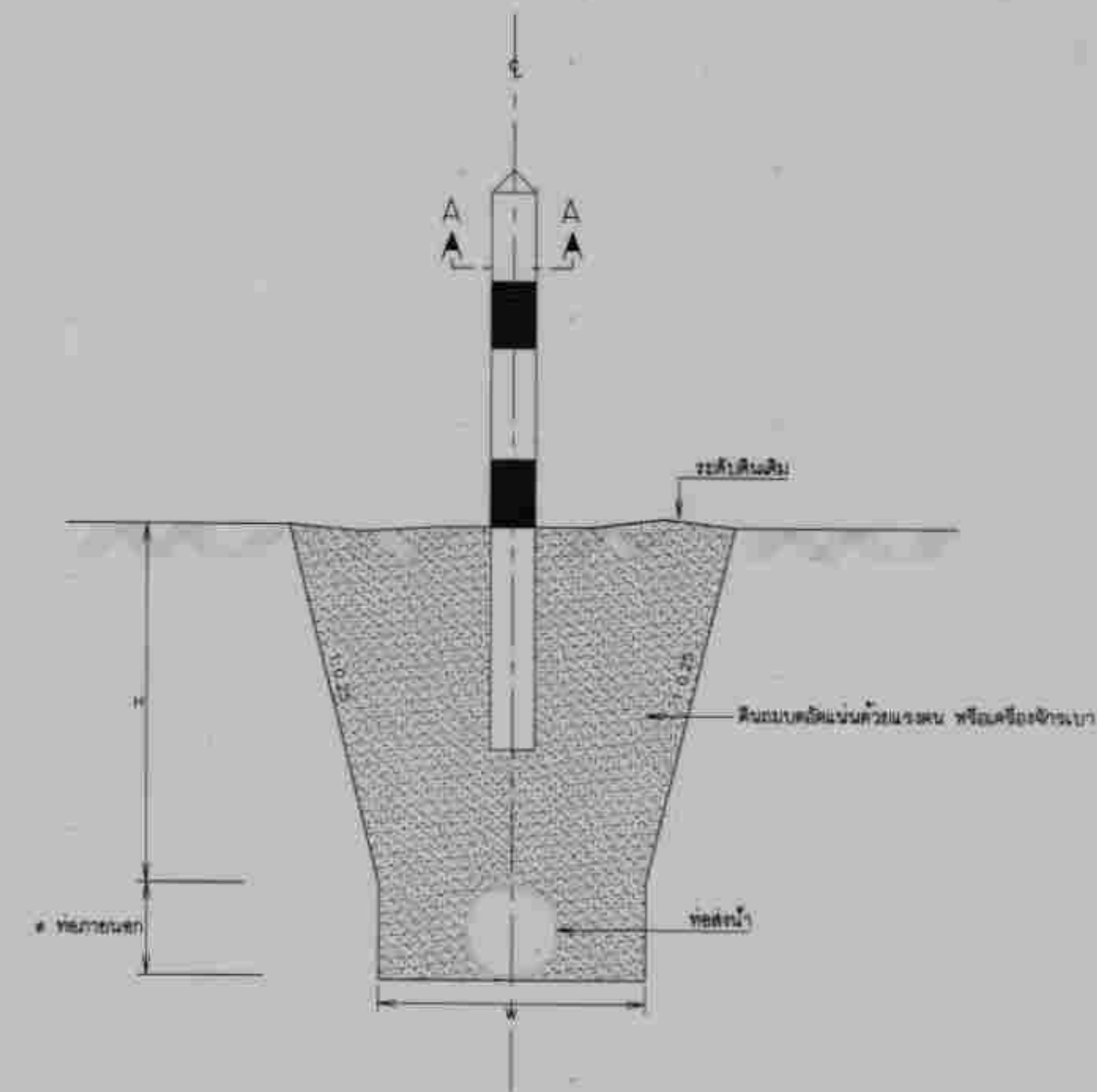
แสดงรูปตัดขวางทั่วไปของแกวท่อ มาตราส่วน 1:20
