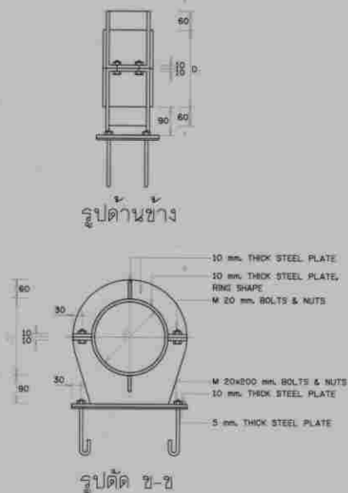
PIPE SUPPORT สำหรับท่อเหล็กขนาด Ø 300 มม.
