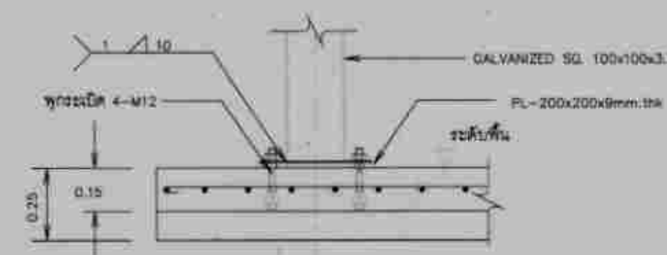
รูปตัด ก1 - ก1 ขนาดฐาน 1:5
