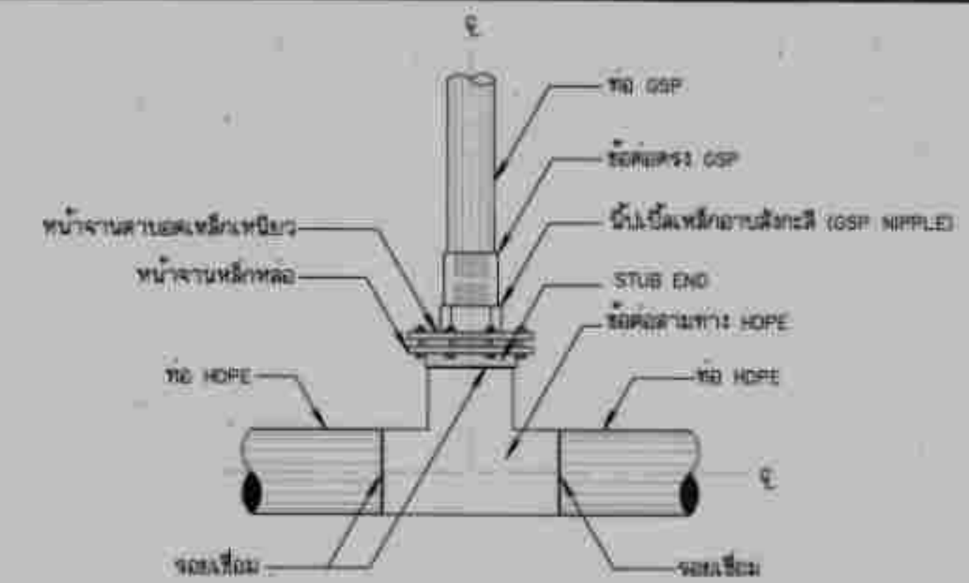
การบรรจุบล็อกลูกท่อสามทาง HDPE กับท่อ GSP แบบข้อต่อ
