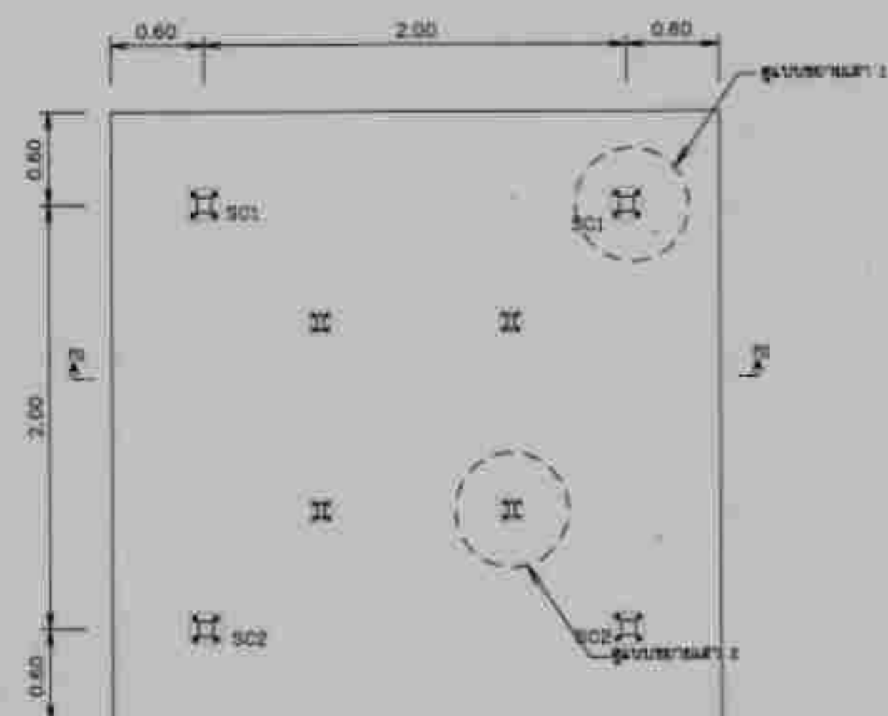
แปลนฐานรับเครื่องกรองเกษตร โมดูลขนาดฐาน
