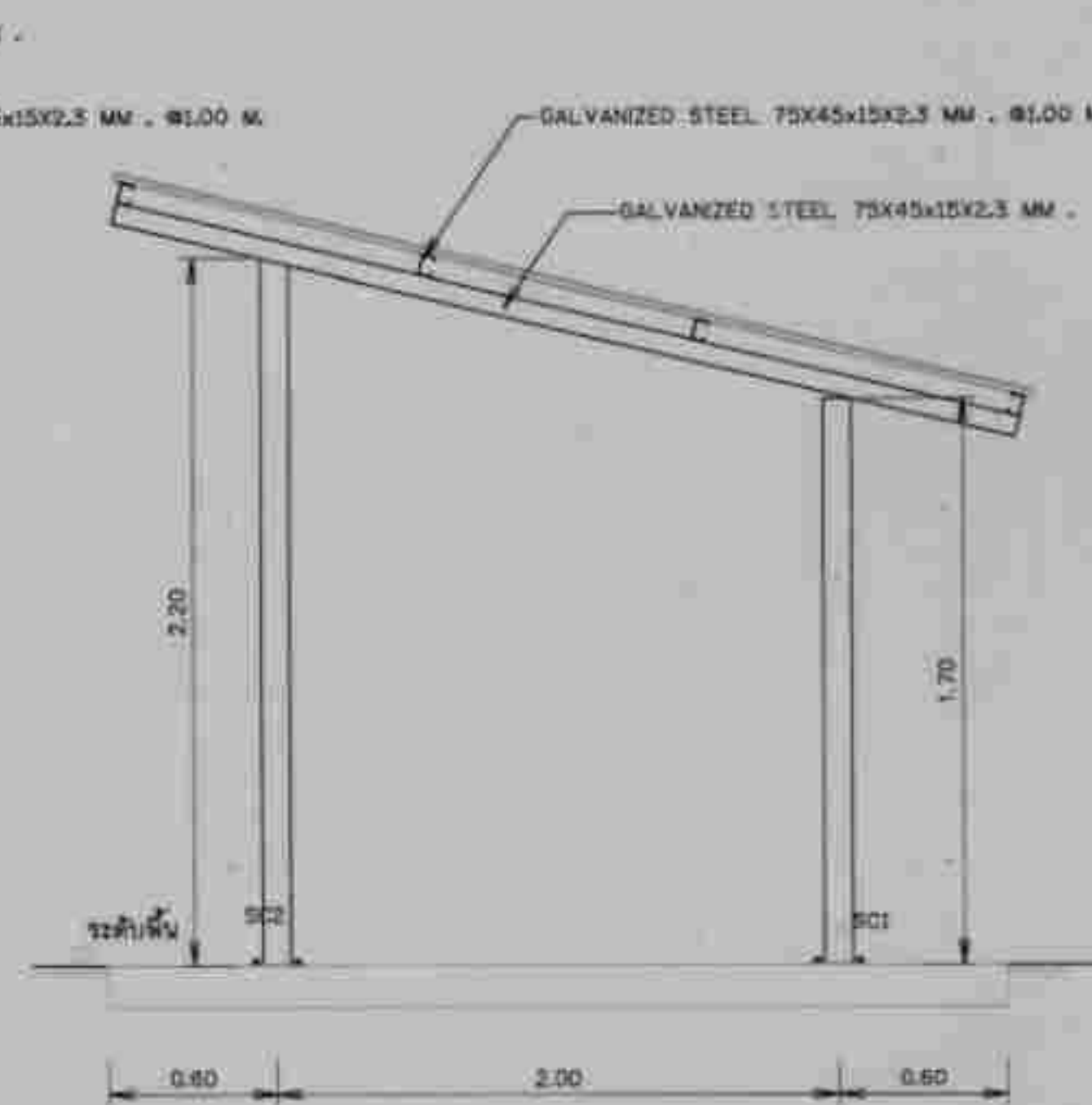
รูปด้าน 4 โมดูลขนาดฐาน
