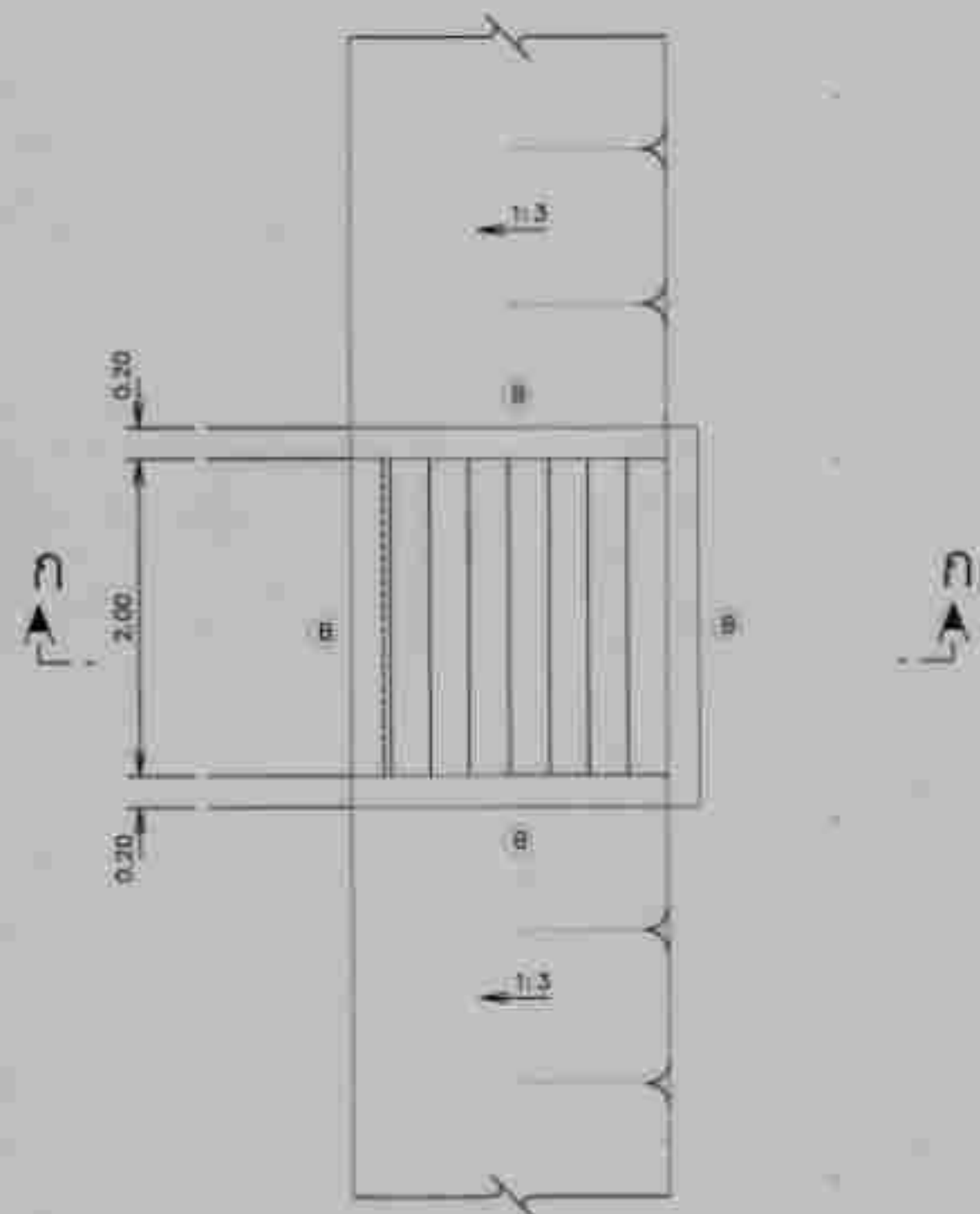
แปลนอาคารป็นโด คสล.
