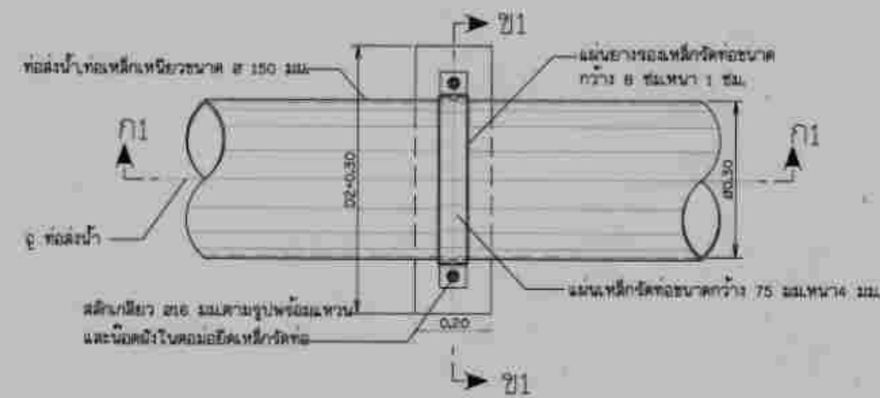
แปลนการยึดท่อ ไม่แสดงขนาดราส่วน
