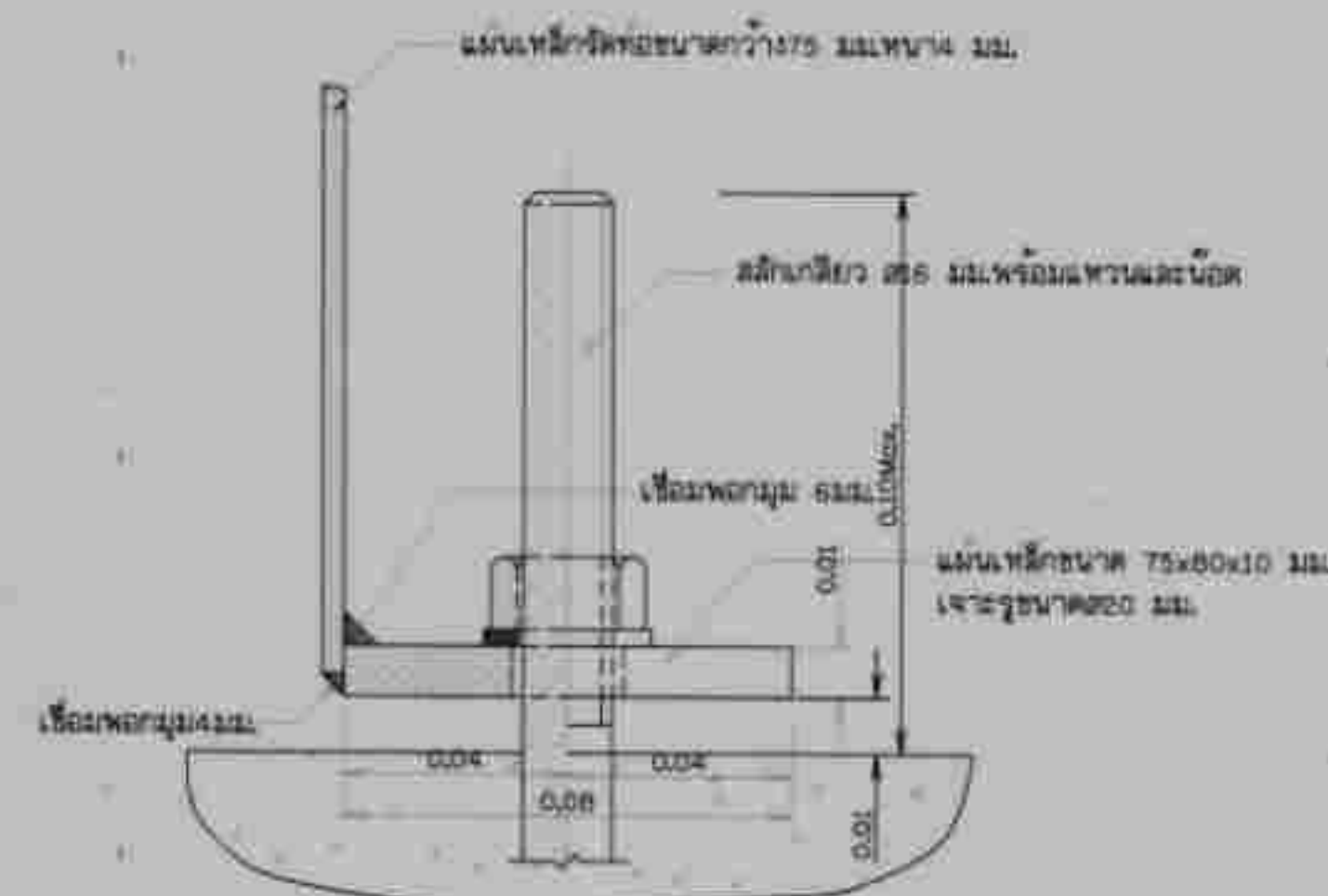
แปลนการยึดท่อ ไม่แสดงขนาดราส่วน
