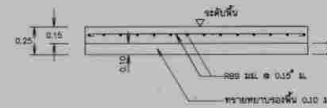
รูปตัด ก1 - ก1 ขนาดฐาน 1:20
