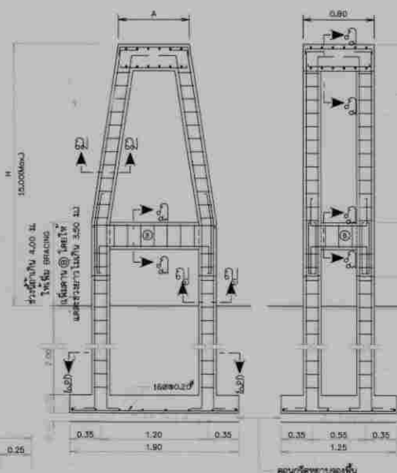
ดอมอรับท่อแบบที่ 3
