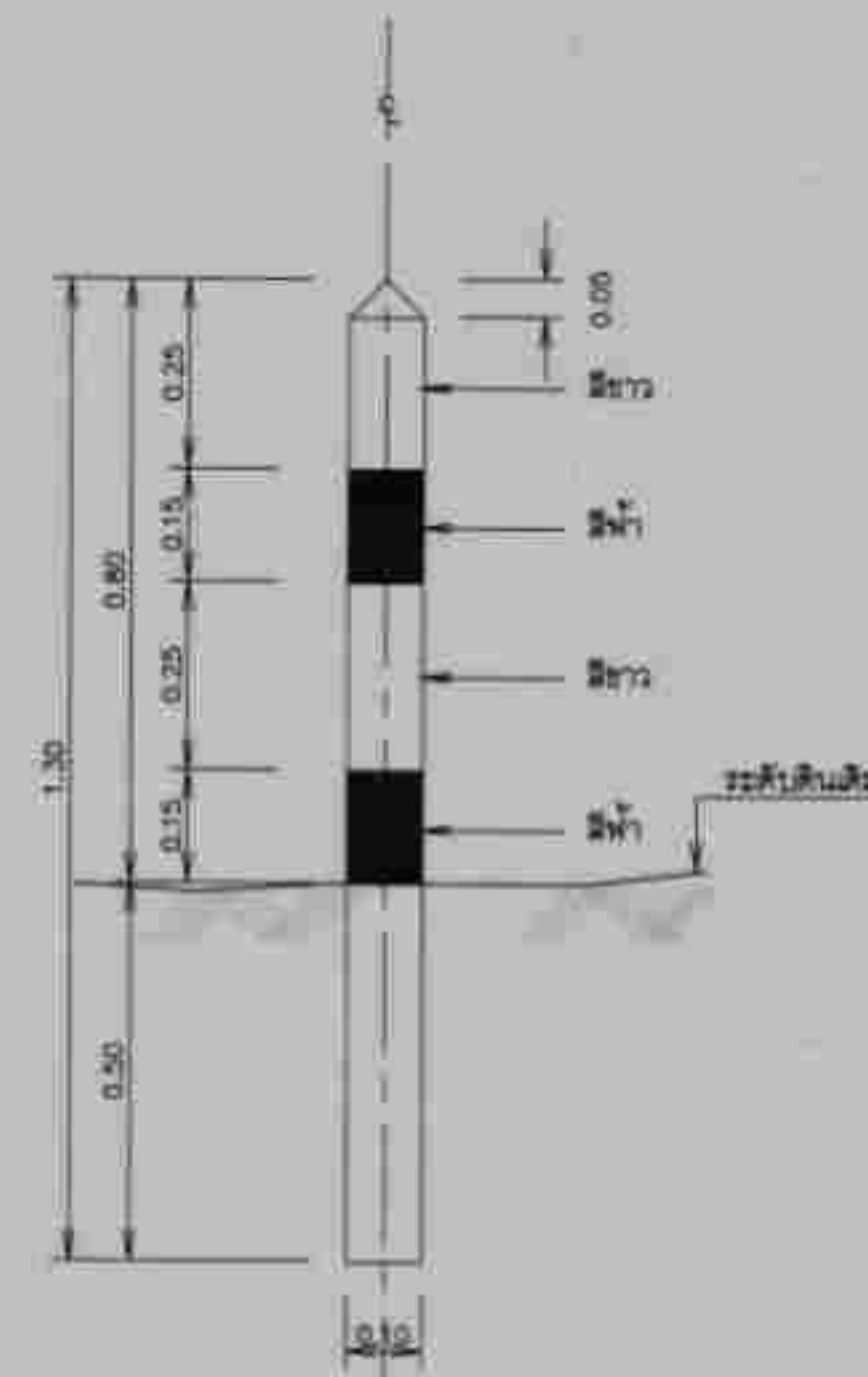
แสดงลัดส่วนหลักบ่อแกวท่อ มาตราส่วน 1:10
