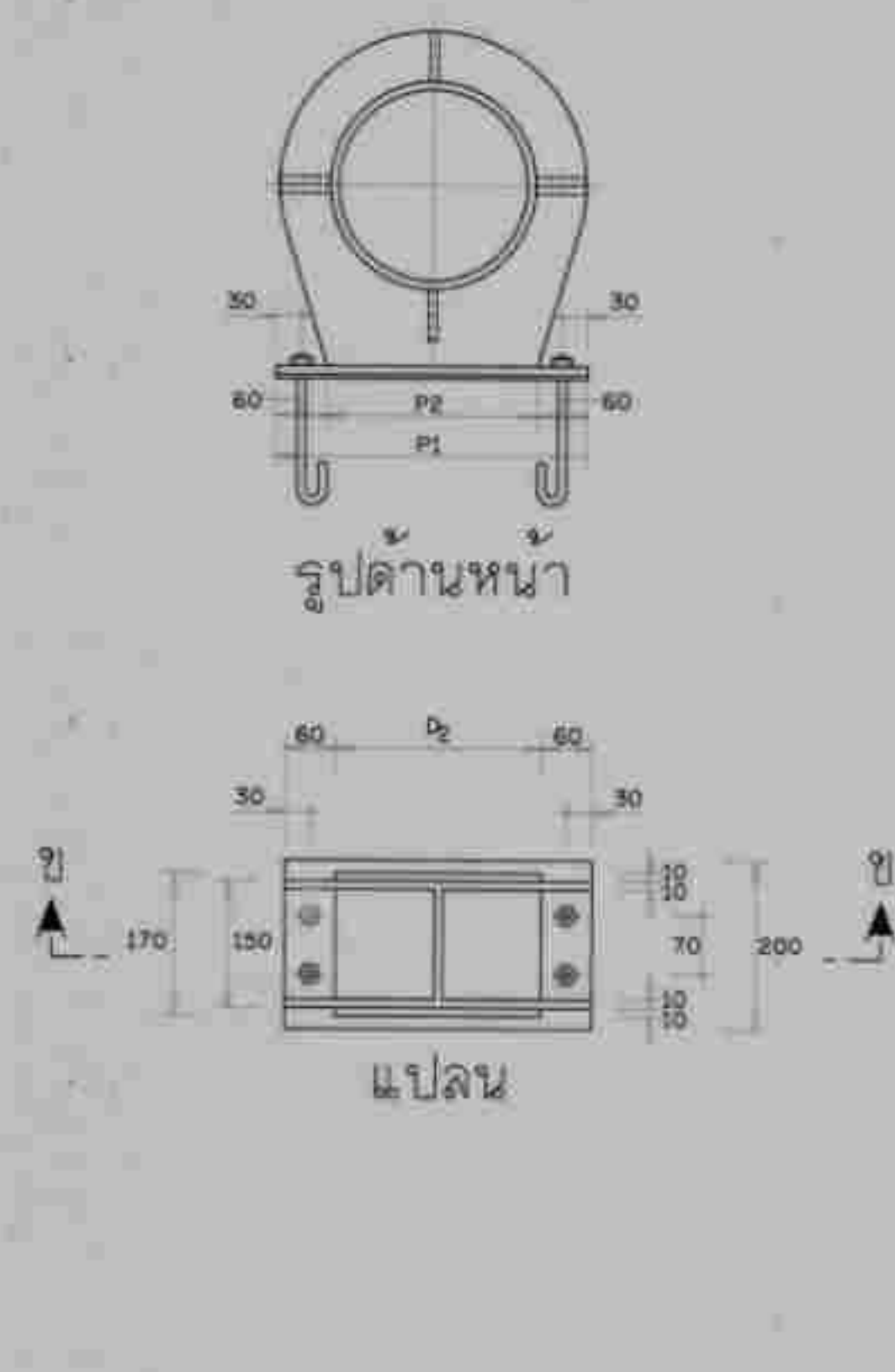
PIPE SUPPORT สำหรับท่อเหล็กขนาด Ø 300 มม.
