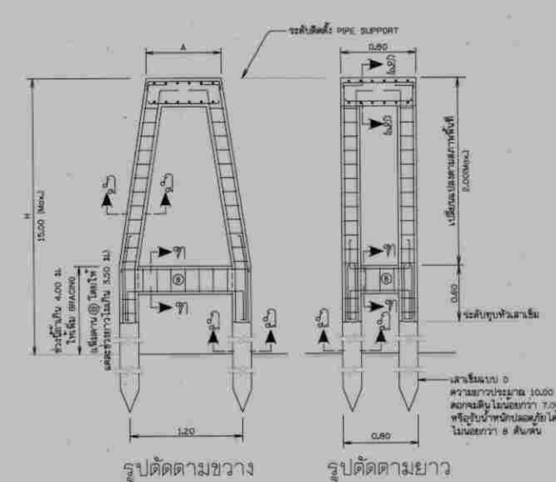
การเสริมเหล็ก ตอม่อแบบที่ 4
