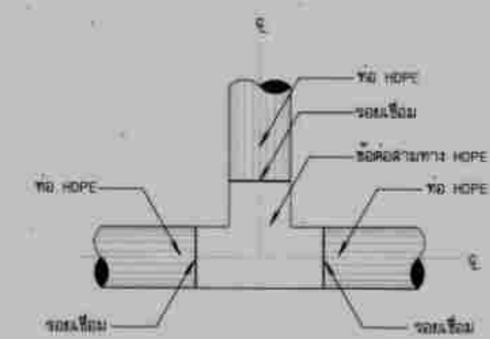
การบรรจุบล็อกลูกท่อสามทาง HDPE กับท่อ HDPE
