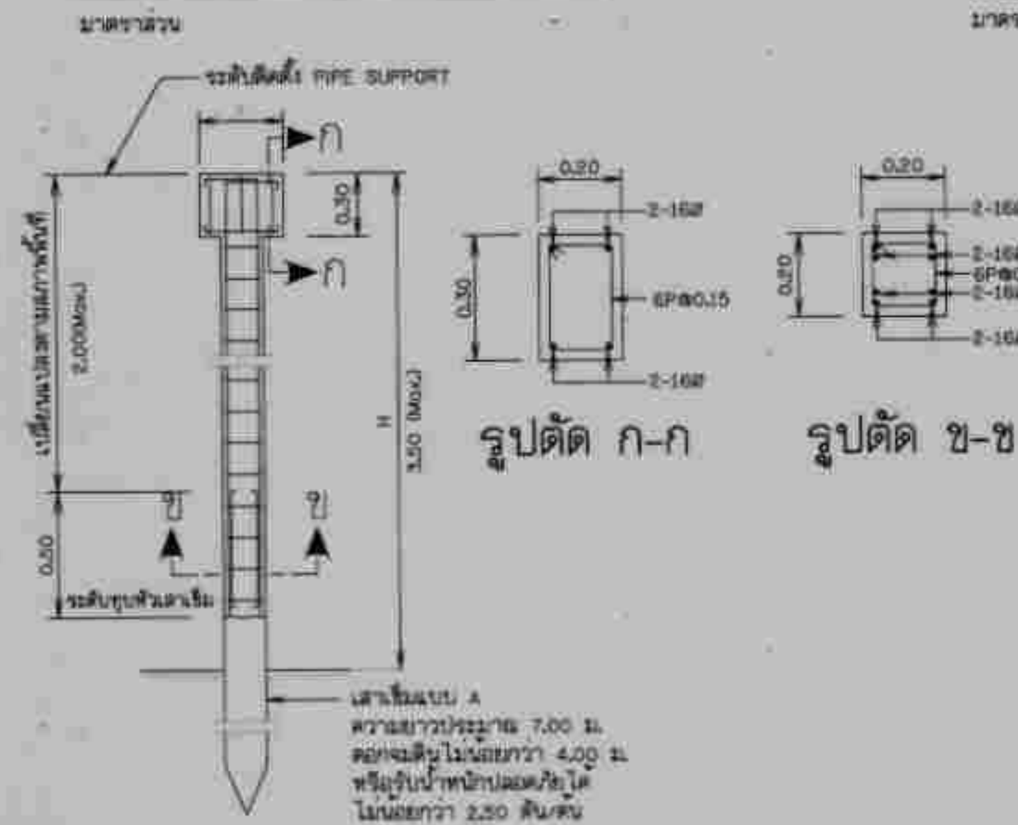
การเสริมเหล็ก ดอม่อบบที่ 1
