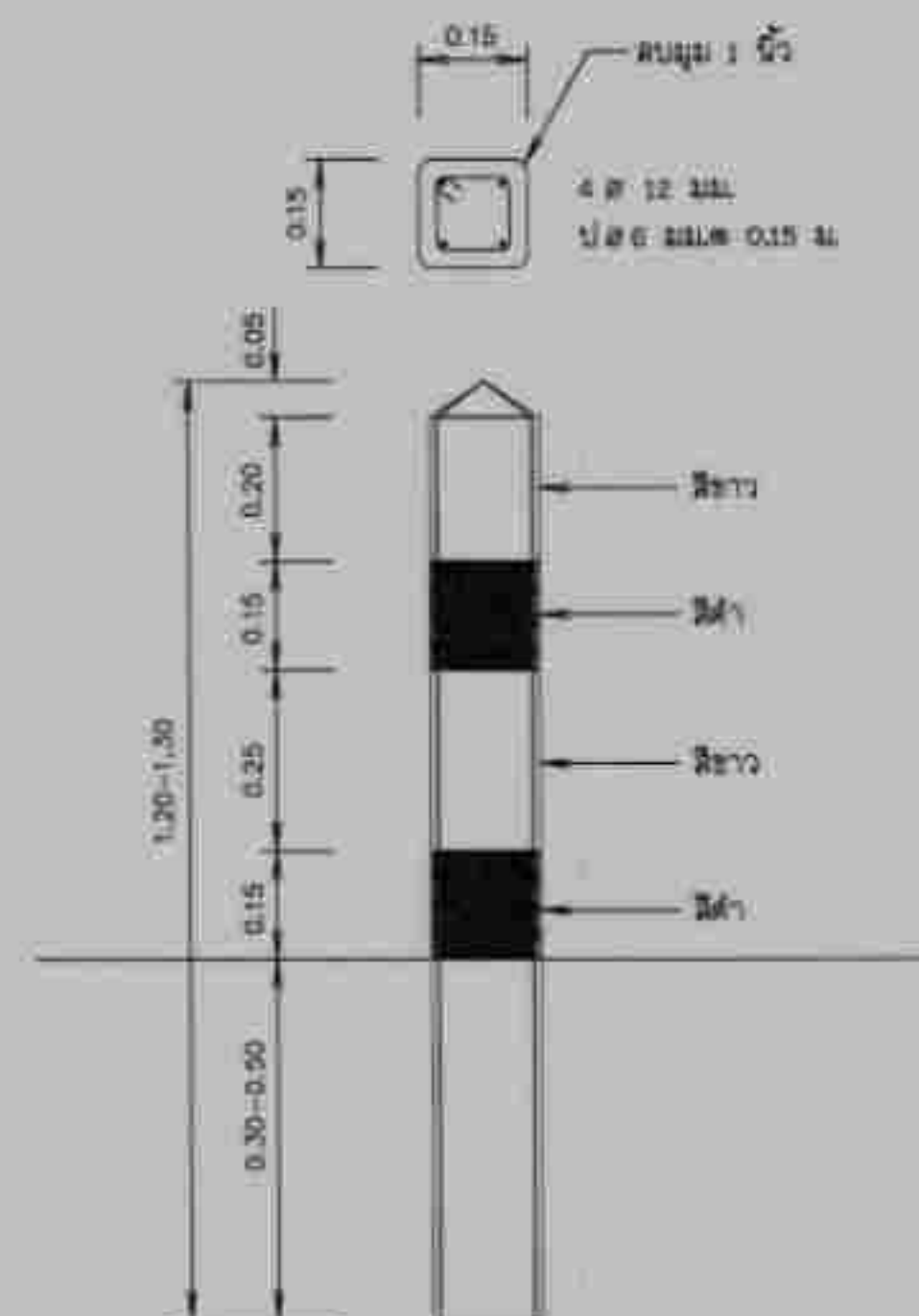
แบบขยายหลักโครงสร้าง คสล.
