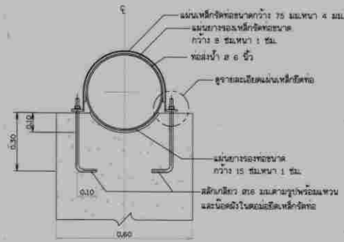
แปลนการยึดท่อ ไม่แสดงขนาดราส่วน
