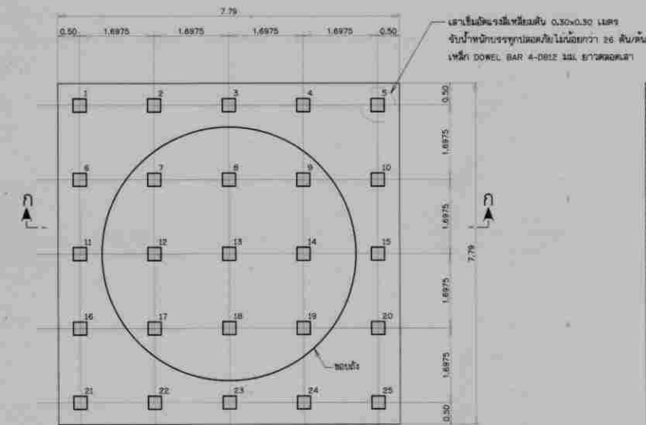
แบบฐานรากแบบเสาเข็ม
