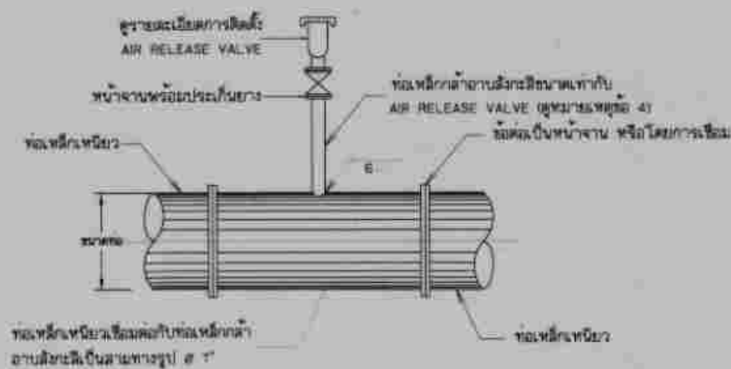
รายละเอียดข้อต่อแบบที่ 1
