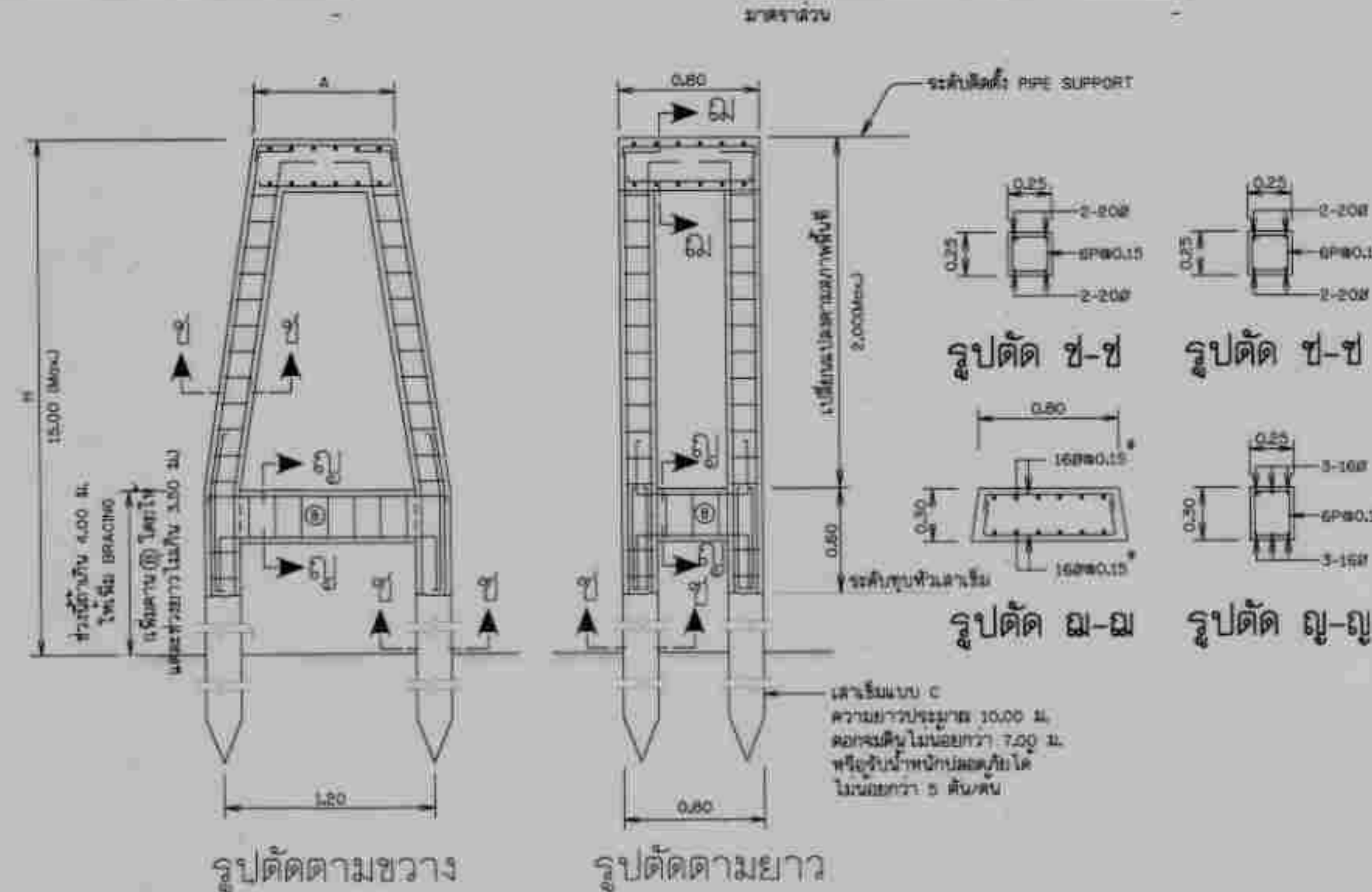
ต่อม่อรับทอแบบที่ 2
