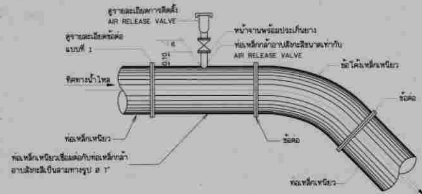
AIR RELEASE VALVE แบบท่อลงน้ำขามหอย
