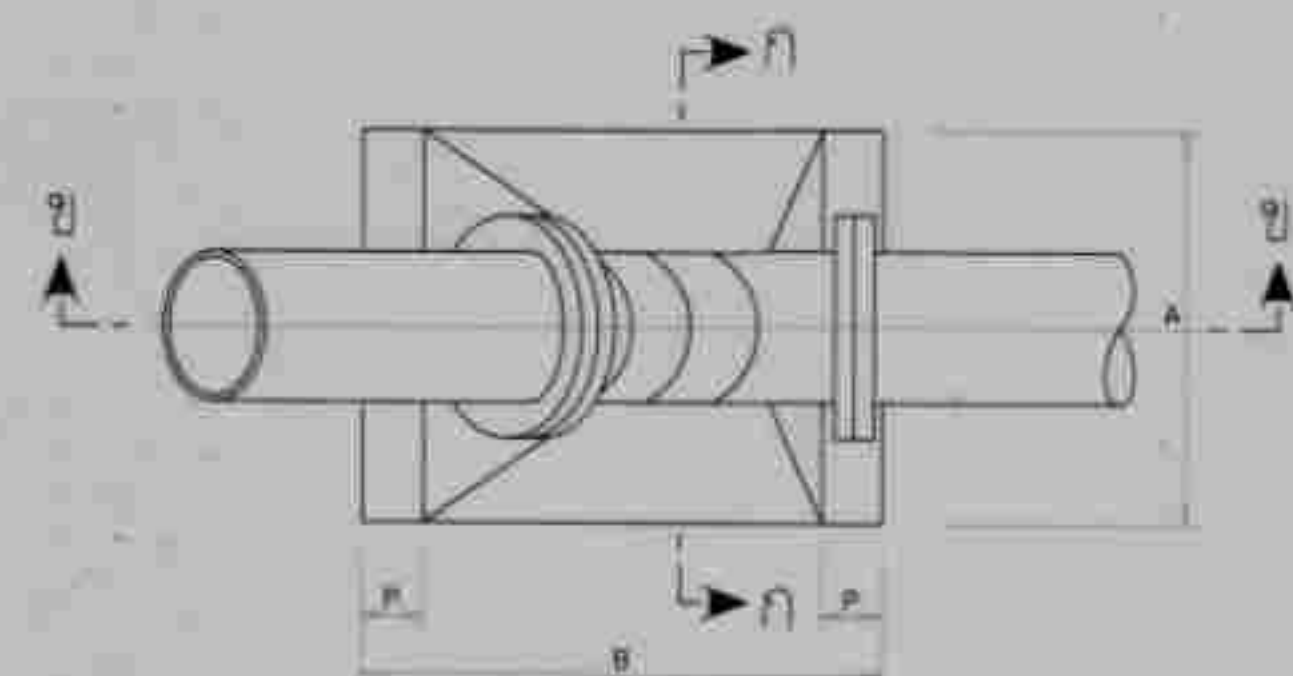
แปลน THRUST BLOCK รับท่อต่อโค้งแนวตั้ง
