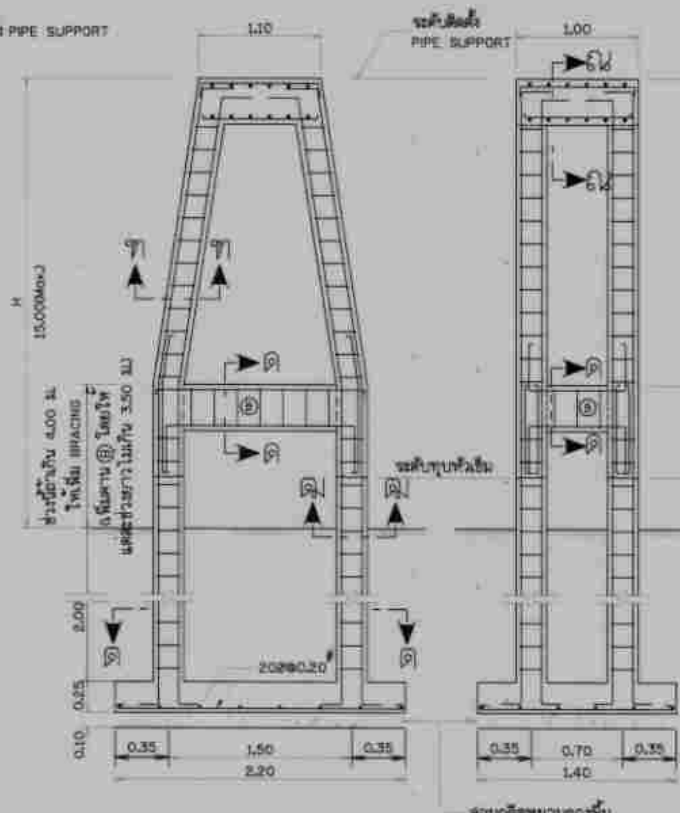
ดอมอรับท่อแบบที่ 5
