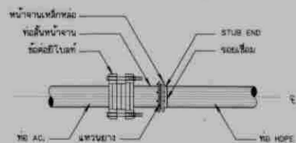
การบรรจุบล็อกลูกท่อ AC. กับท่อ HDPE
