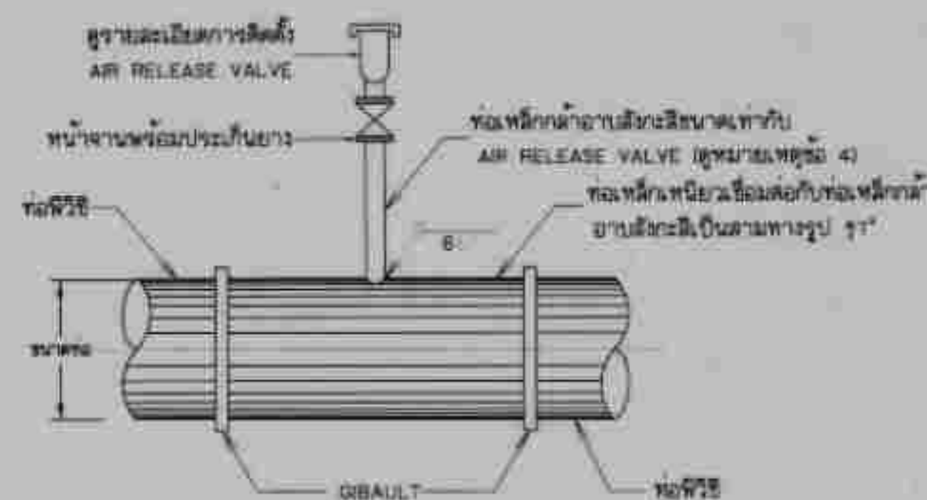
รายละเอียดข้อต่อแบบที่ 2
