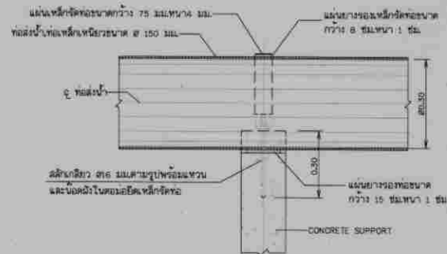
แปลนการยึดท่อ ไม่แสดงขนาดราส่วน
