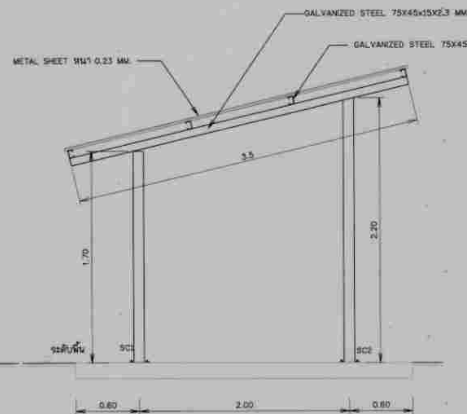
รูปด้าน 2 โมดูลขนาดฐาน
