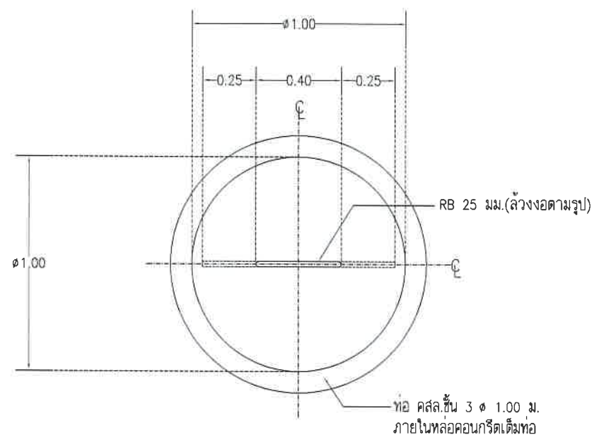
แปลนแท่นส่อมยึดอาคารโรงสูบน้ำ
