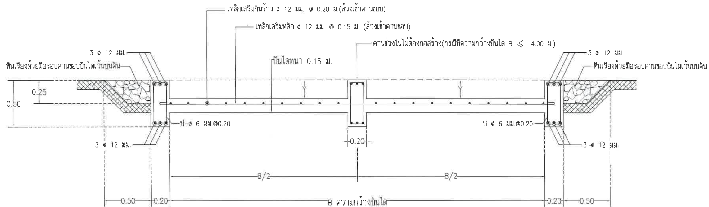
ขยายคานช่วงใน มาตราส่วน 1:25
