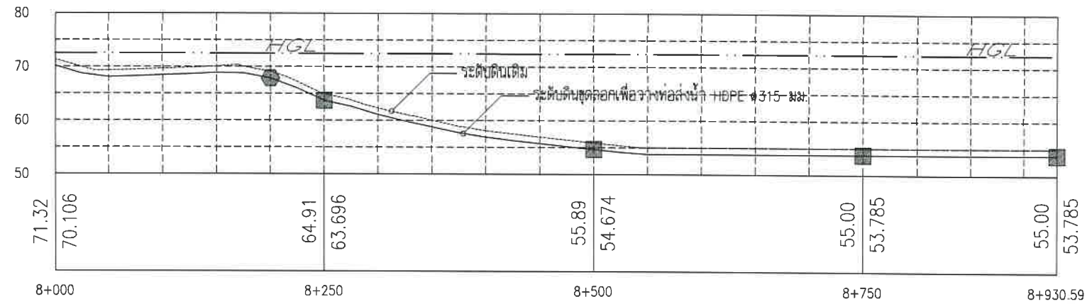
PROFILE แนวท่อส่งน้ำ LINE R
