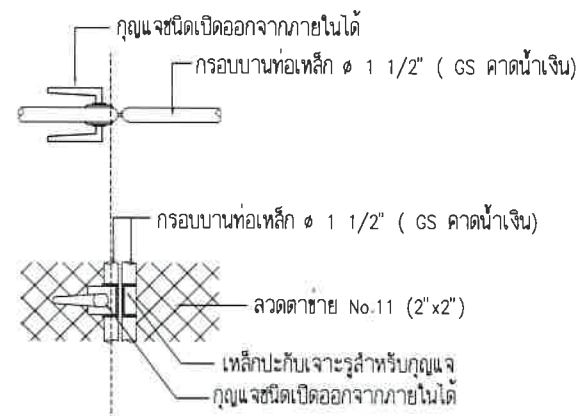
แบบขยาย 2
