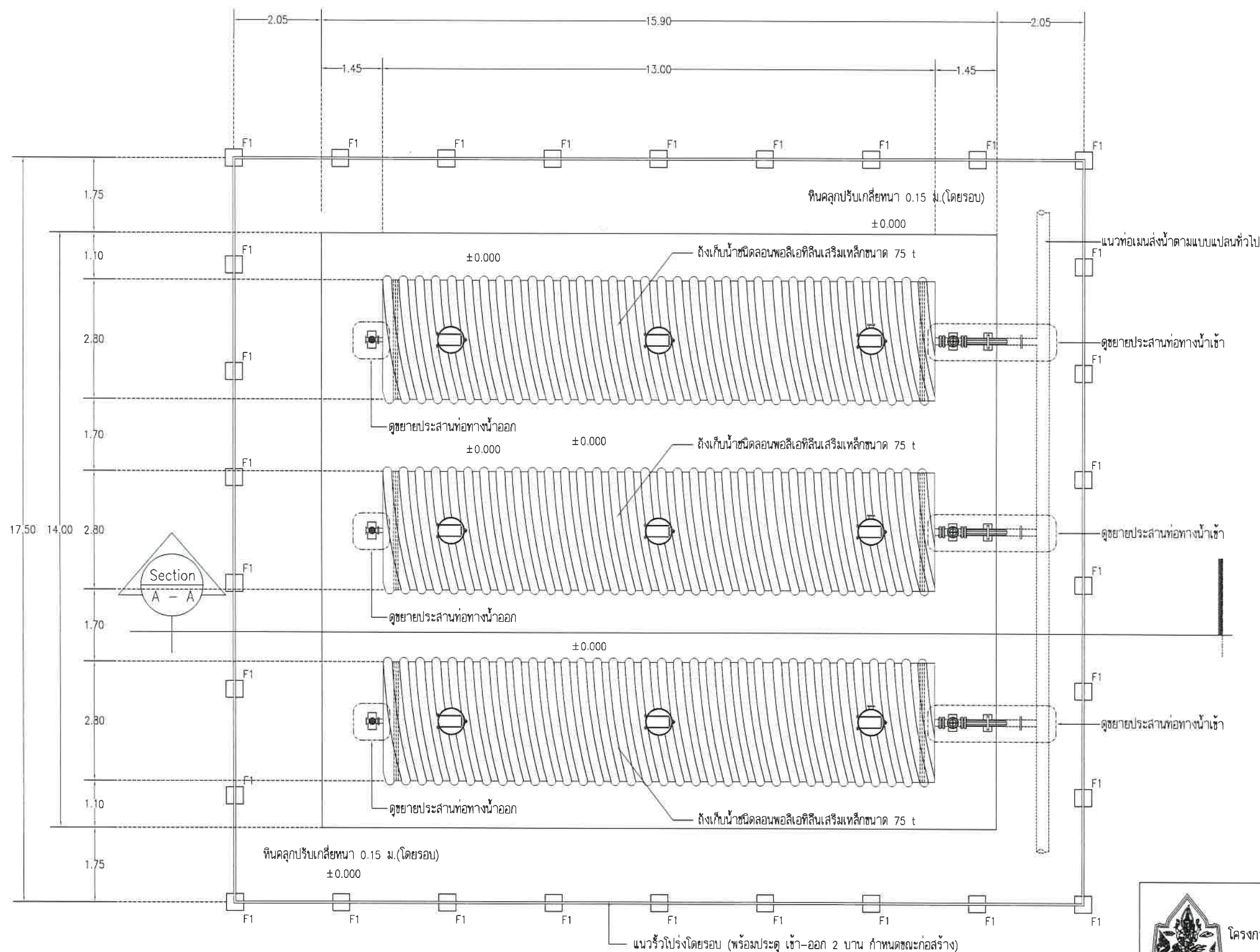
แผนผังถังเก็บน้ำสำรอง ชนิดลอนพอลิเอทิลีนเสริมเหล็ก ขนาด 75 T จำนวน 3 ชุด
