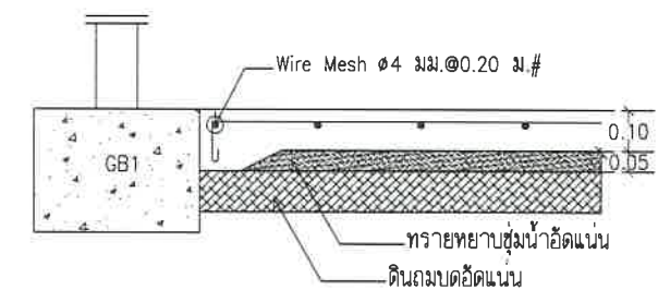
ขยายพื้น GB1
