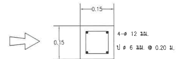
ขยายเสาป้ายใต้ป้าย - หัวเสา
