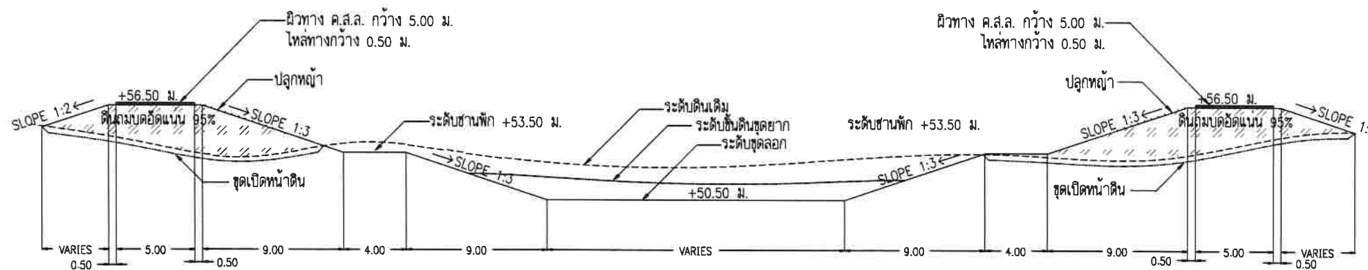
รูปตัดทั่วไปงานขุดลอก
