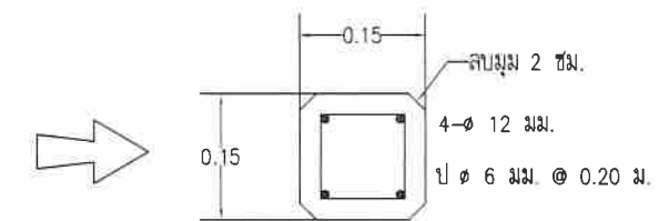
ขยายเสาป้ายฐานเสา - ใต้แผ่นป้าย
