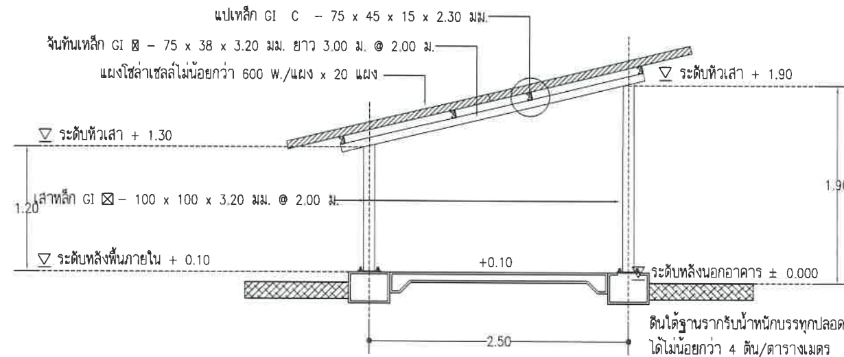
รูปตัดตามขวาง
