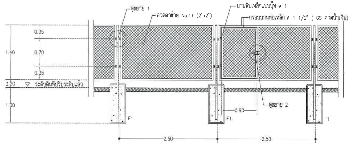
รูปด้านรั้วโปร่ง-ประตู
