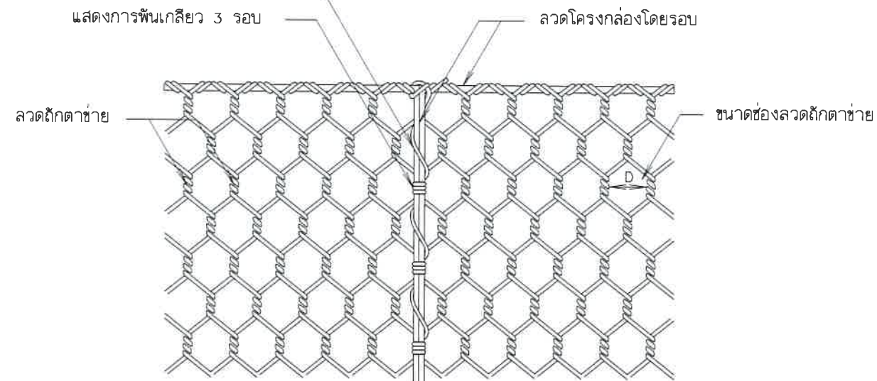
รูปแสดงการพันลวดระหว่างกล่องลวดตาข่ายและฝาปิด
