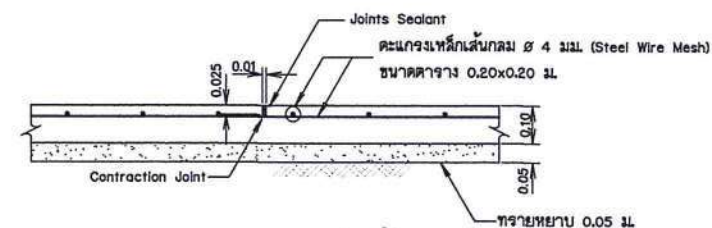
แบบขยายรอยต่อพื้น (Contraction Joint) ไม่แสดงขนาดจริง
