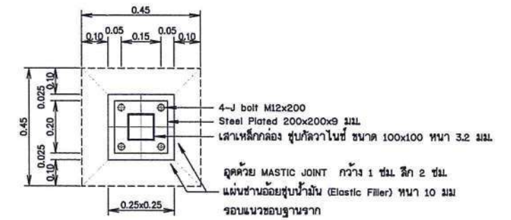
รูปตัด ก-ก ไม่แสดงขนาดจริง
