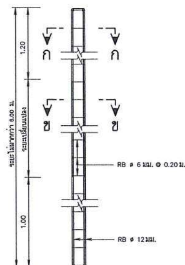
รายละเอียดส่่าย คสล.
