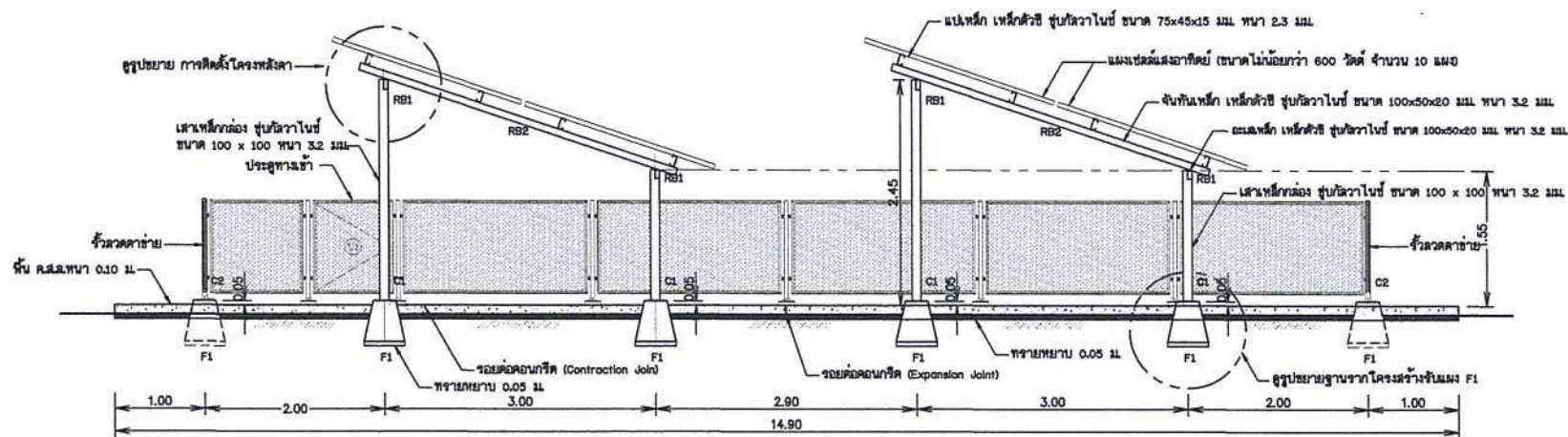
รูปด้านข้าง ไม่แสดงขนาดจริง
