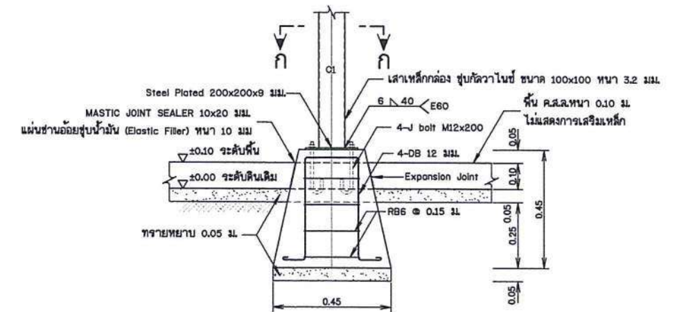
รูปขยายฐานรากโครงสร้างรับแผง F1 (ต่อม่อ คสล. หล่อสำเร็จรูปพร้อมติดตั้ง) ไม่แสดงขนาดจริง
