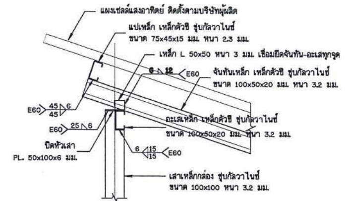
รูปขยาย การติดตั้งโครงหลังคา ไม่แสดงขนาดจริง
