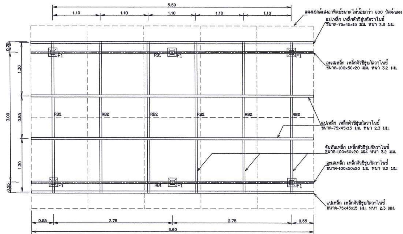
แปลนฐานรากและโครงหลังคา ไม่แสดงขนาดจริง
