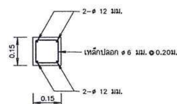
รายละเอียดส่่าย คสล.
