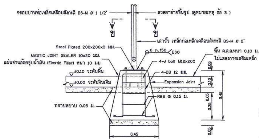
รูปขยายฐานรากโครงสร้างรับแผง F1 (คอม่อ คสล. หล่อสำเร็จรูปพร้อมติดตั้ง) ไม่แสดงมาตราส่วน
