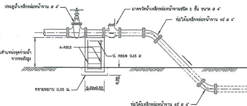
14. การติดตั้งมาตรวัดน้ำบนพื้นดิน ๔"
