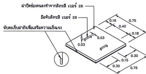
ขยายฝาปิดช่องคนลง
