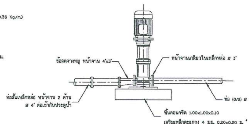
15. การต่อท่อเครื่องสูบน้ำ
