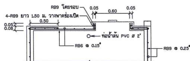
แสดงการเสริมเหล็กฝาลัง
