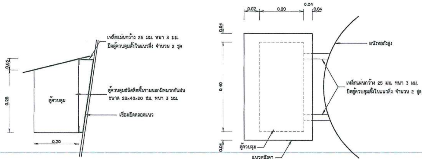
แบบขยายตัวควบคุม ไม่แสดงมาตราส่วน
