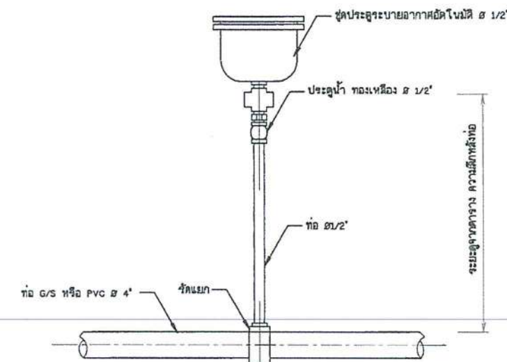
12. การติดตั้งประตูละบายอากาศอัตโนมัติ
