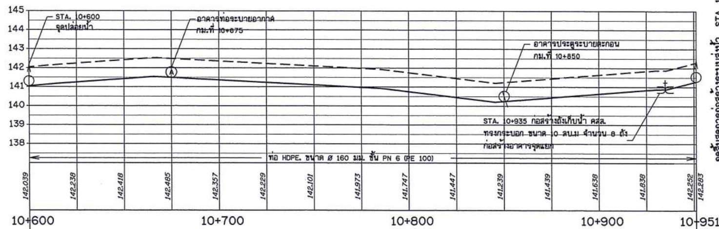
รูปตัดตามแนวยาว STA. 10+600 - 10+951
