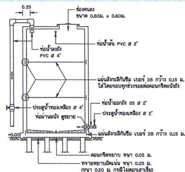
รูปตัด (1)
