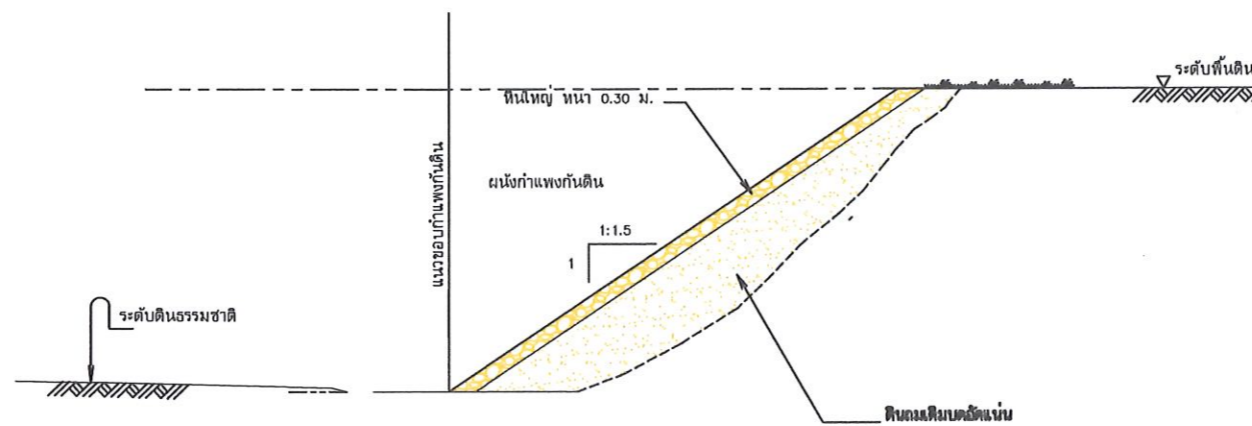
รูปตัดทั่วไปแสดงการเรียงหินในกล่องที่ความลาดชัน 1:1.5 (เฉพาะแห่ง)
