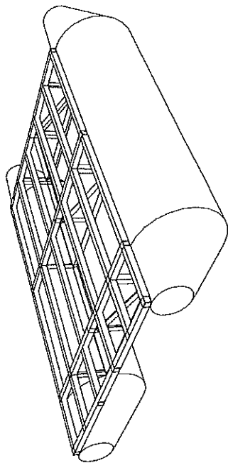
รูปแสดงการติดตั้งโครงเหล็ก
