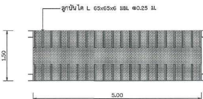
แบบขยายสะพานช่วงที่ 6 มาตราส่วน 1 : 100
