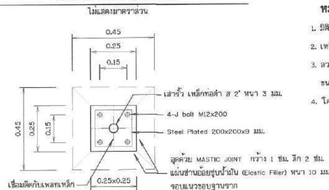
รูปขยายฐานรากโครงสร้างรับแผง F2 (ต่อม่อ คสล. หลังสำเร็จรูปพร้อมติดตั้ง)
