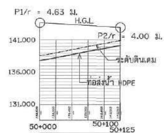
รูปตัดตามแนวยาวแสดง H.G.L. กม. 50+000
