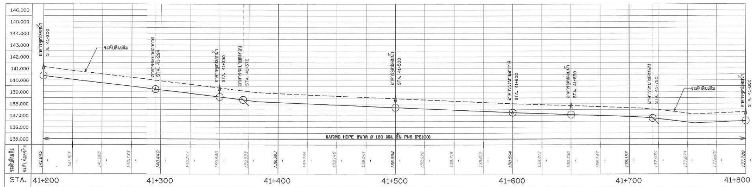
รูปตัดตามแนวยาว กม. 40+000 STA. 41+200 - 41+800
