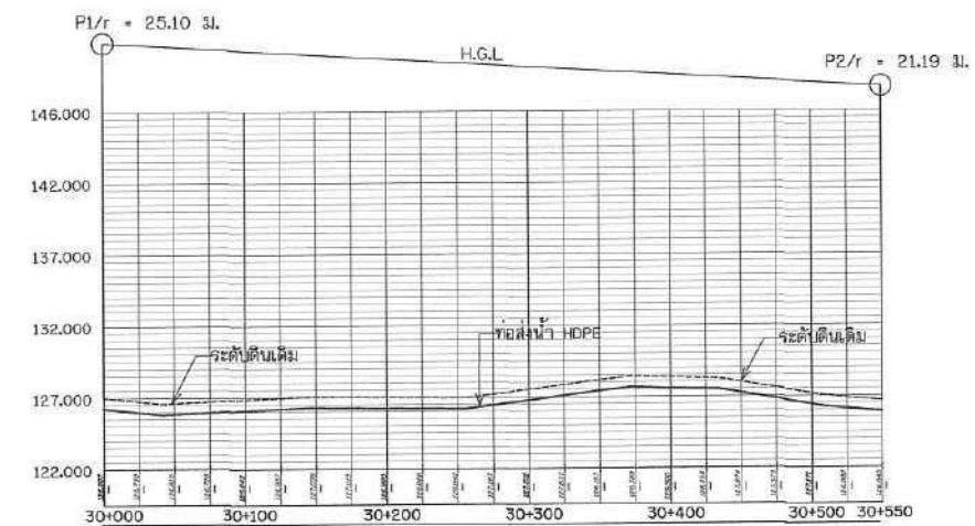
รูปตัดตามแนวยาวแสดง H.G.L. กม. 30+000
