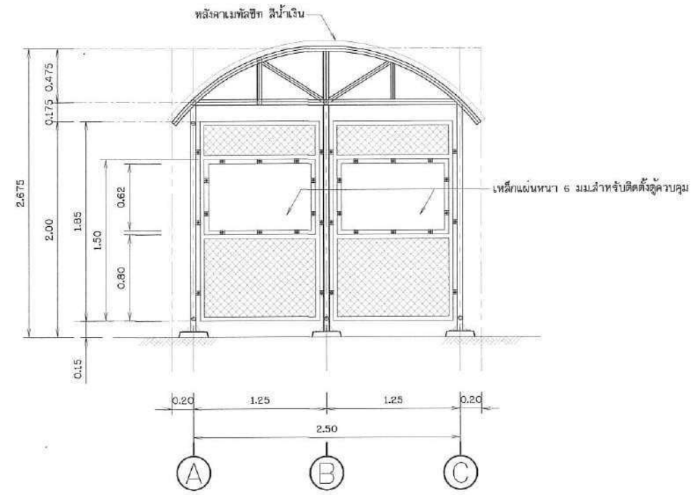
รูปด้าน 2 ไม่แสดงขนาดราวจับ
