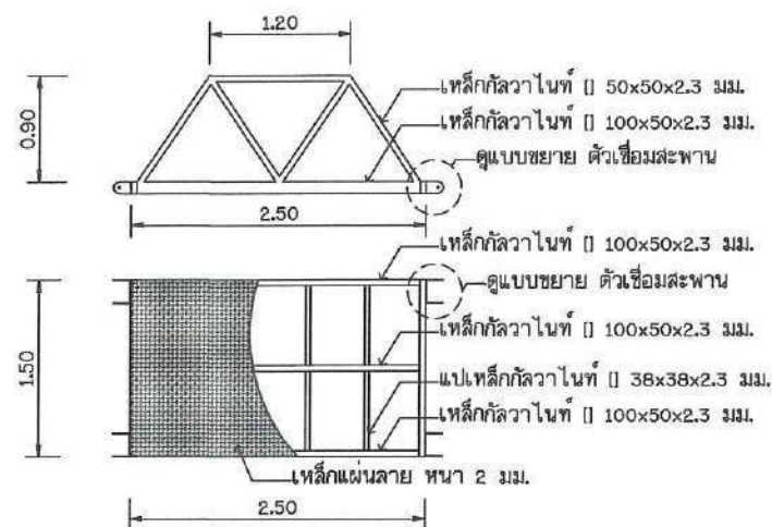
แบบขยายสะพานช่วงที่ 1 มาตราส่วน 1 : 100
