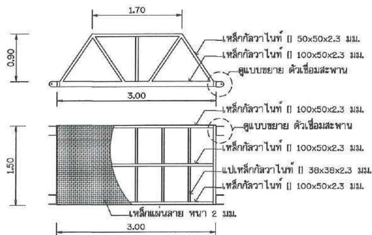
แบบขยายสะพานช่วงที่ 2 มาตราส่วน 1 : 100
