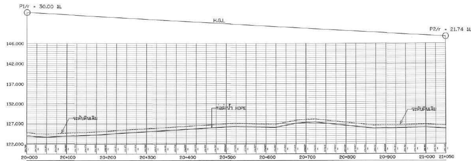
รูปตัดตามแนวยาวแสดง H.G.L. กม. 20+000
