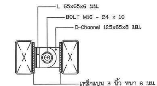
แบบขยายสะพานช่วงที่ 10 มาตราส่วน 1 : 100
