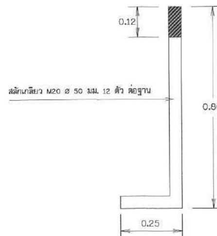
แบบขยายสลักเกลียวยึดฐาน มาตราส่วน 1:10
