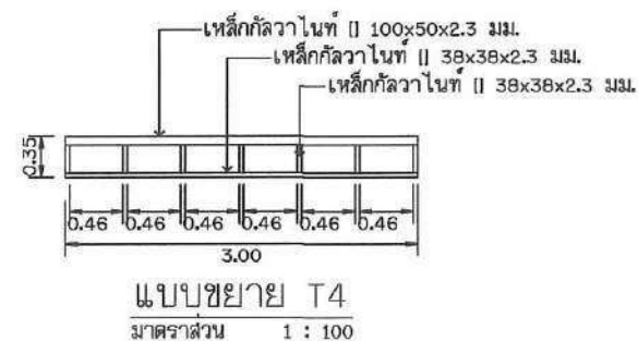
แบบขยายสะพานช่วงที่ 4 มาตราส่วน 1 : 100
