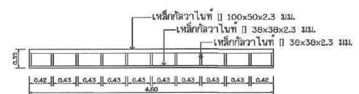
แบบขยาย T2 มาตราส่วน 1 : 100
