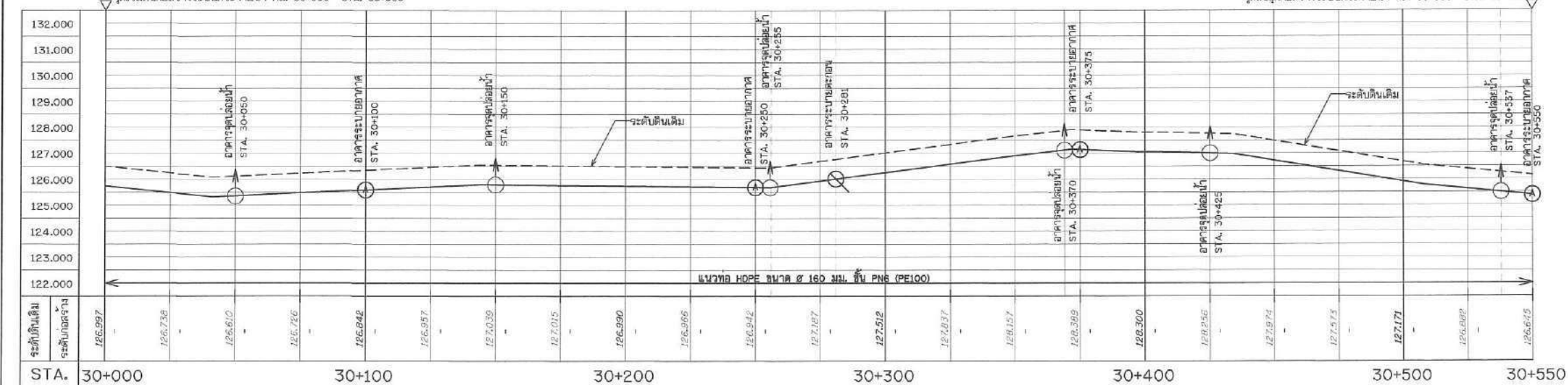
รูปตัดตามแนวยาว กม. 30+000 STA. 30+000 - 30+550 1:1,000 1:100
