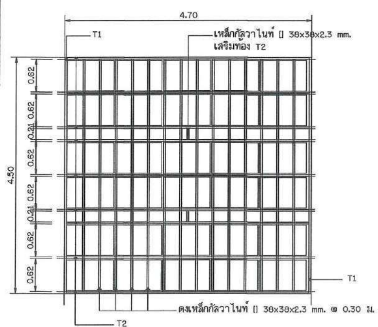
แปลนโครงรับพื้น มาตราส่วน 1 : 100
