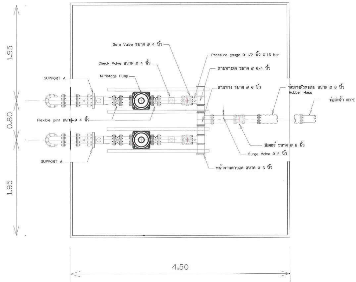
แปลนแสดงการติดตั้งเครื่องสูบน้ำ ขนาด 7.5 กิโลวัตต์ ไม่แสดงมาตราส่วน
