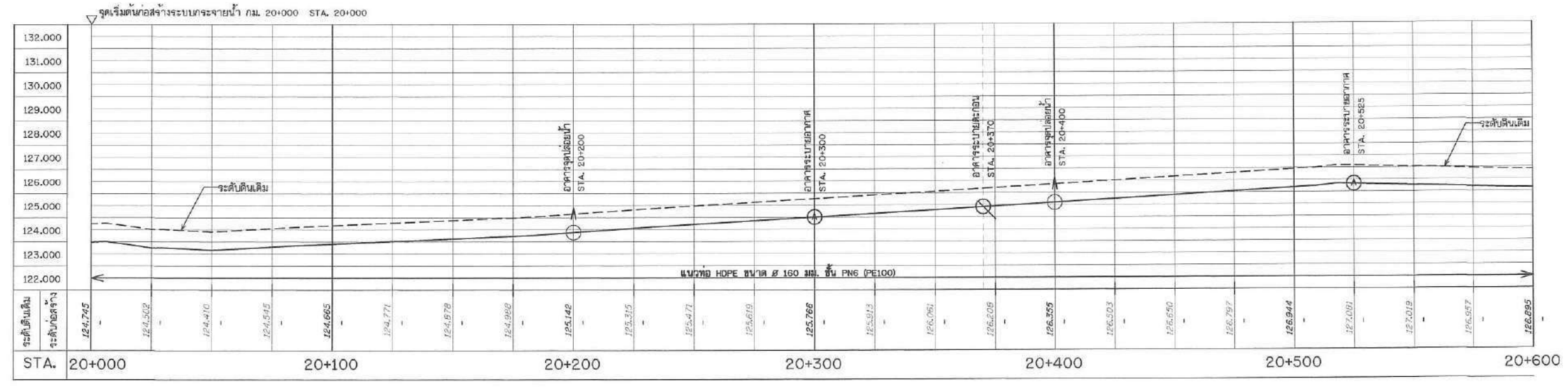
รูปตัดตามแนวยาว กม. 20+000 STA. 20+000 - 20+600
