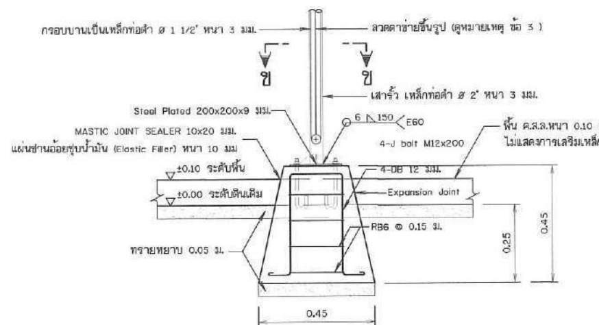
รูปขยายฐานรากโครงสร้างรับแผง F2 (ต่อม่อ คสล. หลังสำเร็จรูปพร้อมติดตั้ง)
