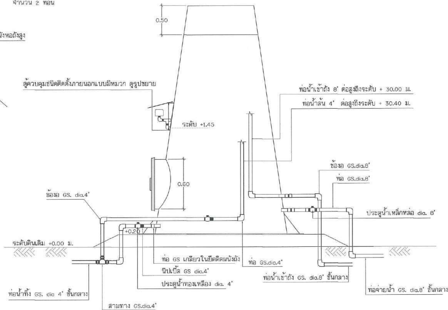
แบบแสดงการเดินท่อในถังแชมเปญ ไม่แสดงมาตราส่วน
