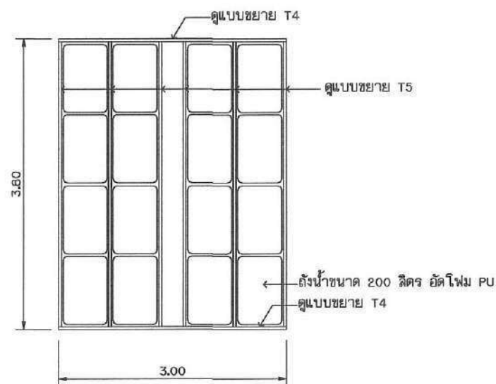
แบบขยายสะพานช่วงที่ 4 มาตราส่วน 1 : 100
