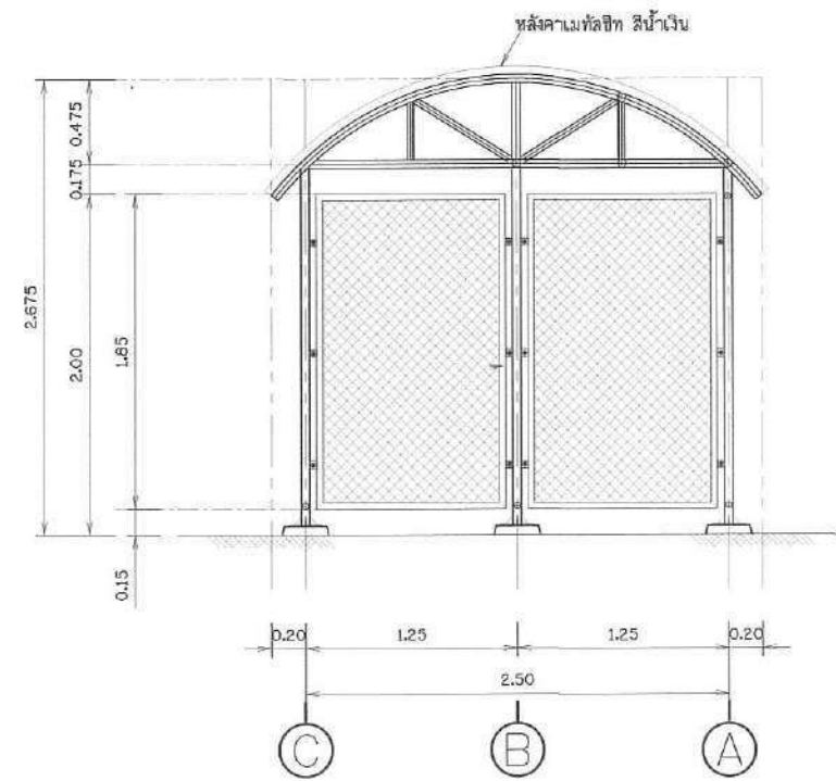
รูปด้าน 4 ไม่แสดงขนาดราวจับ
