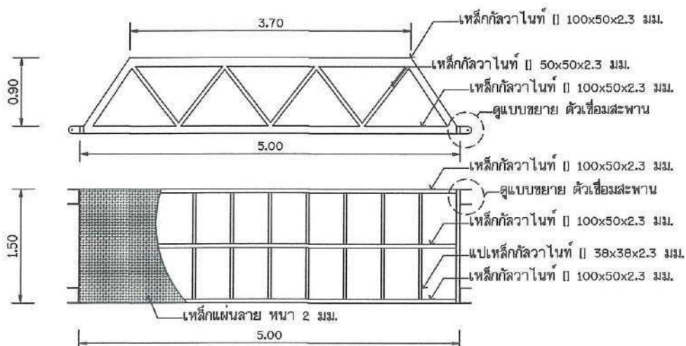
แบบขยายสะพานช่วงที่ 3 มาตราส่วน 1 : 100
