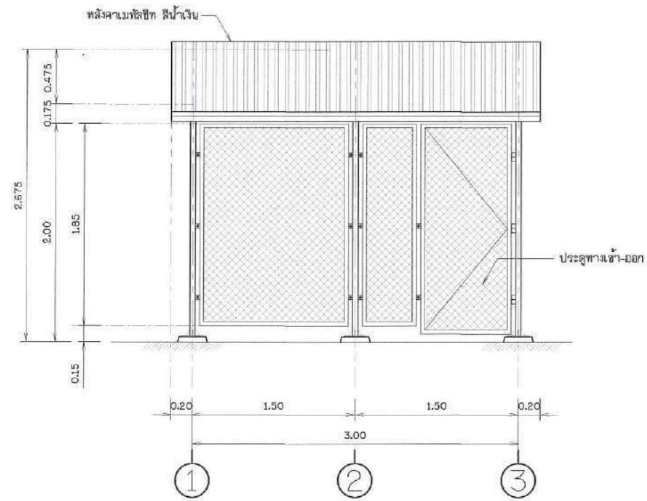
รูปด้าน 1 ไม่แสดงขนาดราวจับ
