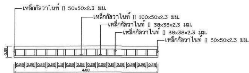
แบบขยาย T1 มาตราส่วน 1 : 100
