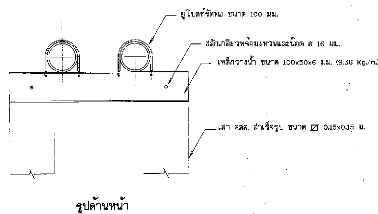
13. เสาคอมม่อนรับท่อชุด และแบบขยายอุปกรณ์รัดท่อ ไม่แสดงขนาดราส่วน
