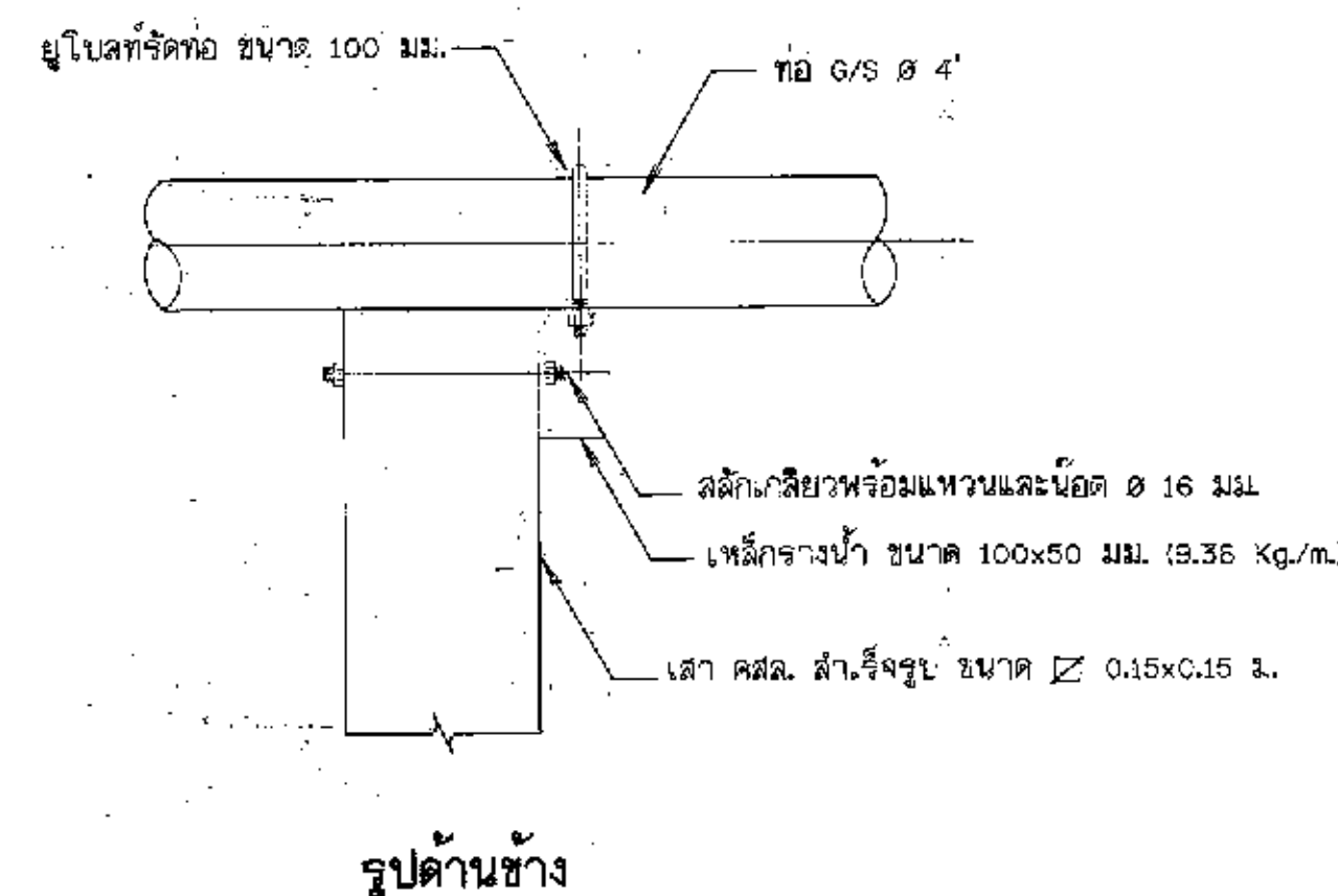
13. เสาคอมม่อนรับท่อชุด และแบบขยายอุปกรณ์รัดท่อ ไม่แสดงขนาดราส่วน
