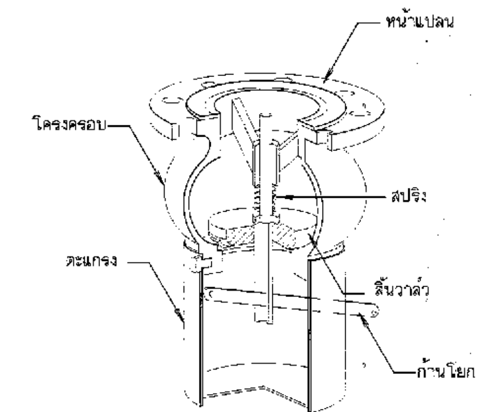
ฟุตวาล์ว แบบก้านโยก ไม่แสดงขนาดราส่วน
