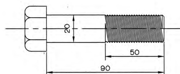
สลักเกลียวขนาด M20 ไม่แสดงมาตรฐาน
