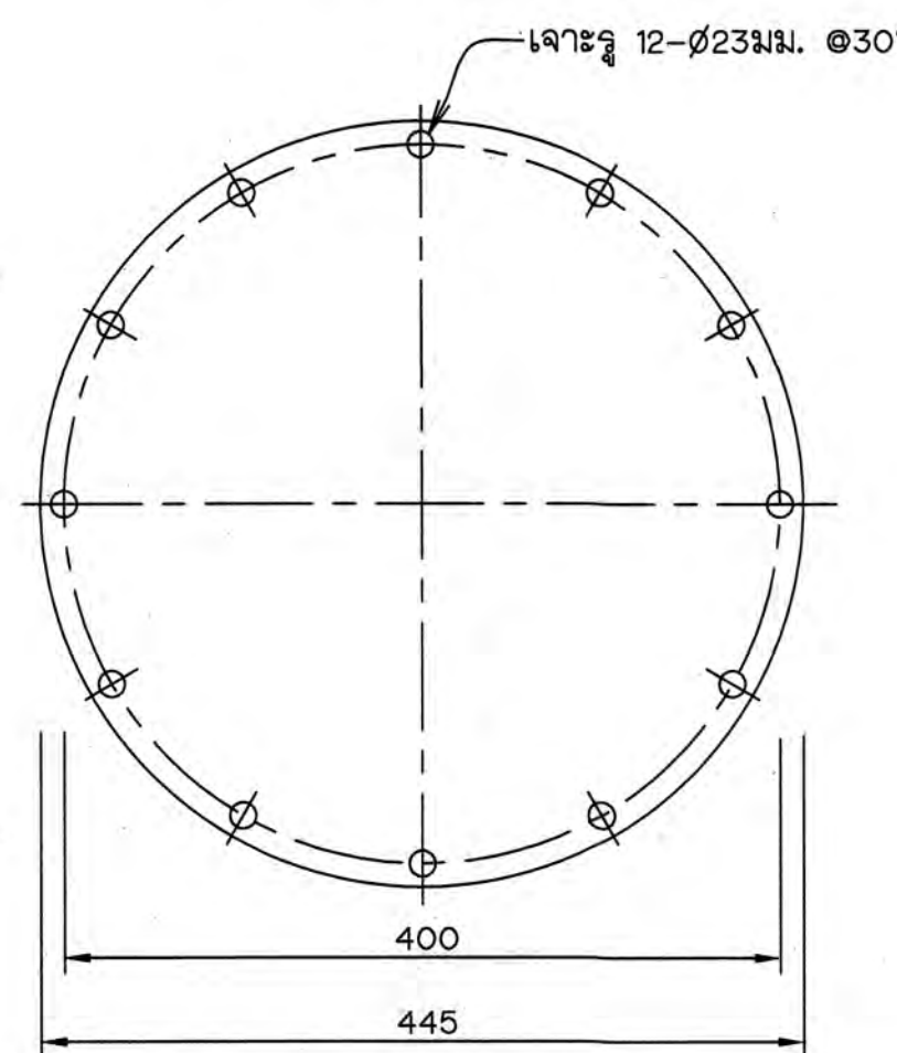
หน้าจานตาบอด
