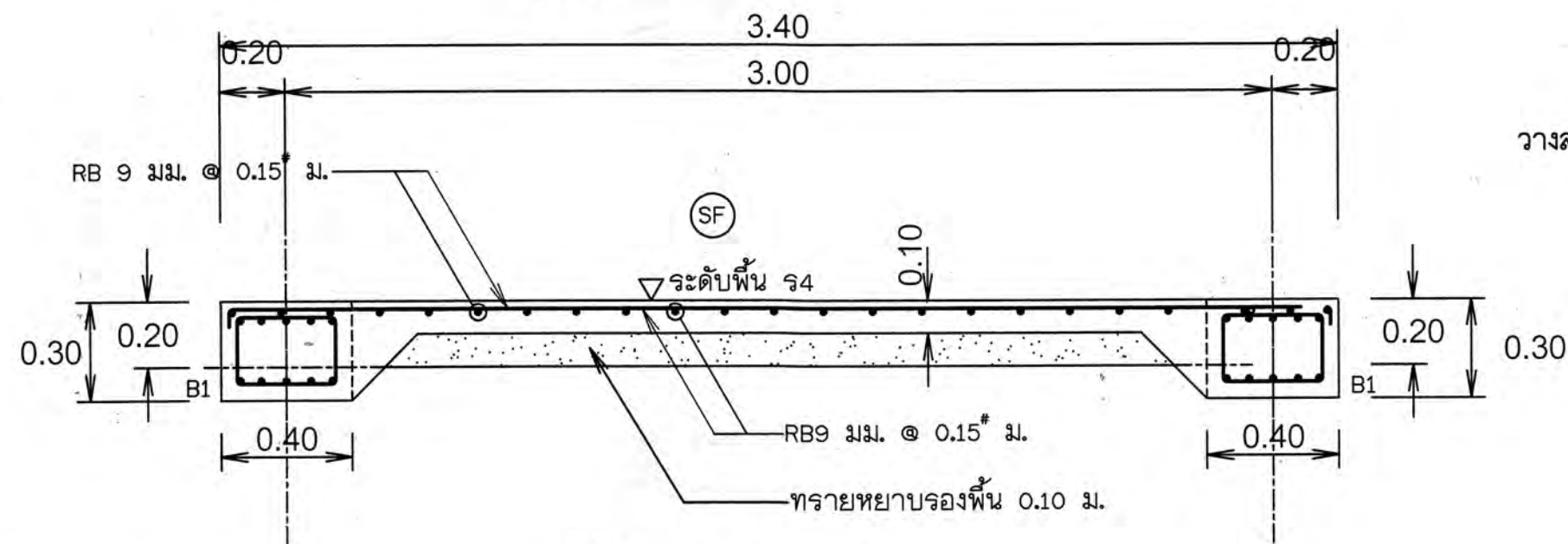
รูปตัด ก1 - ก1
