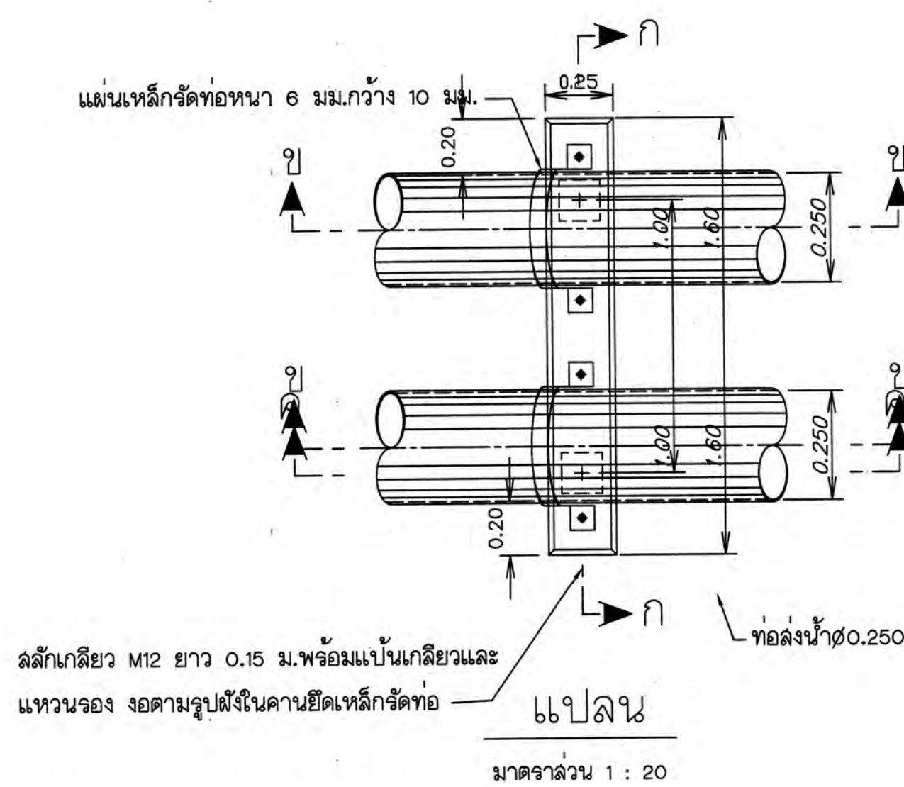
รายละเอียดทอริมตลิ่ง ลาด 1:20
