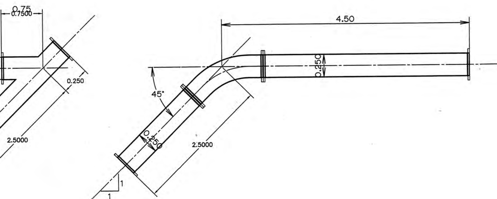
รายละเอียดทอริมตลิ่ง ลาด 1:1
