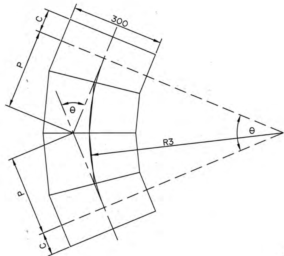
ข้อโค้ง 4 ชั้น
