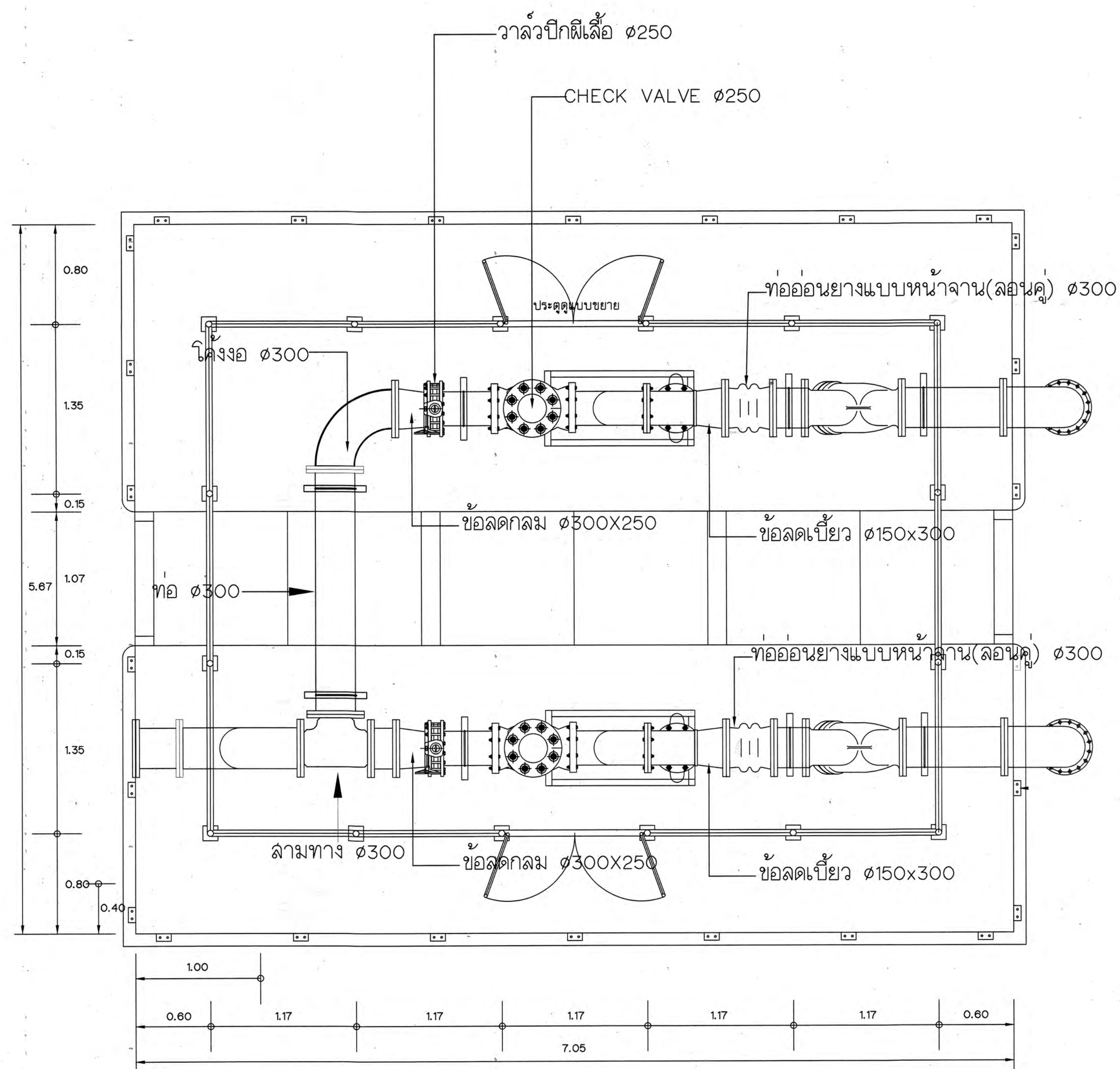
แปลนประลันทอภายในระบบ
