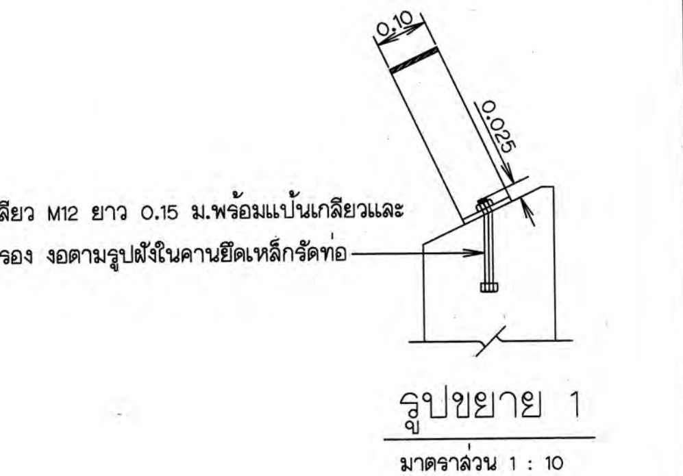
รายละเอียดทอริมตลิ่ง ลาด 1:10
