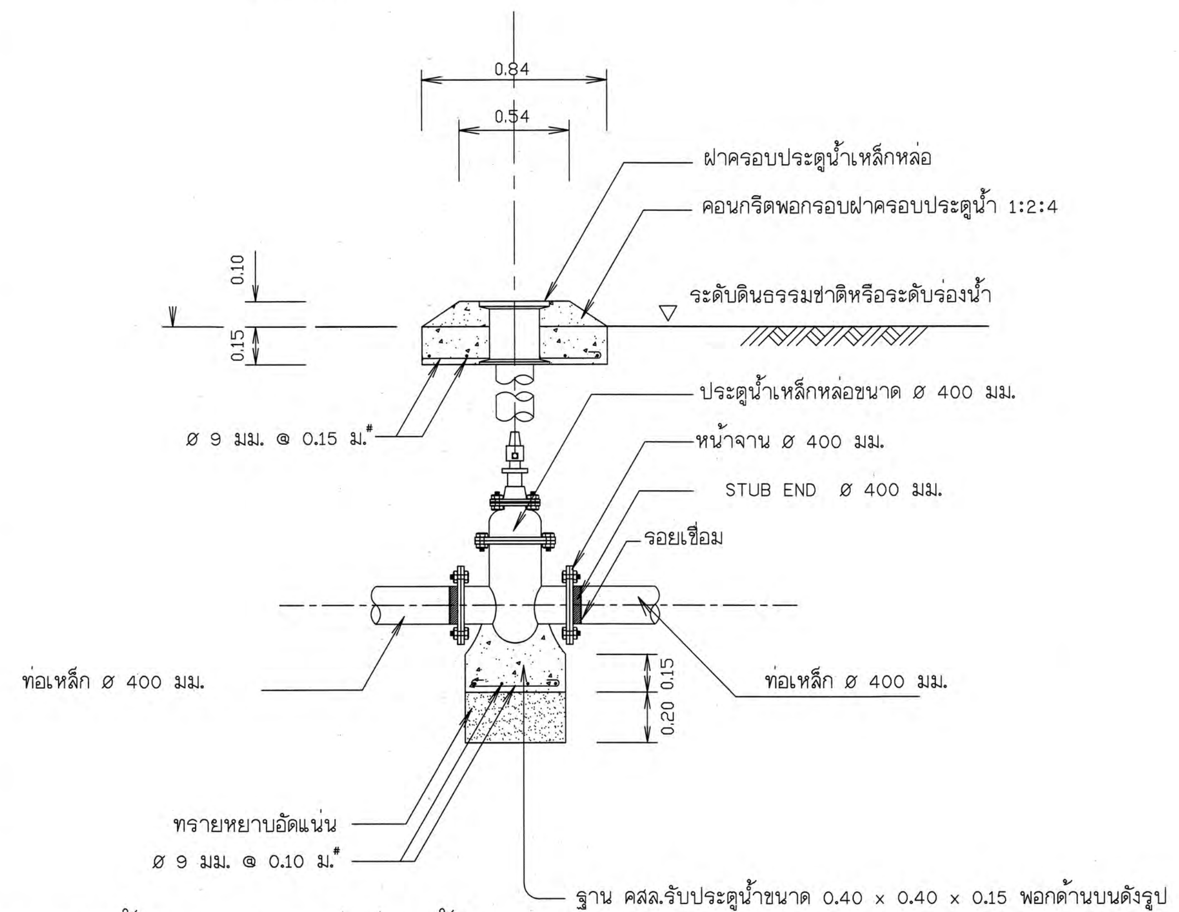
รูปตัด ก - ก แสดงการติดตั้งประตูควบคุมท่อจ่ายน้ำ ขนาด 400 มม.
