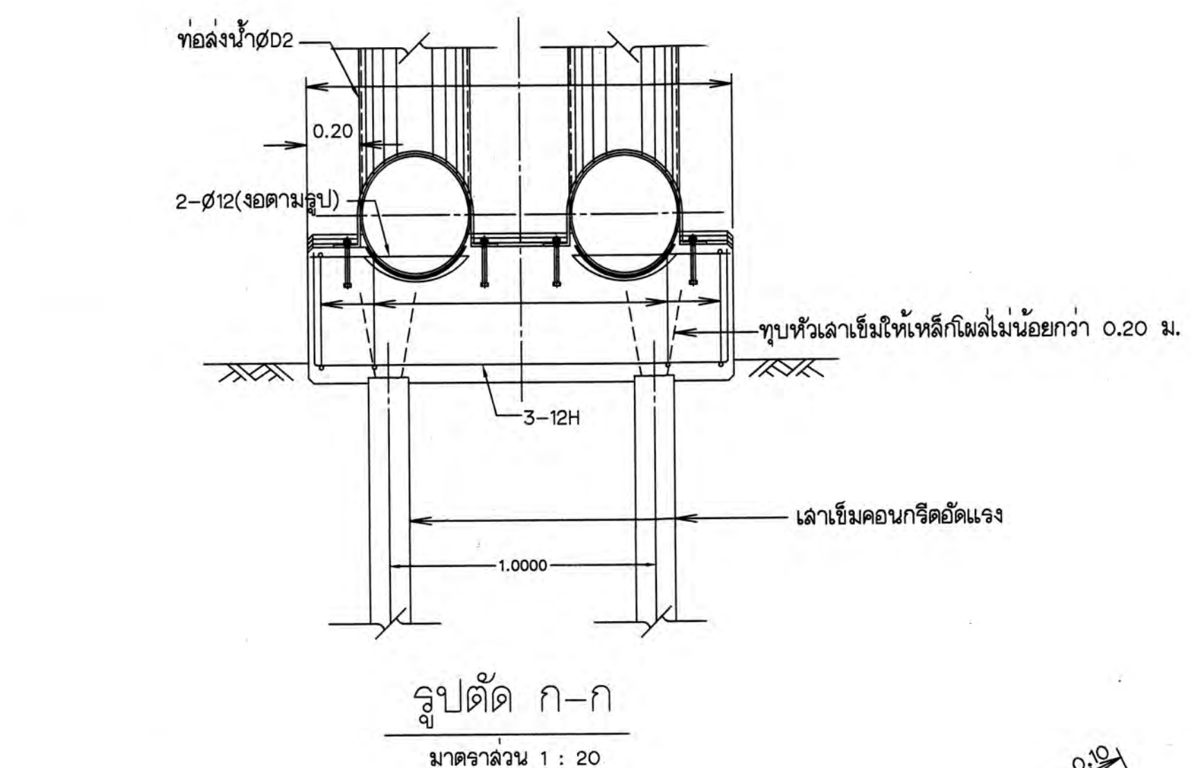
รายละเอียดทอริมตลิ่ง ลาด 1:20
