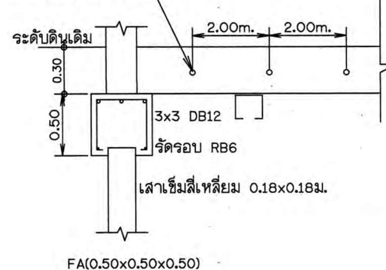
แบบขยายฐานรากรับคานรั้ว (FE)
