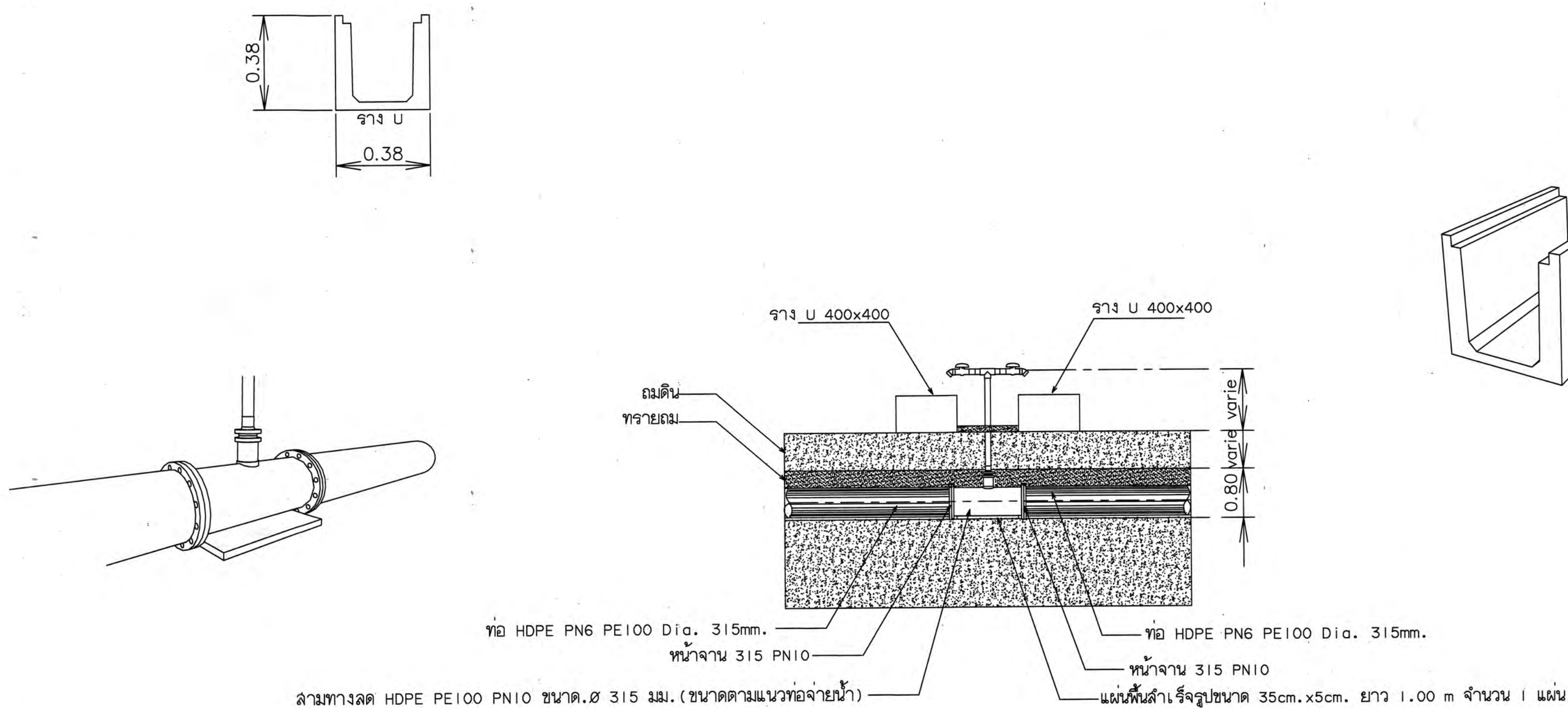
รูปตัด แสดงการติดตั้งจุดกระจายน้ำสำหรับท่อHDPE Dia.315mm.
