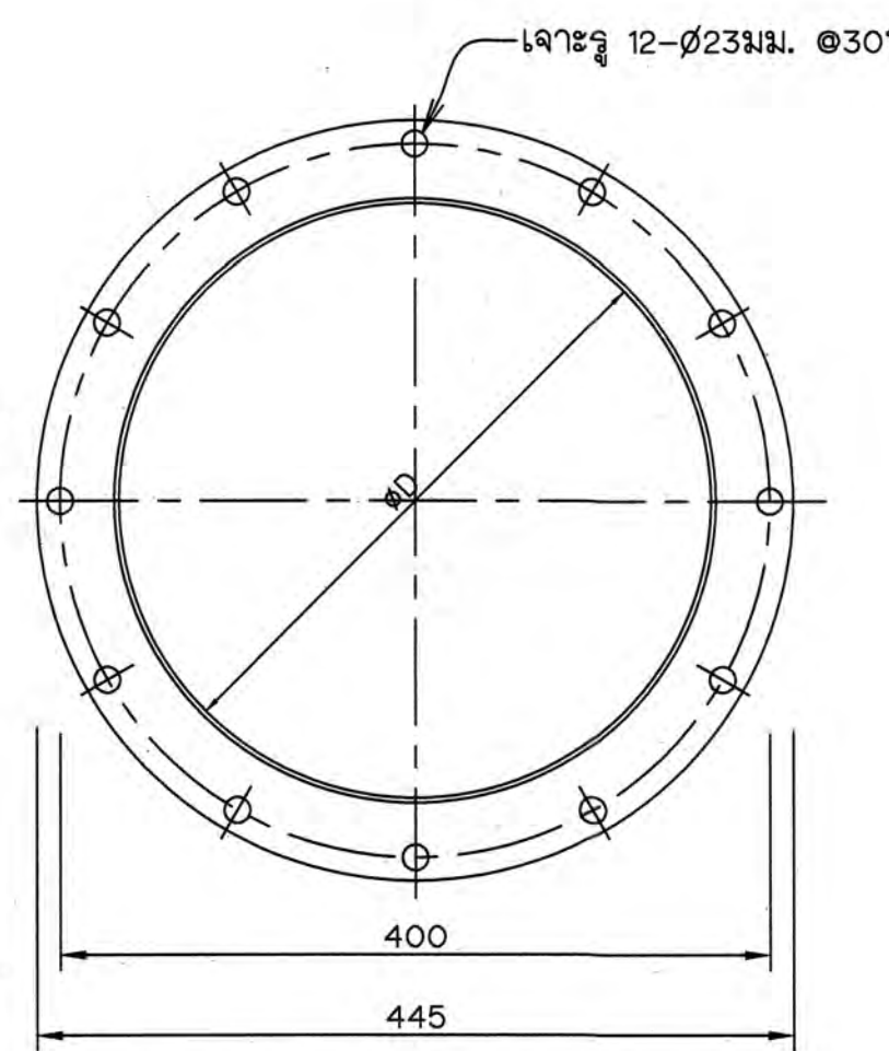
หน้าจานตาดี
