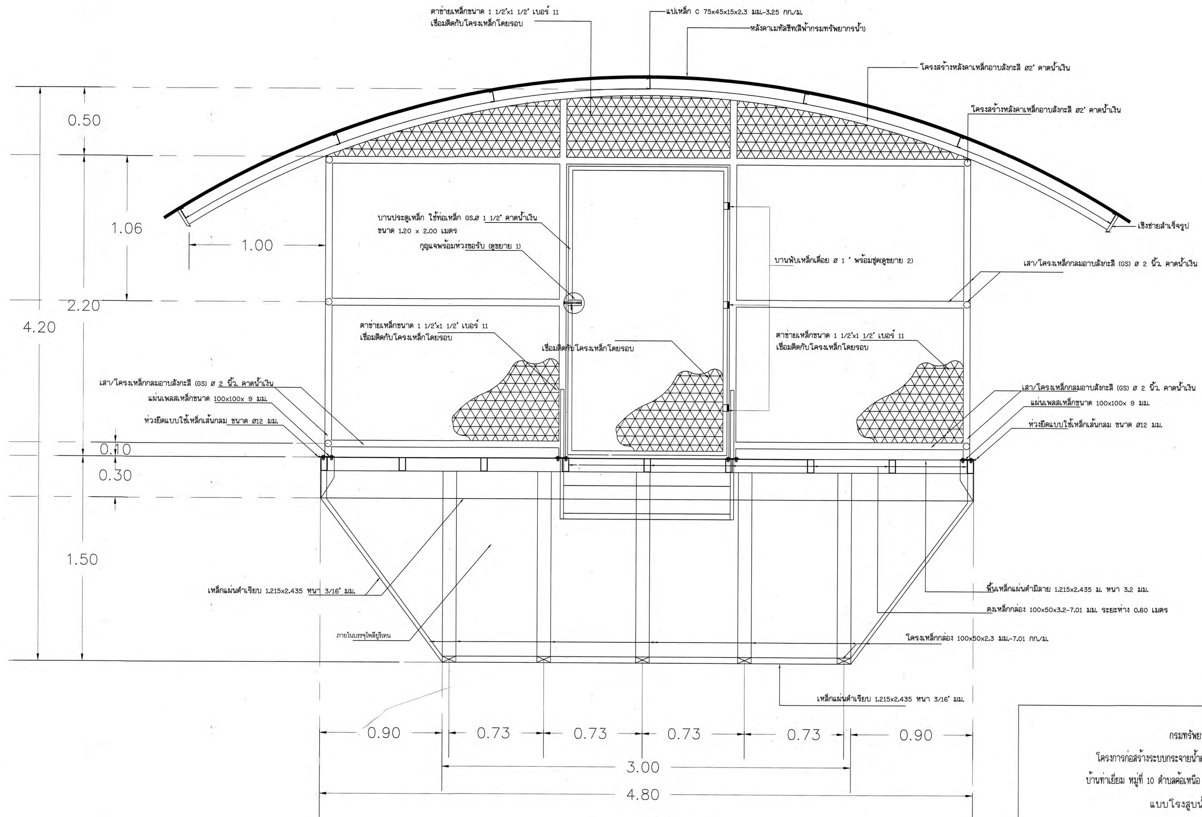
รูปตัด A-A
