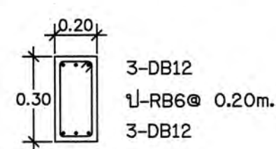
แบบขยายโครงสร้างคานรั้ว (BE)
