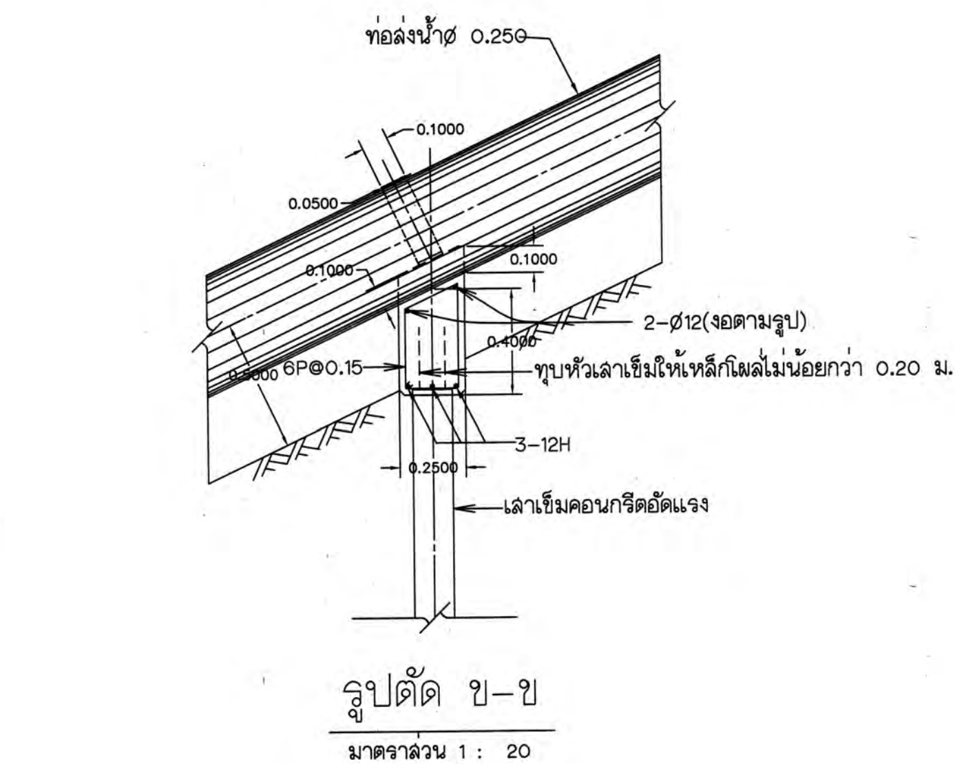
รายละเอียดทอริมตลิ่ง ลาด 1:20
