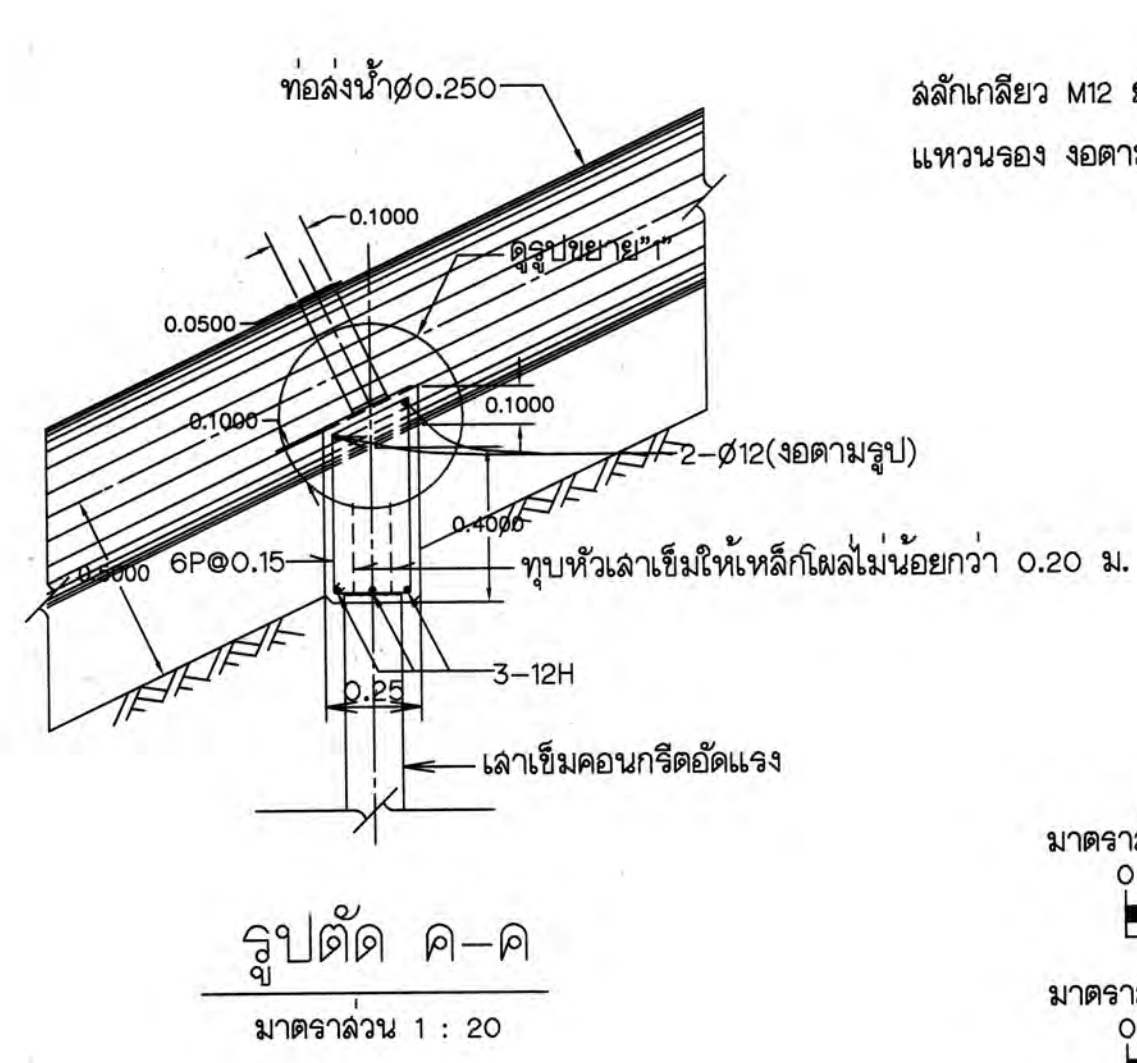
รายละเอียดทอริมตลิ่ง ลาด 1:20
