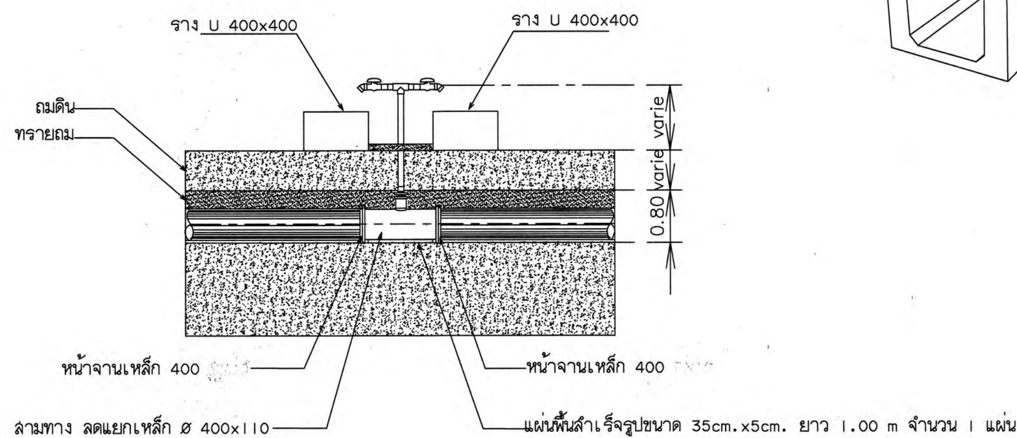
รูปตัด แสดงการติดตั้งจุดกระจายน้ำสำหรับท่อเหล็กขนาด Dia.400mm.
