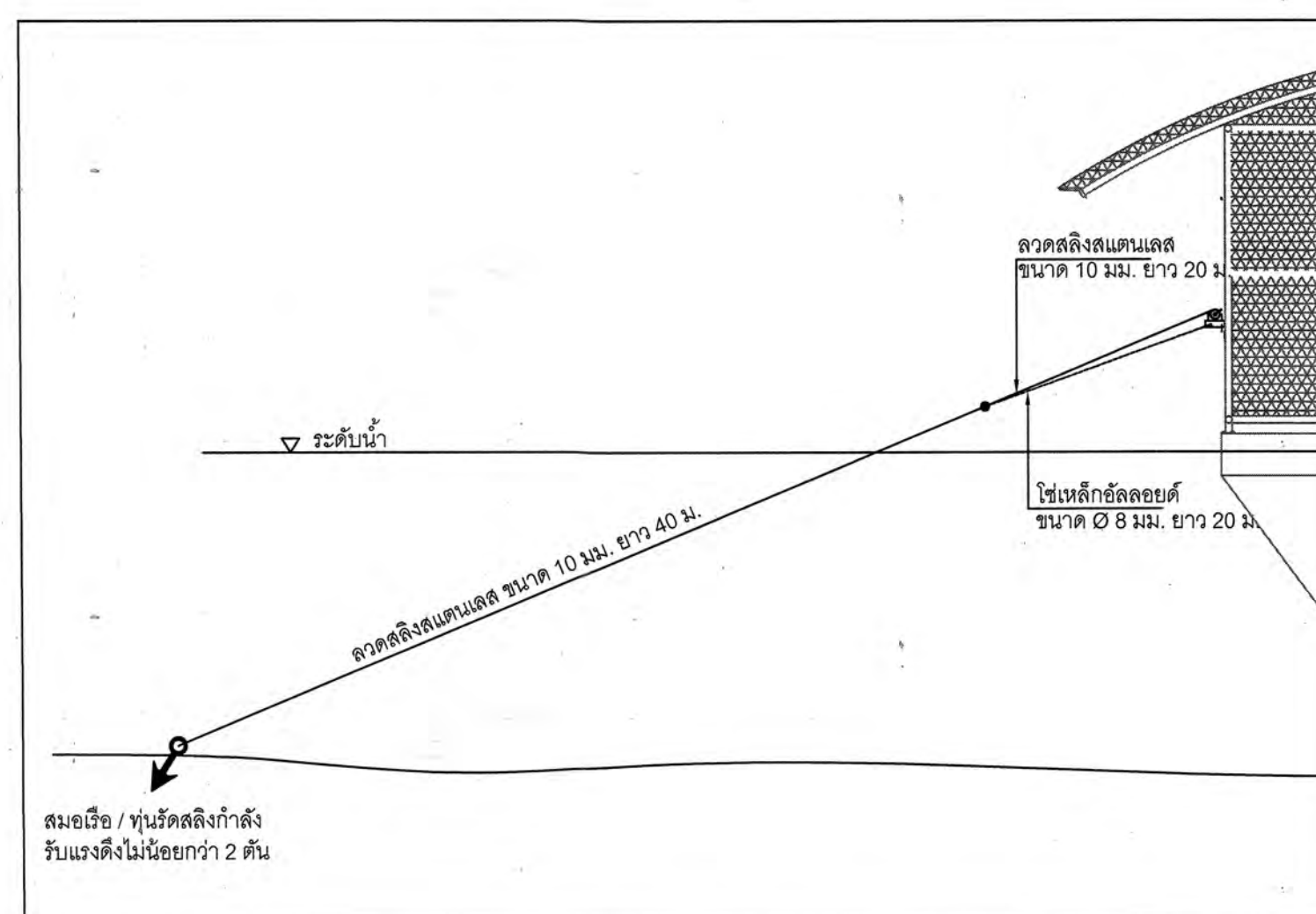
แบบขยายแสดงการยึดแพสพูนน้ำ
