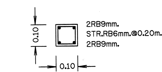
รูปตัด ก - ก
