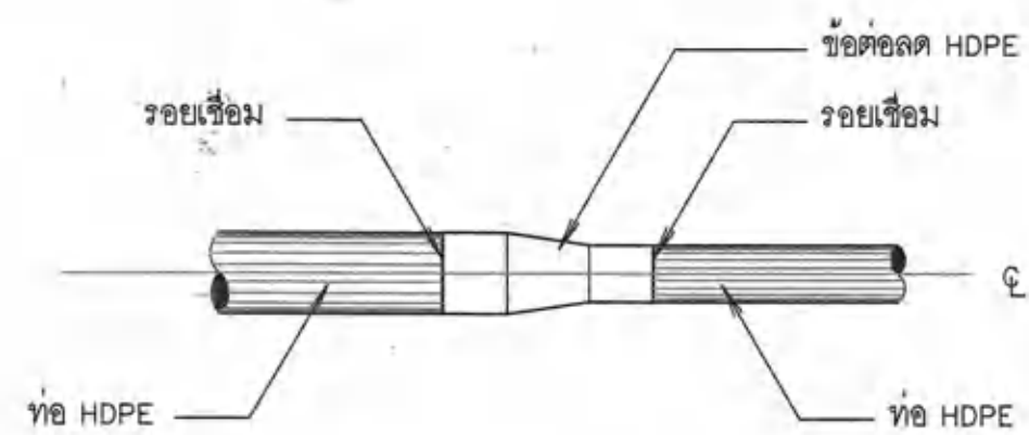
การบรรจุบ่อ HDPE กับข้อต่อท่อ HDPE
