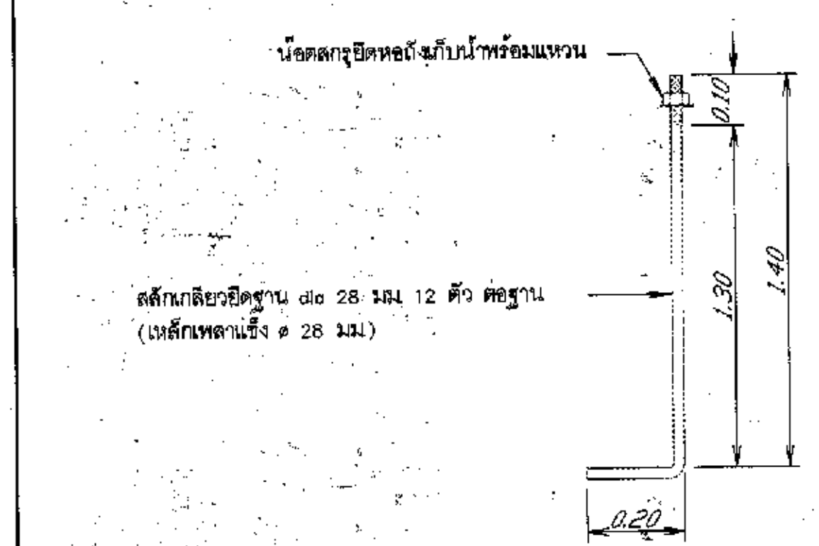
แบบขยายสลักเกลียวยึดฐาน ไม่แสดงมาตราส่วน
