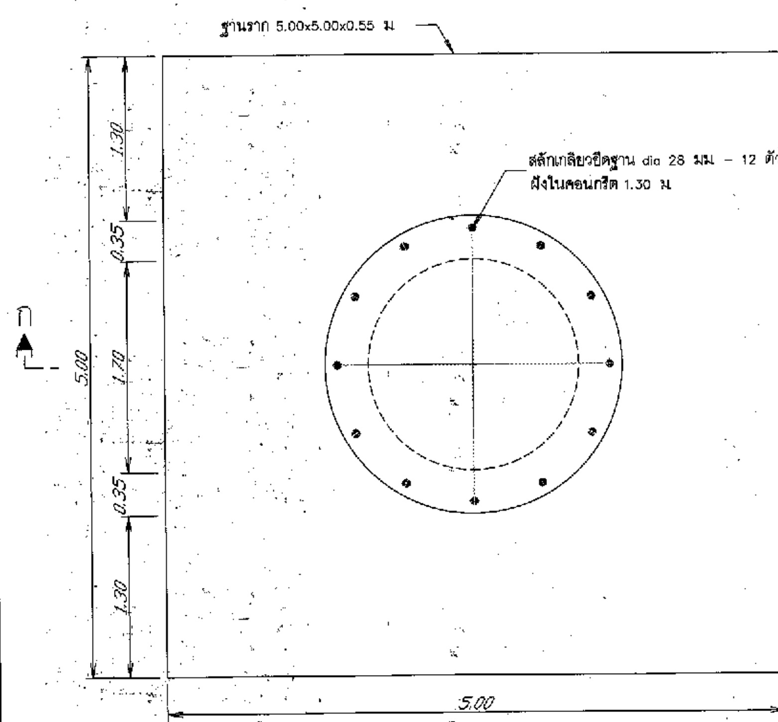
แปลน ฐานรากหอดึงสูง (แบบฐานแผ่) ไม่แสดงมาตราส่วน
