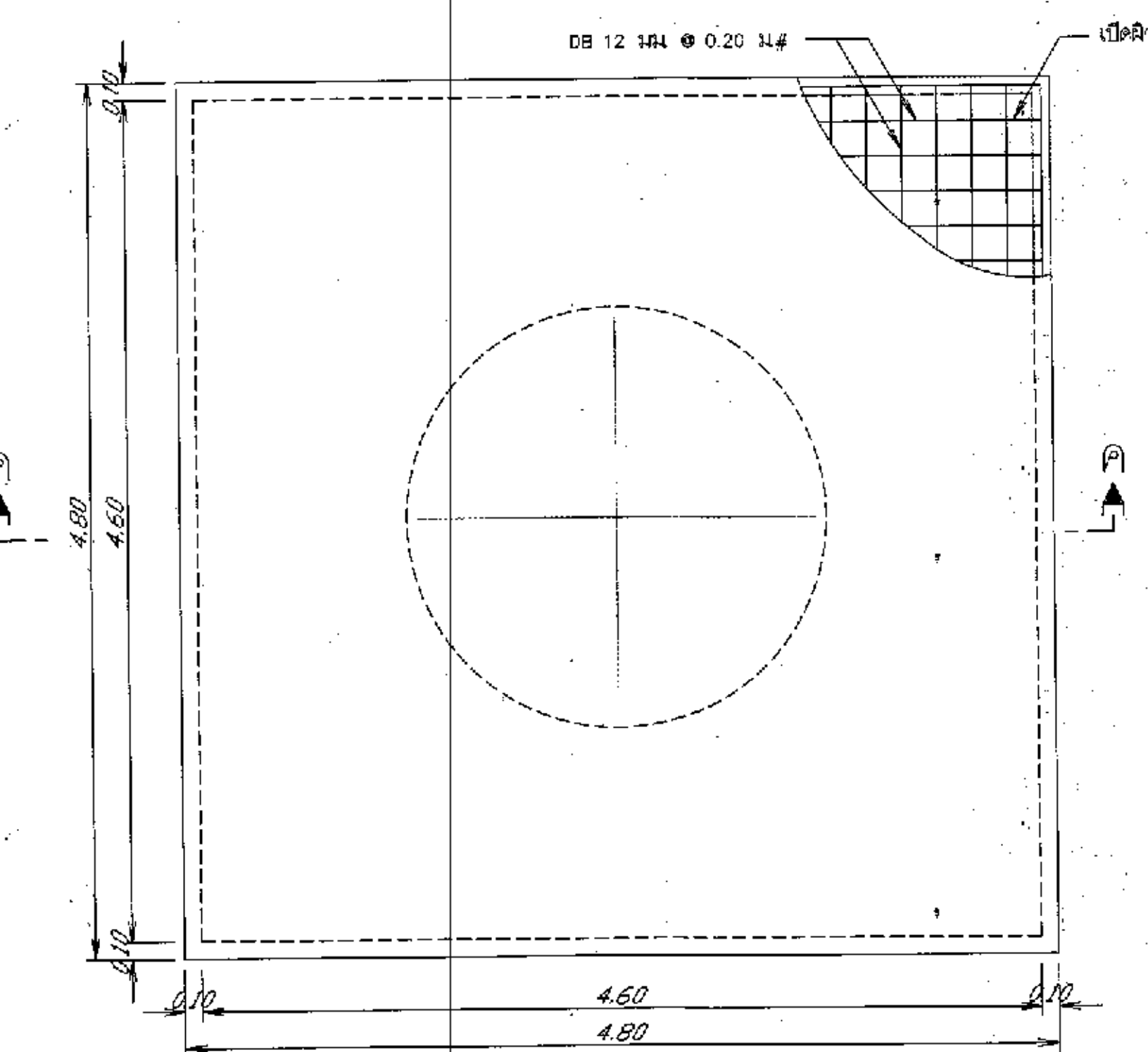
แปลนพื้นคอนกรีตเสริมเหล็ก ไม่แสดงมาตราส่วน
