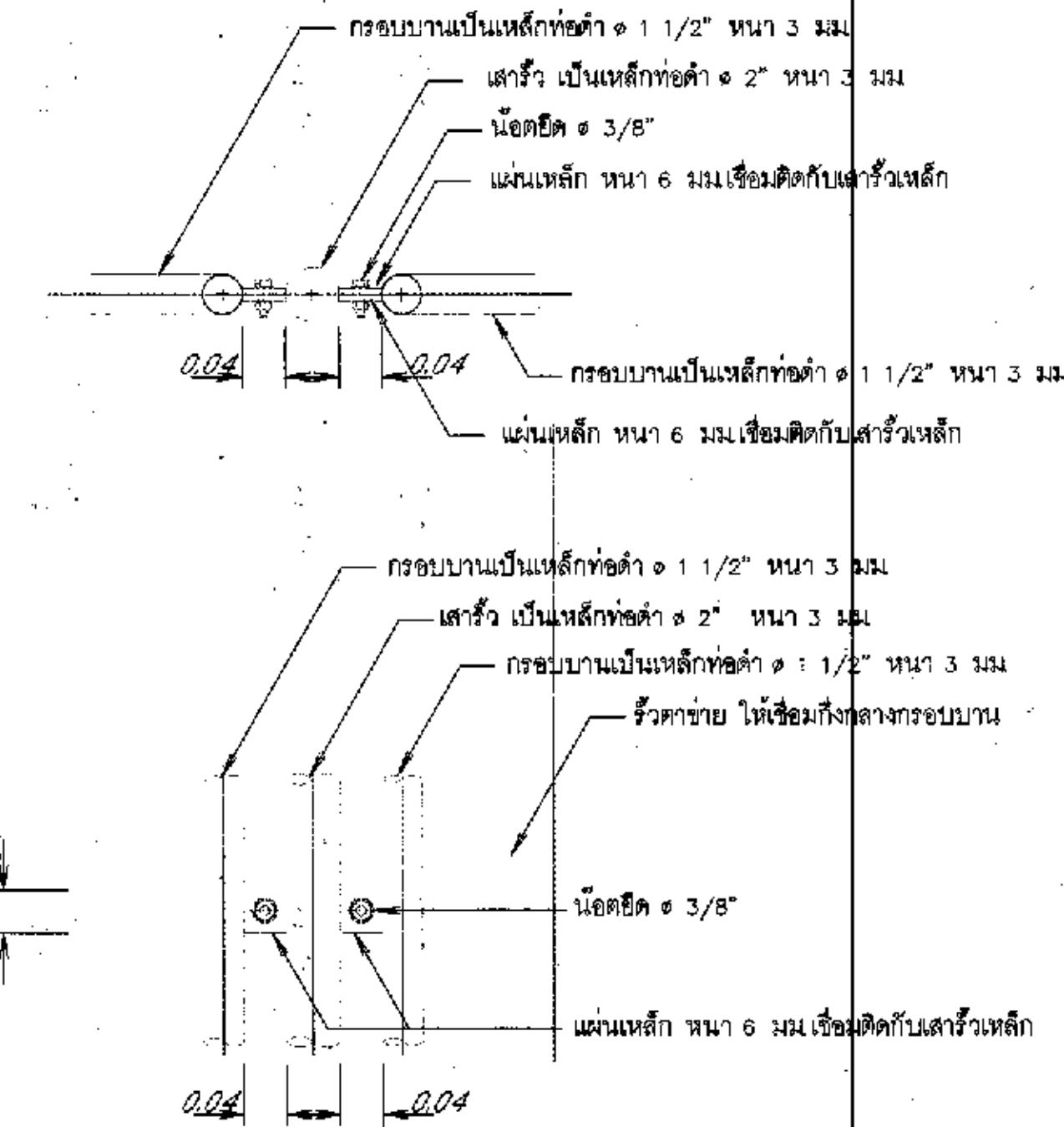
แบบขยายรายละเอียดแสดงการยึดระหว่างรื้อกับเสา ไม่แสดงมาตราส่วน
