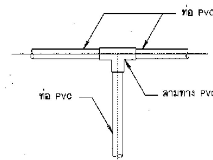
10. แบบการต่อสามทาง PVC ไม่แสดงมาตราส่วน
