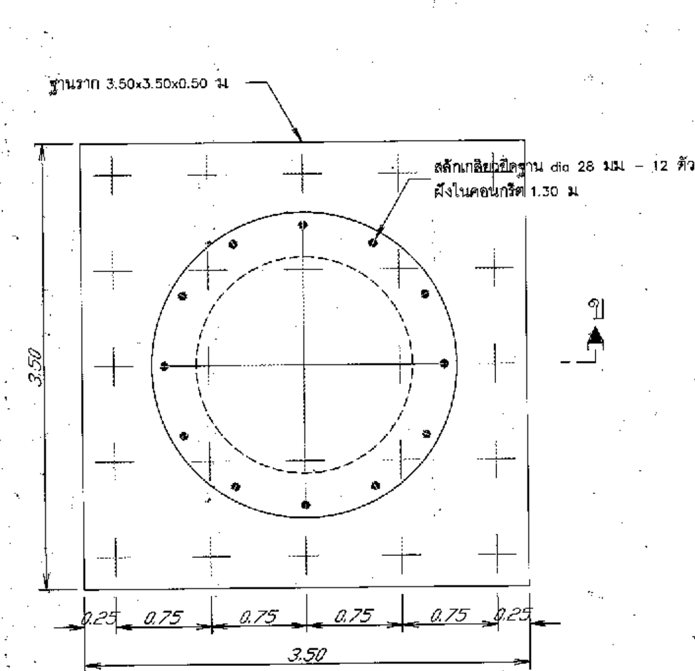
แปลน ฐานรากหอดึงสูง (แบบเสาเข็ม) ไม่แสดงมาตราส่วน
