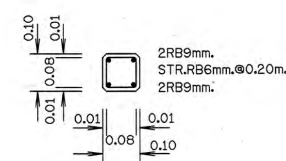
รูปตัด ข - ข
