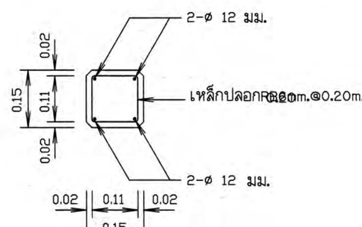
รูปตัด ข - ข
