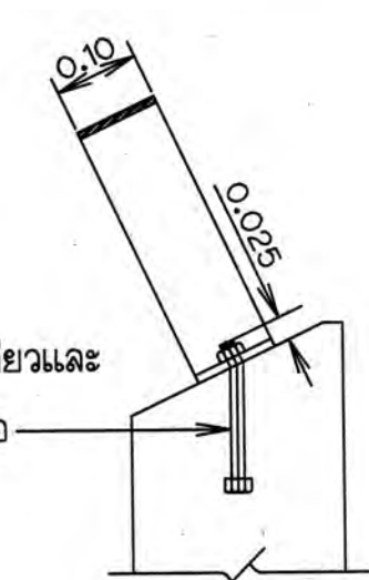
รูปขยาย 1
