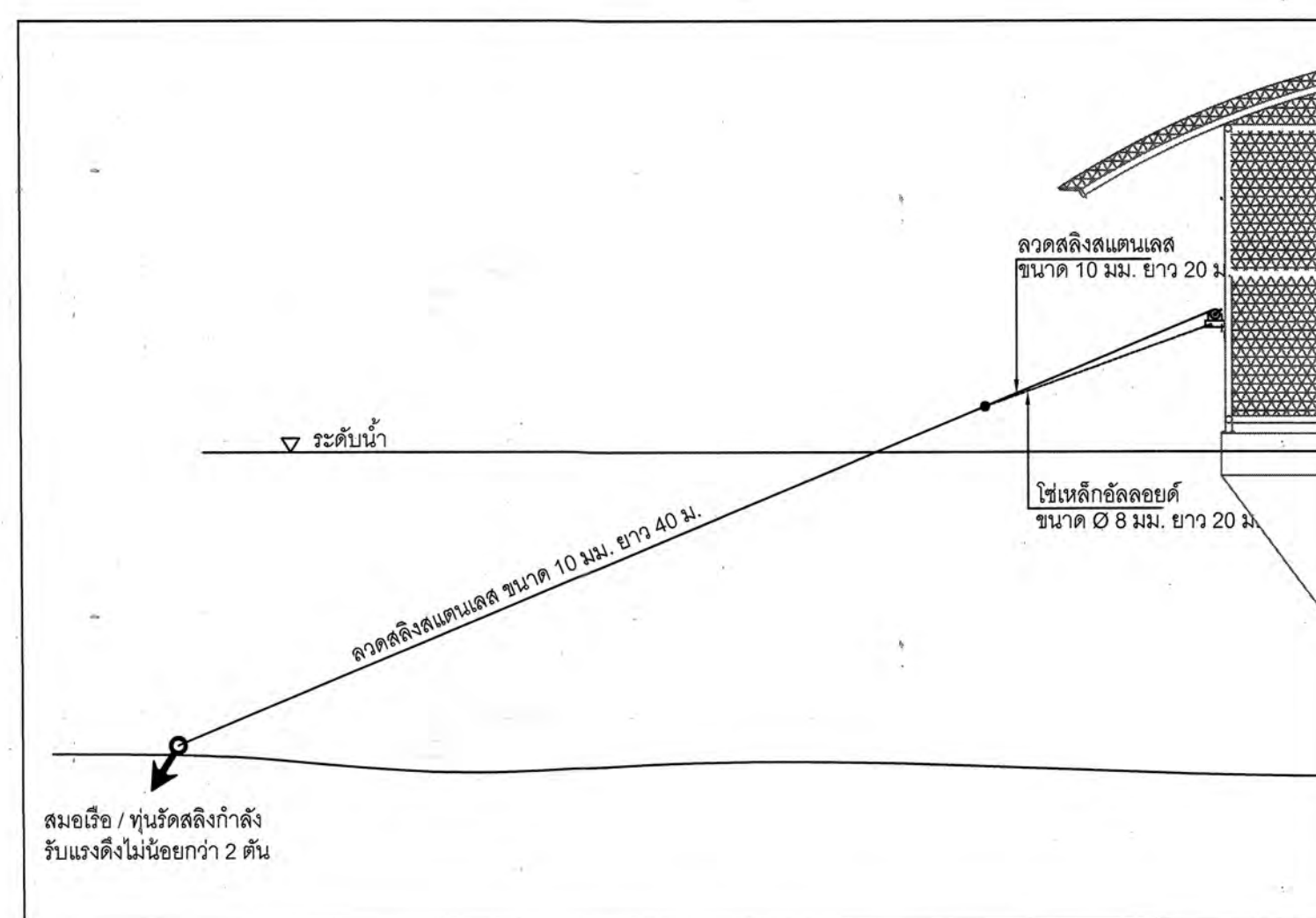
แบบขยายแสดงการยึดแพสสน้ำ
