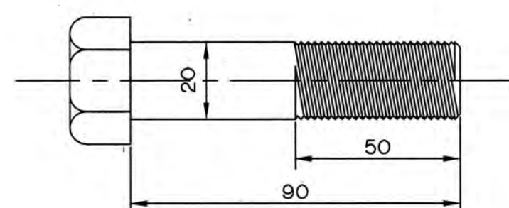
สลักเกลียวขนาด M20 ไม่แสดงมาตราส่วน
