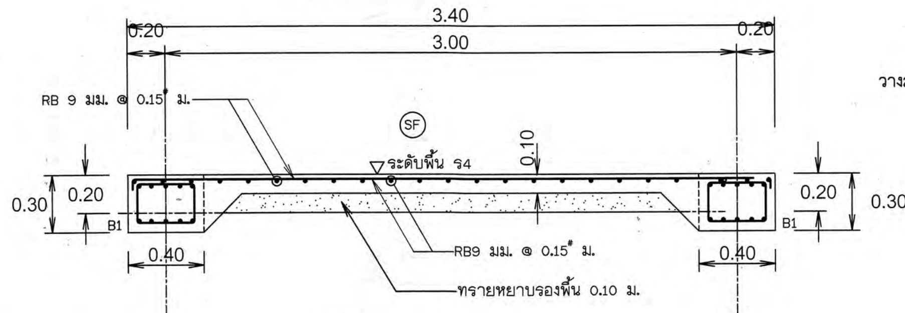
รูปตัด ก1 - ก1
