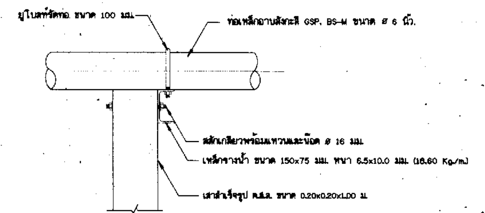
รูคานข้างเสาต่อมอรับท่อ และแบบขยายอุปกรณ์รัดท่อ
