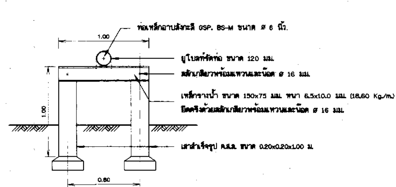
แบบขยายการติดตั้งจุดที่ 2
