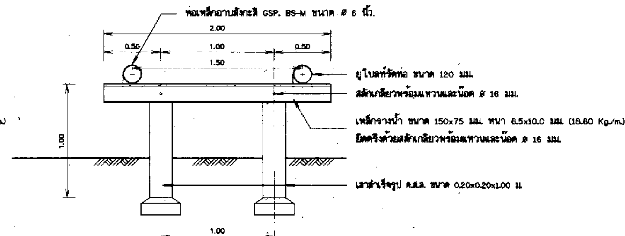
แบบขยายการติดตั้งจุดที่ 3
