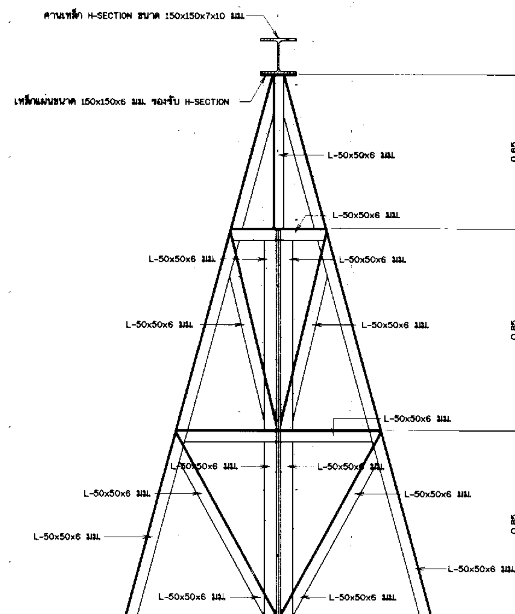
รูปขยายชาตังรูปตัว A รับคานาเหล็ก
