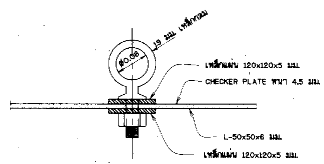
รูปขยายห่วงยึดแปะสูบน้ำ มาตราส่วน 1 : 5
