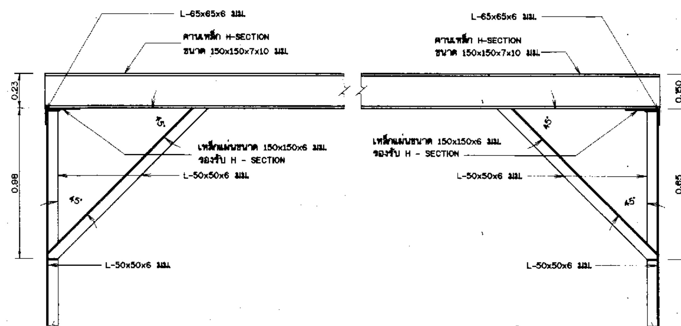
รายละเอียดคานาเหล็กยกเครื่องสูบน้ำ
