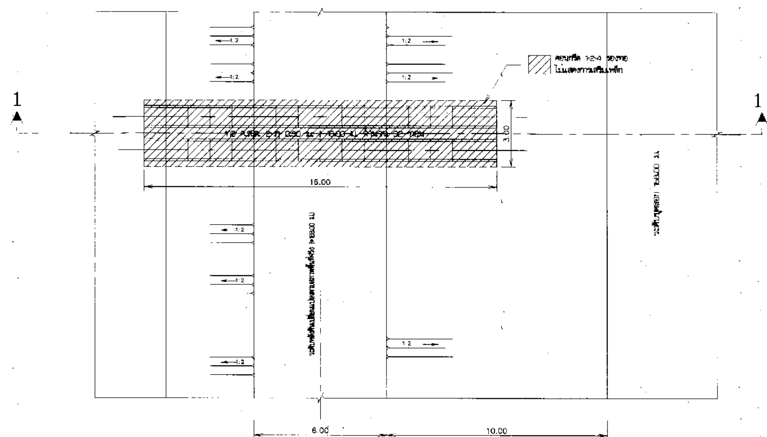
แปลนวางท่อทางน้ำเข้า คสล. ขนาด 2-Ø 0.80 ม. X 16.00 ม. 1:100
