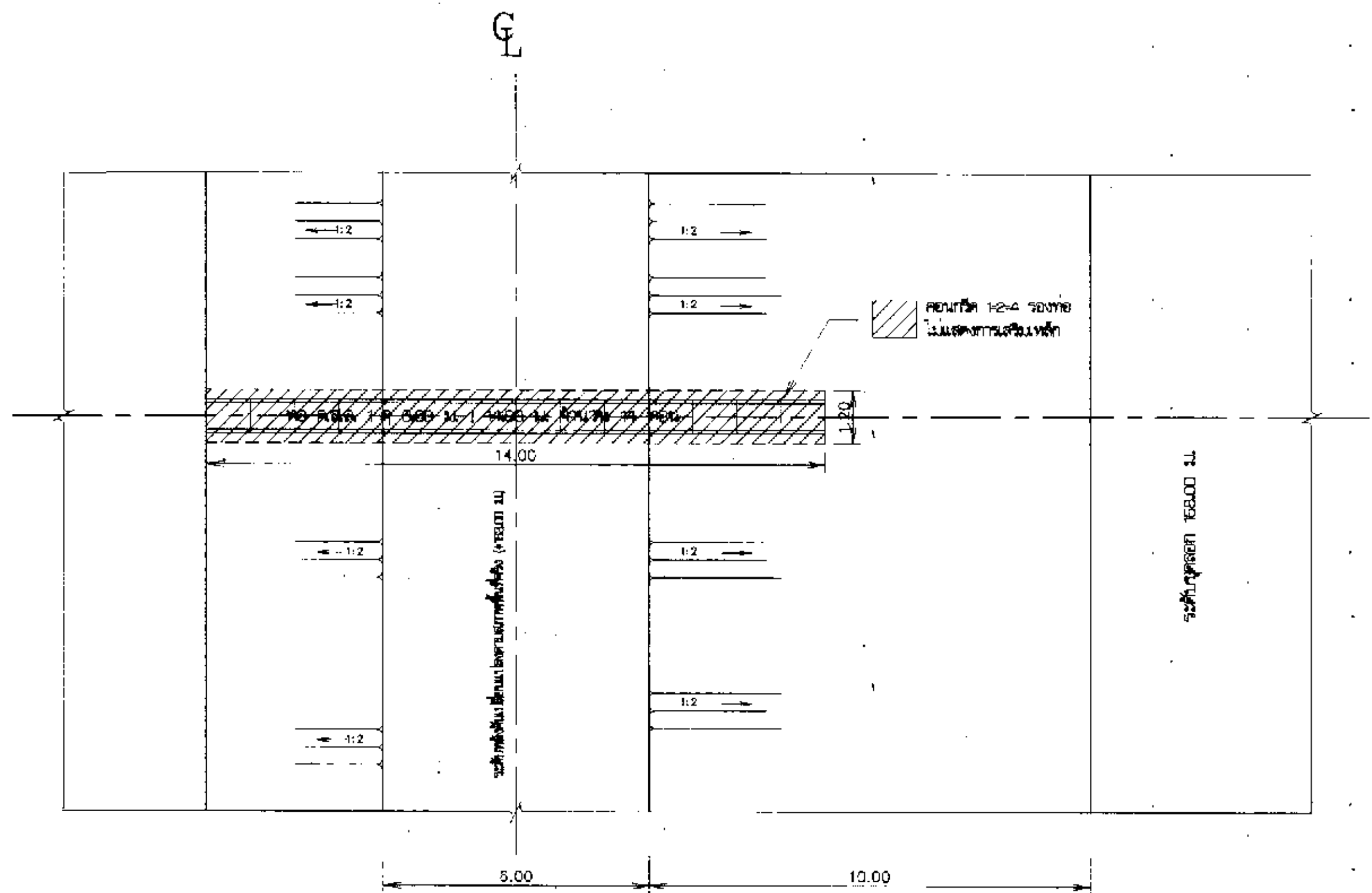
แปลนวางท่อทางน้ำเข้า คสล. ขนาด 1-Ø 0.60 ม. X 14.00 ม. มาตราส่วน 1:100
