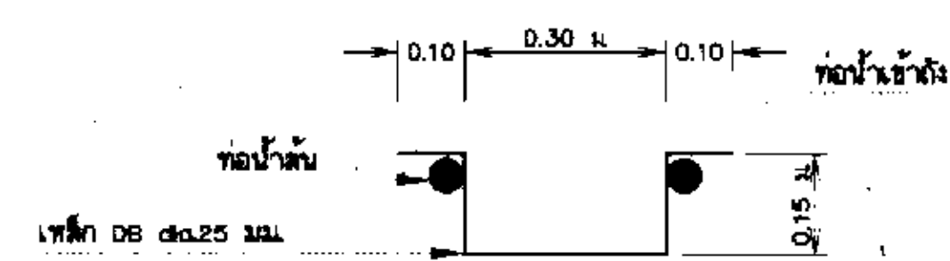
แปลนขยายบ้านโต
