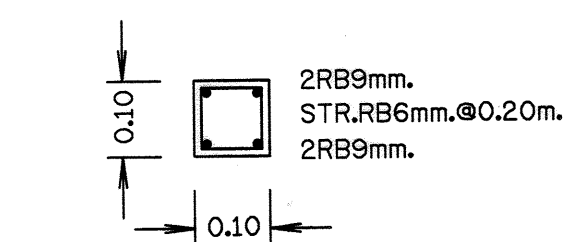
รูปตัด ก - ก
