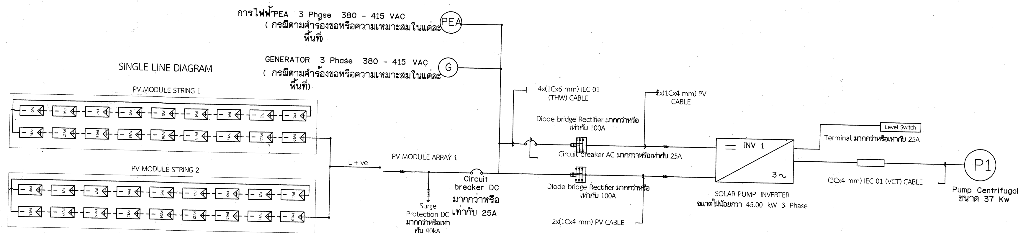
แผนผังระบบไฟฟ้า และไดอะแกรมไฟฟ้า ระบบกระจายน้ำด้วยพลังงานแสงอาทิตย์
