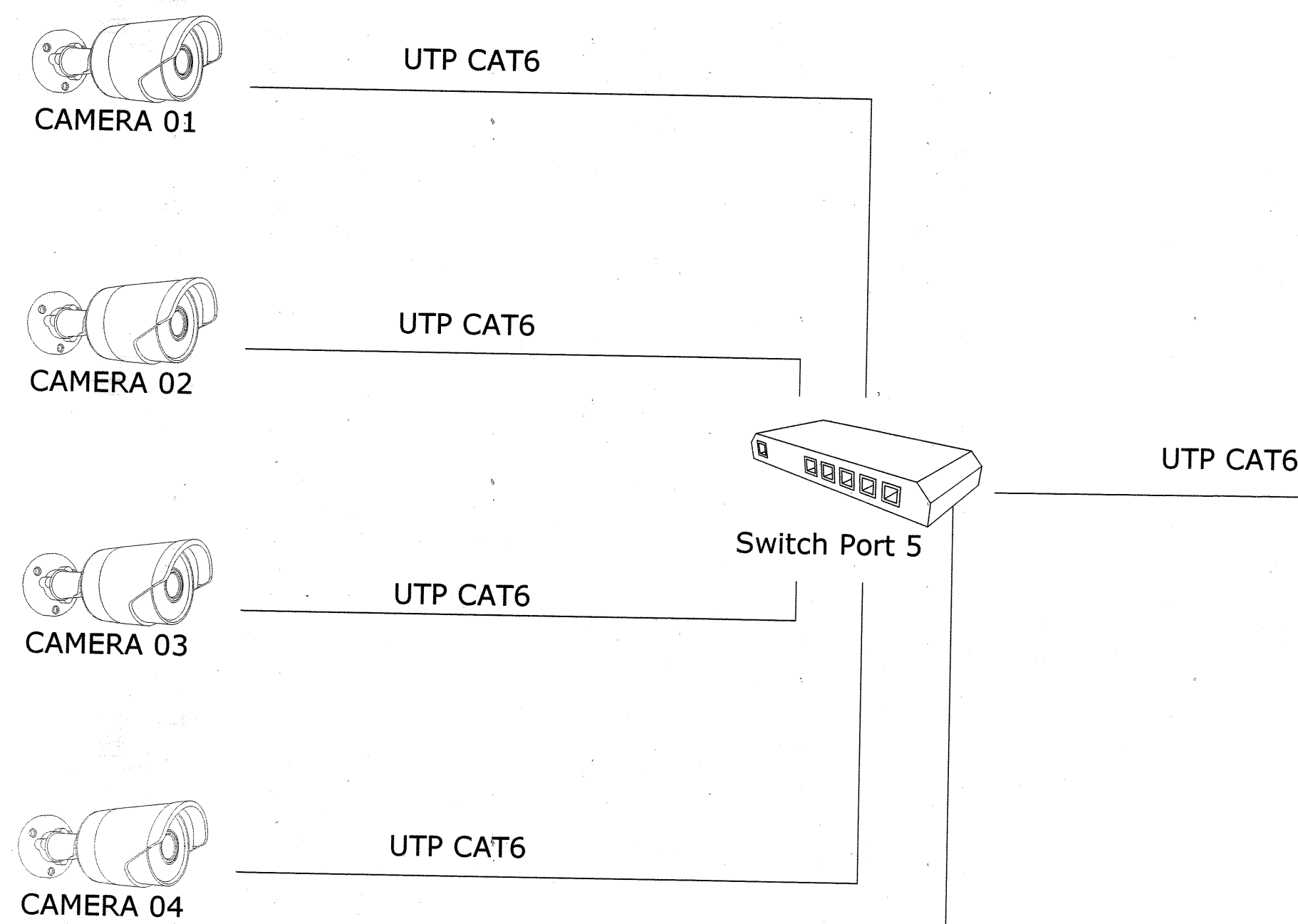
แผนภาพแสดงการติดตั้งกล้องวงจรปิดในบริเวณโครงการ
