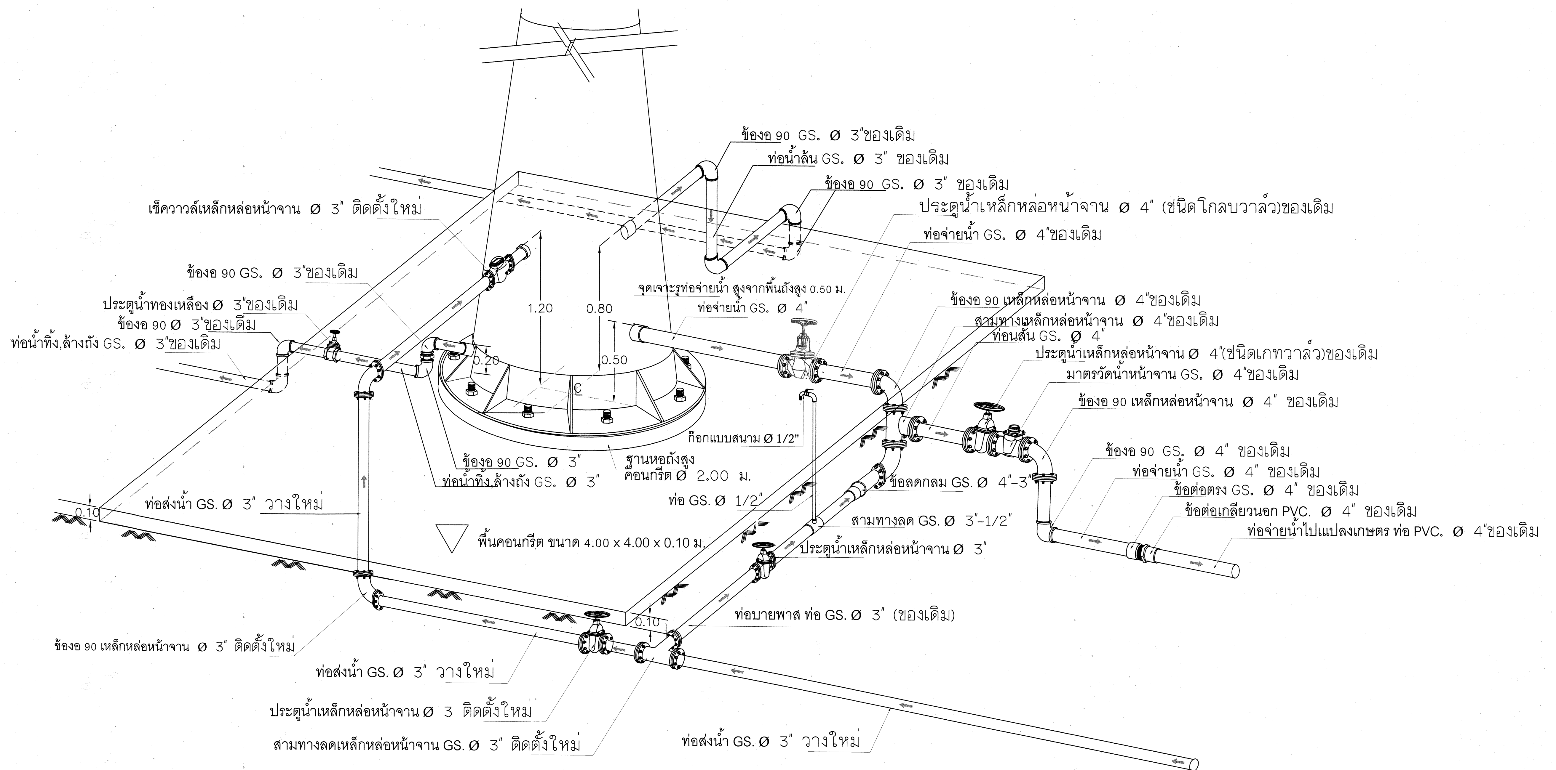
ขยายการประสานท่อระหว่างระบบ ระบบกระจายน้ำพลังงานแสงอาทิตย์ขนาด 4 กิโลวัตต์ Scale 1:30
