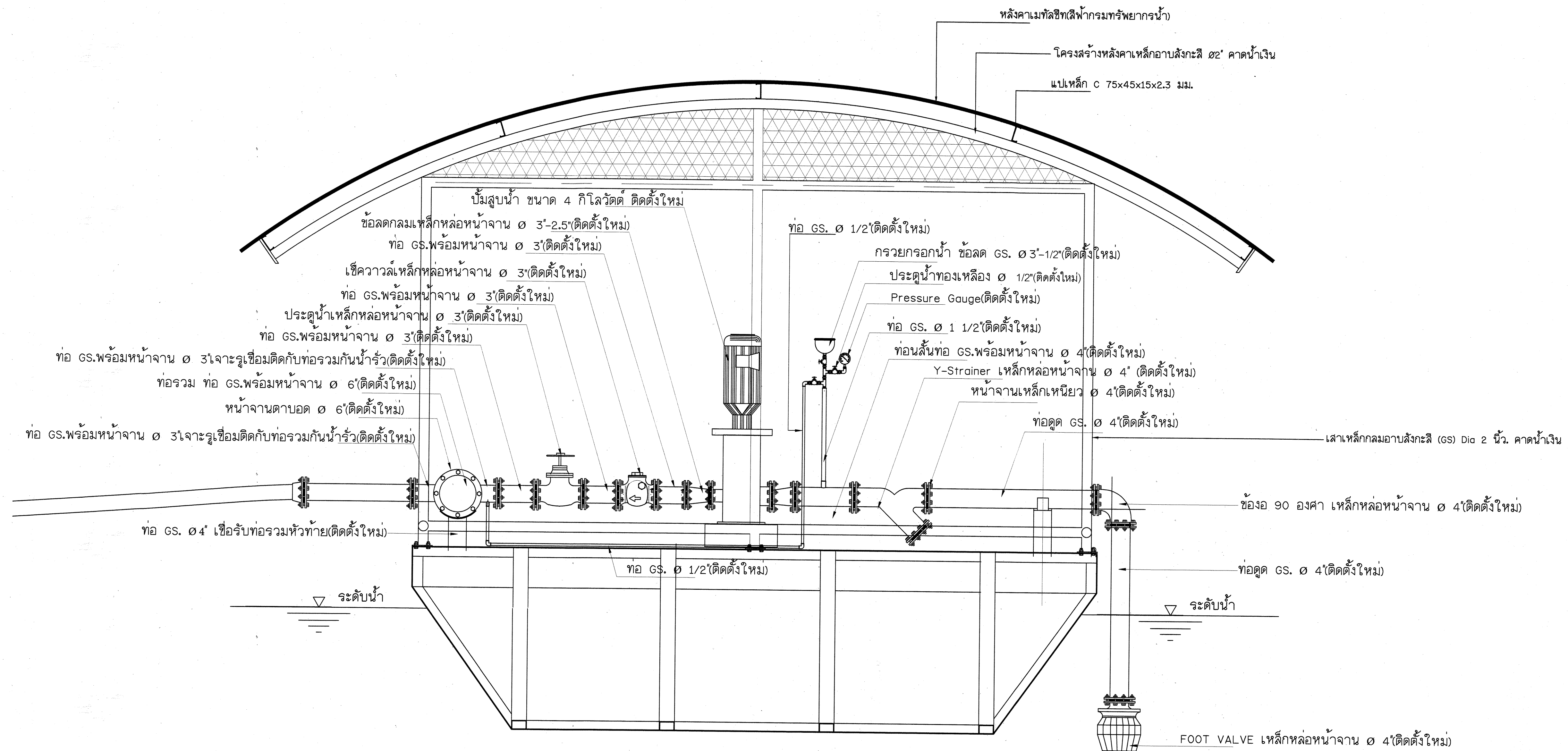
รูปตัด A-A ไม่แสดงขนาดบางส่วน
