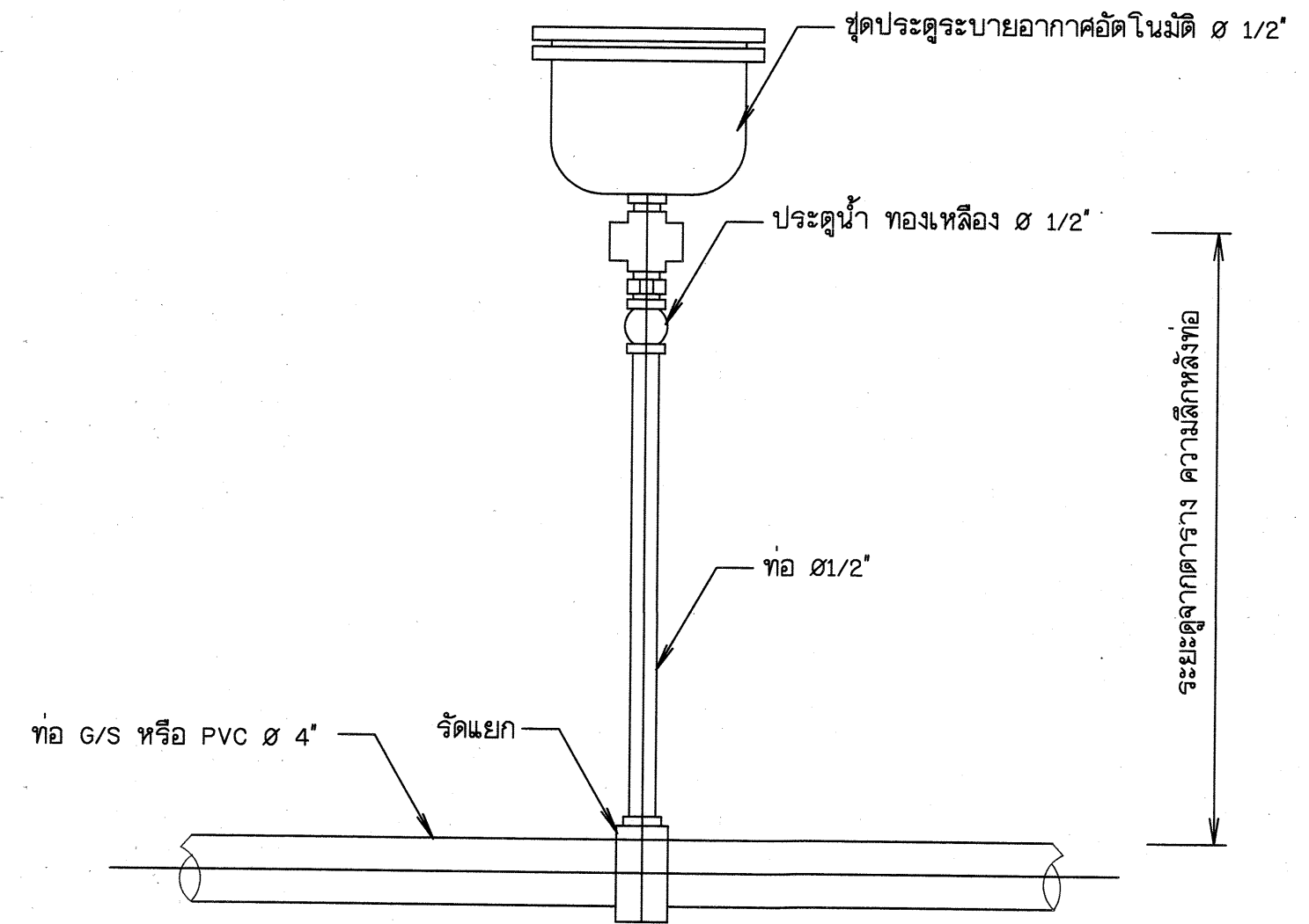
12. การติดตั้งประตูระบายอากาศอัตโนมัติ ไม่แสดงมาตราส่วน
