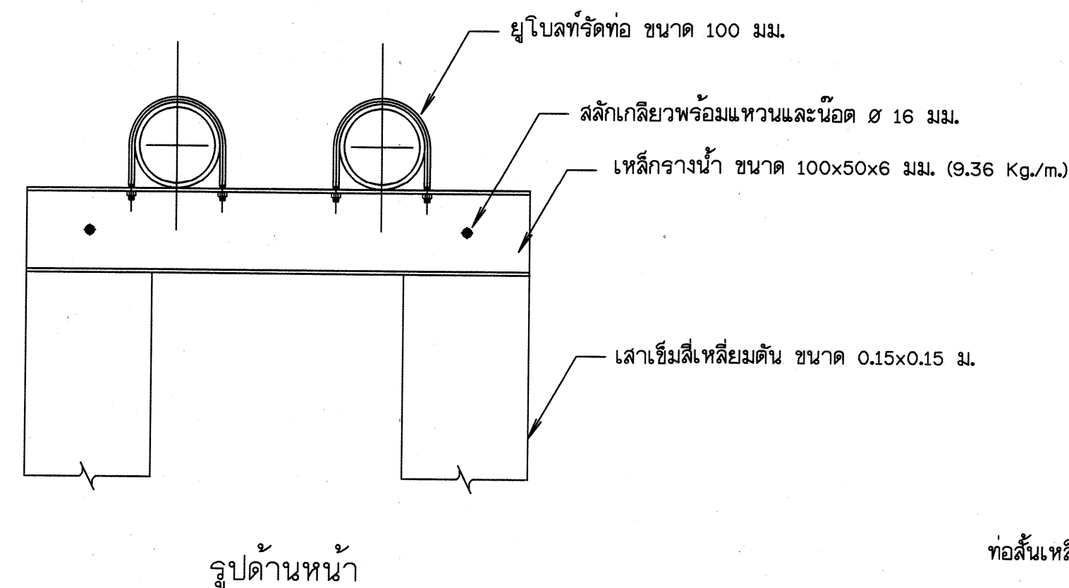
13. เสาค้ำจุนรับท่อวัด และแบบขยายอุปกรณ์วัดท่อ ไม่แสดงมาตราส่วน
