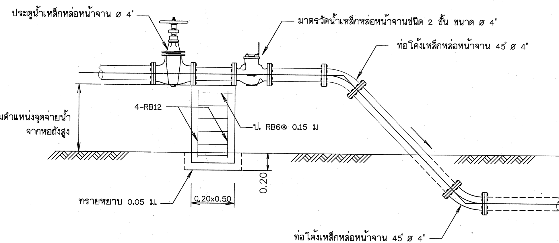
14. การติดตั้งมาตรวัดน้ำบนพื้นดิน 4" ไม่แสดงมาตราส่วน
