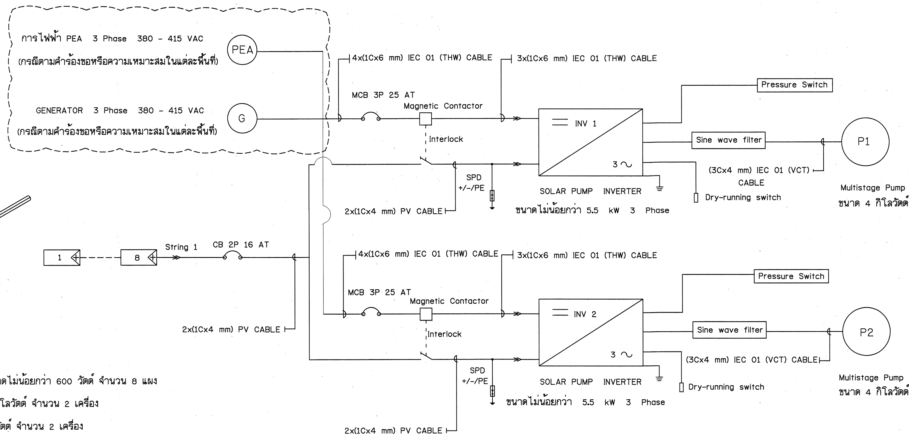
แผนผังระบบไฟฟ้า และไดอะแกรมไฟฟ้า ระบบกระจายน้ำด้วยพลังงานแสงอาทิตย์ ขนาด 4 กิโลวัตต์
