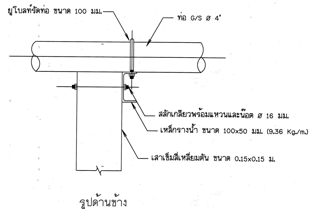
13. เสาค้ำจุนรับท่อวัด และแบบขยายอุปกรณ์วัดท่อ ไม่แสดงมาตราส่วน
