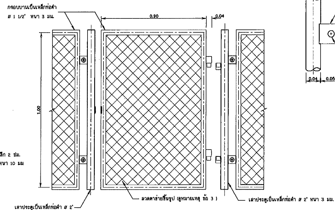
แบบขยายสายผู้น ไม่แสดงมาตราส่วน
