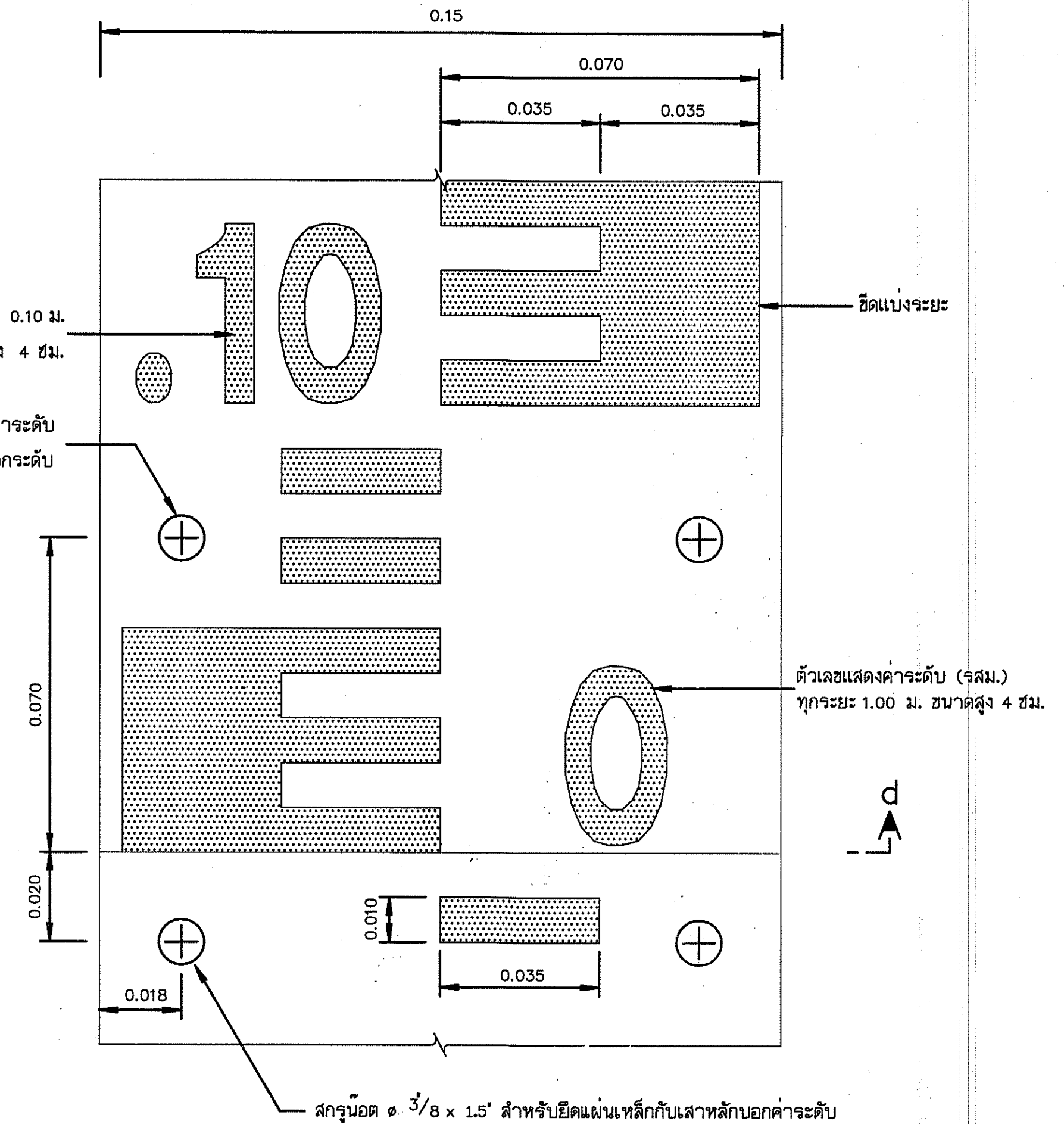
ขยายแผ่นหลักบอกระดับ
