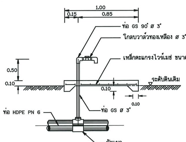
แปลนจุดปล่อยน้ำ มาตราส่วน No Scale
