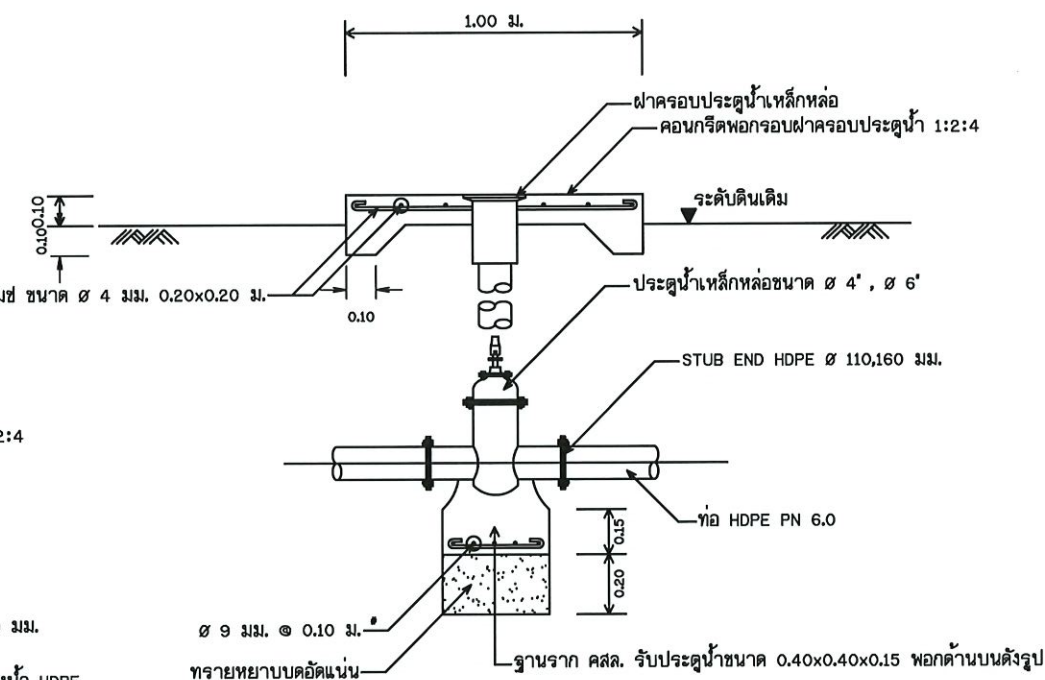
แปลนจุดปล่อยน้ำ มาตราส่วน No Scale
