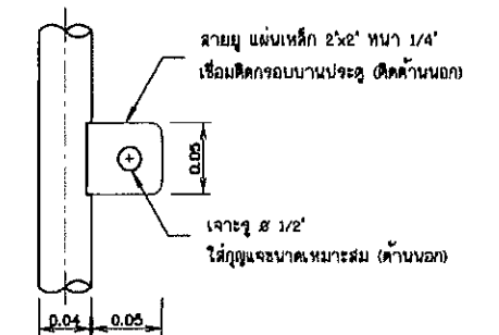
แบบขยายสายผู้น ไม่แสดงมาตราส่วน
