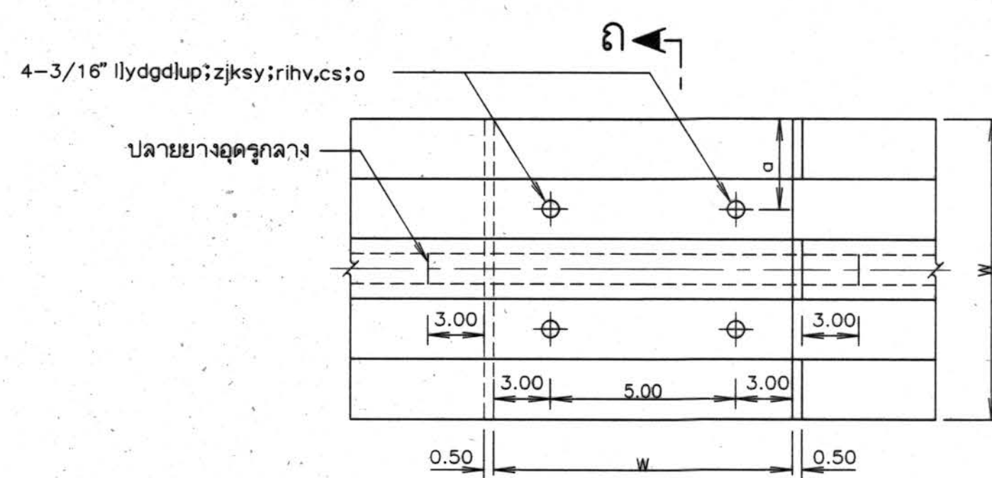
การต่อตรง ไม่แสดงมาตราส่วน
