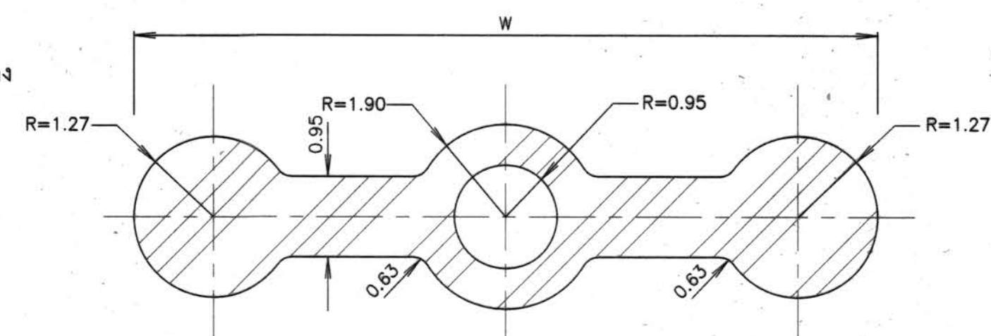
TYPE "A" ไม่แสดงมาตราส่วน
