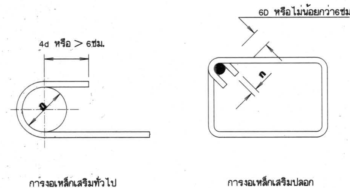
แสดงการดัดงอเหล็กเสริม มาตราส่วน 1:20
