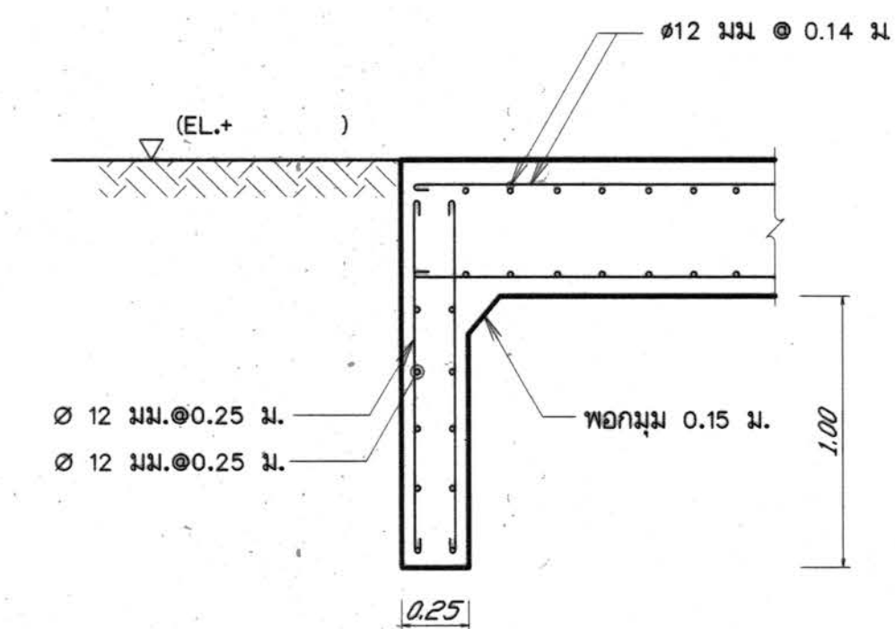
แบบขยาย 1-1 มาตราส่วน 1:25
