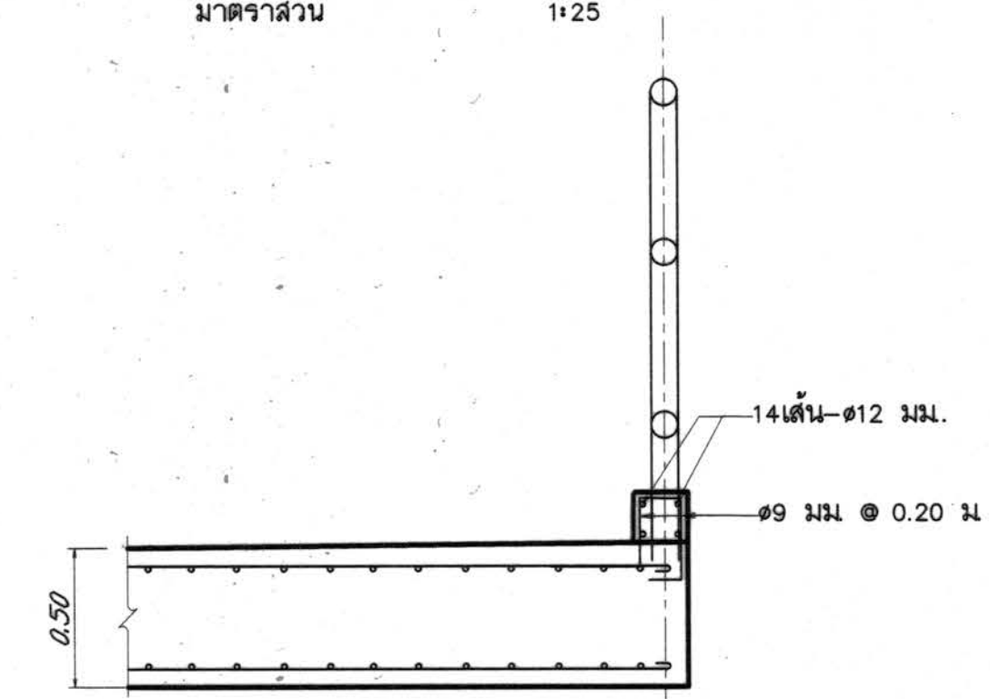
แบบขยาย 1-2 มาตราส่วน 1:25
