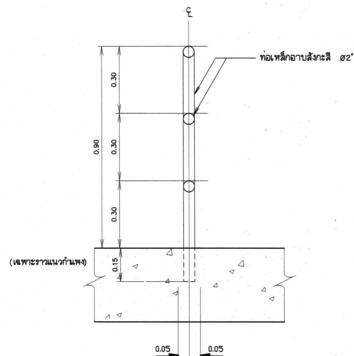
รูปตัด D - D มาตราส่วน 1:10
