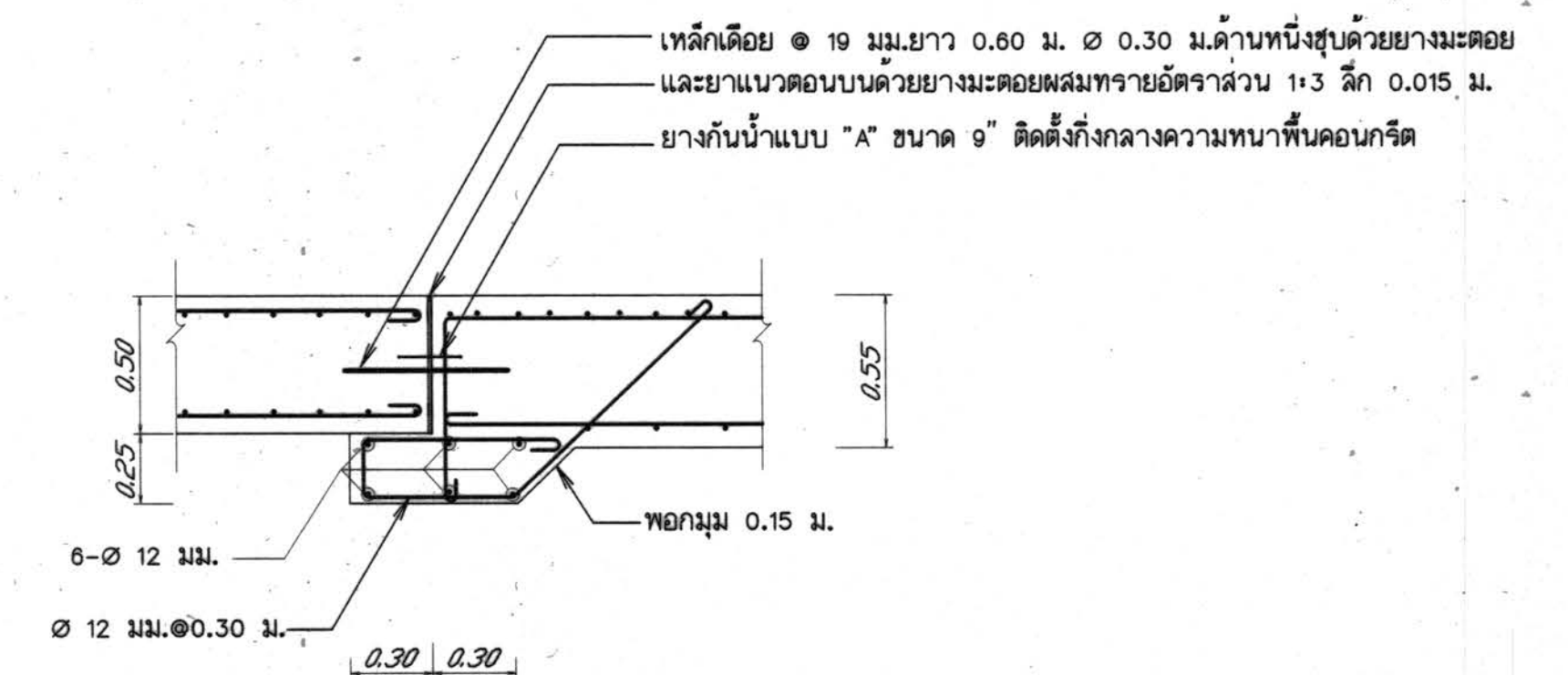
แบบขยาย 1-3 มาตราส่วน 1:25
