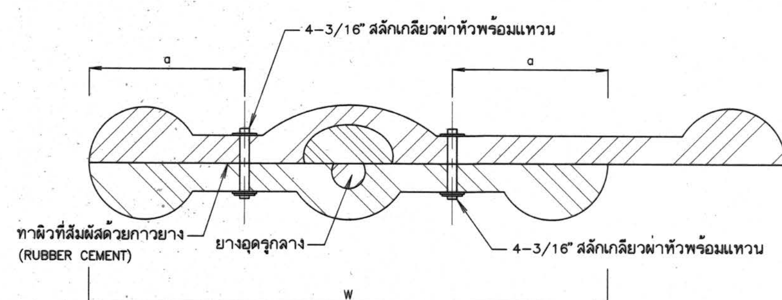
รูปตัด ท-ท ไม่แสดงมาตราส่วน
