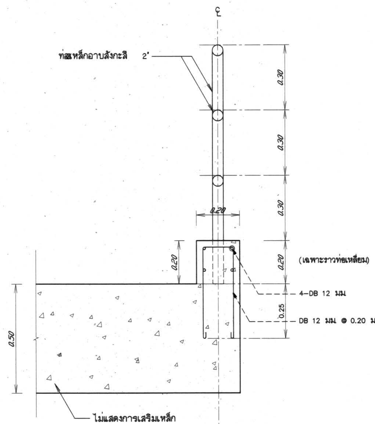
รูปขยาย CURB มาตราส่วน 1:10
