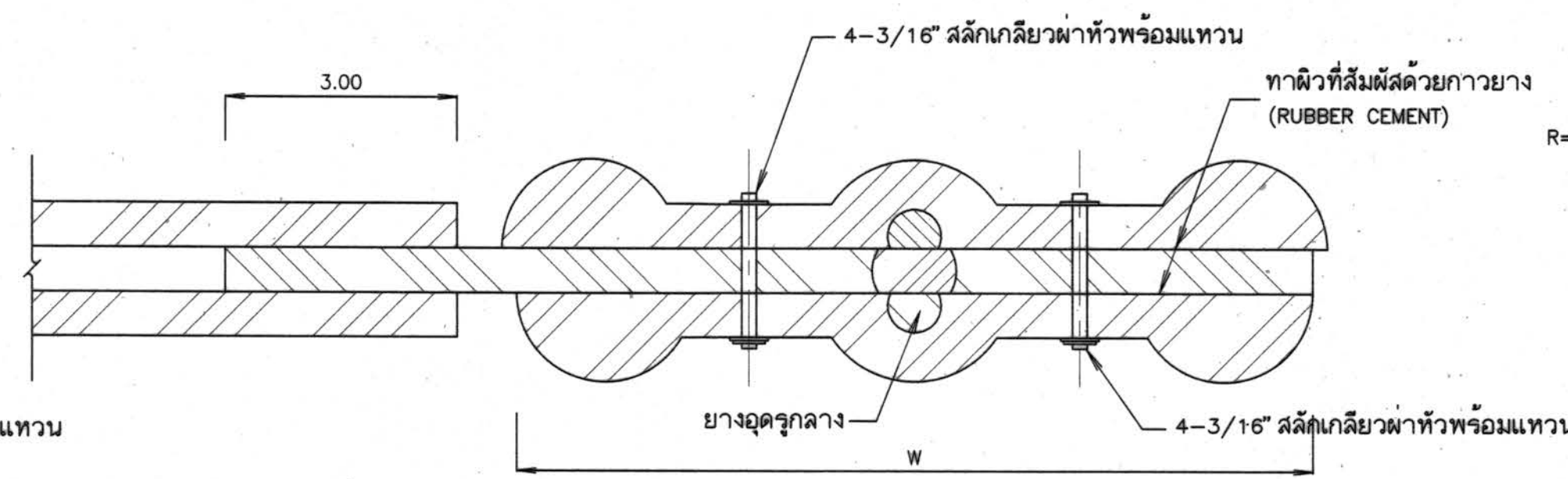
รูปตัด น-น ไม่แสดงมาตราส่วน
