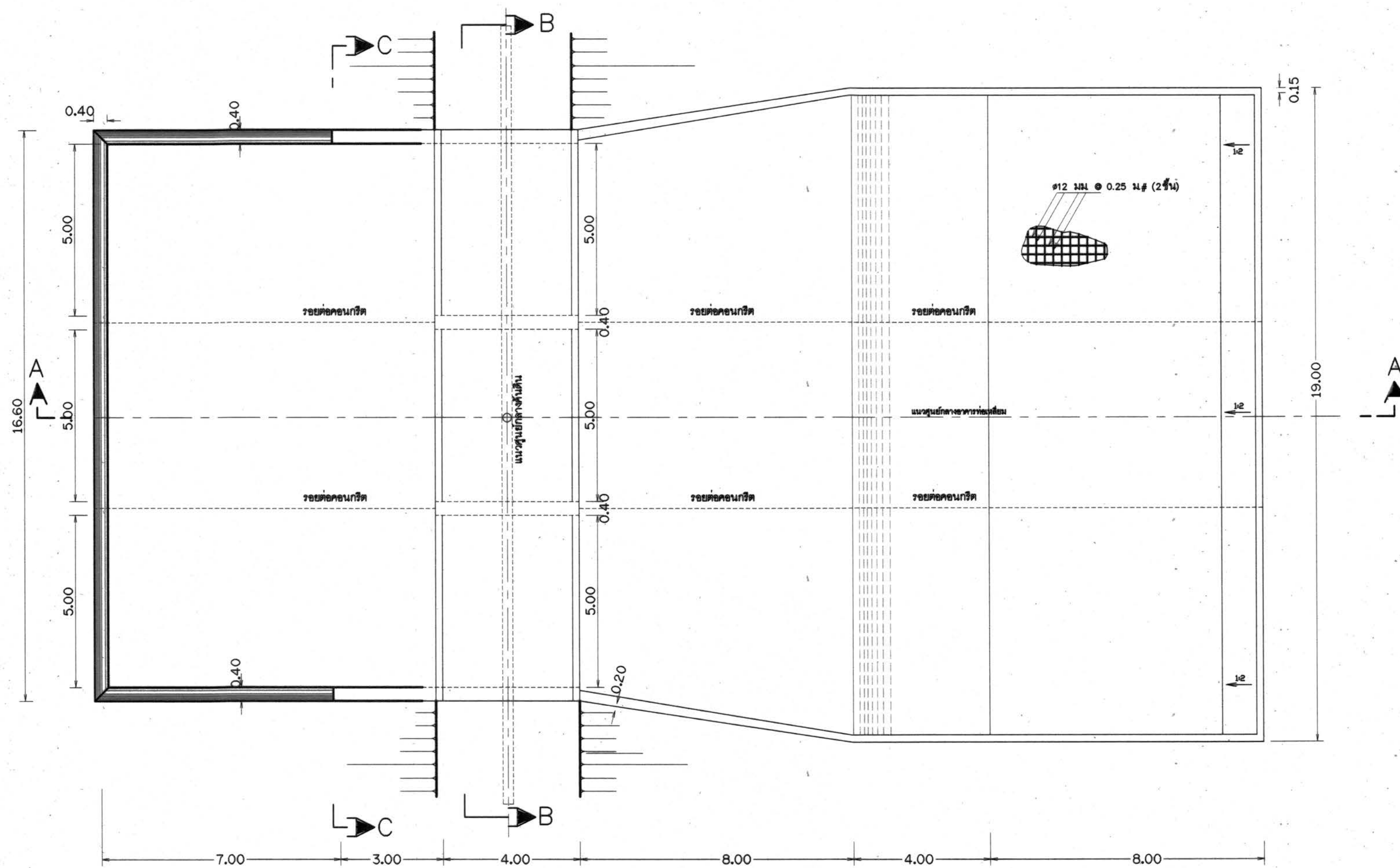
แปลนอาคารระบายน้ำ มาตราส่วน 1:100
