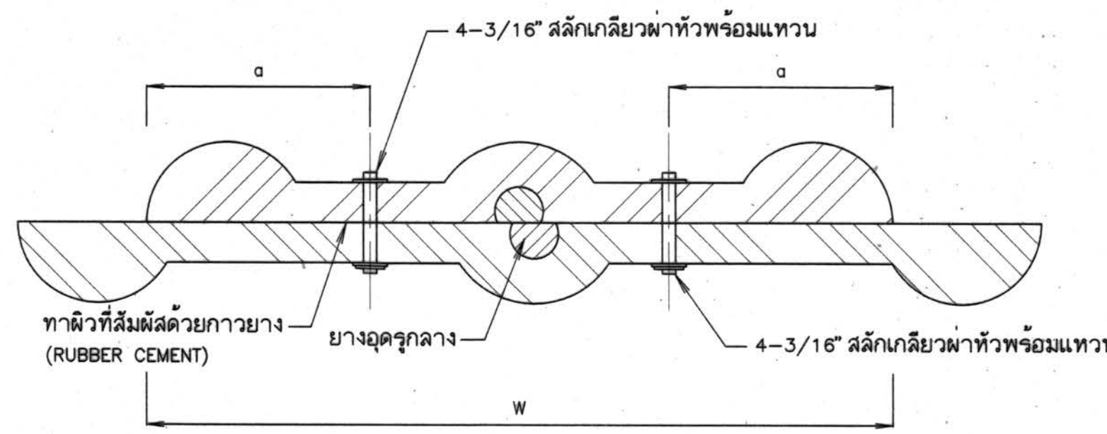
รูปตัด ๖-๖ ไม่แสดงมาตราส่วน
