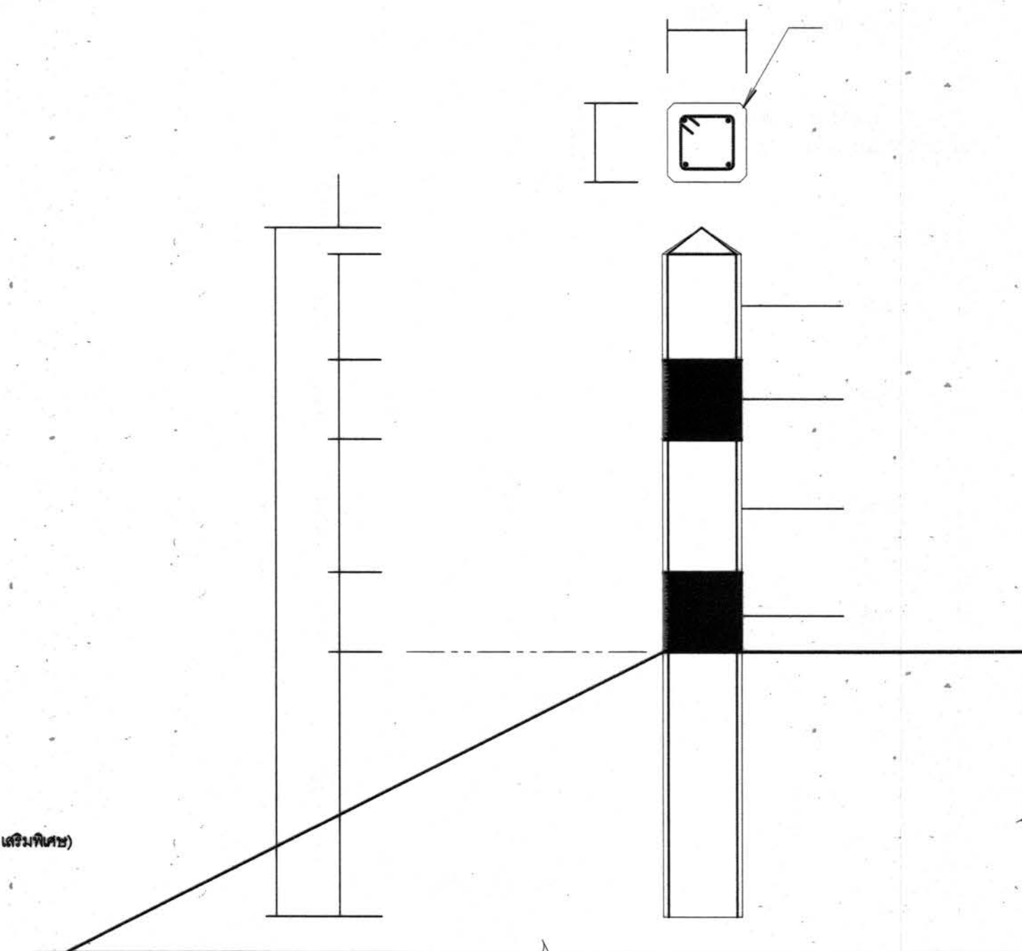
แบบขยายหลักริมคันดิน
