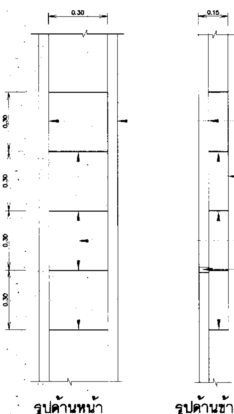
แบบขยายบันได และการยึดท่อน้ำขึ้นและท่อน้ำเข้าถัง มาตราส่วน 1 : 10
