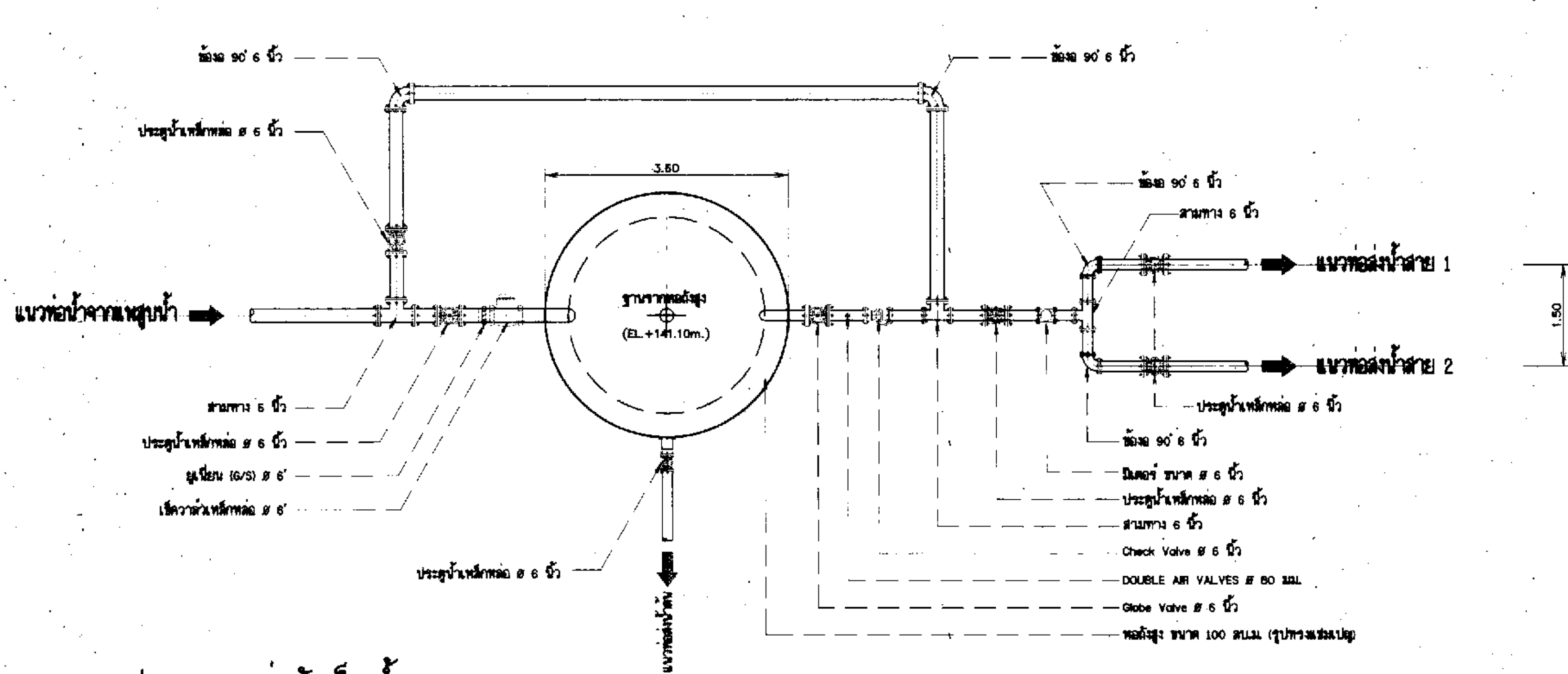
แปลนระบบท่อถึงเก็บน้ำ มาตราส่วน 1:50
