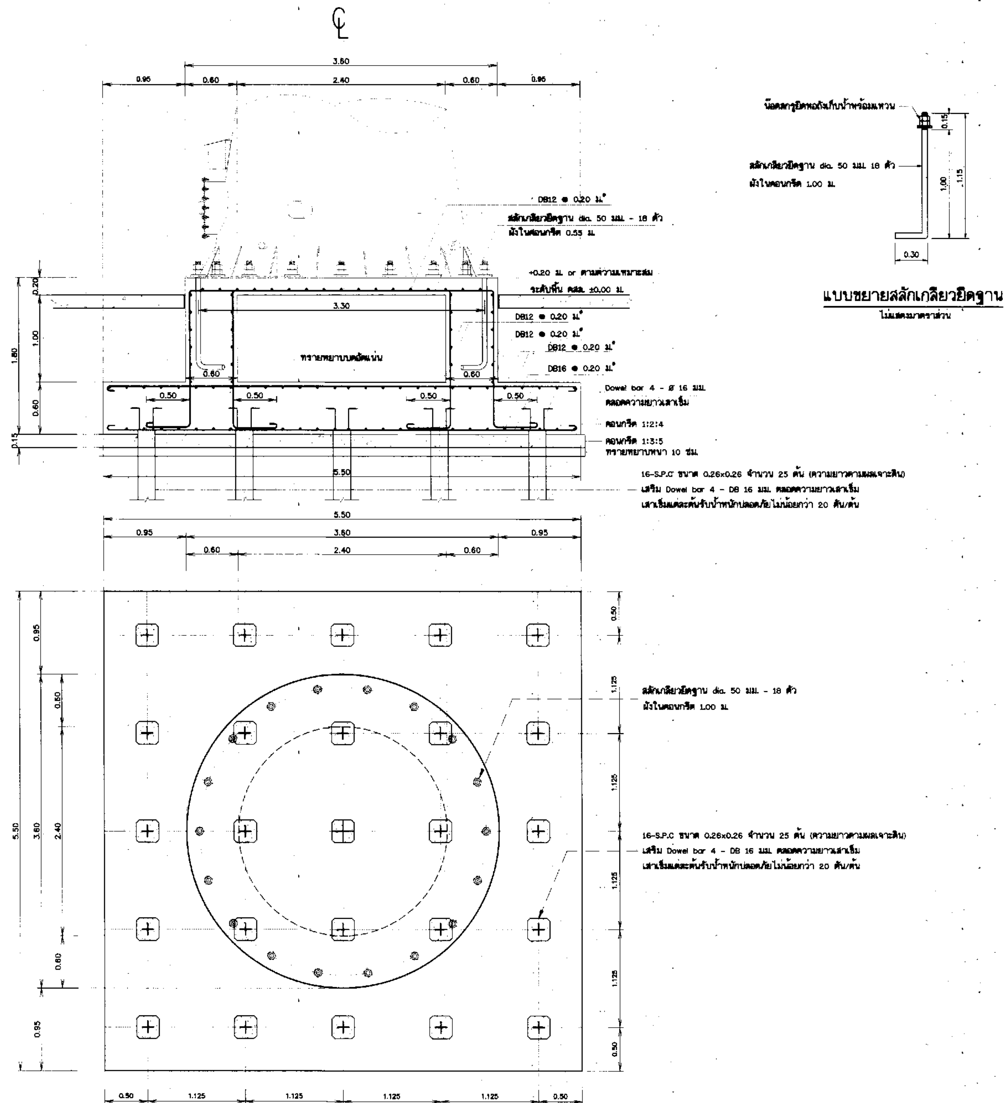
แบบขยายฐานจากท่อถังสูง (แบบเสาเข็ม)
