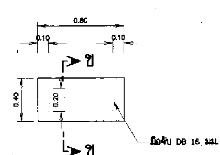
แปลนฝาปิด มาตราส่วน 1:20
