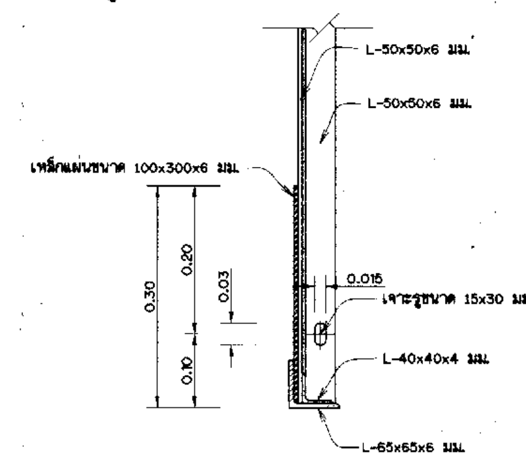
รูปตัด ง-ง
