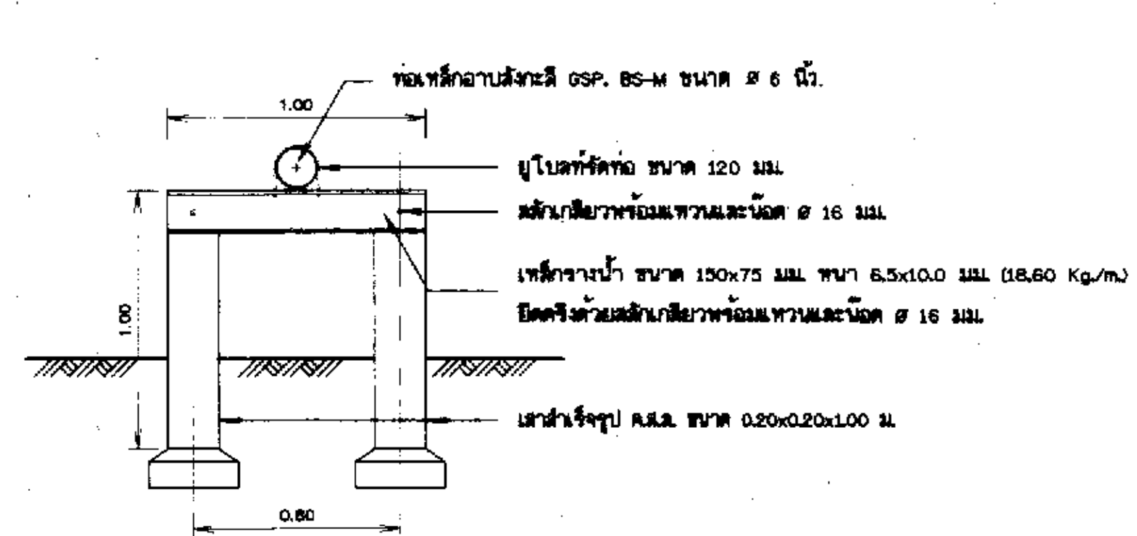
แบบขยายการติดตั้งท่อจุดที่ 2
