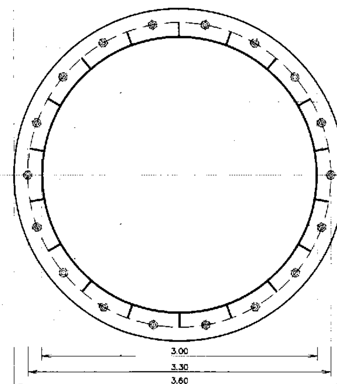
แบบขยายเหล็กแผ่นฐาน
