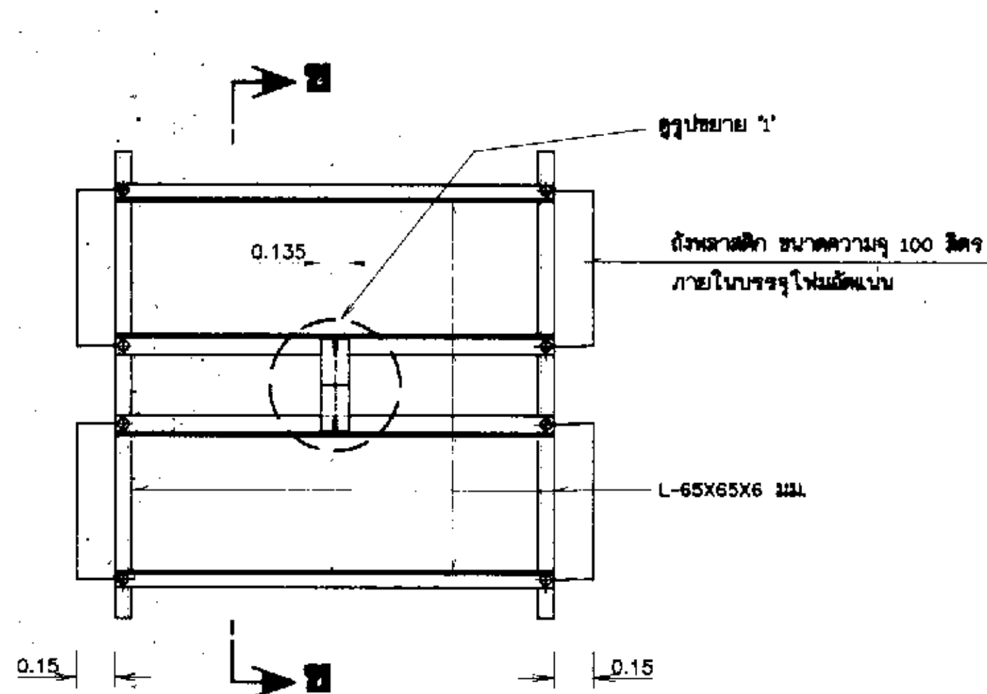
แปลน รายละเอียดฐานวางท่อวางตัวพอน
