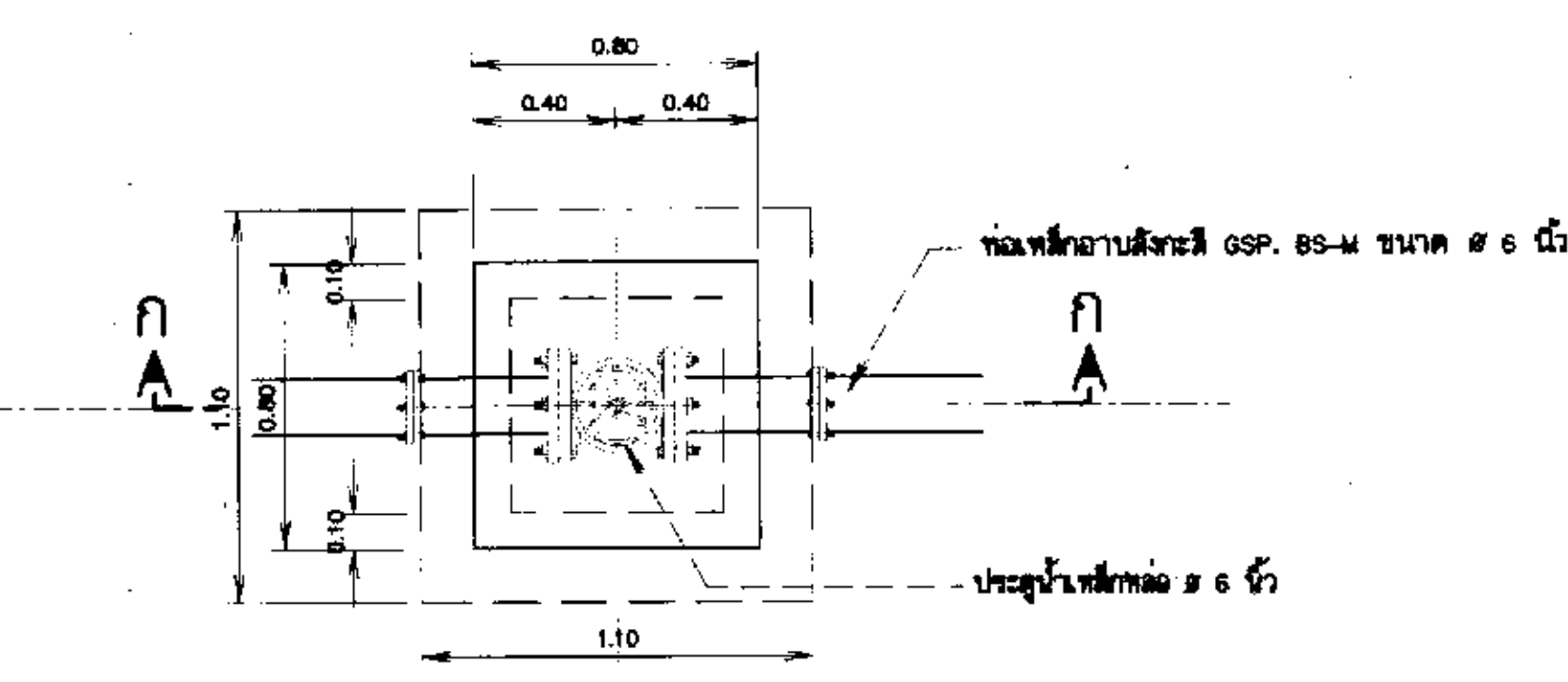
อาคารบ่อประตูปังคังน้ำ มาตราส่วน 1:20
