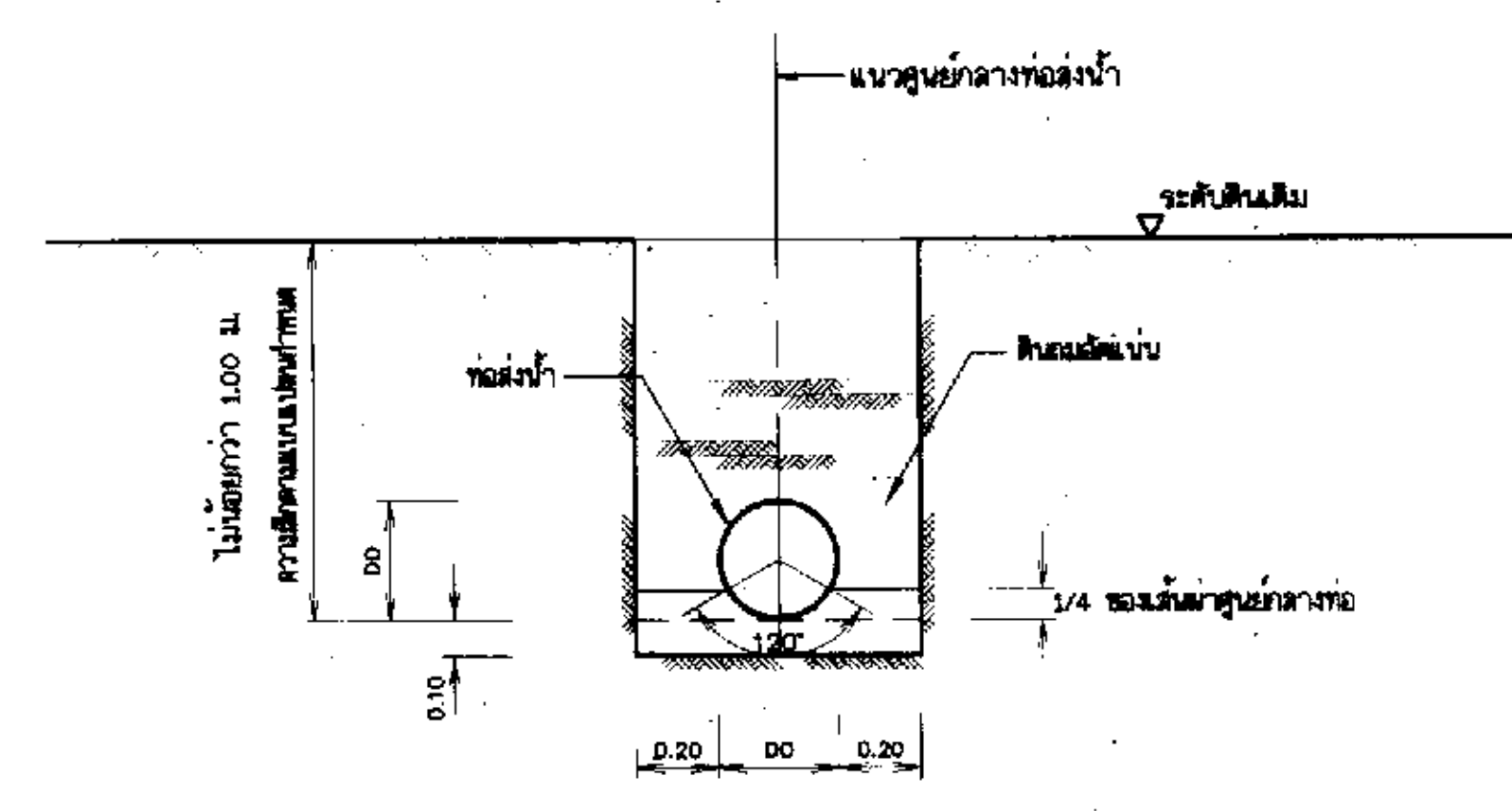
รูปตัดขวางการฝังท่อน้ำดิบ ไม่แสดงมาตราส่วน
