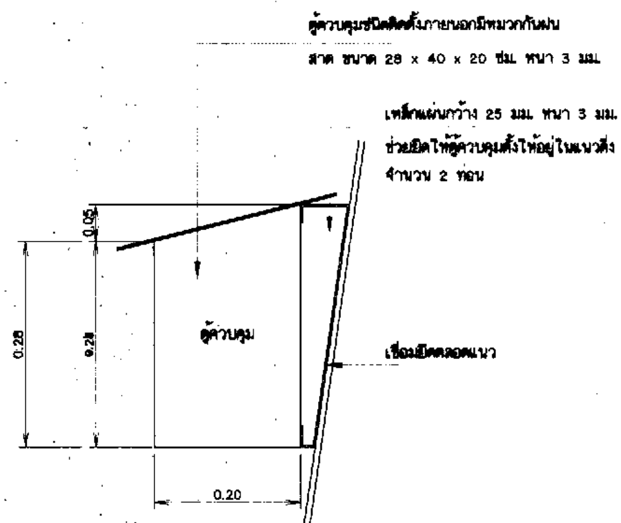
แบบขยายถังเก็บน้ำ มาตราส่วน 1 : 5
