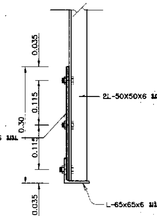
รูปตัด ข - ข
