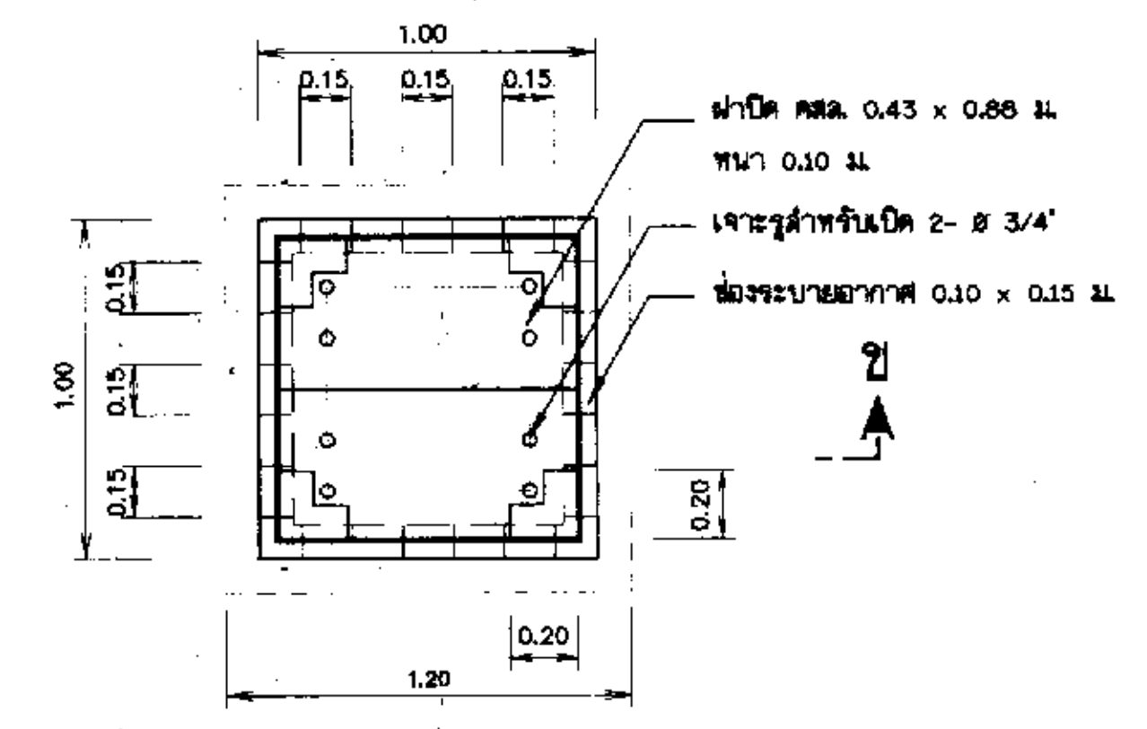
แปลนอาคารทอระบายอากาศ มาตราส่วน 1:20
