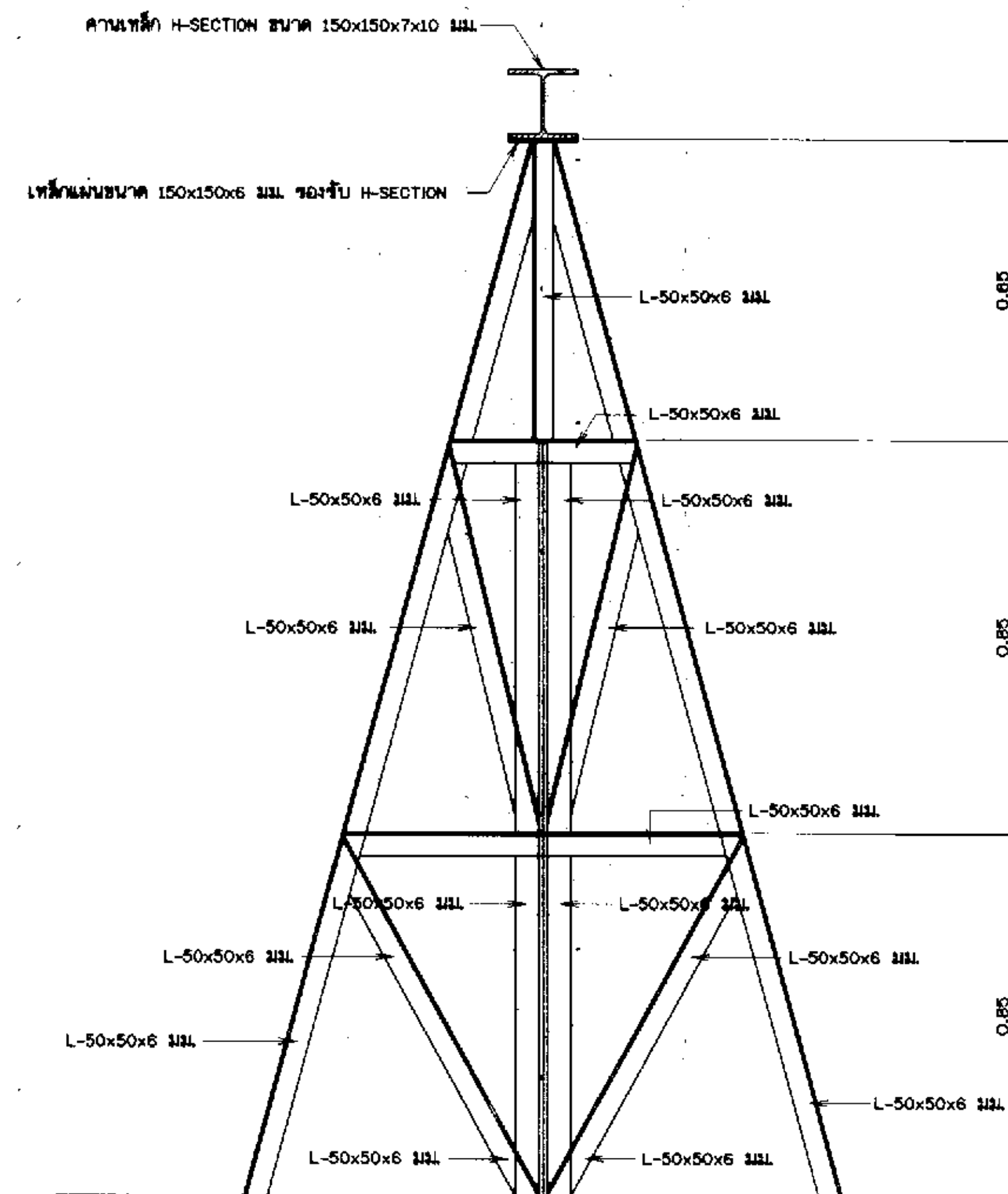
รูปขยายชาตังรูปตัว A รับคานาเหล็ก
