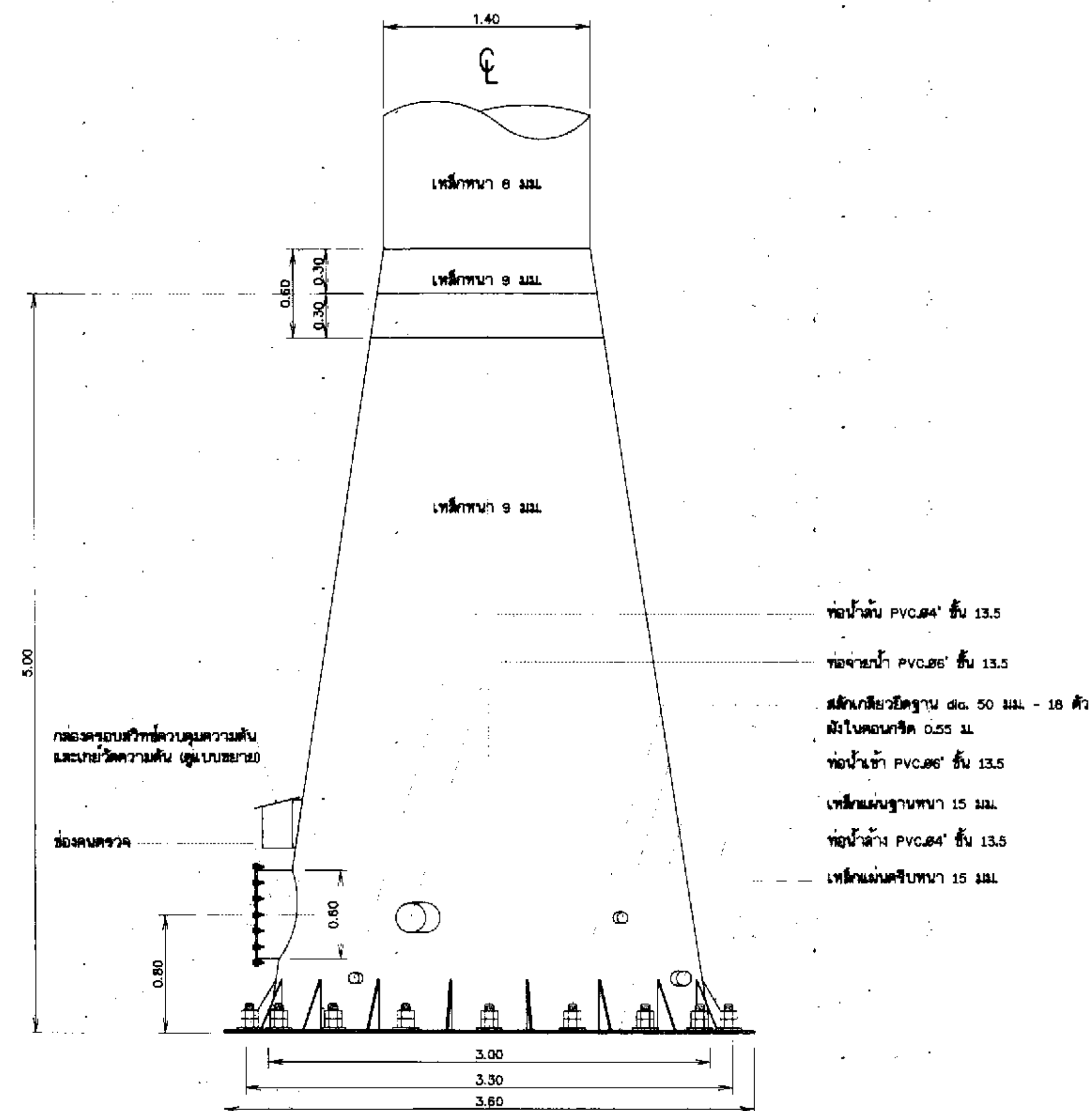
แบบขยายเหล็กแผ่นฐาน
