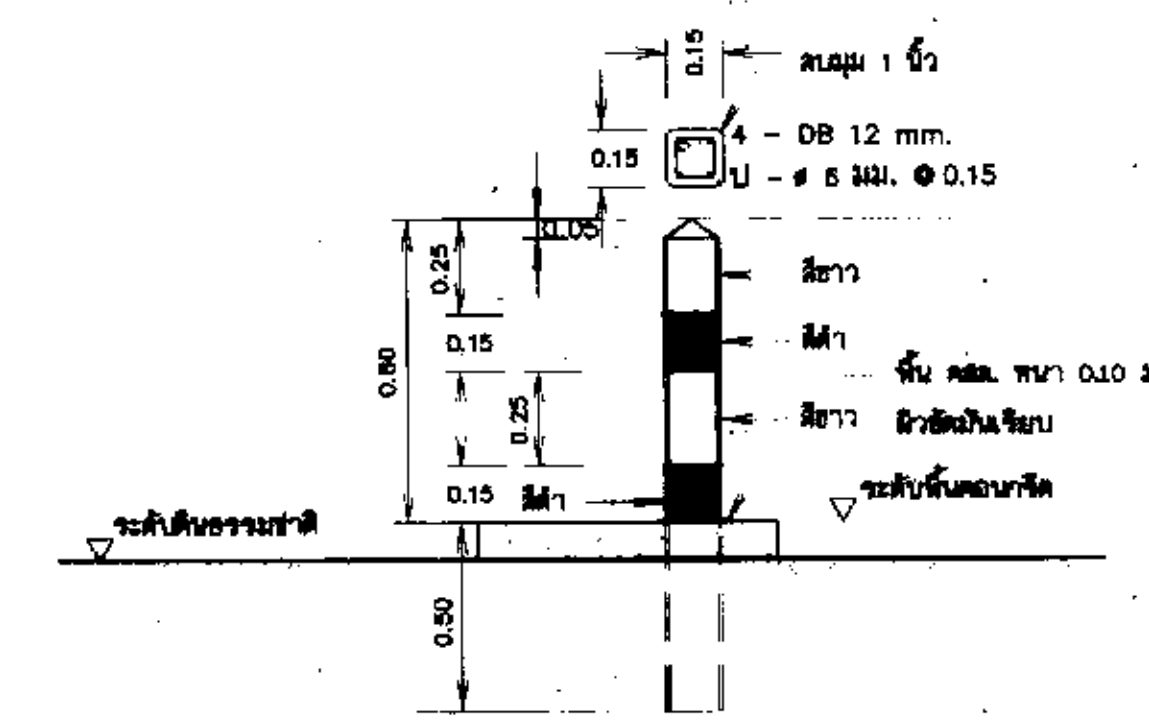
แบบขยาย หลักโค้ง คสล. มาตราส่วน 1:20
