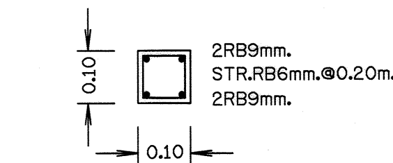
รูปตัด ก - ก มาตรฐาน 1:10
