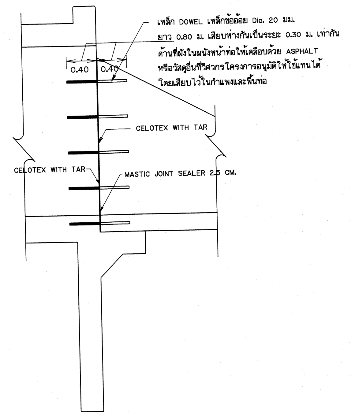
รายละเอียดรอยต่อเพื่อการขยายตัว มาตราส่วน 1:20
