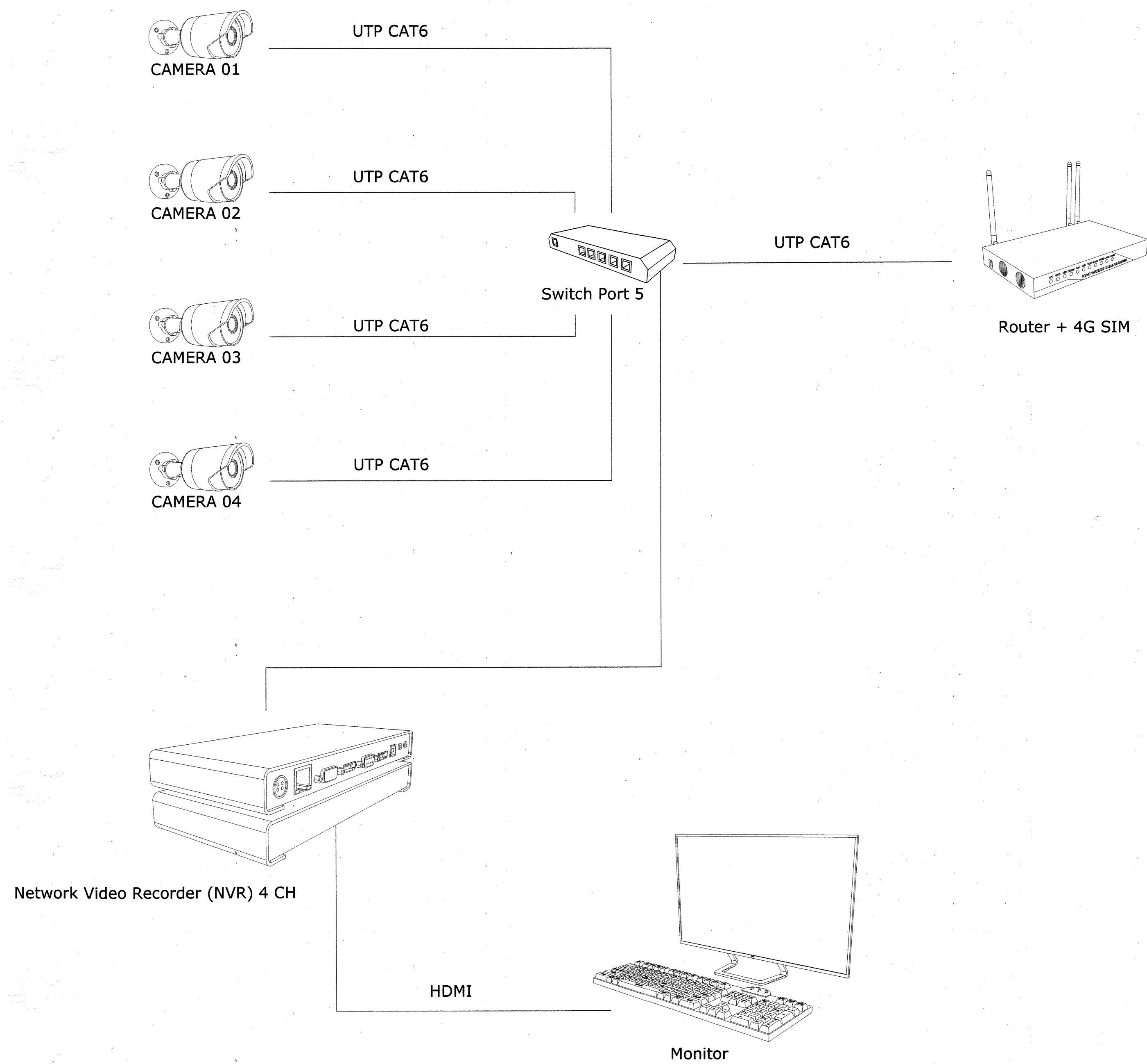
แผนภาพแสดงการติดตั้งกล้องวงจรปิดในบริเวณโครงการ
