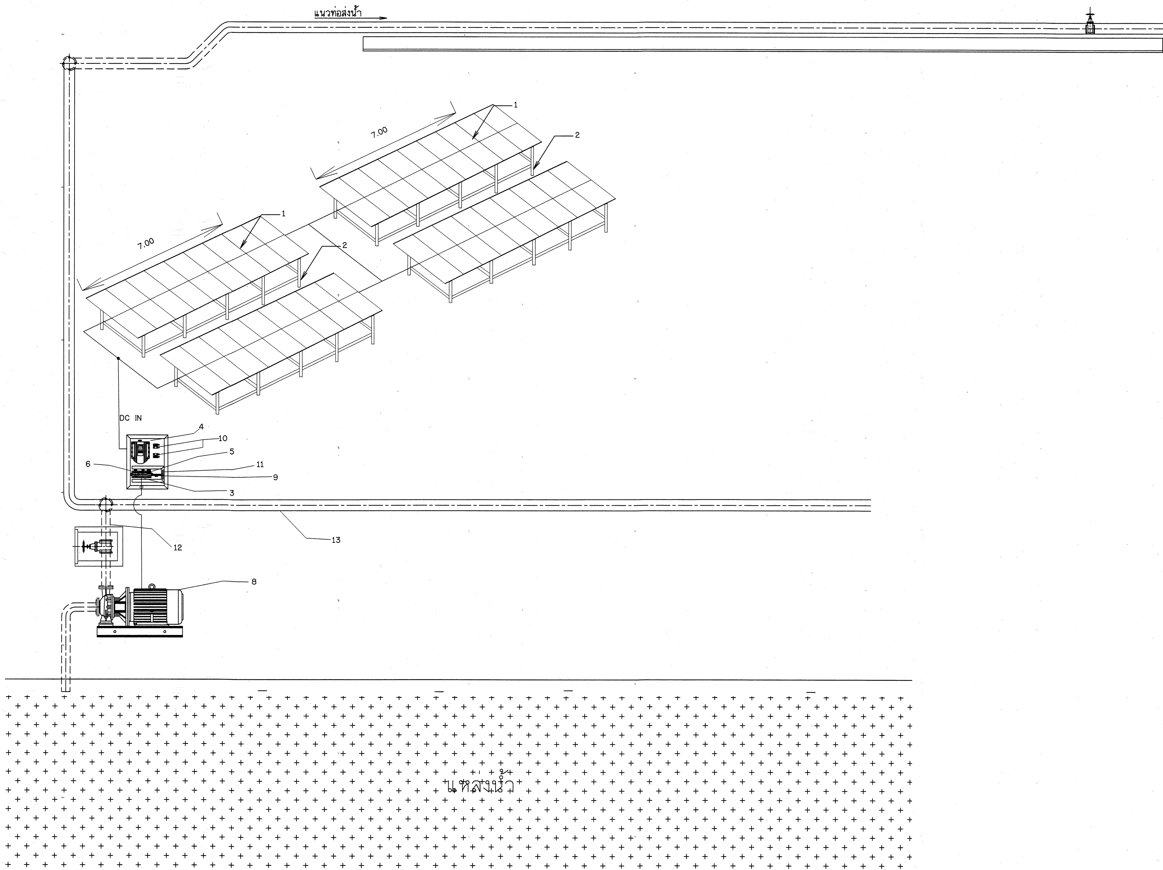
แบบระบบกระจายน้ำด้วยพลังงานแสงอาทิตย์ มาตราส่วน ไม่แสดงมาตราส่วน
