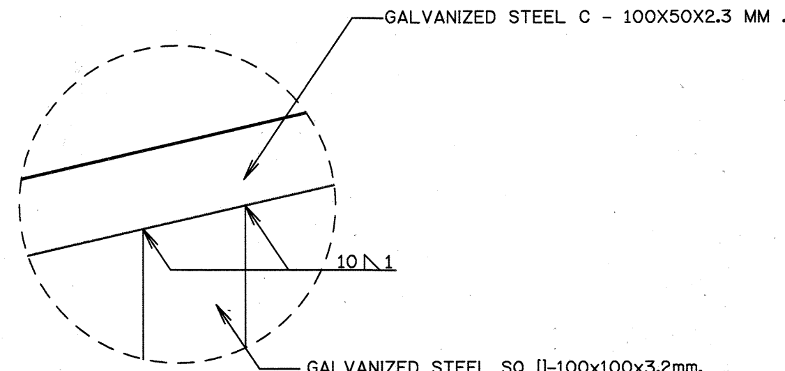
รูปขยาย 2 มาตราส่วน 1:10
