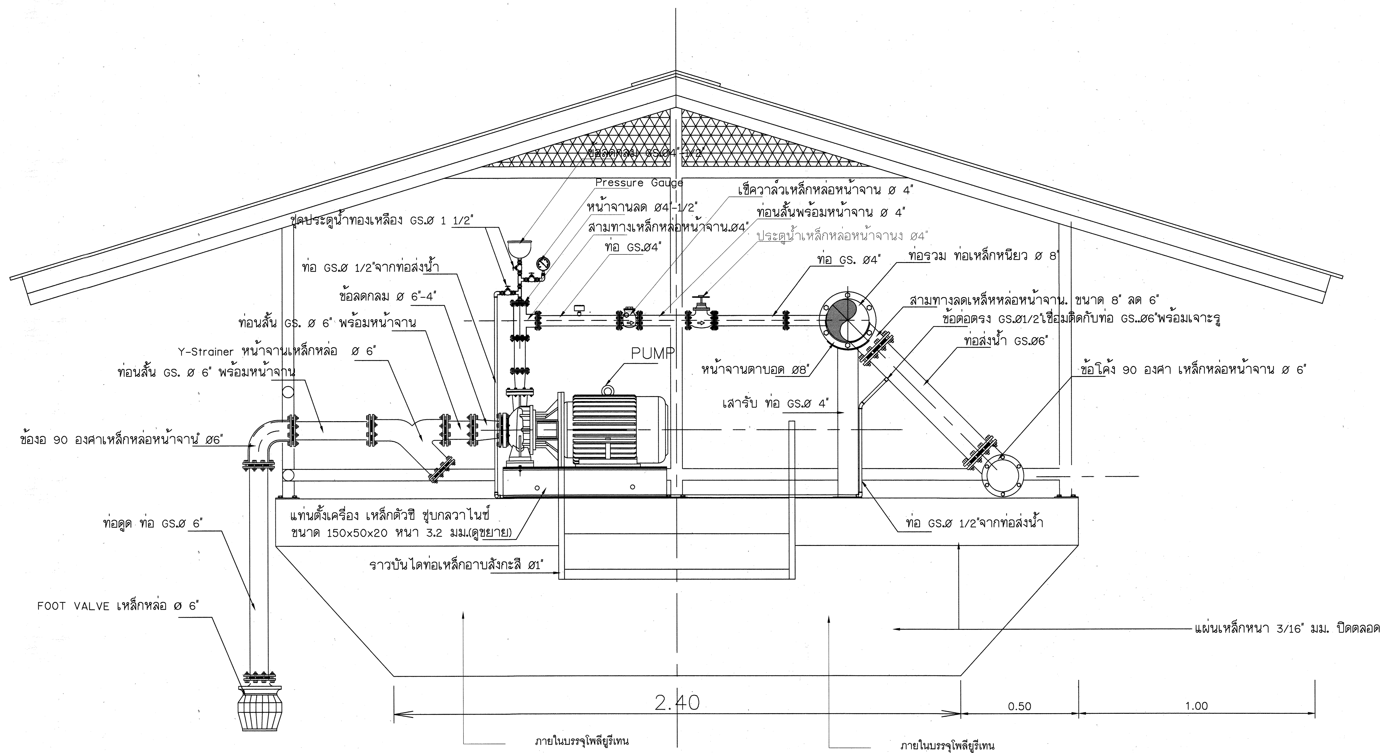
รูปตัดขยายการติดตั้งเครื่องสูบน้ำที่พลอยตัวเดิม ไม่แสดงมาตราส่วน
