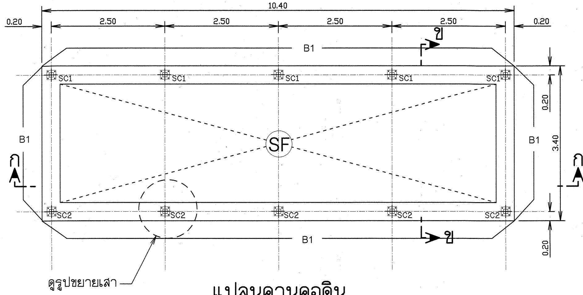
แปลนคานคอดิน
